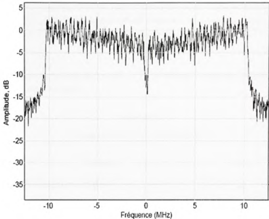
Figure 4.15 Spectre du signal OFDM-16 QAM pondéré par une fenêtre de Hanning pris après le canal pour E_b/N_0 = 30 dB
