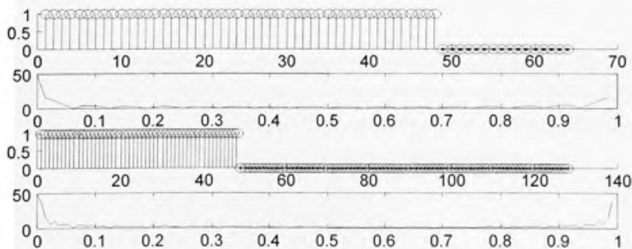
Figure 2.7 FFT de 48 échantillons sur 64, et 128 points
