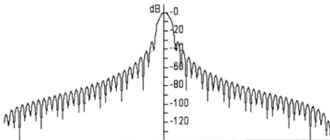
Figure 2.13 FFT de 64 échantillons d'une fenêtre Hanning
