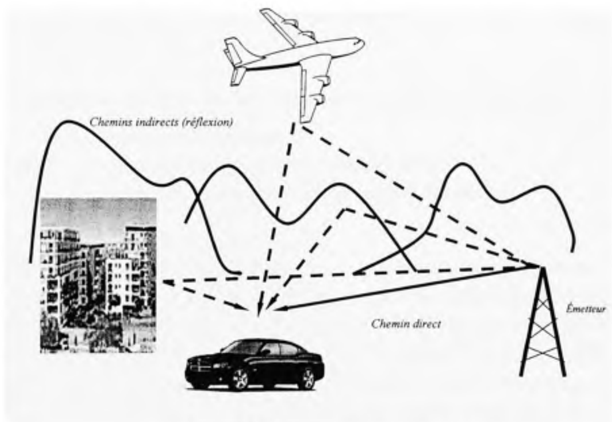
Figure 1.1 Propagation par trajets multiples (Tiré de Nee, Richard Van, 2000)
