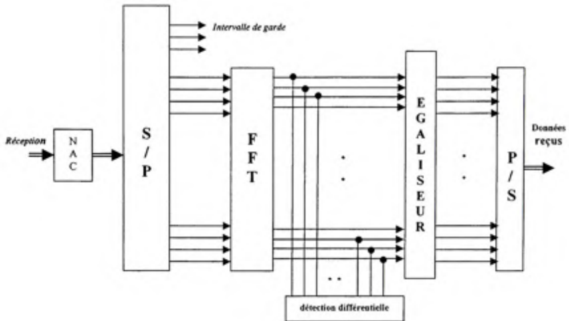
Figure 2.17 Récepteur OFDM avec la détection différentielle
