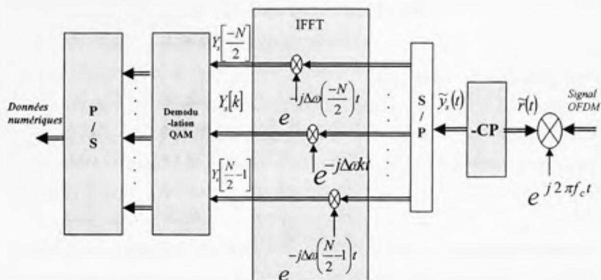
Figure 2.6 Schéma de récepteur du système OFDM
