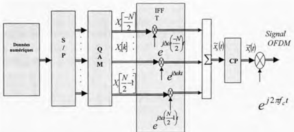
Figure 2.3 Schéma d'émission du système OFDM
