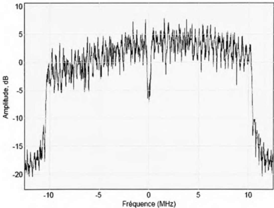
Figure 4.19 Spectre du signal OFDM-64 QAM pondéré par une fenêtre de Hamming pris après le canal pour E_b/N_0 = 30 dB
