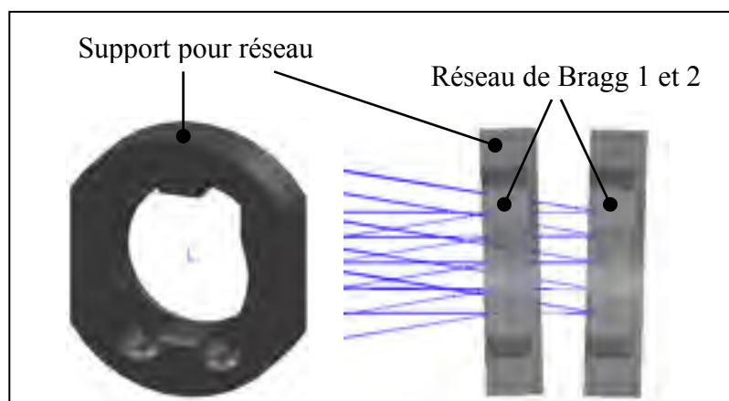
Figure 3.18 Support pour réseaux de Bragg en volume
