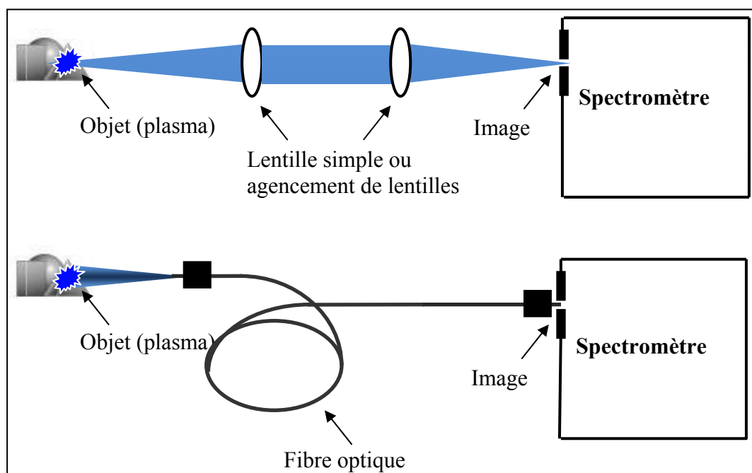
Figure 3.6 Système de collection de la lumière du plasma
