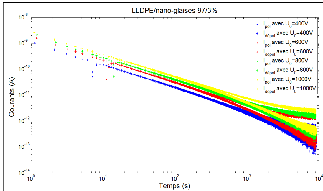
Figure 5.5 Courants de polarisation et de dépolarisation en fonction du temps pour des tensions de polarisation de 400, 600, 800 et 1000V pour du LLDPE/nano-glaises 97/3 %
