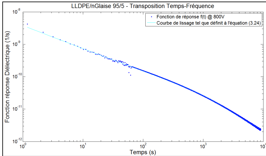
Figure 3.13 Fonction de réponse et sa courbe de lissage tel que défini à l'équation (3.24) en fonction du temps pour un échantillon de LLDPE/nano-glaises 95/5 et une tension continue de 800V
