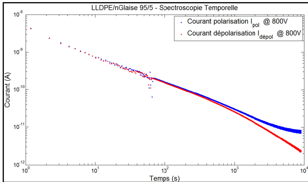
Figure 3.11 Courants de polarisation et de dépolarisation en fonction du temps pour un échantillon de LLDPE/nano-glaises 95/5 et une tension continue de 800V
