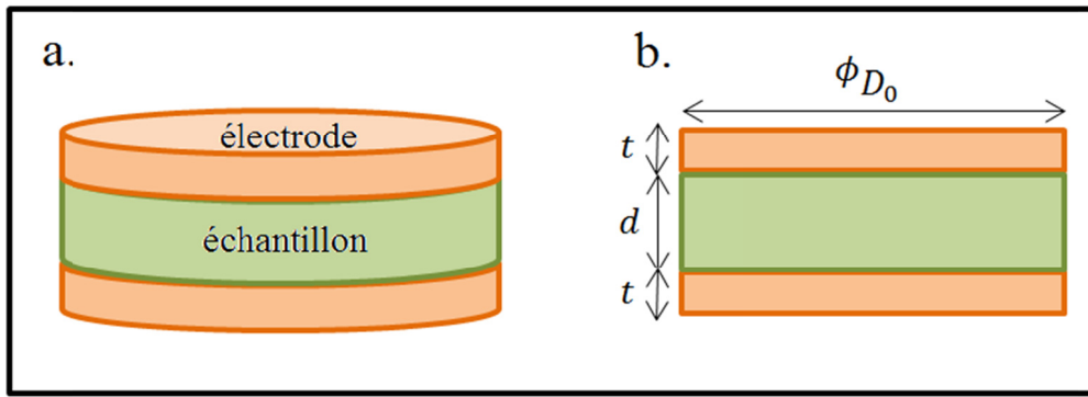
Figure 3.1 Configuration plan-plan a. Représentation spatiale b. Représentation plane
