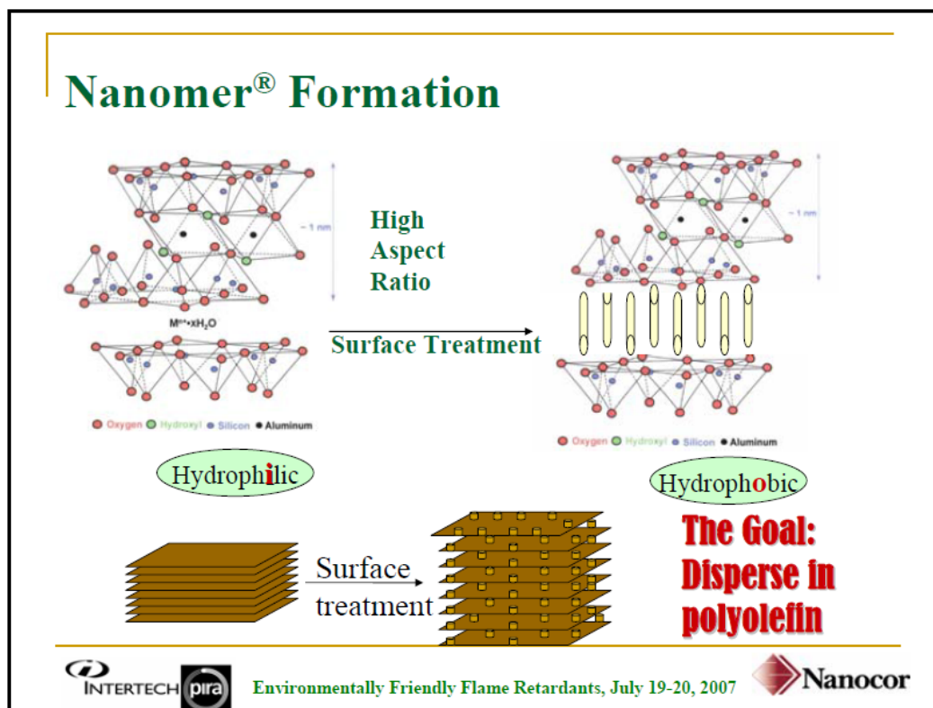
Figure 2.3 Structure moléculaire et traitement de surface des nano-glaises de Nanocor Tirée de Lan (2007a)
