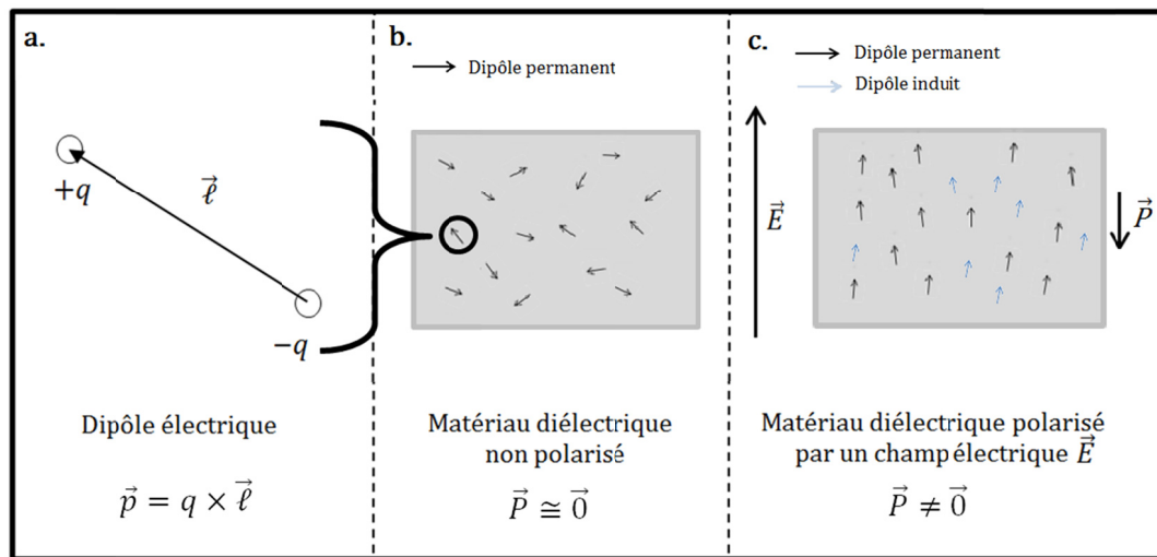
Figure 1.1 Polarisation d'un matériau diélectrique
