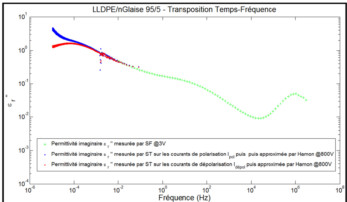
Figure 3.15 Permittivité imaginaire en fonction de la fréquence pour les mesures de spectroscopie fréquentielle (SF) et de spectroscopie temporelle (ST) approximée par Hamon pour les courants de polarisation et de dépolarisation
