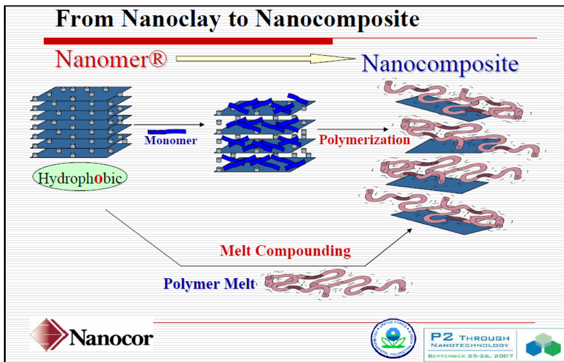
Figure 2.2 Technique de fabrication du mélange-maître nanoMax® de Nanocor Tirée de Lan (2007b)
