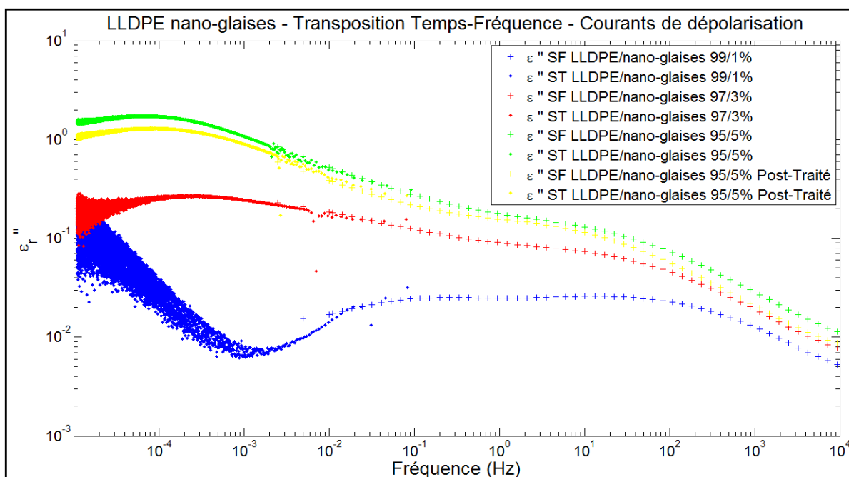
Figure 5.8 Permittivité relative imaginaire en fonction de la fréquence par SF et ST par transposition dans le domaine des fréquences par l'approximation d'Hamon pour les courants de dépolarisation pour des nanodiélectriques LLDPE/nano-glaises de composition massiques 1, 3, 5 % ainsi que 5% post-traité
