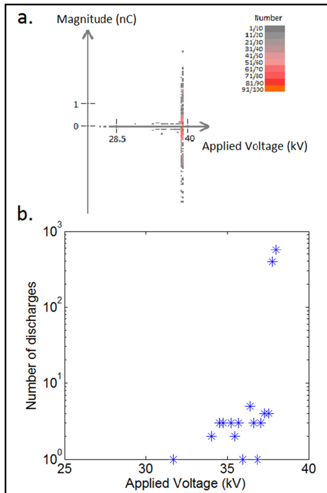
Figure 4.3 Décharges partielles en fonction de la tension appliquée
