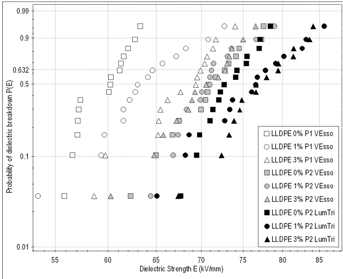
Figure 4.2 Probabilité cumulative de rupture diélectrique P(E) en fonction du champ électrique E représentée sur diagramme de probabilité Weibull
