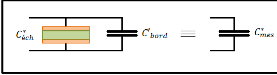
Figure 3.4 Représentation sous forme de circuit électrique de l'effet de bord
