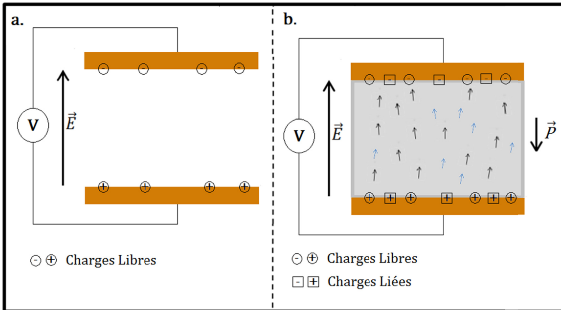
Figure 1.3 Charges sur les armatures d'un condensateur a. Dans le vide b. Avec un matériau diélectrique
