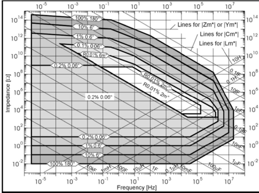
Figure 3.3 Spécification de la précision de l'analyseur de réponse fréquentielle Alpha-A de Novocontrol Tirée de Novocontrol Technologies (2010)
