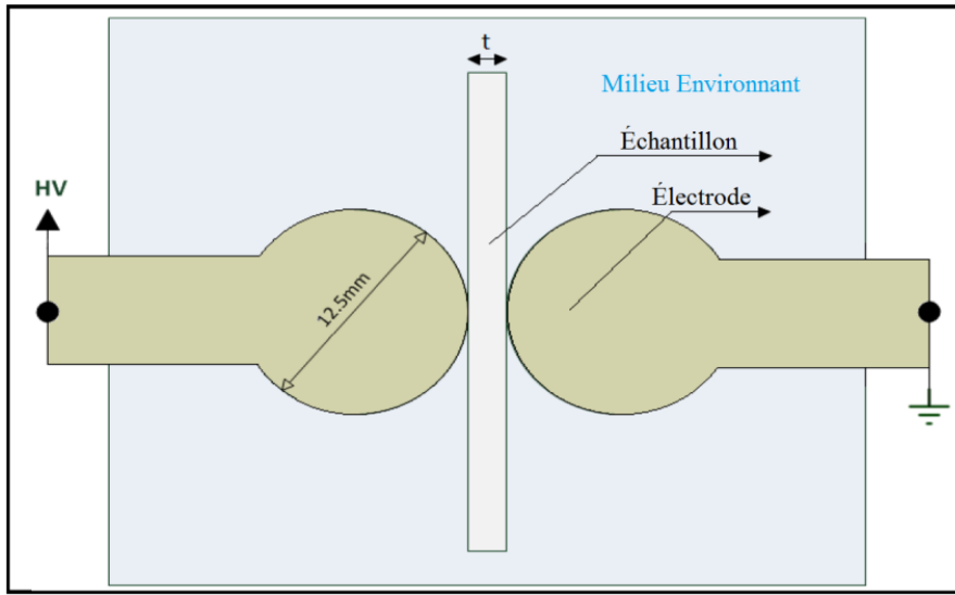
Figure 4.1 Configuration d'une mesure de rigidité diélectrique
