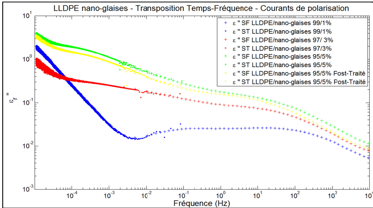
Figure 5.7 Permittivité relative imaginaire en fonction de la fréquence par SF et ST par transposition dans le domaine des fréquences par l'approximation d'Hamon pour les courants de polarisation pour des nanodiélectriques LLDPE/nano-glaises de composition massiques 1, 3, 5 % ainsi que 5% post-traité
