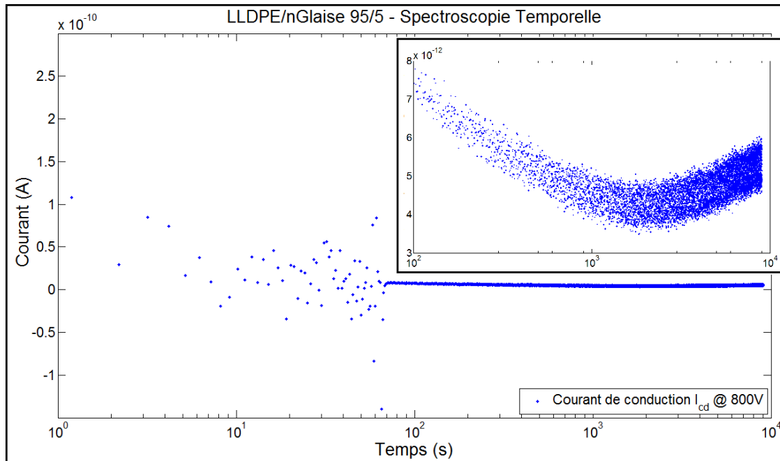
Figure 3.12 Courants de conduction en fonction du temps pour un échantillon de LLDPE/nano-glaises 95/5 et une tension continue de 800V
