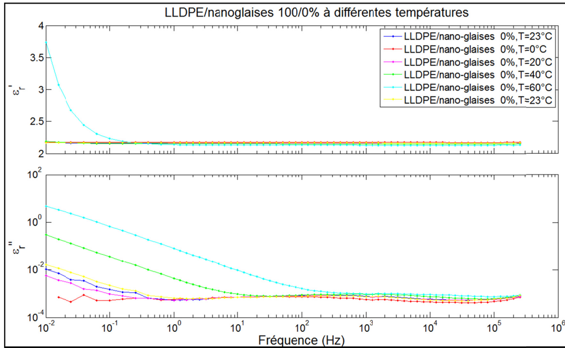
Figure 5.1 Permittivités relative réelle \varepsilon_r' et imaginaire \varepsilon_r'' en fonction de la fréquence pour un échantillon référence de LLDPE pur et à différentes températures
