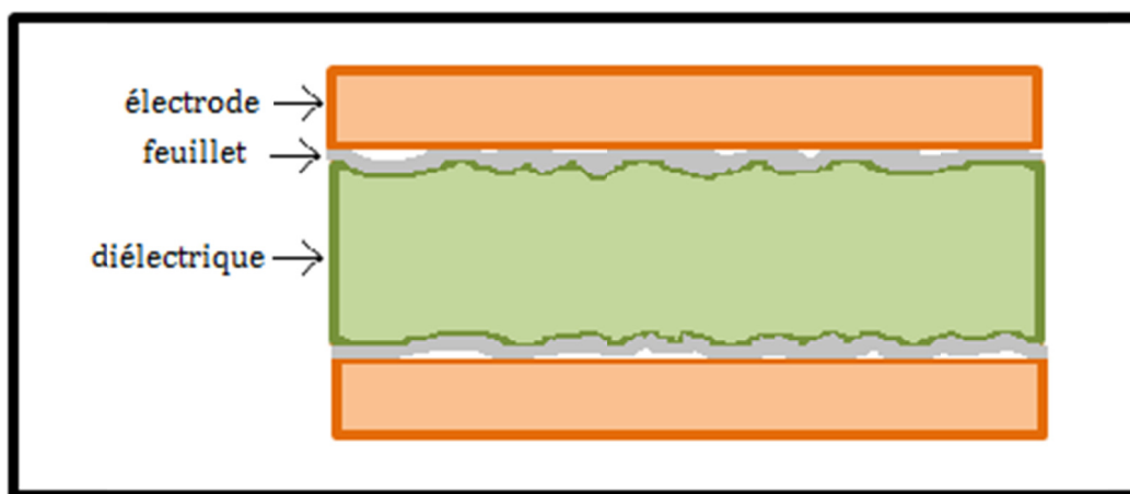
Figure 3.7 Représentation schématique de l'utilisation de feuillets conducteurs
