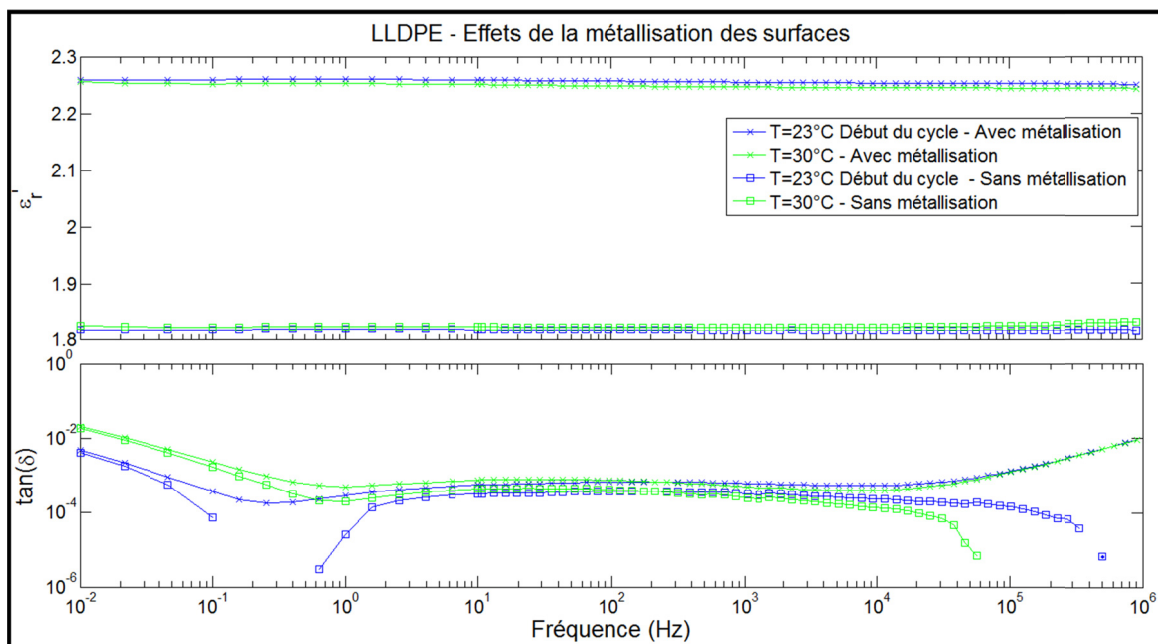
Figure 3.8 Comparaison de l'effet de la métallisation des surfaces sur la permittivité réelle et la tangente de perte mesurées pour du LLDPE 100% aux températures de 23^{\circ}\text{C} et 30^{\circ}\text{C}
