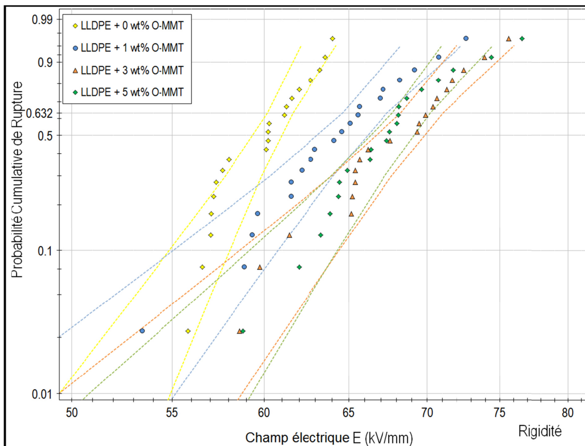
Figure 6.1 Probabilité cumulative de rupture diélectrique P(E) en fonction du champ électrique E représentée sur diagramme de probabilité Weibull pour du LLDPE avec 0, 1, 3 et 5% en nano-glaises
