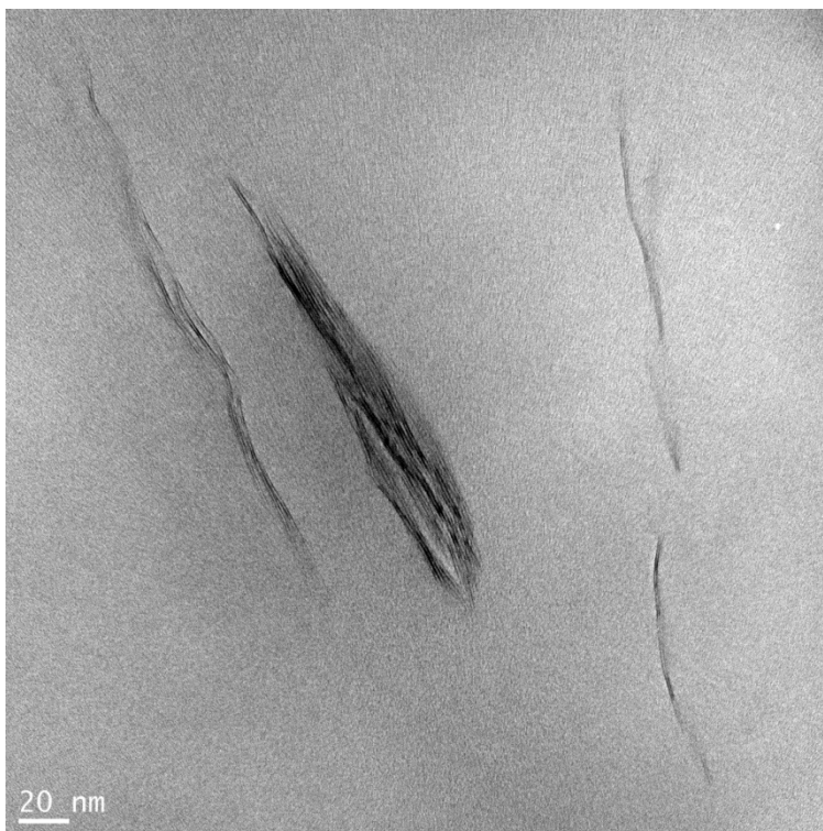
Figure 2.6 Image TEM à 20nm d'un échantillon LLDPE/nano-glaises 97/3 %
