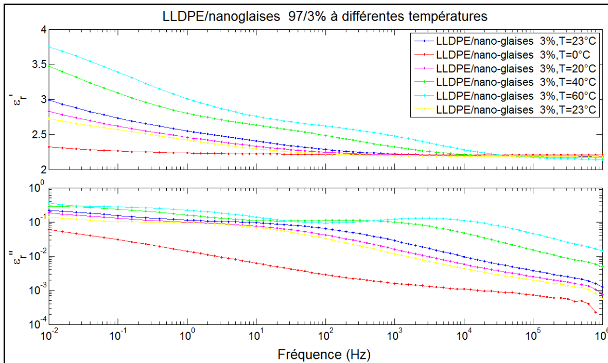
Figure 5.2 Permittivités relative réelle \epsilon'_r et imaginaire \epsilon''_r en fonction de la fréquence pour un échantillon LLDPE/nano-glaises 97/3 et à différentes températures
