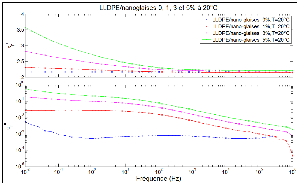
Figure 5.3 Permittivités relatives réelles et imaginaires en fonction de la fréquence des nanodiélectriques LLDPE 0, 1, 3 et 5% à 20°C
