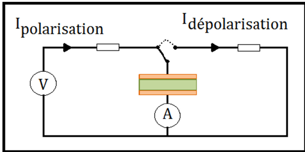
Figure 3.10 Représentation schématique d'un montage de spectroscopie diélectrique
