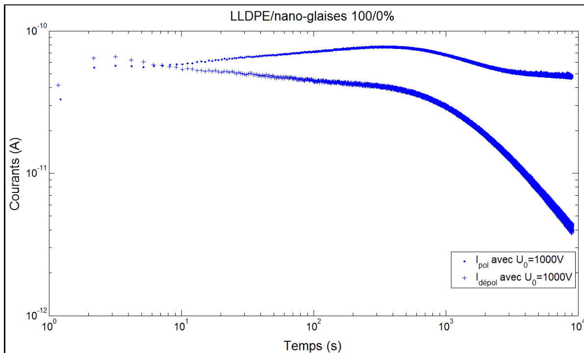
Figure 5.6 Courants de polarisation et de dépolarisation en fonction du temps et pour une tension de polarisation de 1000V pour du LLDPE/nano-glaises 100/0 %
