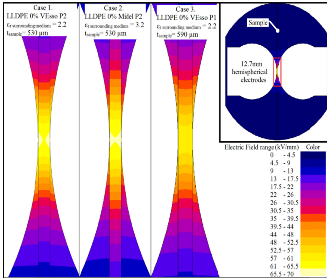
Figure 4.4 Modélisation de la distribution du champ électrique. L'inlet représente la configuration de la modélisation et la figure représente trois cas agrandis correspondant à la zone encadrée de rouge au centre des électrodes
