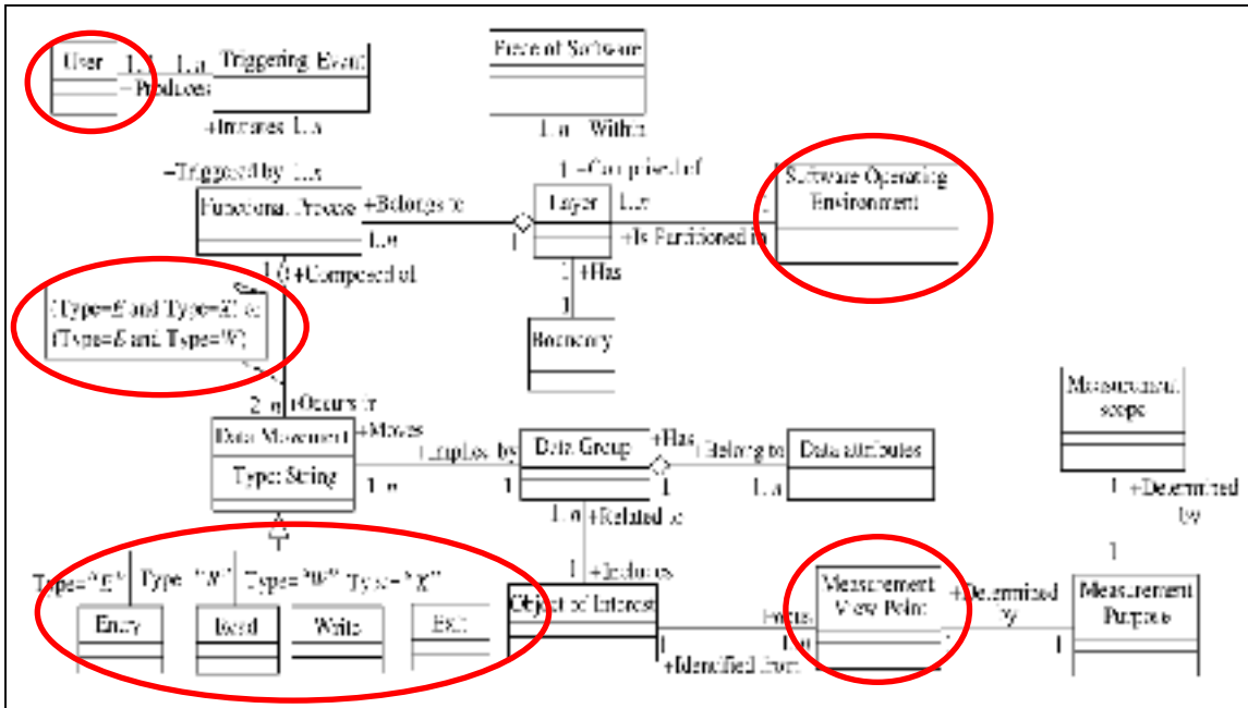
Figure 4.1 Méta-Modèle COSMIC tiré de Condori-Fernandèz et al. (2007)
