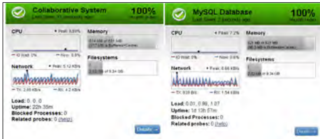
Figure 5.7 État global des conteneurs du système
