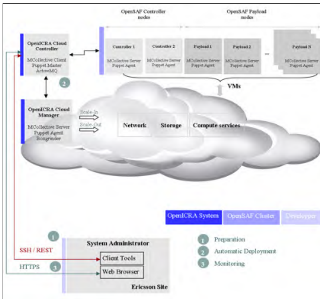
Figure 5.1 Processus de déploiement de l'intergiciel OpenSAF
