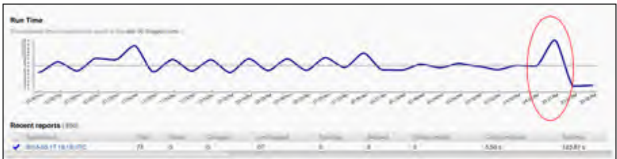
Figure 5.3 Temps d’exécution du démon Puppet dans le nœud du contrôleur
