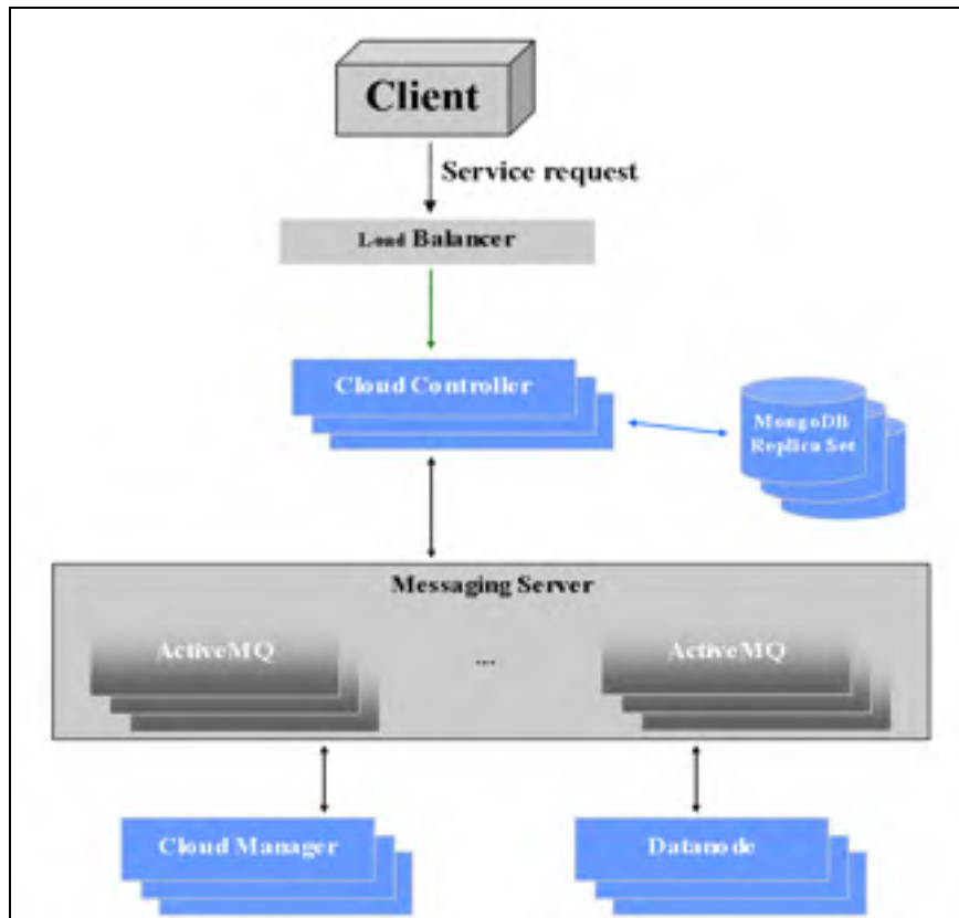
Figure 3.1 Architecture proposée avec une redondance des principaux composants
