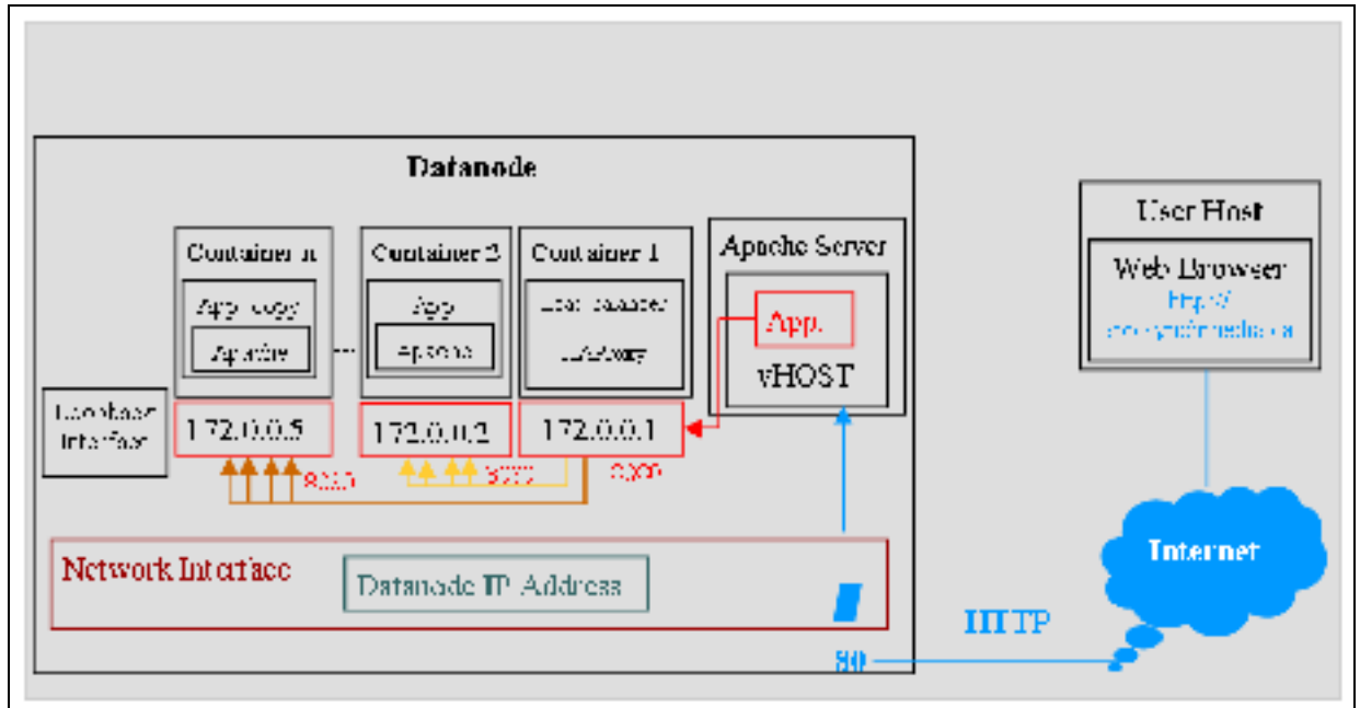
Figure 3.2 Mise à l'échelle automatique : Communication TCP inter-conteneur
