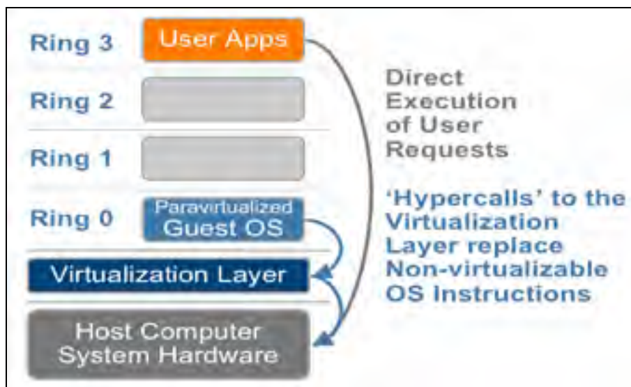
Figure 2.9 Approche de la paravirtualisation Tirée de VMware (2007)
