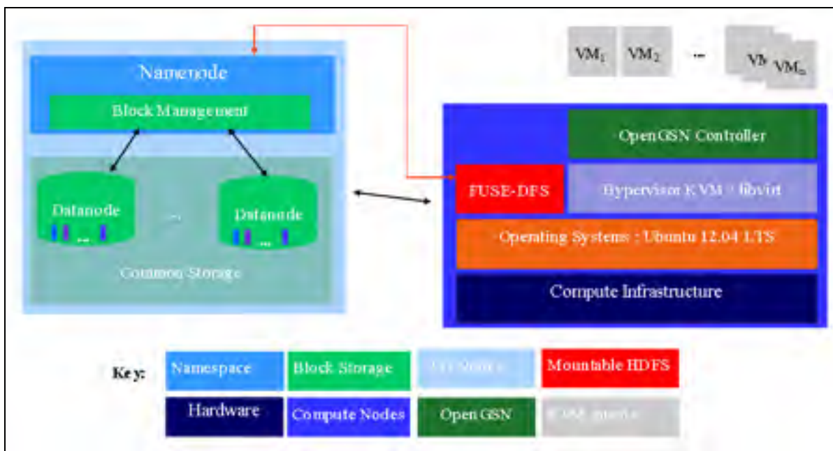
Figure 3.5 Intégration du système de fichiers distribué HDFS avec le réseau GSN
