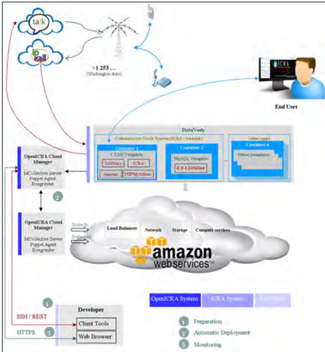
Figure 5.6 Architecture globale du système collaboratif ICRA
