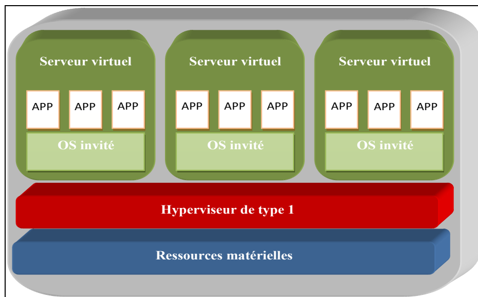
Figure 2.1 Hyperviseur de type 1
