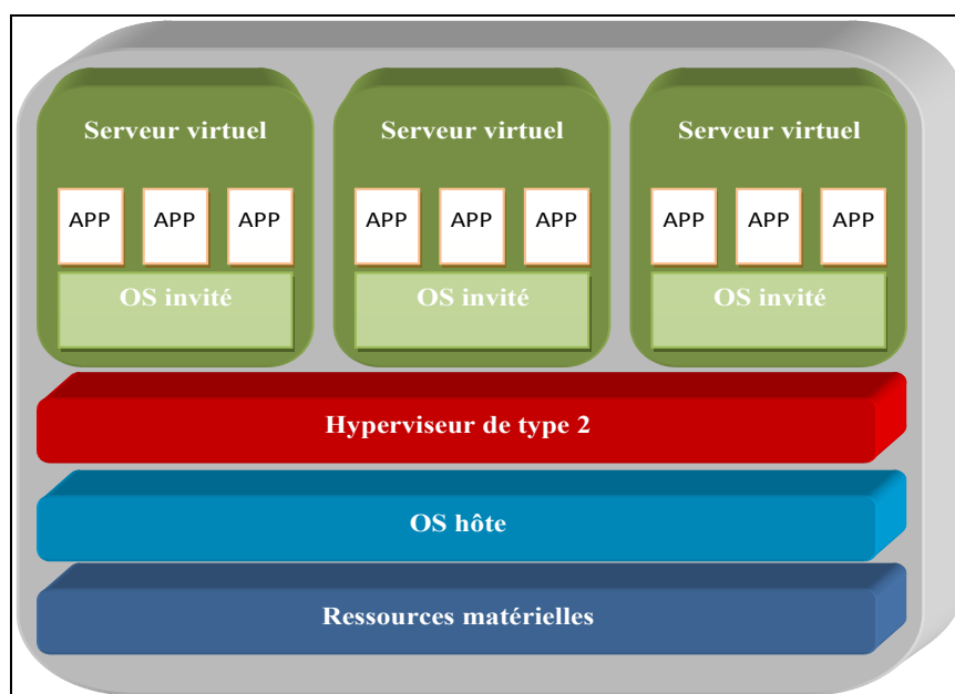
Figure 2.2 Hyperviseur de type 2
