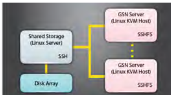
Figure 3.3 Système de stockage actuel de GSN Tirée de GSN Middleware Team (2011)
