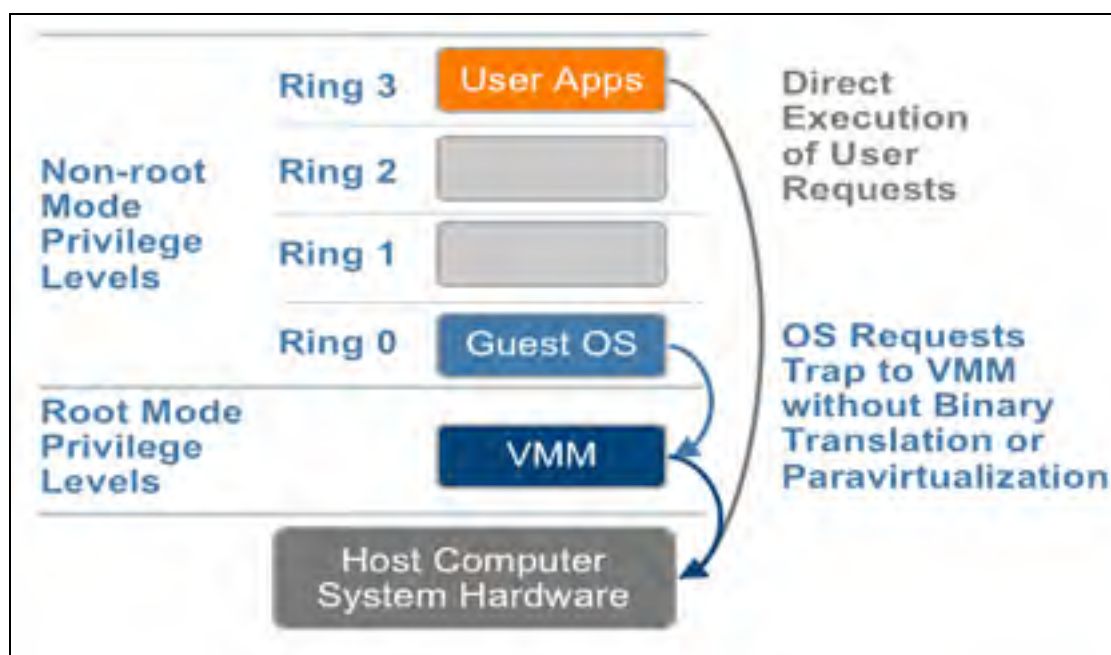
Figure 2.10 Approche de la virtualisation assistée par matériel Tirée de VMware (2007)
