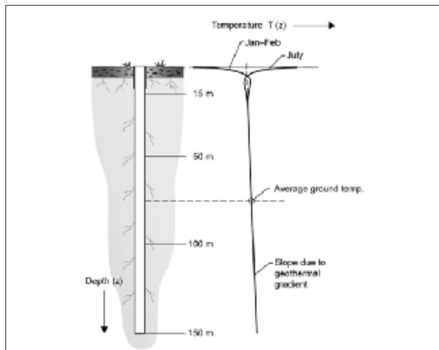
Figure 1.3 Le profil de température dans le sol. Tiré de (Gehlin, 1998a)
