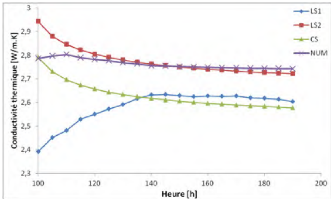
Figure 5.31 La conductivité thermique estimée avec les différentes méthodes. Le premier point est fixé, le dernier point varie avec les données enregistrées.
