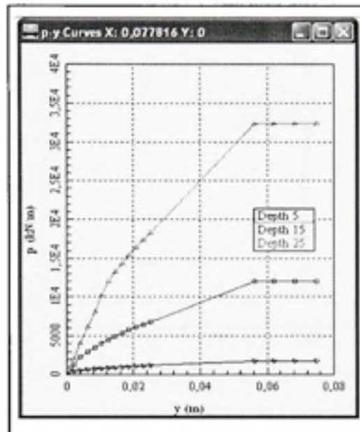
Figure VI.1 Courbes P - y .
