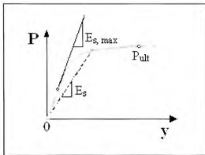
Figure 3.12 Courbe ( P-y ) incluant P_{ult} et E_s (Adapté de Reese et al., 2006)
