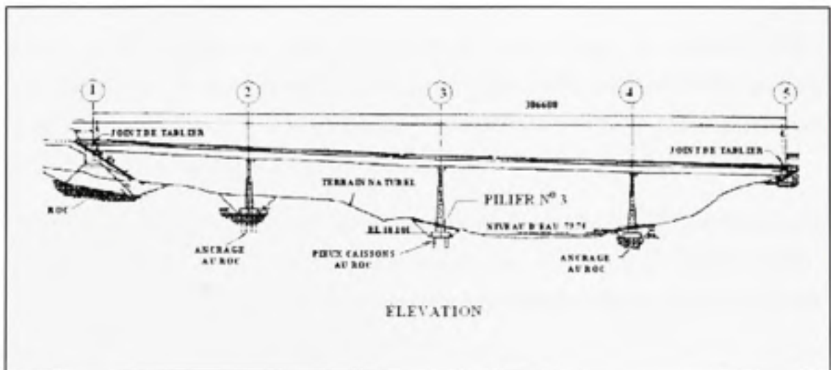
Figure 4.1 Plan en élévation.
