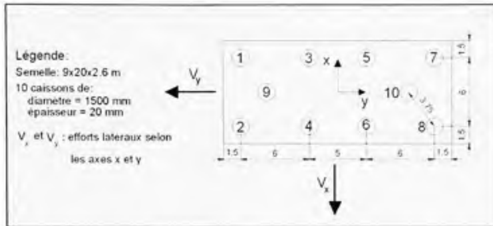
Figure 4.2 Description de la semelle avec la disposition des dix caissons.
