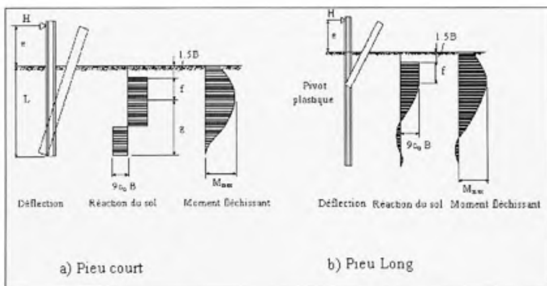
Figure 3.4 Mécanismes de rupture pour un pieu libre en tête sous charge latérale dans un sol cohérent. (Adapté de Broms, 1964a)
