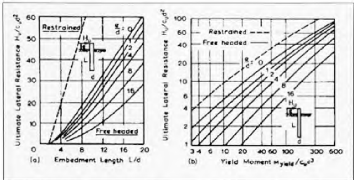
Figure 3.8 Résistance latérale ultime : a) pieu rigide et b) pieu souple dans un sol cohérent selon Broms (1964a). (Tiré de Poulos et Davis, 1980)
