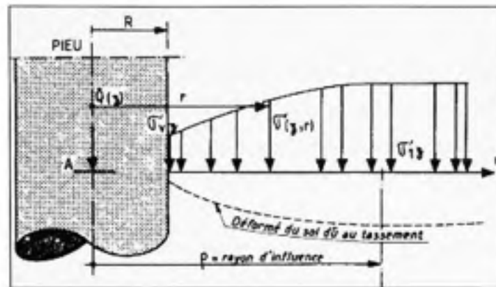
Figure 2.18 Effet d'accrochage. (Tiré de Philipponnat et Hubert, 1998)
