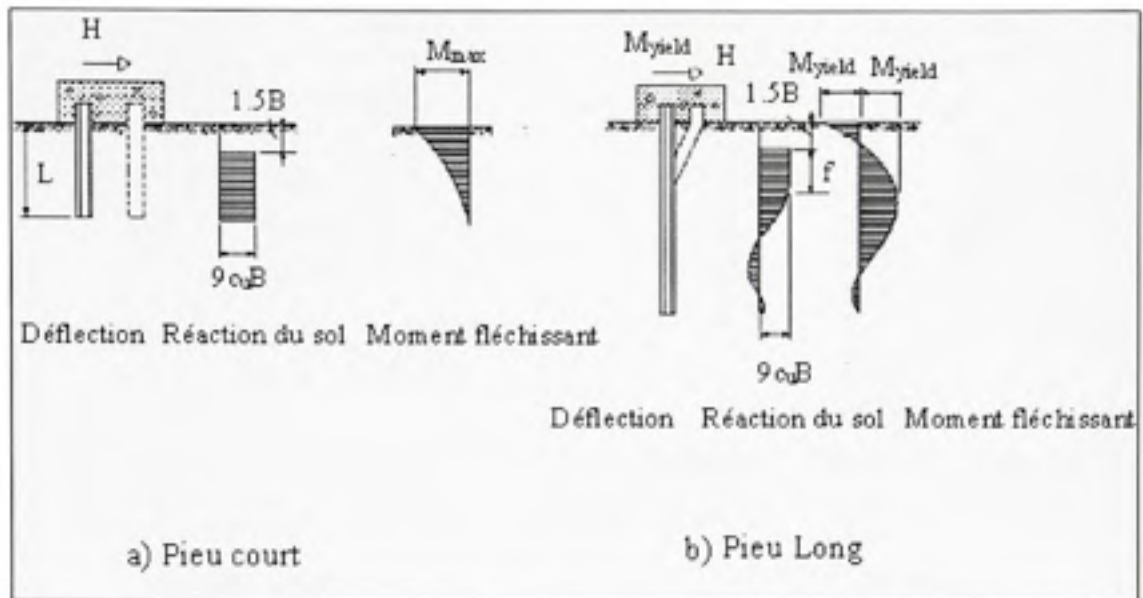
Figure 3.5 Mécanismes de ruptures pour un pieu fixe en tête sous charge latérale dans un sol cohérent. (Adapté de Broms, 1964a)
