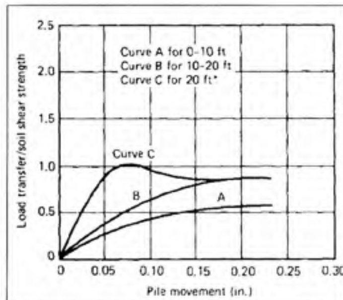
Figure 2.25 Courbes de transfert pour les pieux tubulaires dans l'argile. (Modèle de Coyle et Reese, 1966)
