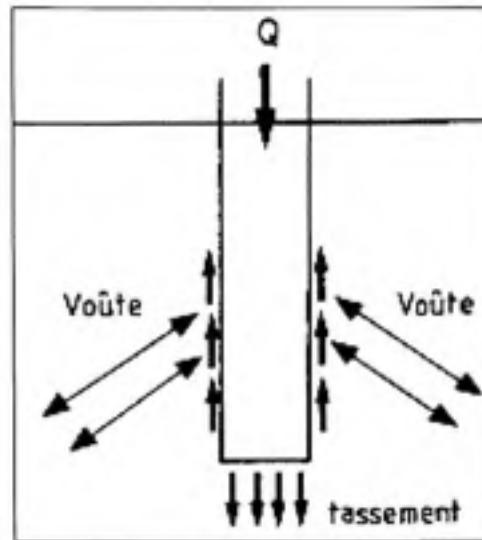
Figure 2.8 Effet de voûte. (Tiré de Philipponnat et Hubert, 1998)
