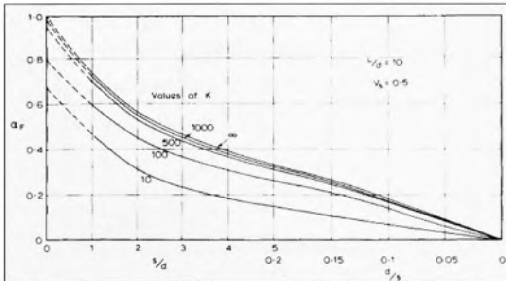
Figure 2.31 Coefficient d'interaction pour pieux flottants. (Tiré de Poulos et Davis, 1980)
