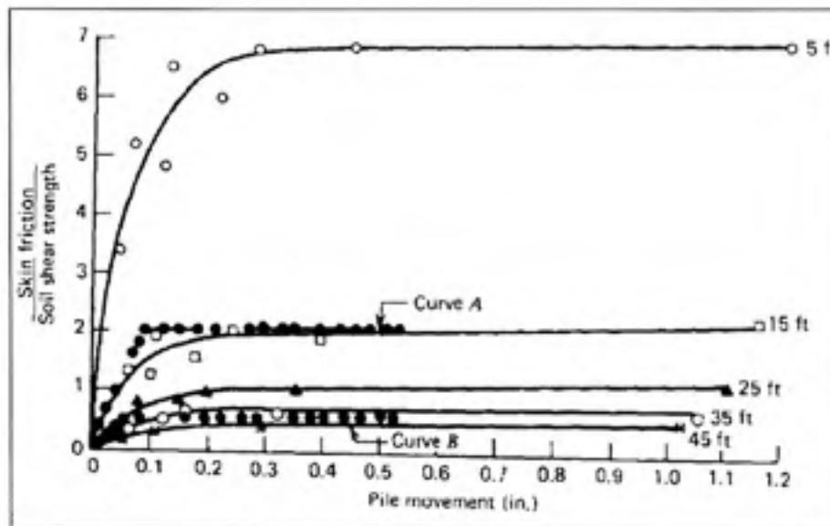
Figure 2.26 Courbes de transfert pour les pieux en acier installés dans les sables saturés. (Tiré de Coyle et Sulaiman, 1967)
