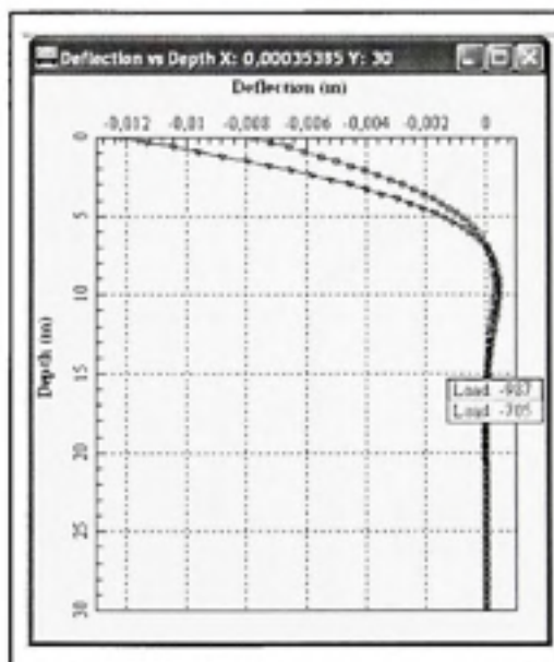
Figure VI.2 Déplacements versus profondeur.
