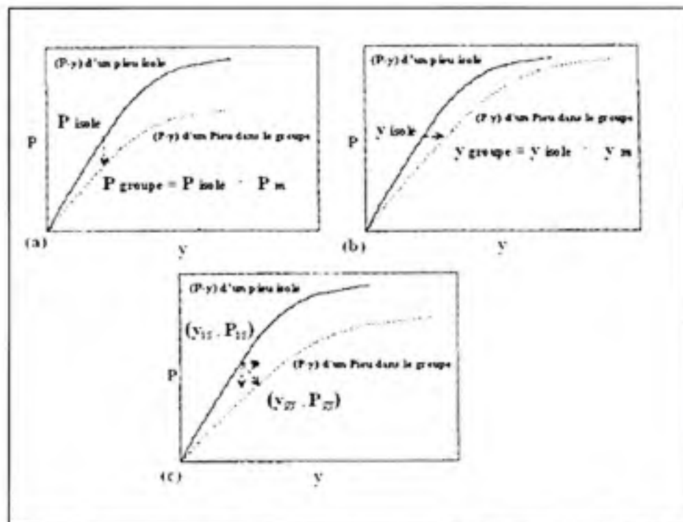
Figure 3.18 Approches de modification de courbes de réaction ( P-y ) d'un pieu en groupe : a) multiplicateur P_m ; b) multiplicateur y_m et c) multiplicateur de module. (Adapté de Fan et Long, 2006)
