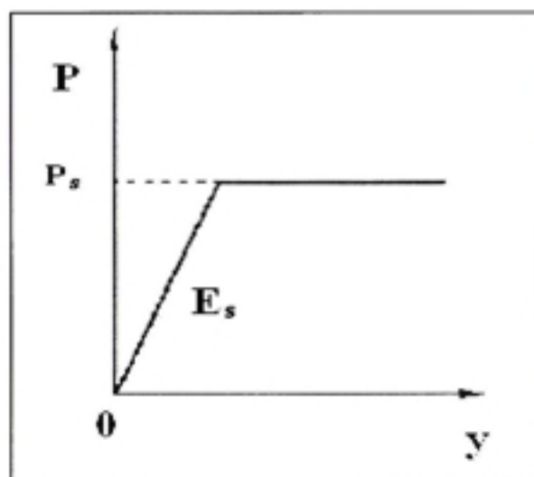
Figure 3.15 Loi de mobilisation de réaction tangentielle. (Adapté de Frank, 1995)
