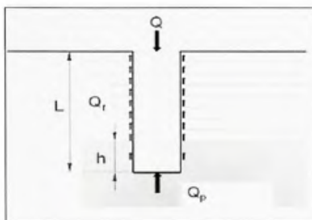
Figure 2.1 Pieu isolé soumis à une charge verticale. (Tiré de Philipponnat et Hubert, 1998)
