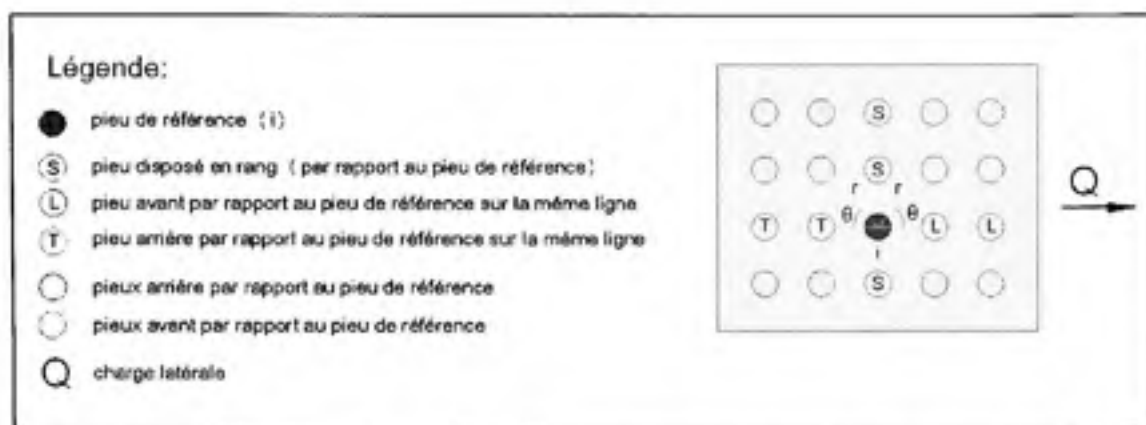
Figure 3.20 Disposition des pieux par rapport au pieu de référence (i). (Adapté de Salgado, 2008)
