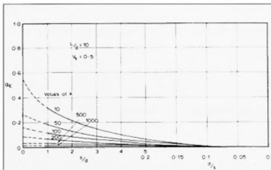
Figure 2.33 Coefficient d'interaction pour pieux porteurs en pointe. (Tiré de Poulos et Davis, 1980)
