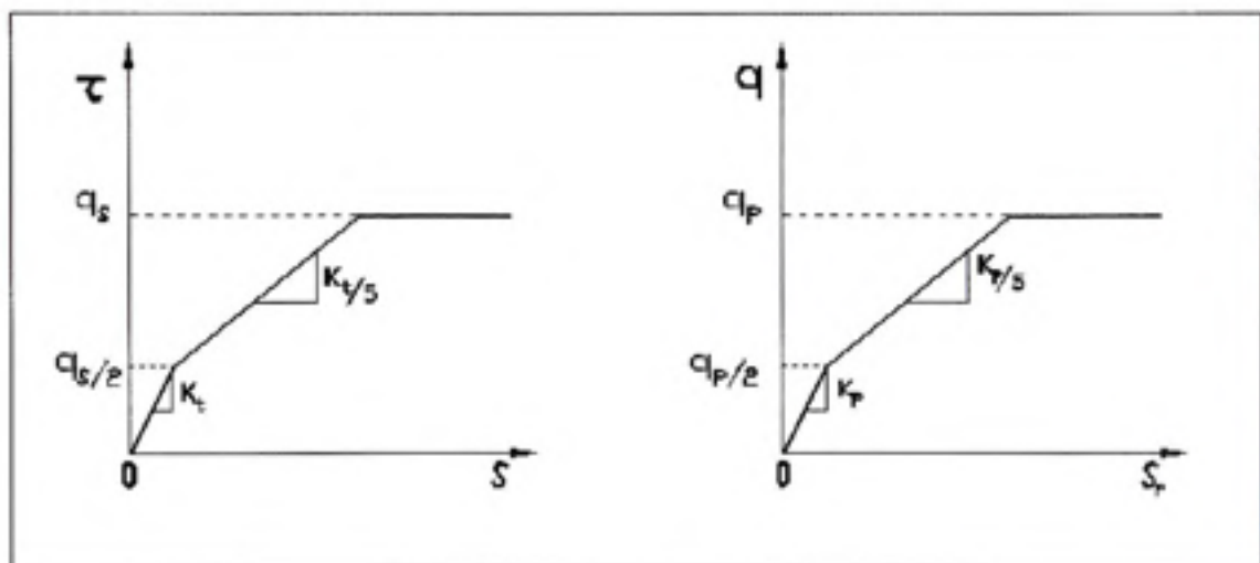
Figure 2.27 Lois de mobilisation du frottement latéral et de l'effort de pointe unitaires. (Adapté de Frank et Zhao, 1982)
