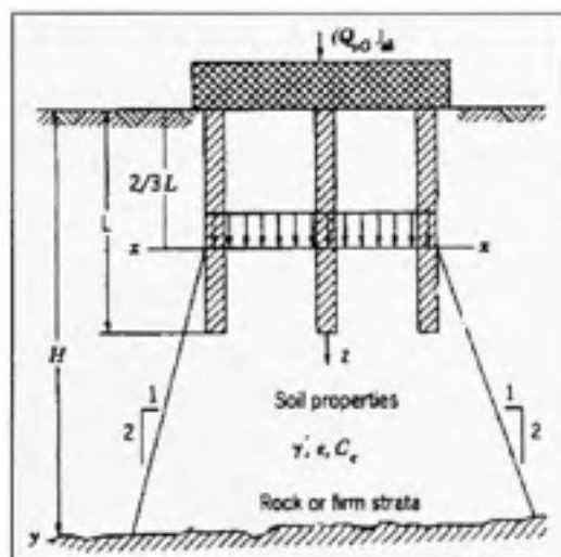
Figure 2.30 Répartition des contraintes pour pieux flottants dans une argile homogène. (Tiré de Prakash et Sharma, 1990)
