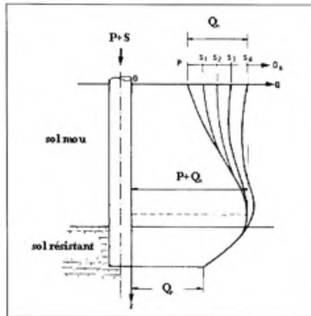
Figure 2.17 Déformations élastiques dues à la charge ( S ) conduisent à réduire le FN. (Tiré de Combarieu, 1985)
