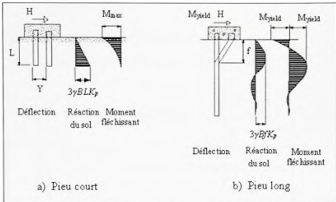
Figure 3.7 Mécanismes de ruptures pour un pieu fixe en tête sous charge latérale dans un sol pulvérulent. (Adapté de Broms, 1964b)
