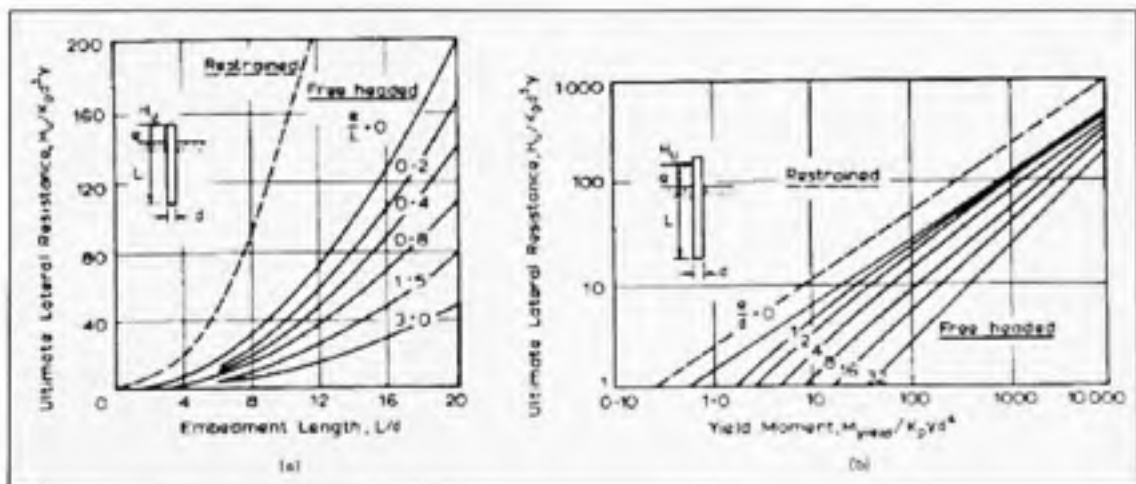
Figure 3.9 Résistance latérale ultime : a) pieu rigide et b) pieu souple dans un sol pulvérulent selon Broms (1964b). (Tiré de Poulos et Davis, 1980)
