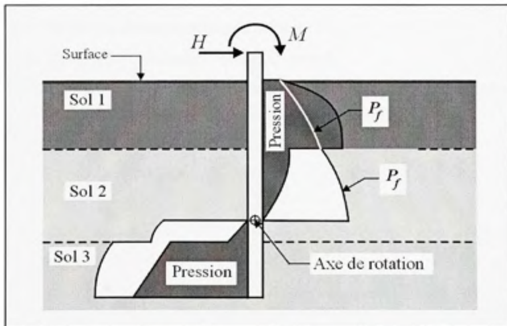
Figure 3.16 Pression sur sol versus pression de fluage.
