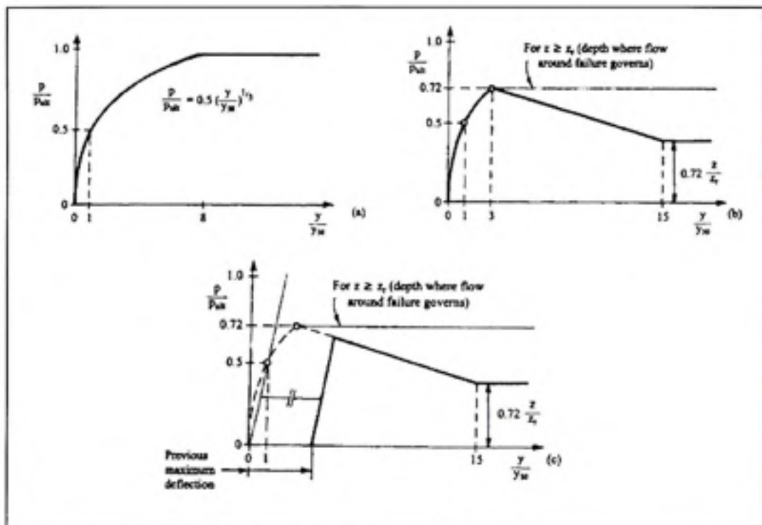
Figure 3.17 Courbe de (P-y) selon la méthode de Matlock pour argile molle sous chargement : a) statique; b) cyclique et c) après cyclique.
