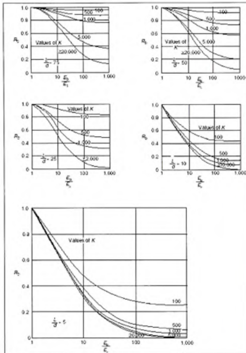
Figure 2.23 Coefficient de correction R_b (Tiré de Poulos et Davis, 1980)
