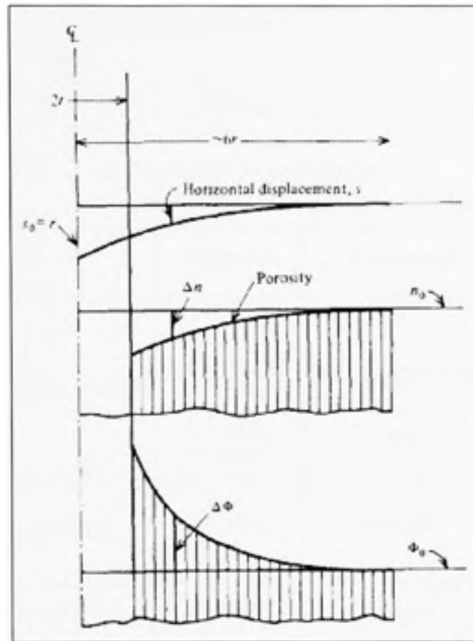
Figure 2.6 Effet de battage de pieu dans le sable. (Tiré de Kézdi et Rétháti, 1988)
