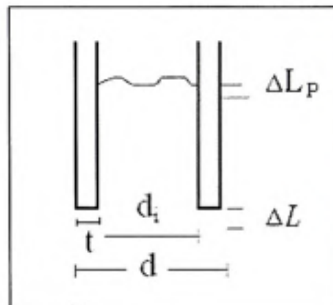
Figure 2.11 Pieu ouvert.
