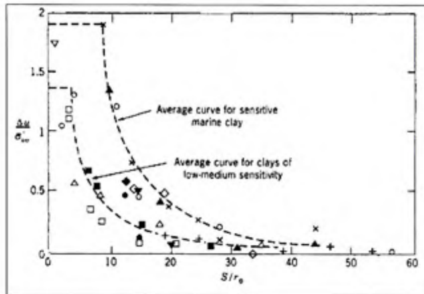
Figure 2.3. Résumé des mesures de l'excès de pression interstitielle. (Tiré de Poulos et Davis, 1980)
