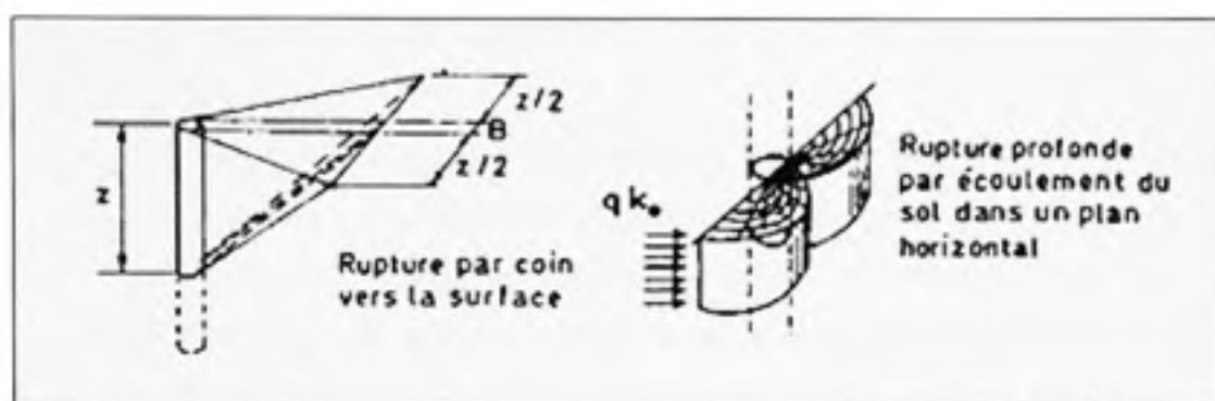
Figure 3.3 Mécanismes de rupture selon Blum et Brinch-Hansen. (Tiré de Baguelin et Gézéquel, 1972)
