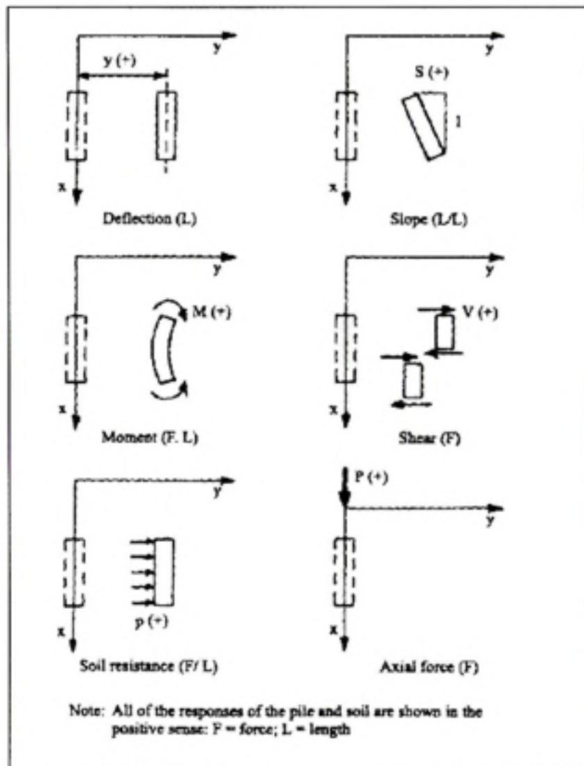
Figure V.1 Convention de signe de LPILE. (Tiré de Reese et Van Impe, 2001)
