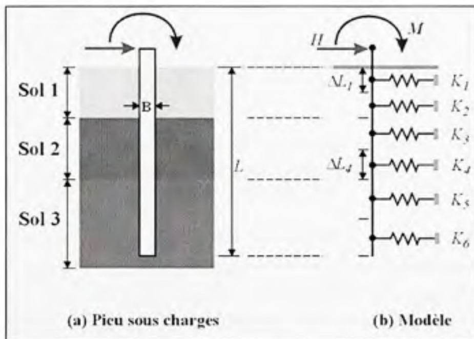
Figure 3.11 Modèle basé sur la théorie de Winkler.
