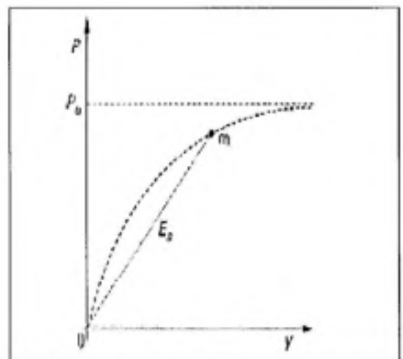
Figure 3.2 Courbe de réaction du sol. (Tiré de Frank, 1995)
