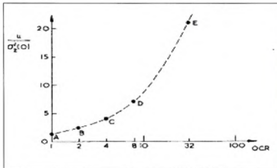
Figure 2.4. Excès des pressions interstitielles au voisinage du pieu à 1.15r_0 en fonction de OCR. (Tiré de Randolph et al. 1979)
