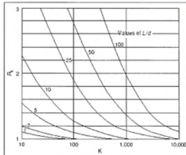
Figure 2.22 Coefficient de correction R_K (Tiré de Poulos et Davis, 1980)
