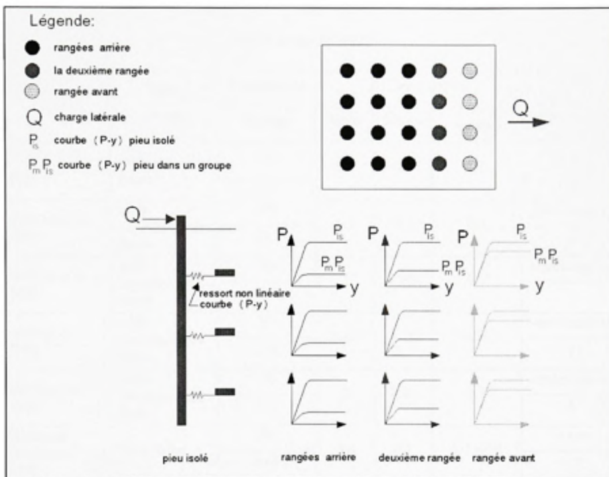
Figure 3.19 Approche P_m pour modification de courbes de réaction (P-y) d'un pieu en groupe. (Adapté de Hannigan et al., 1998)
