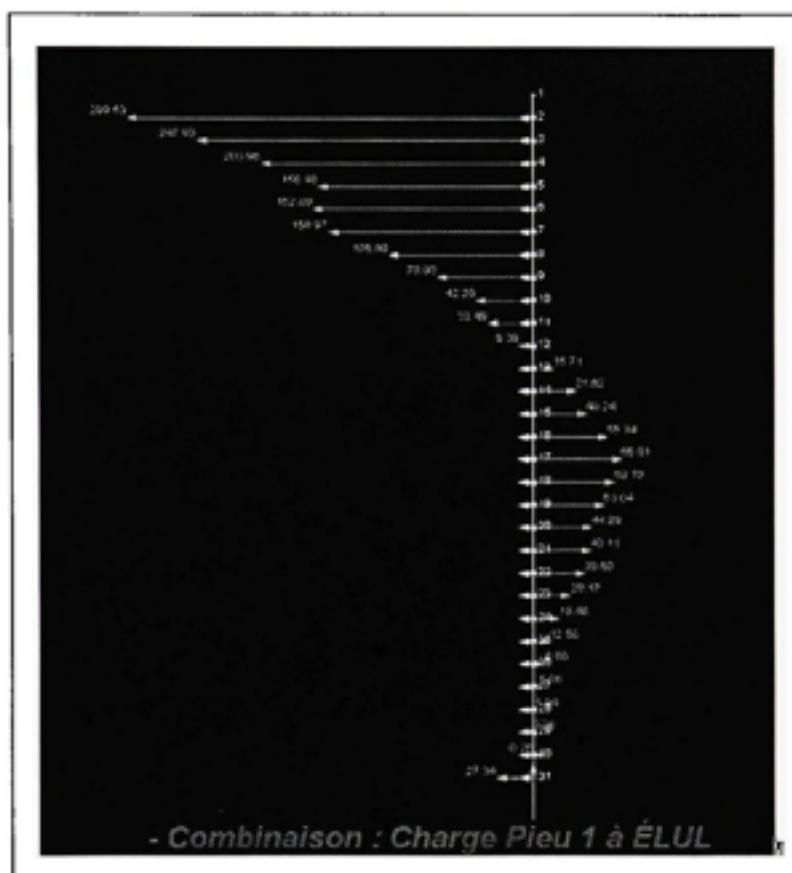
Figure III.2 Forces dans les ressorts versus profondeur. Pieu 1 selon l'axe y.
