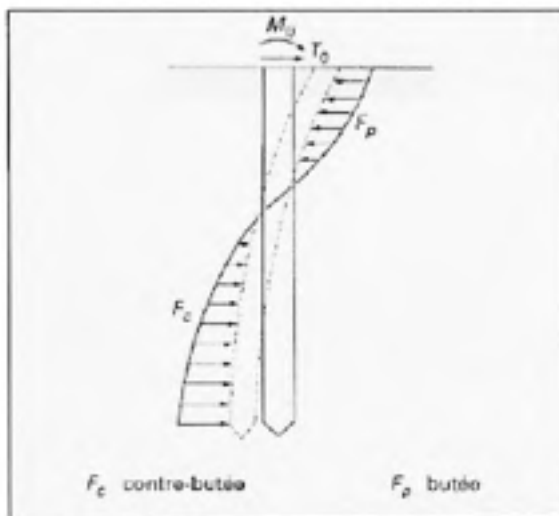
Figure 3.1 Pression et réaction du sol. (Tiré de Frank, 1995)
