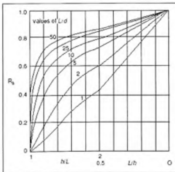
Figure 2.19 Coefficient de correction R_s (Tiré de Poulos et Davis, 1980)
