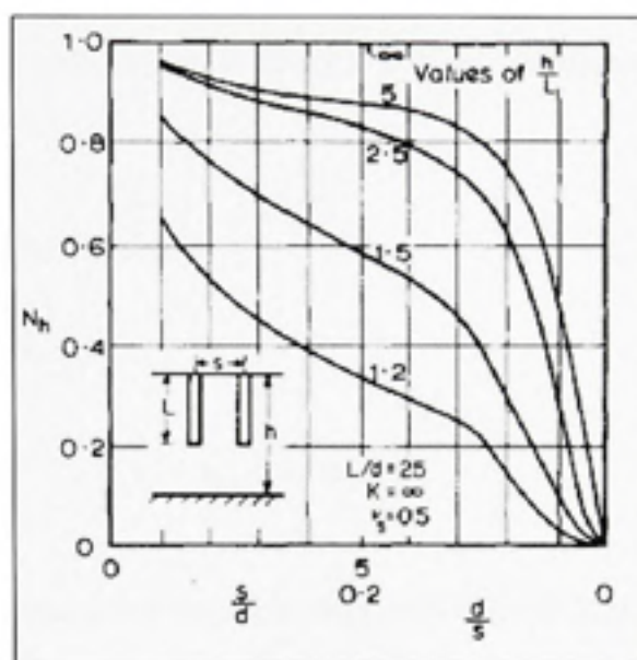
Figure 2.32 Coefficient de correction pour la couche semi-infinie. (Tiré de Poulos et Davis, 1980)
