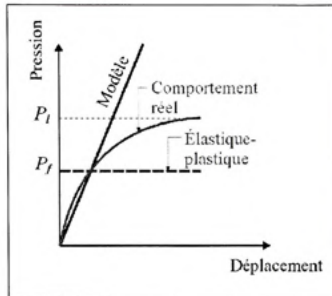
Figure 3.13 Comportement réel du sol versus comportement élasto-plastique.
