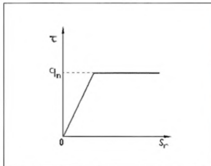
Figure 2.16 Loi de comportement liant le déplacement relatif au cisaillement. (Adapté de Combarieu, 1984)
