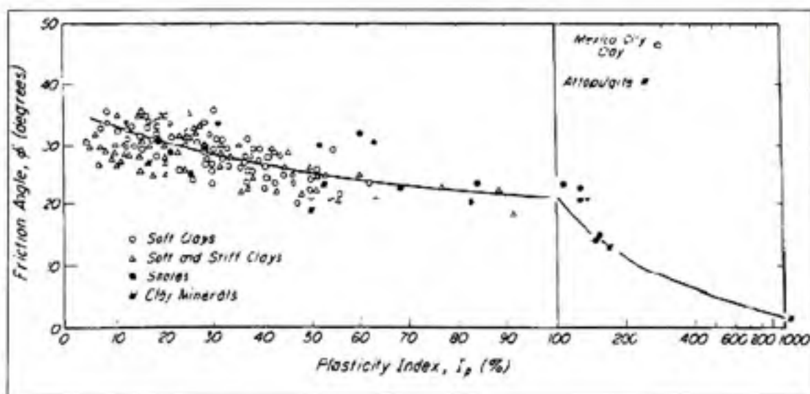
Figure 1.1 Angle \phi' des sols cohérents en fonction de l'indice de plasticité ( I_p ). (Tiré de Terzaghi et al., 1996)
