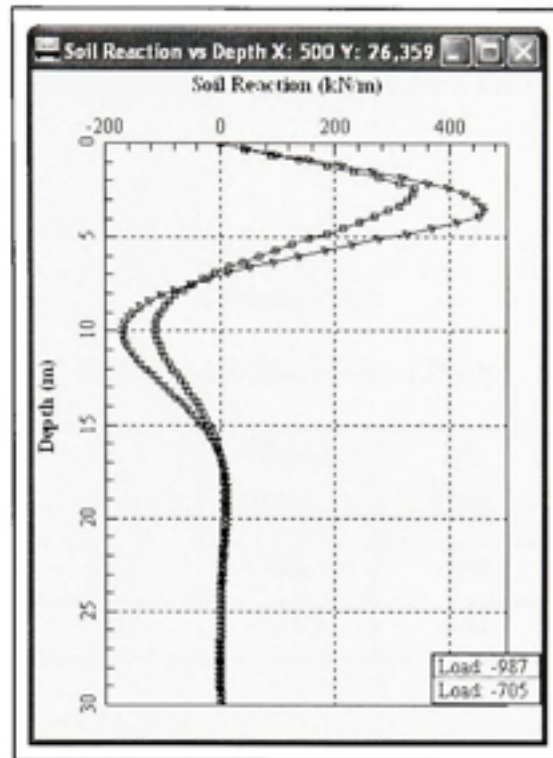
Figure VI.5 Réaction du sol versus profondeur.
