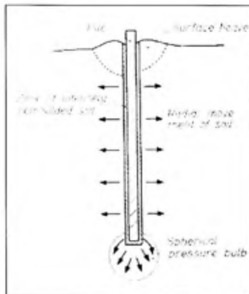
Figure 2.2 Déplacement du sol dû à l'installation du pieu selon Randolph (1983). (Tiré de Kézdi et Rétháti, 1988)
