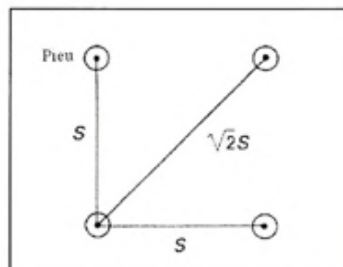
Figure 2.34 Groupe de 4 pieux identiques. (Adapté de Frank, 1995)
