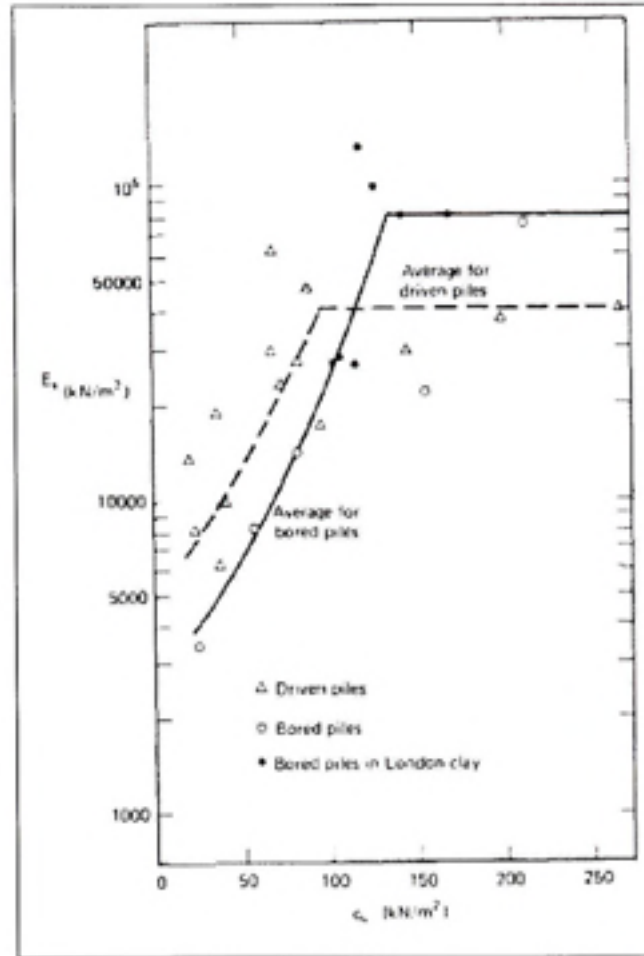
Figure 2.24 Module du sol pour les argiles. (Tiré de Poulos et Davis, 1980)
