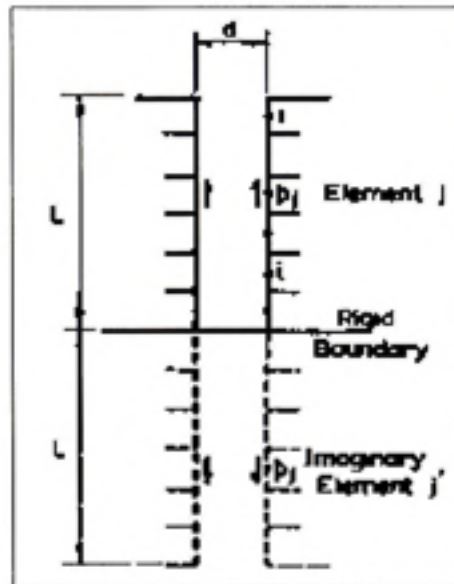
Figure 2.14 Pointe de pieu rigide. (Tiré de Poulos et Mattes, 1969)
