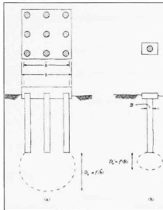
Figure 2.29 Zone d'influence pour tassement : a) de groupe de pieux et b) d'un pieu isolé (Tiré de Prakash et Sharma, 1990)
