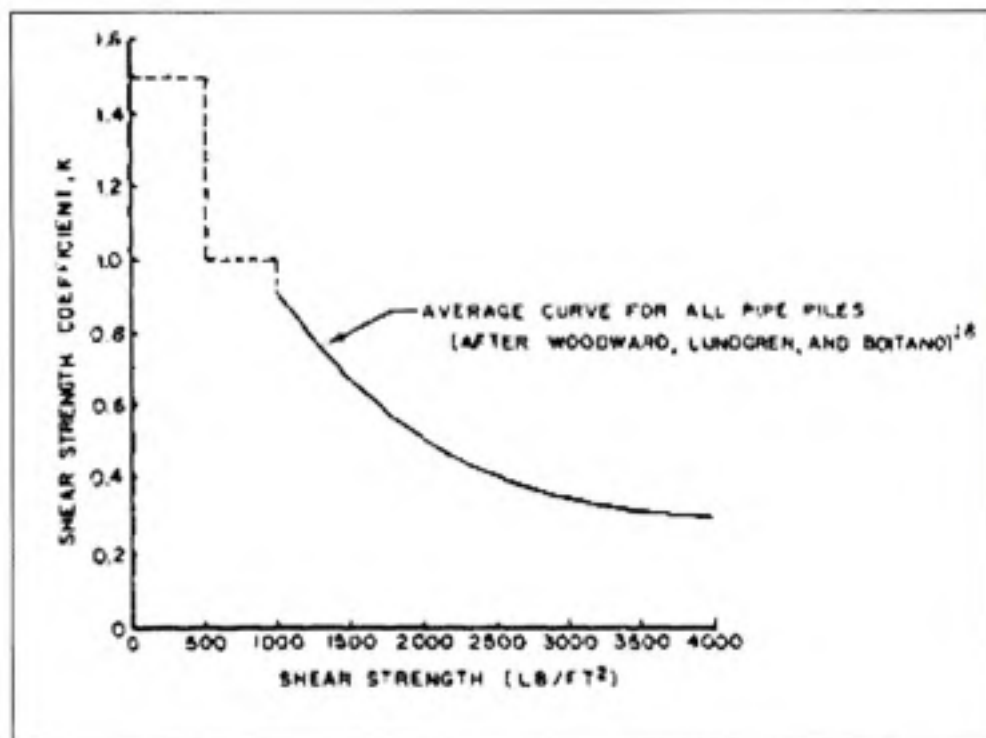
Figure 2.9 Coefficient de réduction de la résistance de cisaillement pour l'argile. (Tiré de Coyle et Reese, 1966)
