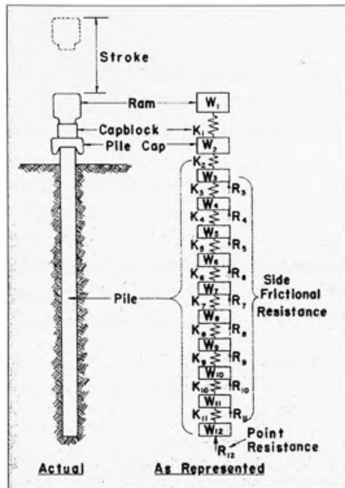
Figure 2.13 Modèle de Smith. (Tiré de Smith, 1960)
