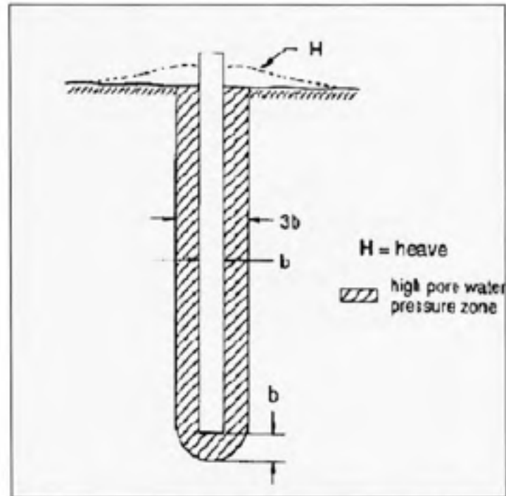
Figure 2.5 Zone remaniée dans les sols cohérents lors de battage de pieux. (Tiré de Hannigan et al., 1998)
