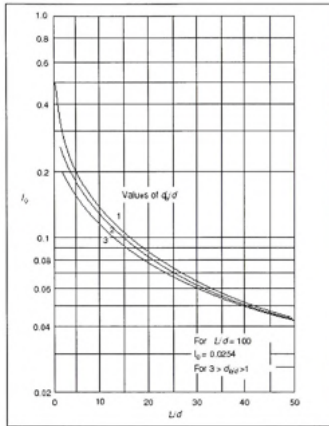
Figure 2.21 Coefficient d'influence pour le tassement I_0 (Tiré de Poulos et Davis, 1980)
