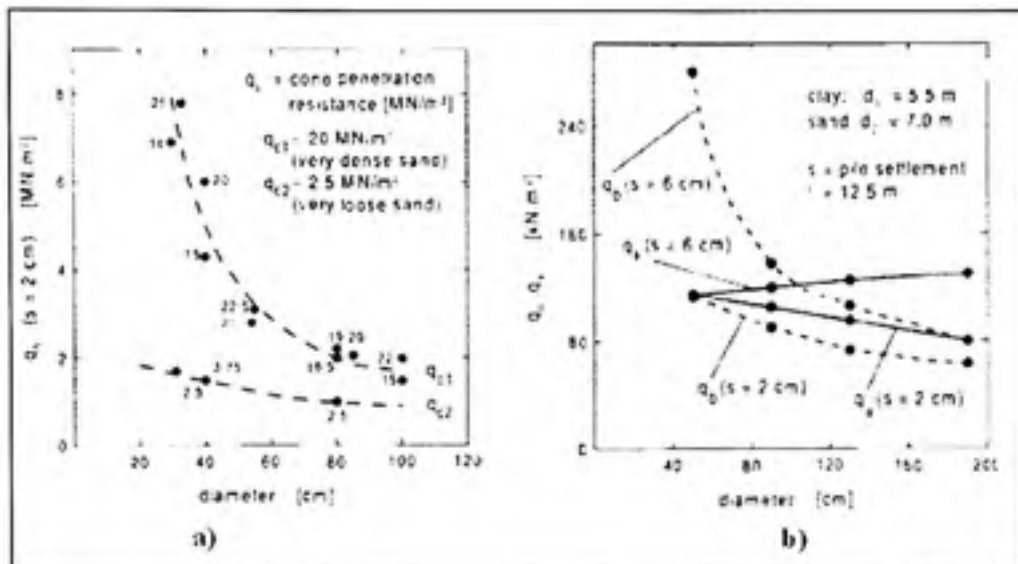
Figure 2.10 Corrélation entre la résistance en pointe et le diamètre de pieu à partir : a) des essais de chargement de pieu et b) les résultats de MEF. (Tiré de Kempfert et al., 2002)
