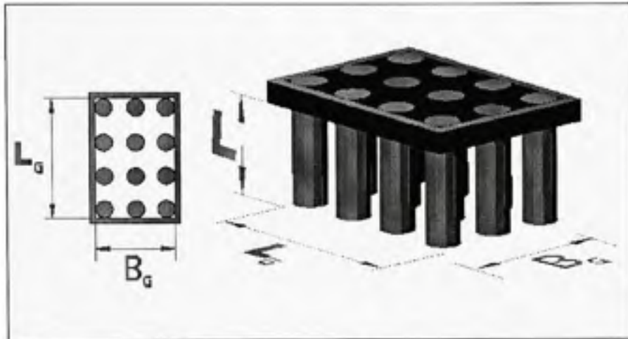
Figure 2.28 Dimensions du bloc monolithique.
