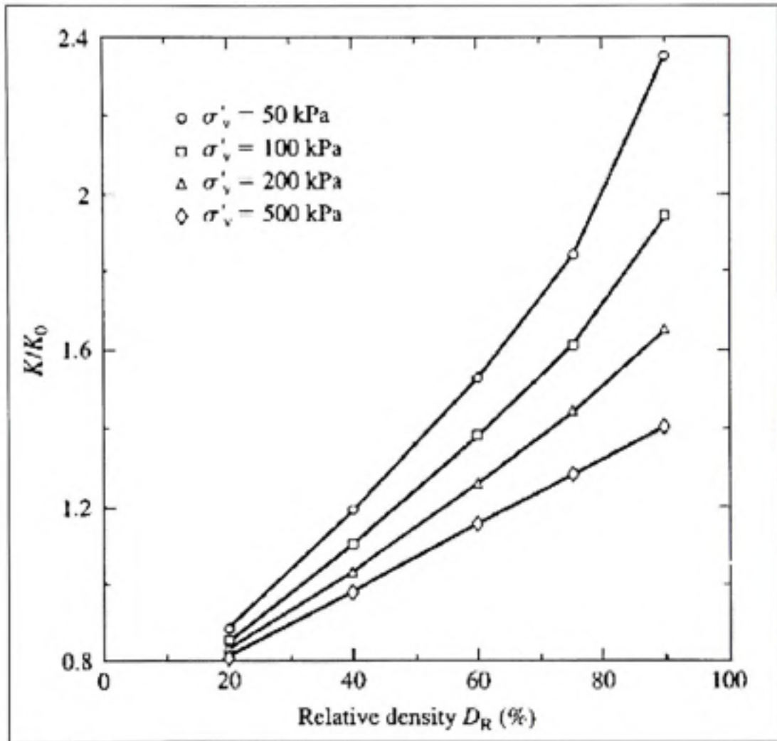
Figure 2.12 Valeurs de K pour les pieux qui ne refoulent pas le sol. (Tiré de Salgado, 2008)
