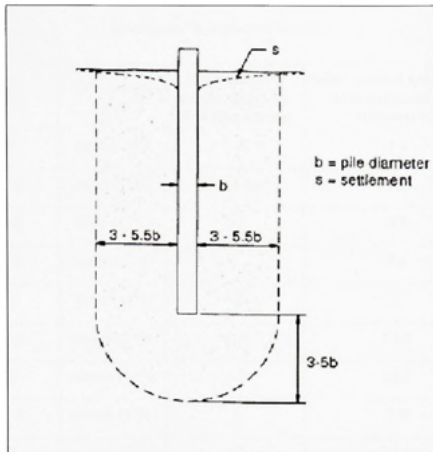
Figure 2.7 Zone densifiée des sols pulvérulents lors de battage de pieux. (Tiré de Hannigan et al., 1998)
