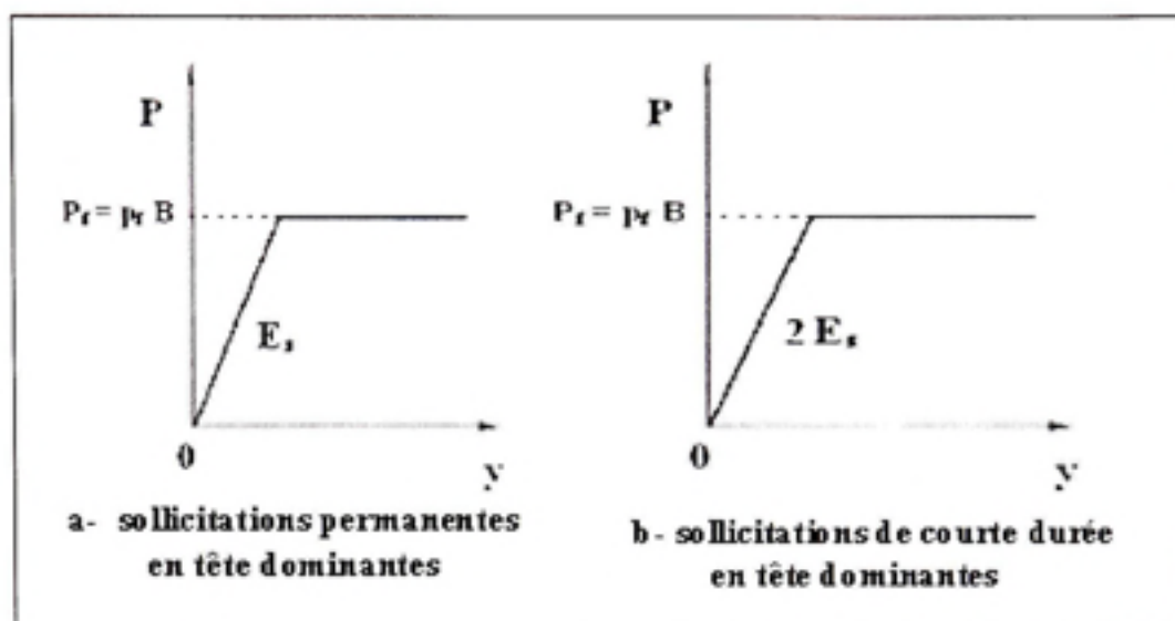
Figure 3.14 Courbe de réaction ( P - y ). (Adapté de Frank, 1995)
