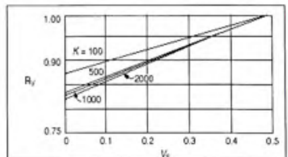
Figure 2.20 Coefficient de correction R_v (Tiré de Poulos et Davis, 1980)
