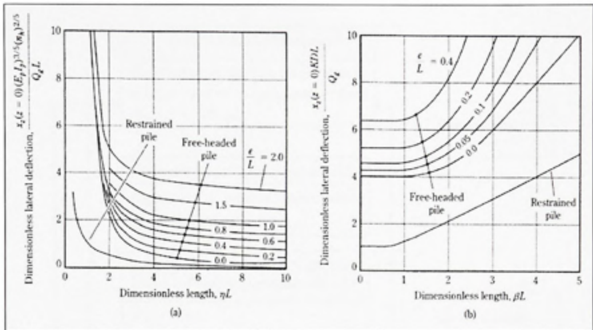
Figure 3.10 Calcul du déplacement selon Broms : a) sol pulvérulent; b) sol cohérent. (Tiré de Das, 2004)
