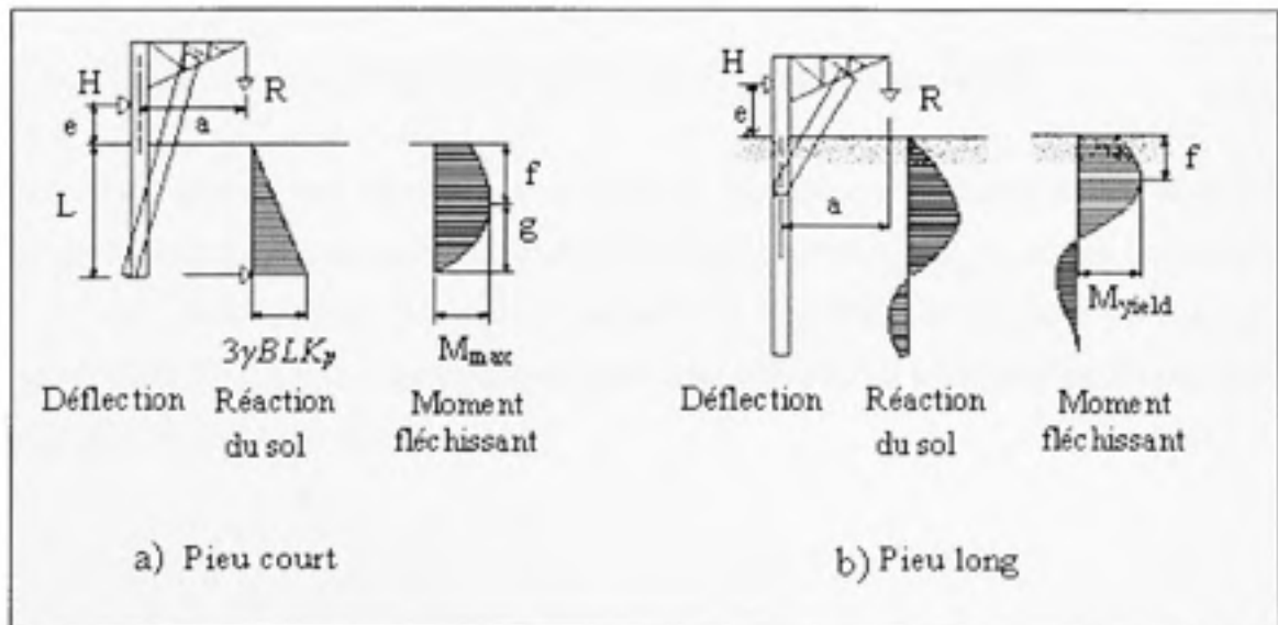
Figure 3.6 Mécanismes de ruptures pour un pieu libre en tête sous charge latérale dans un sol pulvérulent. (Adapté de Broms, 1964b)
