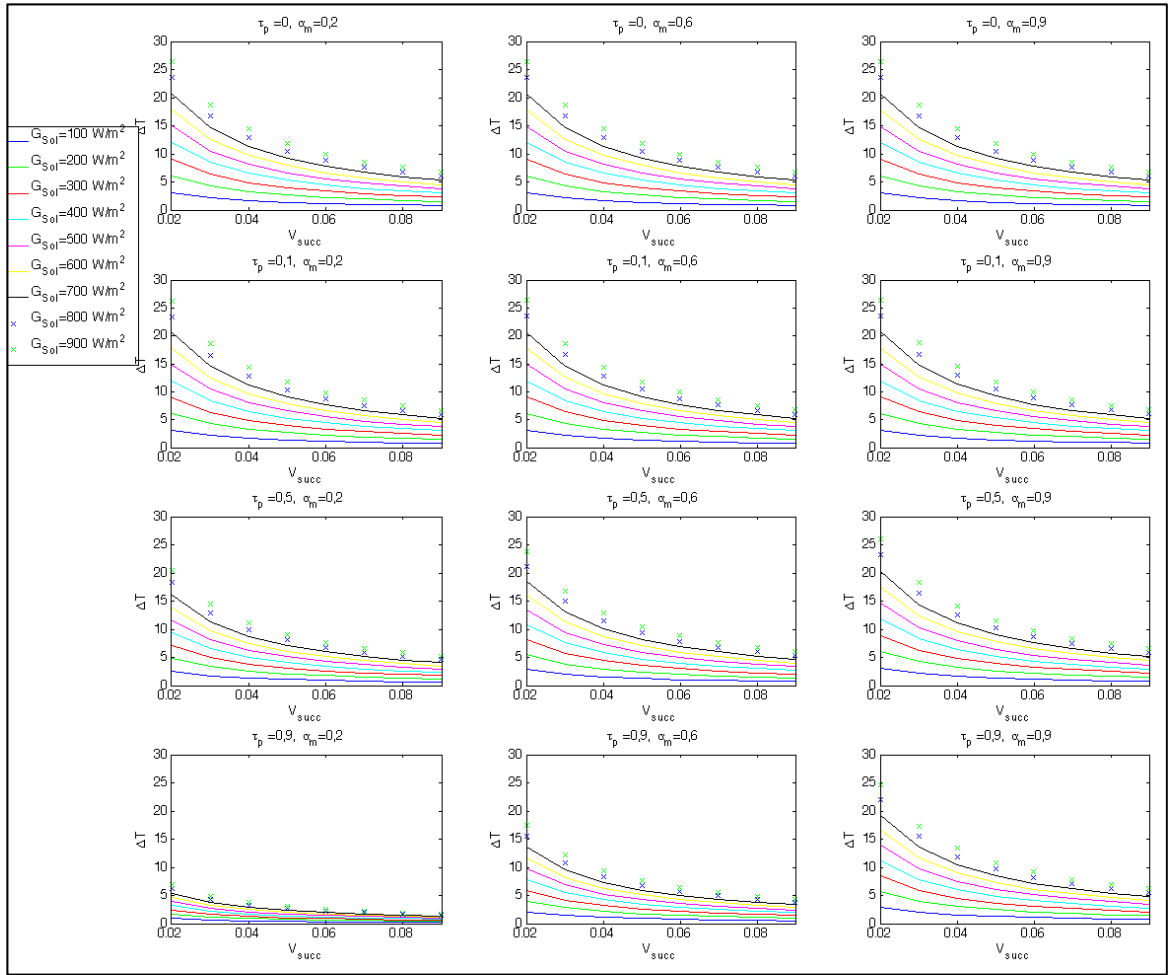
Figure-A IV-3 : Différence de température avec conduction
