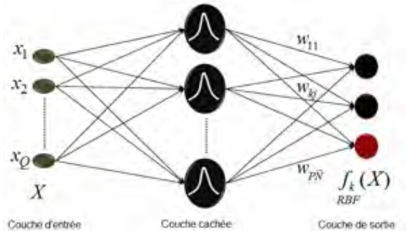
Figure 67 -Architecture de réseaux RBF.
