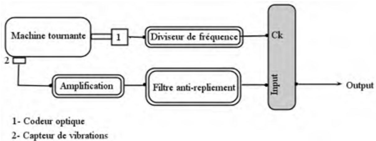
Figure 18 - Chaîne d'acquisition d'échantillonnage angulaire direct.
