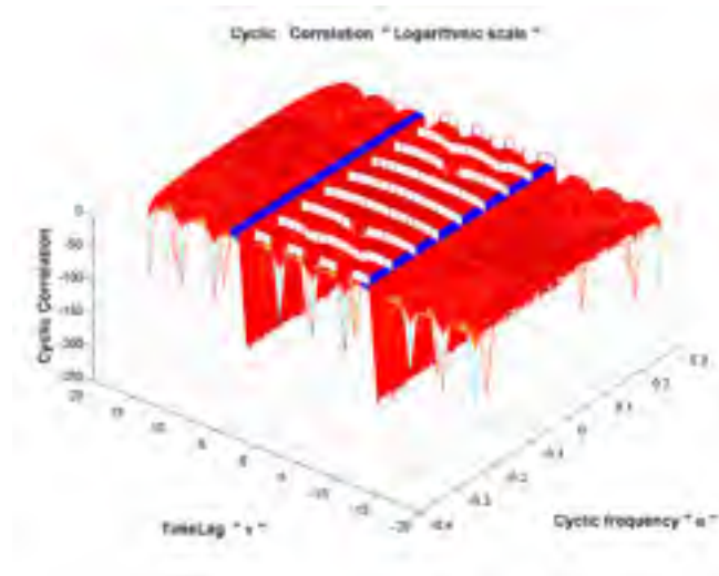
Figure 12 -Fonction d'autocorrélation cyclique en échelle logarithmique d'un train d'impulsions modulé en amplitude.
