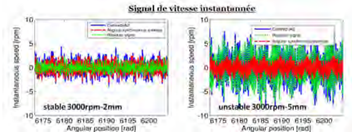
Figure 61 -Décomposition du signal de vitesse instantanée.
