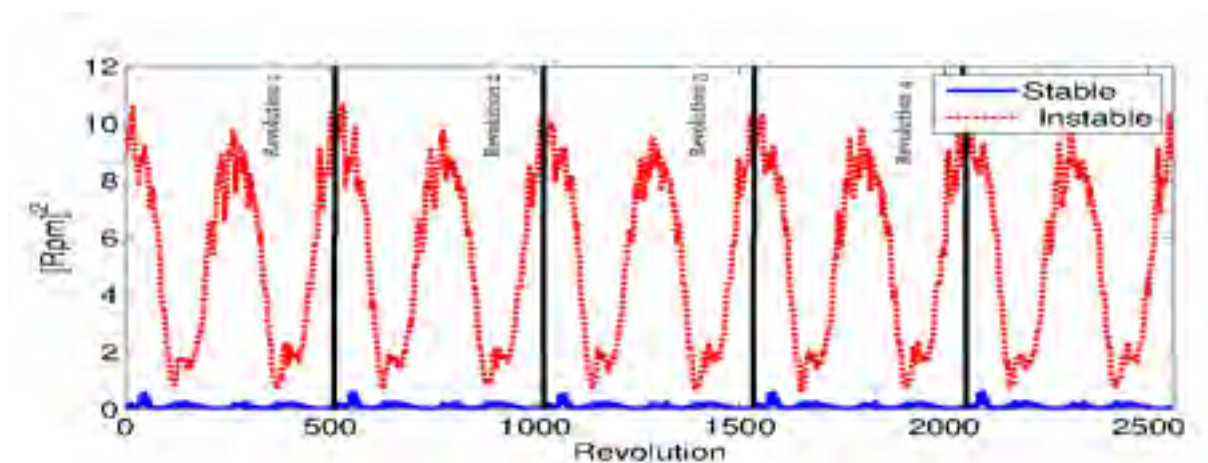
Figure 59 -Variance angulaire synchrone des signaux de force pour les cas stable (bleu continue) et instable (rouge pointillée).
