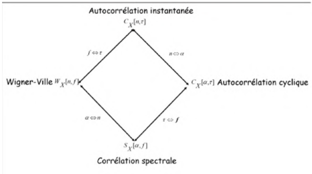
Figure 10 -Espace de représentation d'un processus cyclostationnaire à l'ordre (2).
