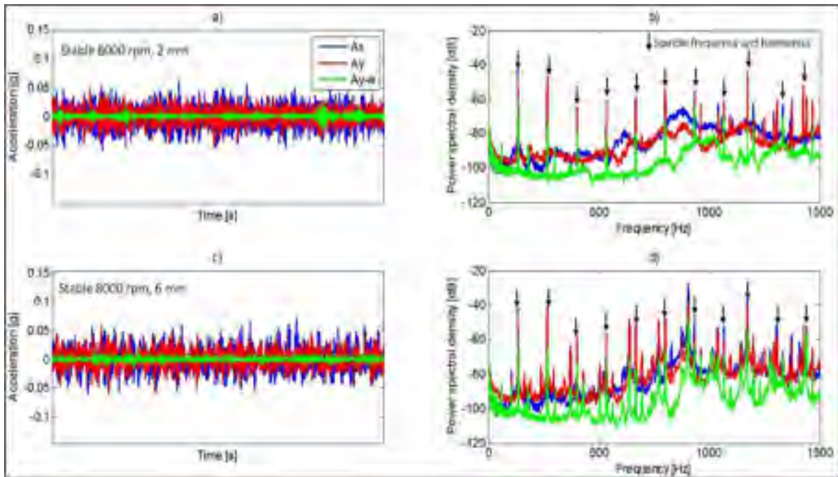
Figure 30 -Présentations temporelles et densité spectrale de puissance des signaux d'accélération. A_x : le signal issu du capteur placé dans la partie non rotative de la broche dans la direction X. A_y : le signal issu du capteur placé dans la partie non rotative de la broche dans la direction Y. A_{yw} : le signal issu du capteur placé sur la pièce dans la direction Y. (a) et (b) présentent les conditions stables (8000rpm, 2mm), (c) et (d) présentent les conditions instables (8000rpm, 6mm). Les paramètres de la PSD sont : la résolution fréquentielle est égale à 1.3 Hz, le nombre de moyennes utilisé est 60, la fenêtre utilisée est hamming et la méthode d'estimation utilisée est le périodogramme de Welch. Les flèches noires indiquent la fréquence de rotation de la broche et ses harmoniques. D'autres composants correspondent aux fréquences du broutage.
