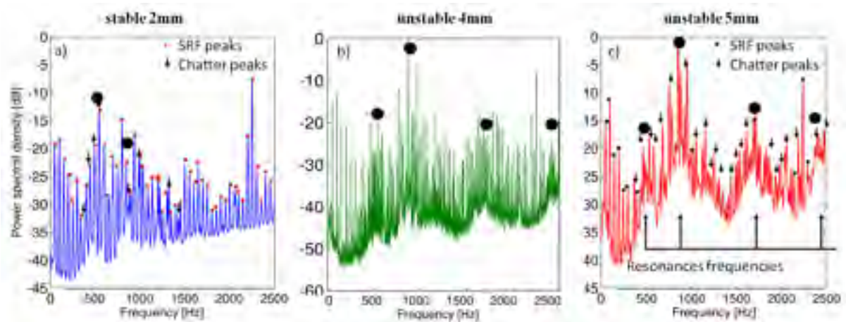
Figure 54 -Densité spectrale de puissance des signaux de vitesse dans différentes conditions. (a) 3000rpm et 2mm. (b) 3000rpm et 4mm. (c) 3000rpm et 5mm. Les points rouges dénotent la fréquence de rotation de la broche et ses harmoniques. Les flèches noires représentent les fréquences liées au broutage. Les disques noirs montrent les résonances.
