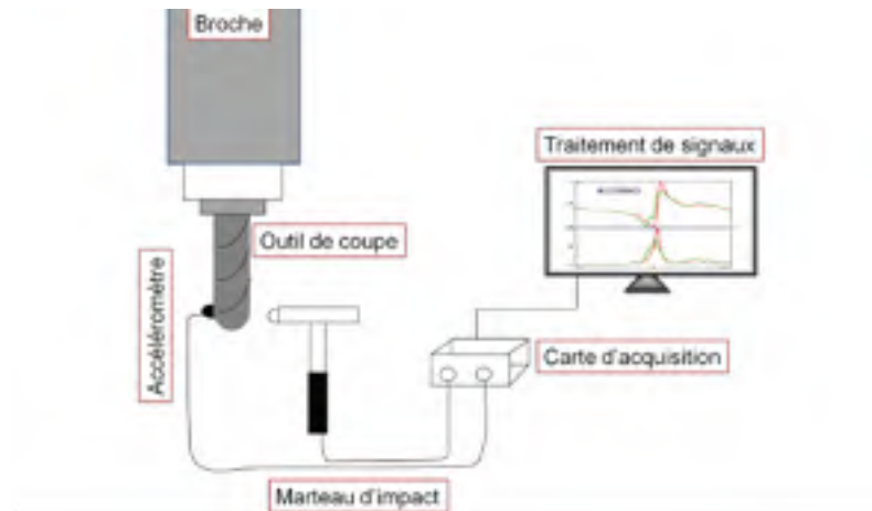
Figure 8 -Schéma de principe de test d'impact.
