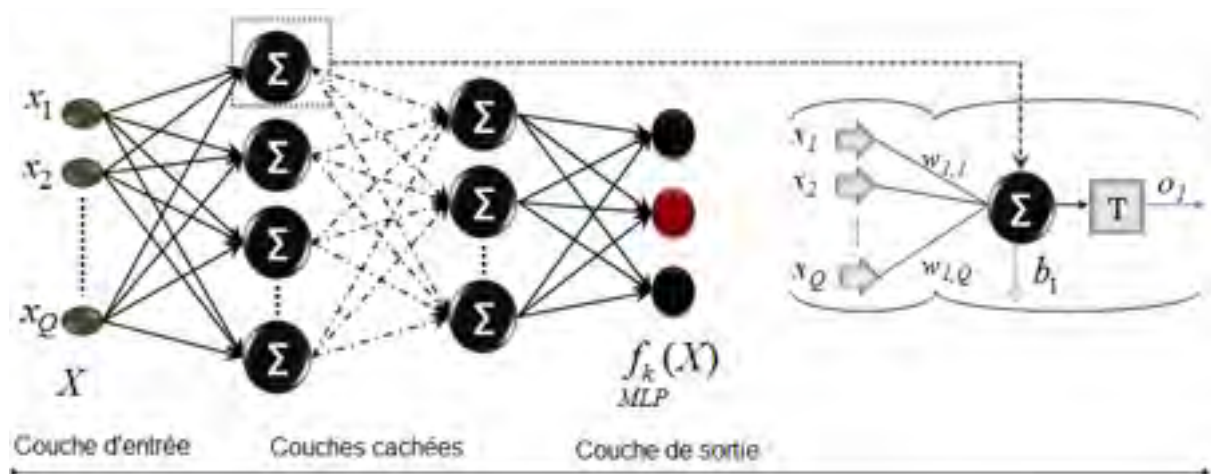
Figure 66 -Architecture du perceptron multicouche (MLP).
