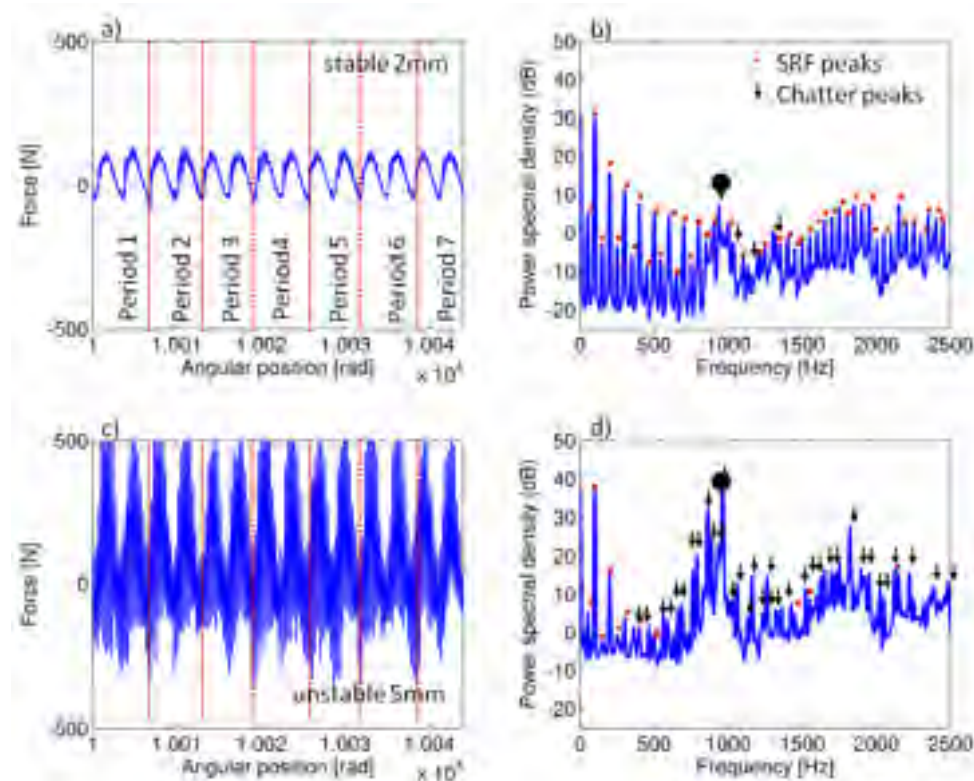
Figure 49 -Représentation angulaire et spectrale (PSD) des signaux de force dans la direction d'avance F_f . (a,b) Conditions stables (3000rpm, 2mm, N 2 dents). (c,d) Conditions instables (3000rpm, 5mm, N 2 dents). Les points rouges caractérisent la fréquence de rotation de la broche et ses harmoniques. Les flèches noires dénotent les fréquences excitées liées au broutage. Les disques noirs montrent les résonances.
