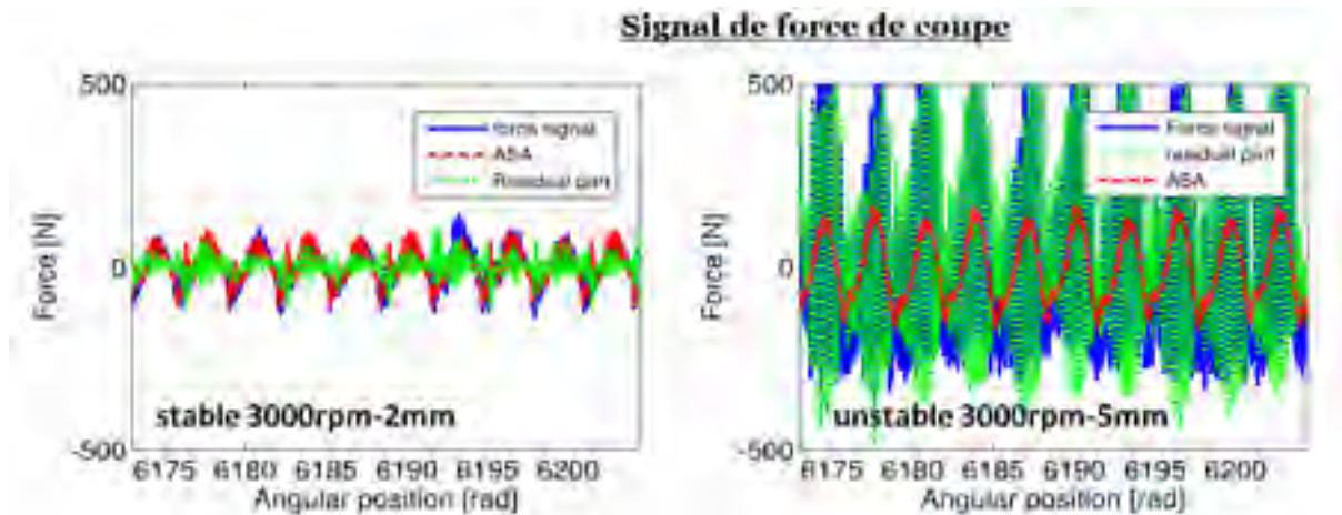
Figure 60 -Décomposition du signal de force de coupe.
