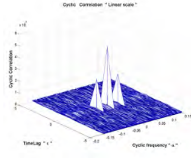
Figure 14 -Fonction d'autocorrélation cyclique en échelle linéaire d'un signal modulé en amplitude. Cette fonction n'est pas nulle pour les fréquences cycliques \alpha = 0 et \alpha = \pm 2f_0 .
