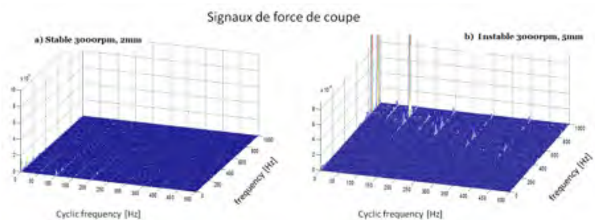
Figure 57 -Corrélation spectrale des signaux de force de coupe dans les cas stable (a) et instable (b).
