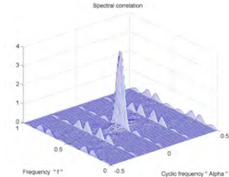
Figure 13 -Fonction de corrélation spectrale d'un train d'impulsions.
