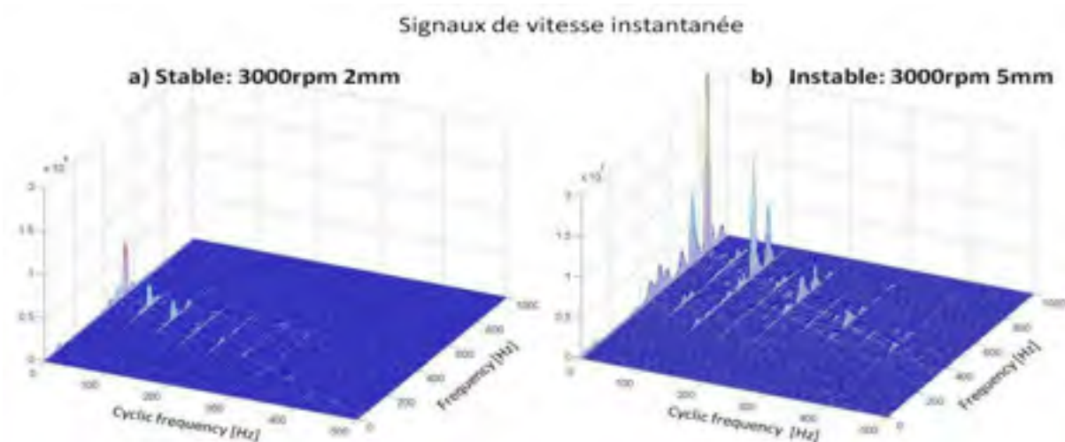
Figure 56 -Corrélation spectrale des signaux de vitesse dans les cas stable (a) et instable (b).
