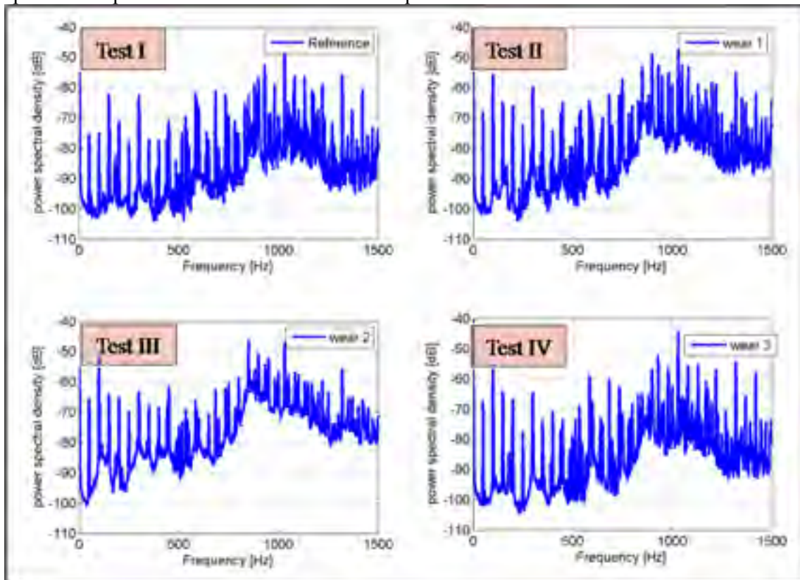
Figure 41 Densité spectrale de puissance de l'usure de l'outil de coupe pour les quatre scénarios.
