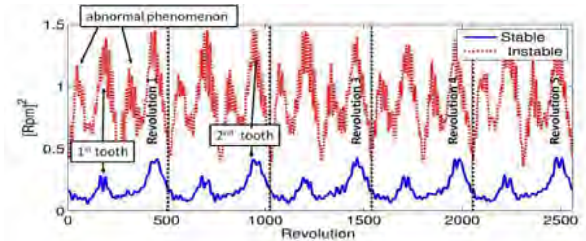
Figure 58 -Variance angulaire synchrone des signaux de vitesse pour les cas stable (bleu continue) et instable (rouge pointillée).
