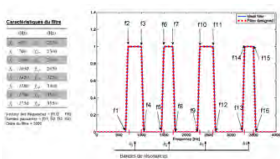
Figure 65 -Caractéristiques du filtre multi bande.
