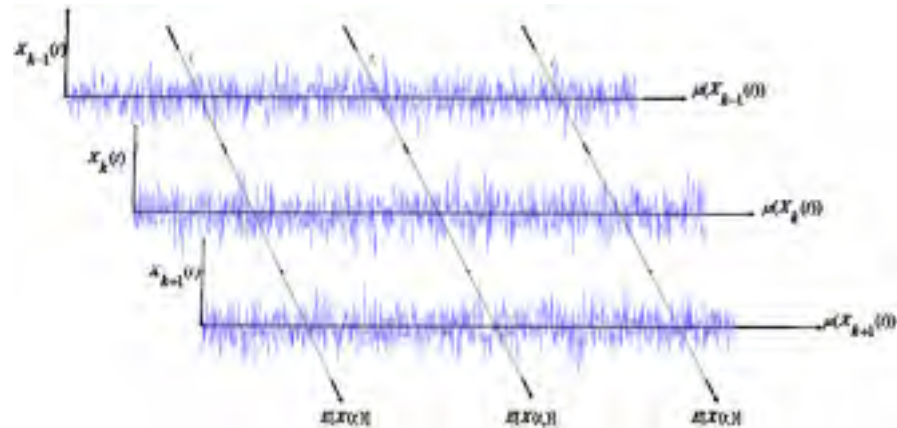
Figure 16 -Processus stationnaire.
