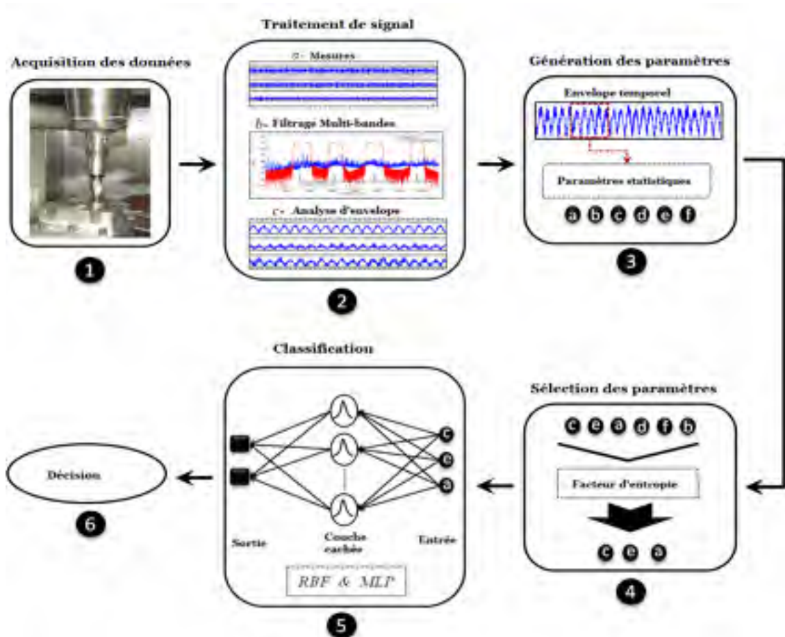
Figure 64 -Méthodologie pour la détection du broutage.
