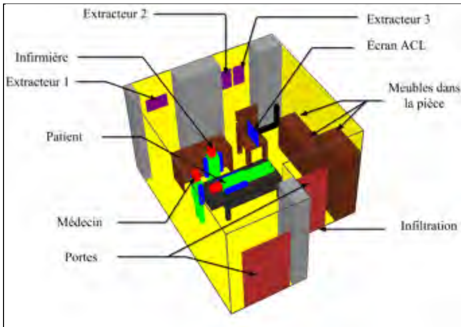
Figure 5.1 Géométrie de l'unité étudiée
