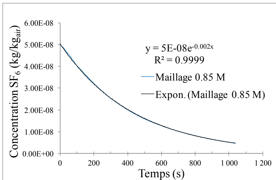
Figure 5.8 Concentration du SF 6 en fonction du temps pour 0,85 million de nœuds
