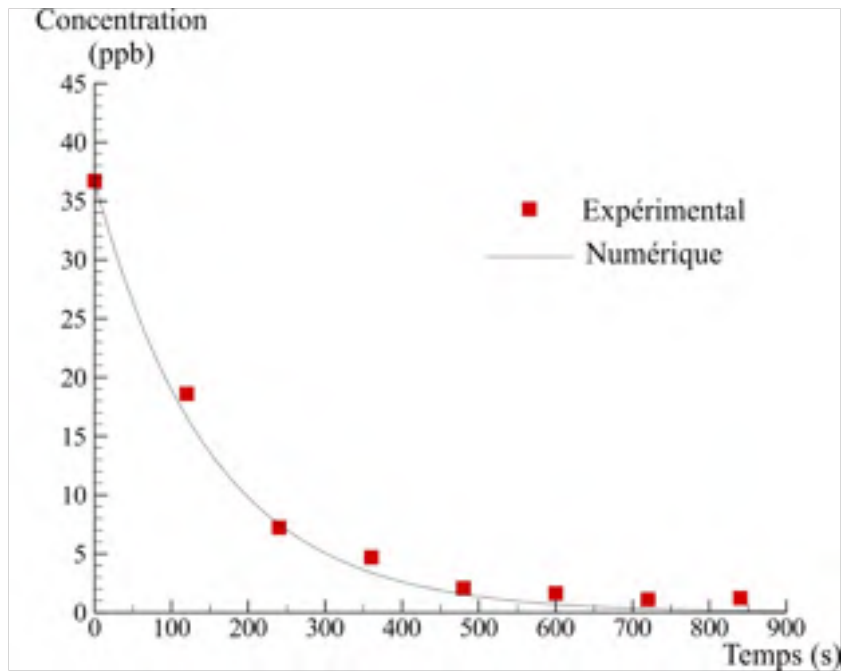
Figure 5.2 Évolution de la concentration de SF 6 en fonction du temps
