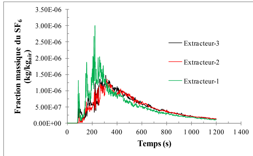
Figure 6.4 Fraction massique de SF 6 au niveau des extracteurs en fonction du temps pour 8 CAH (modèle SP)
