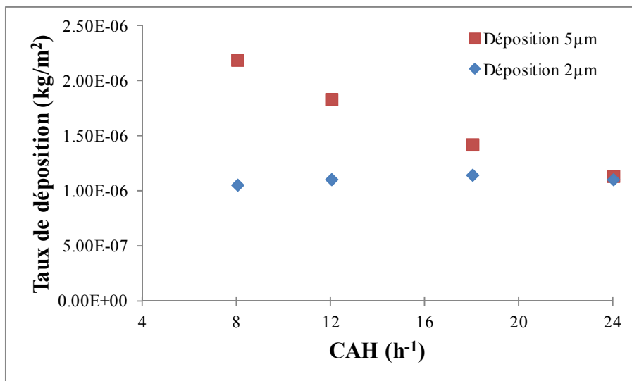
Figure 6.14 Taux de déposition pour 2 et 5 μm
