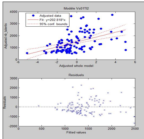
Figure-A IV-6 MRLM et résiduels pour Nb_talents dans Vs01T12
