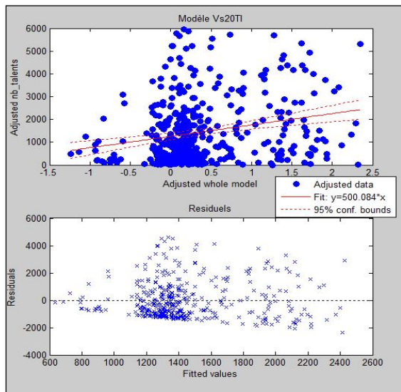
Figure-A IV-7 MRLM et résiduels pour Nb_talents dans Vs20T1
