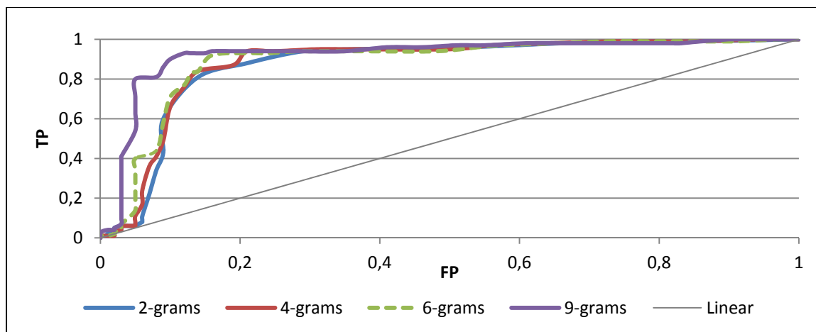
Figure 4.24 Courbe ROC du modèle Arbre n-grams (scénario 1)
