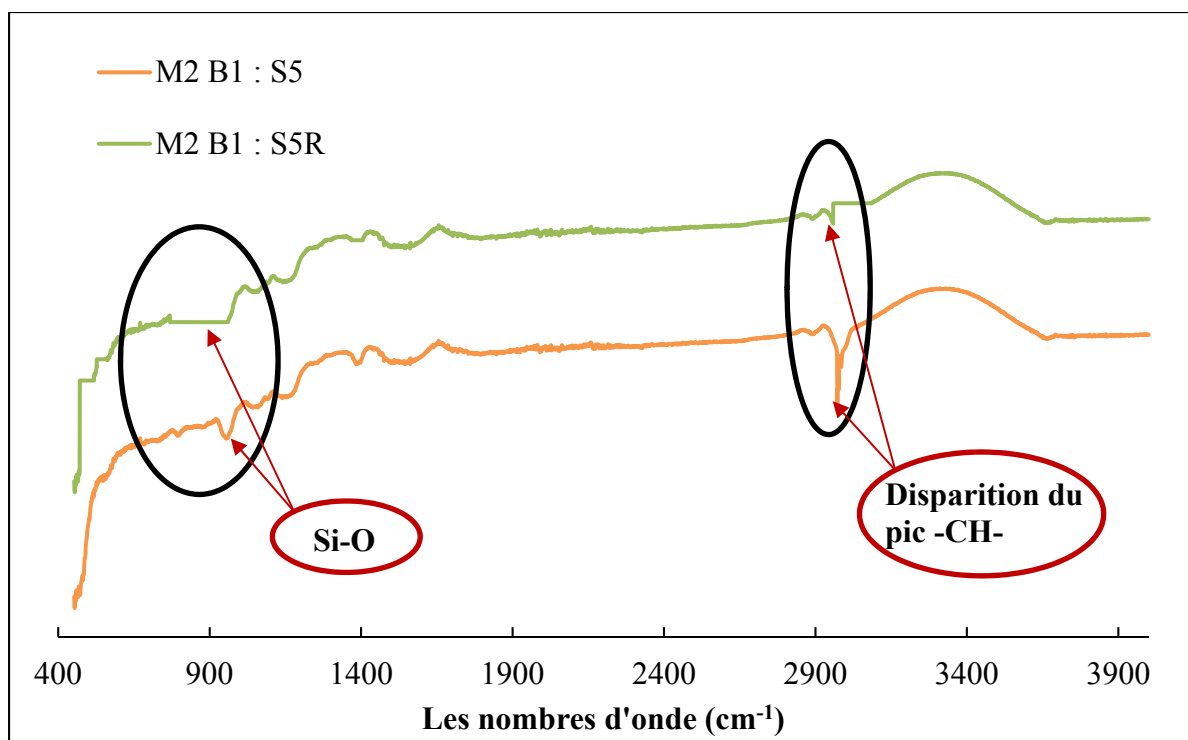
Figure 3.22 Les spectres IR pour le nanocomposite (M2 B2 : S5) et le même nanocomposite après avoir appliquée un protocole de réduction avec le bicarbonate de soude (M2 B2 : S5R)
