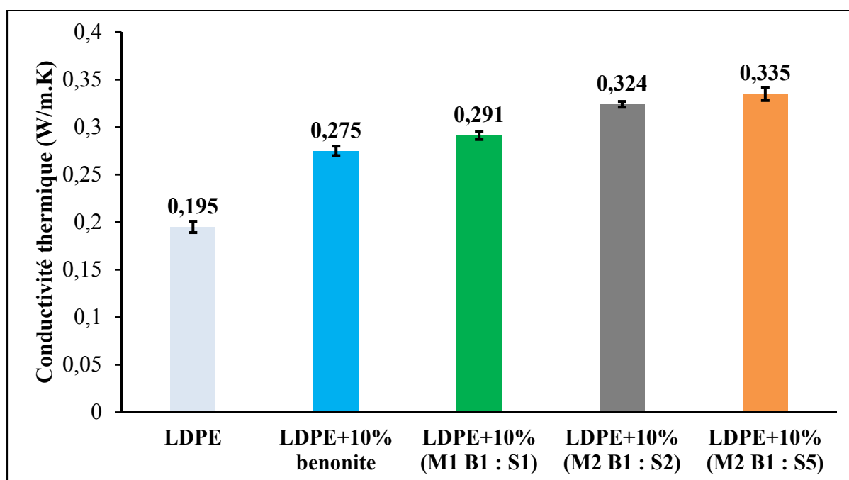
Figure 3.21 La conductivité thermique LPDE, LPDE+10%bentonite, LPDE+10%(M1 B1 : S1), LPDE+10%(M2 B1 : S2), LPDE+10%(M2 B1 : S5)
