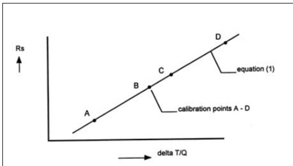
Figure 2.23 Analyse des données de mesure de flux de la chaleur surveillé Tirée de Technical note 50 (2012)
