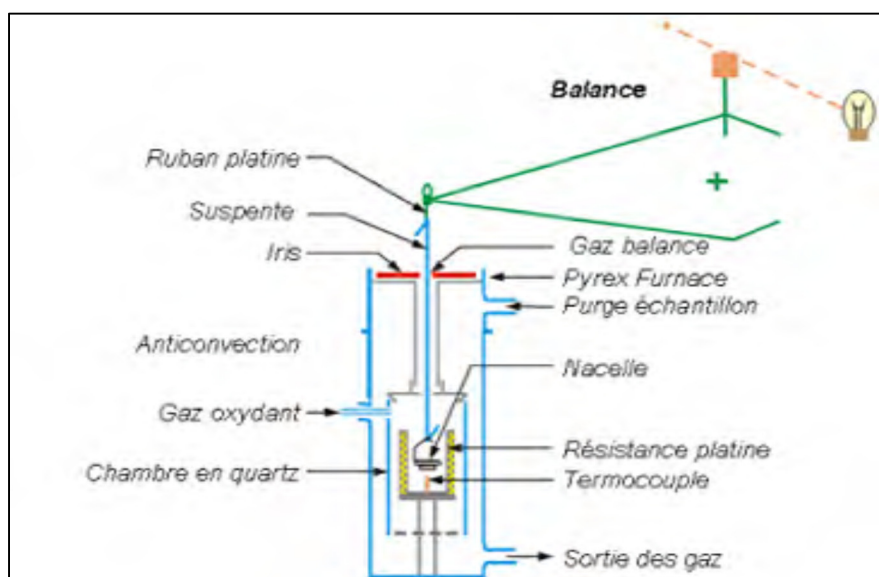
Figure 2.20 Principe de mesure thermogravimétrique Tirée de Zazoum (2014)
