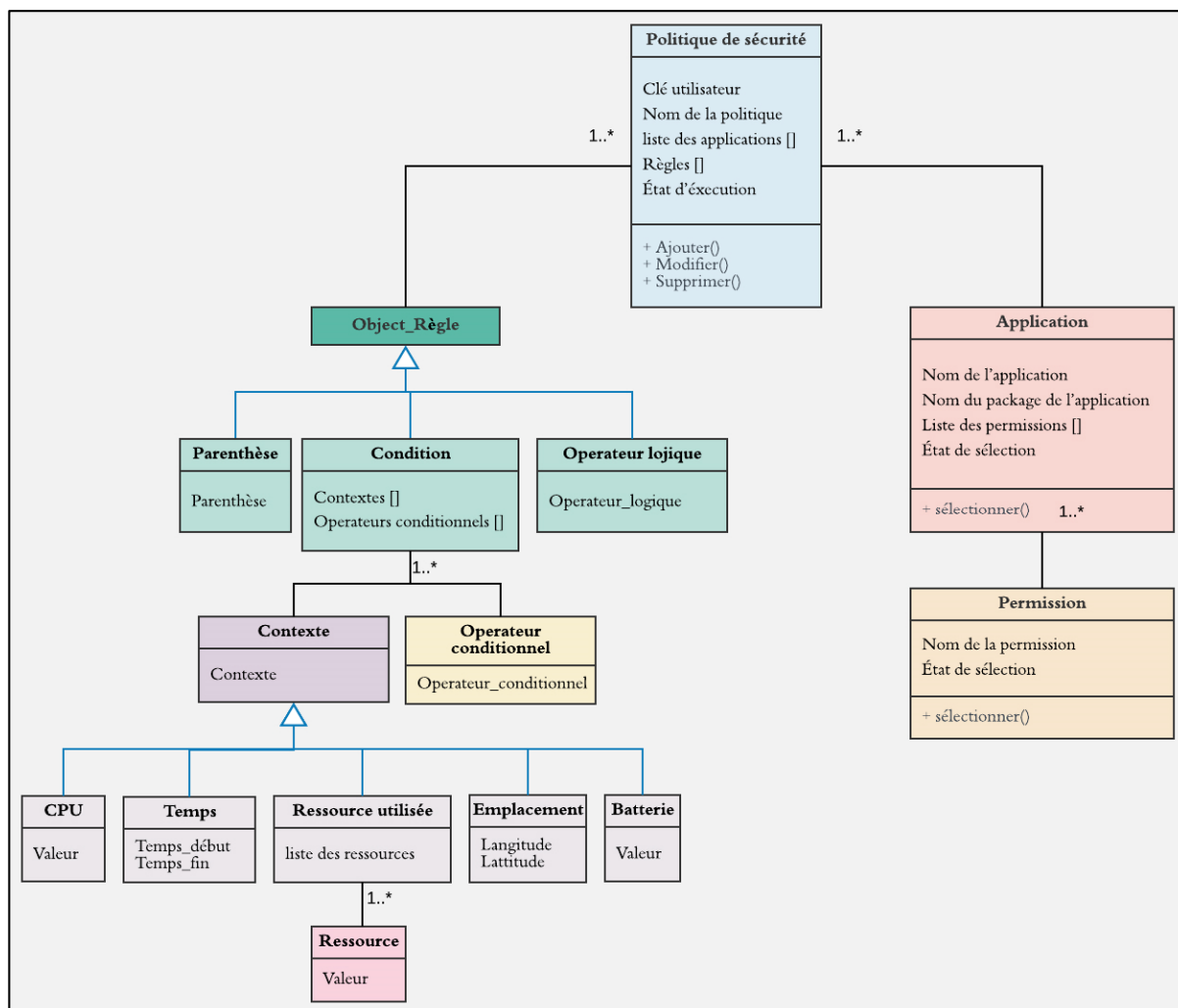
Figure 3.4 Diagramme de classe de la solution APSL
