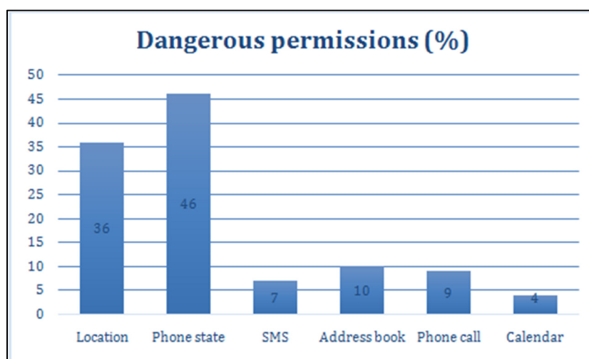
Figure 1.12 La prévalence des autorisations dangereuses des applications Android (Gandhi, 2014)
