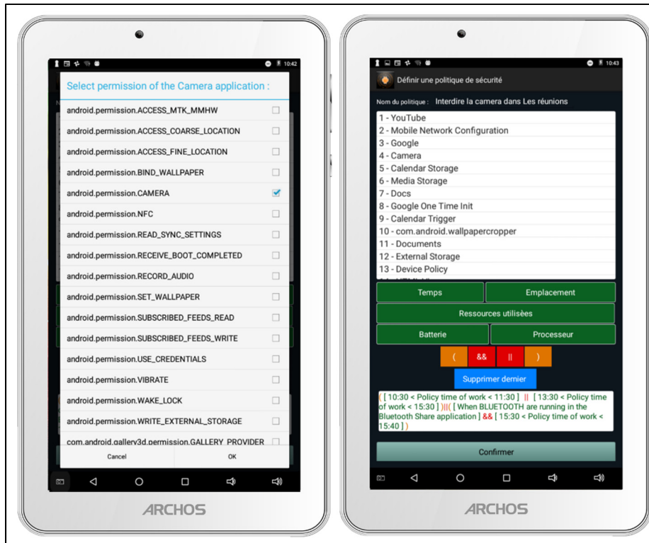
Figure 3.14 Exemple de définition d'une politique de sécurité
