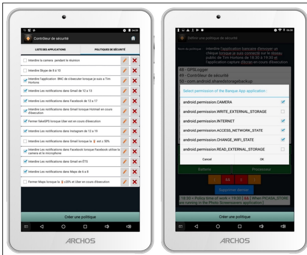
Figure 3.16 L'interface de gestion des politiques de sécurité
