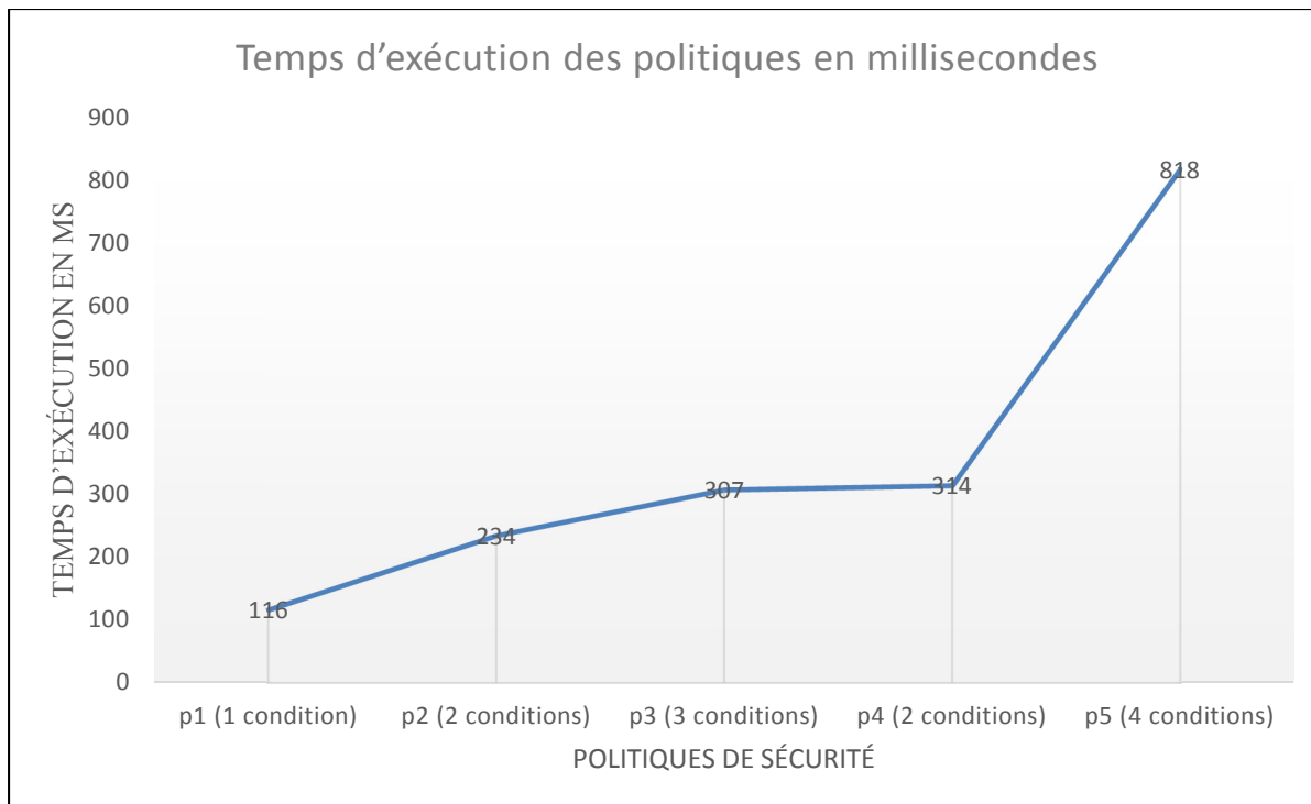
Figure 4.4 Temps d'exécution pour chacune des politiques utilisées
