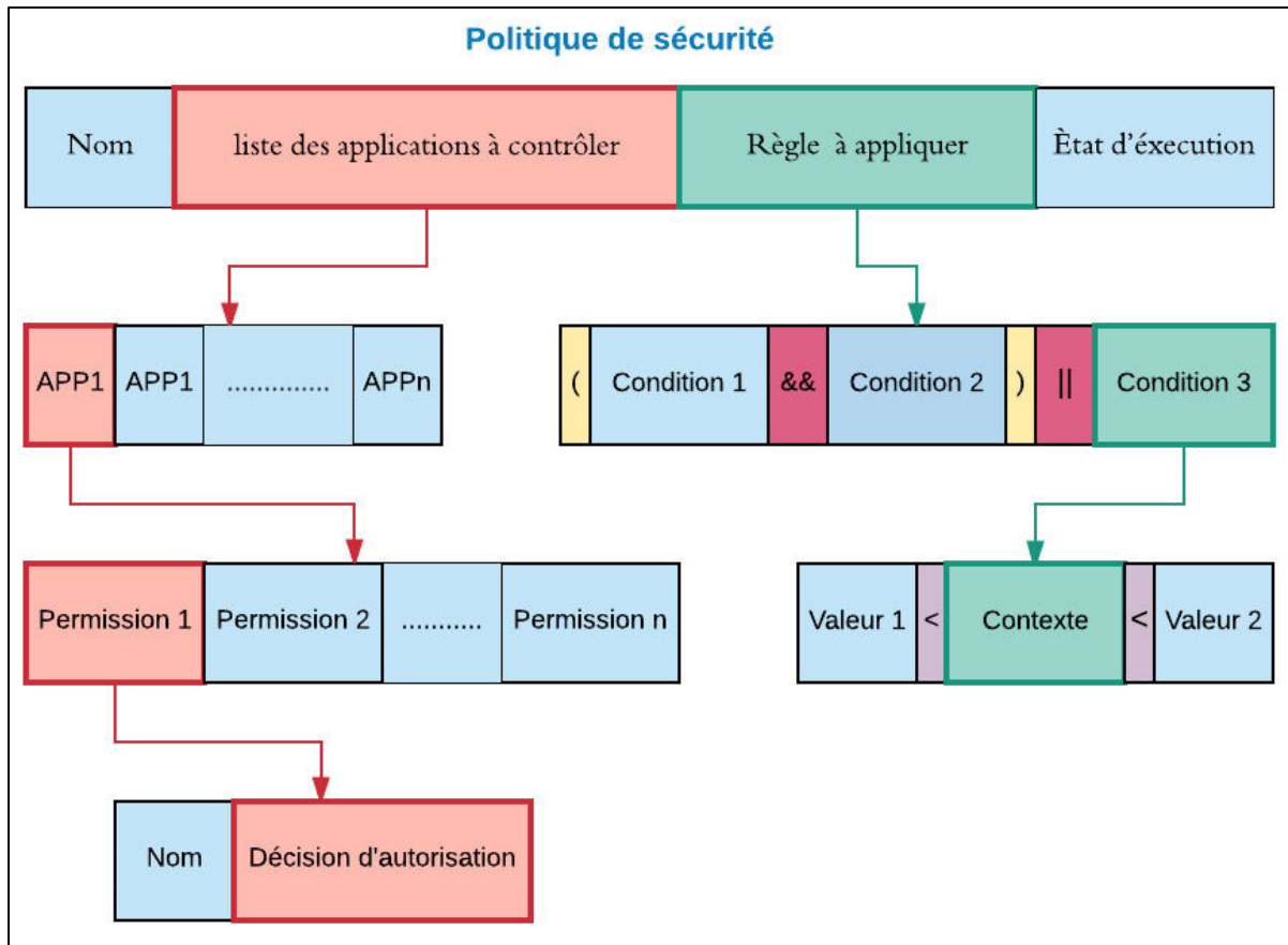
Figure 3.13 Le format principal d'une politique de sécurité
