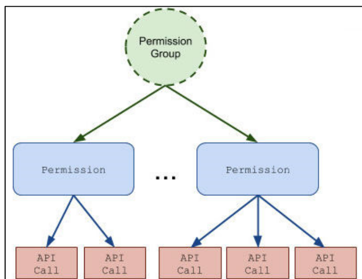
Figure 1.11 Les groupes des permissions des APIs sur Android (Google , 2017)
