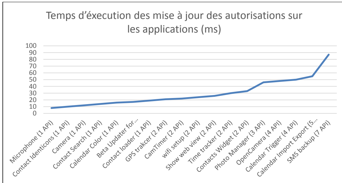
Figure 4.1 Temps d'exécution de la mise à jour des autorisations pour chaque application
