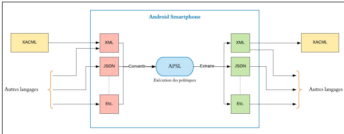
Figure 3.17 Importation et exportation des politiques de sécurité
