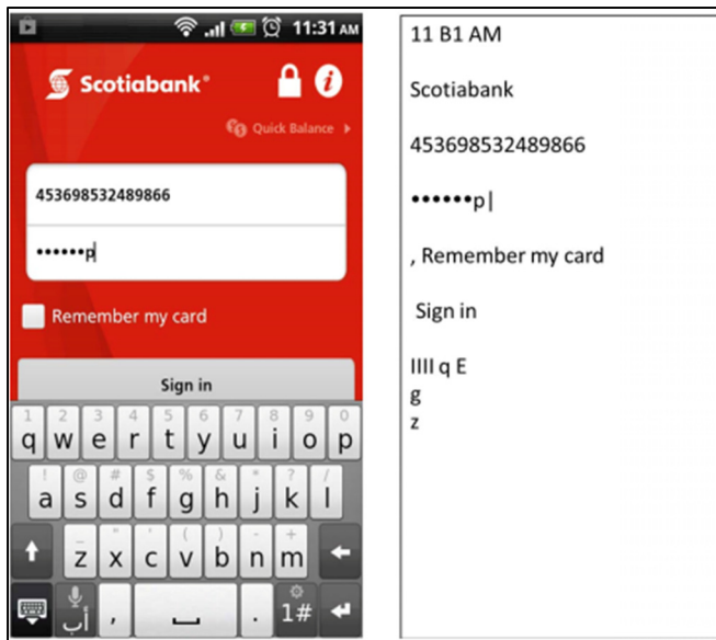
Figure 2.1 Les résultats de la phase d'analyse par OCR (El-Serngawy & Talhi, 2015)
