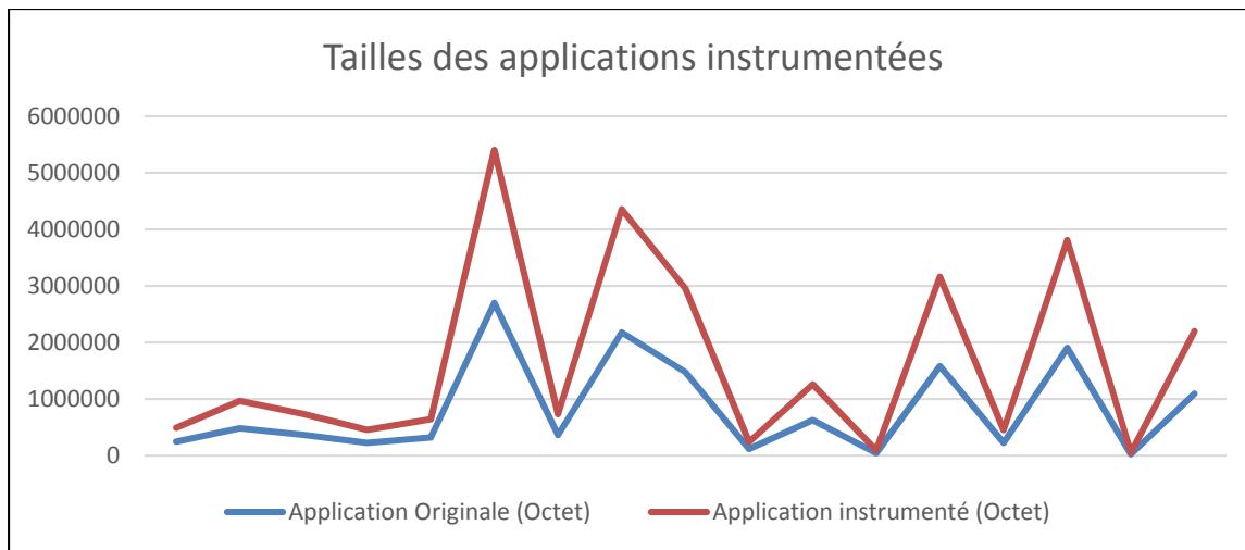
Figure 4.2 Taille des applications avant et après la réécriture
