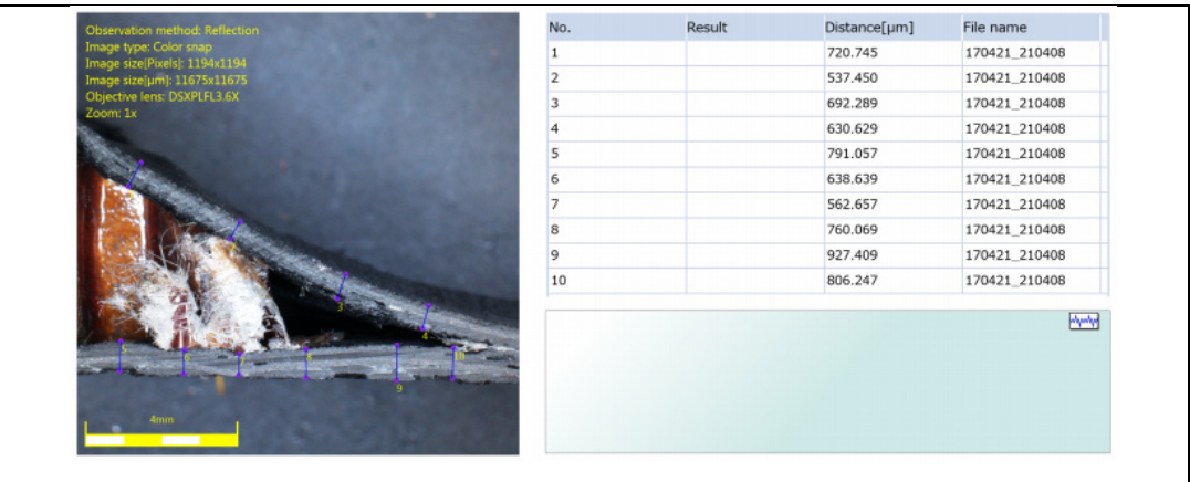
Figure 3.13 Observation microscopique de l’angle de lèvre : découpe à 30 degrés
