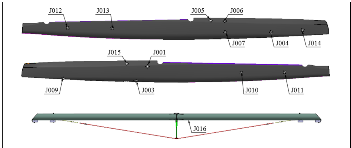
Figure 6.7 Position des jauges (échelle non respectée)
