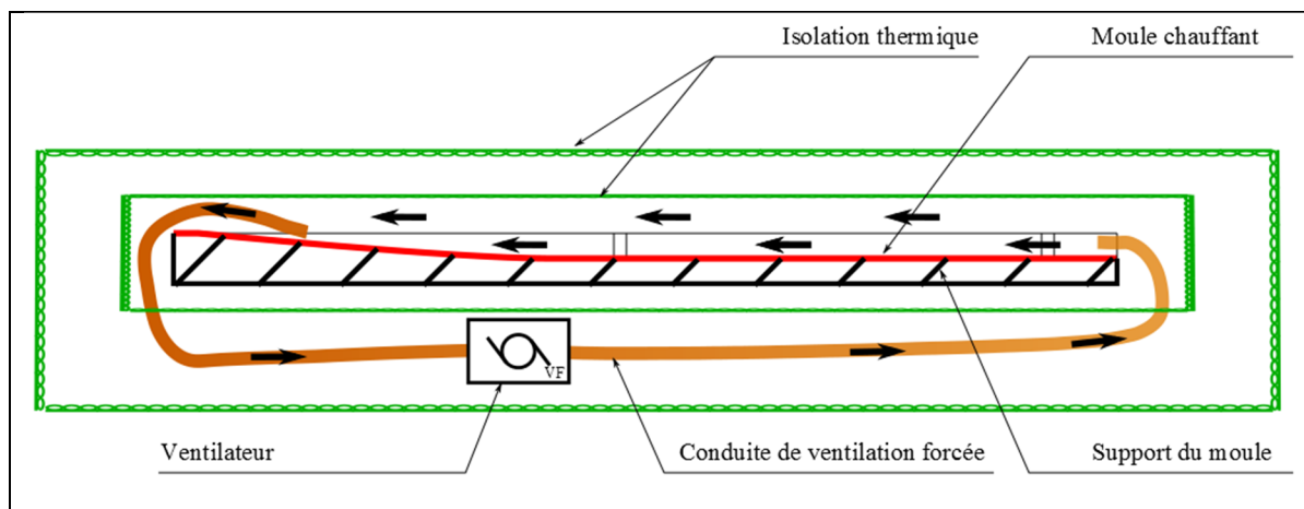
Figure 5.7 Montage de cuisson
