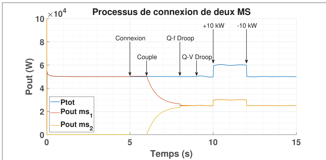
Figure 5.4 Procédure de test pour deux machines synchrones
