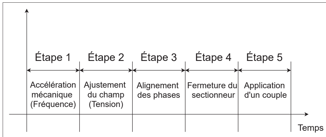
Figure 2.5 Étapes de mise en parallèle de deux générateurs synchrones
