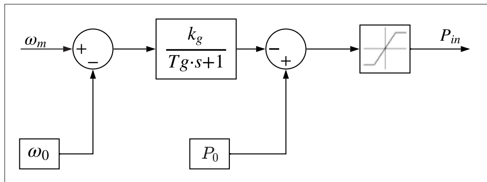
Figure 3.4 Détails du bloc Régulateur
