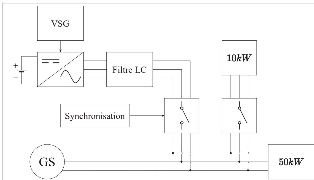
Figure 5.2 Circuit de simulation cas n° 2
