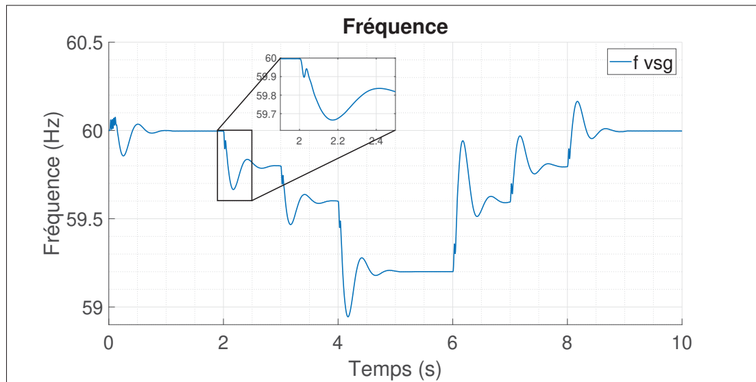
Figure 4.8 Réponse en fréquence aux surcharges
