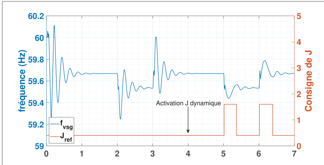
Figure 5.20 Réponse en fréquence avant et après activation d'un moment d'inertie dynamique
