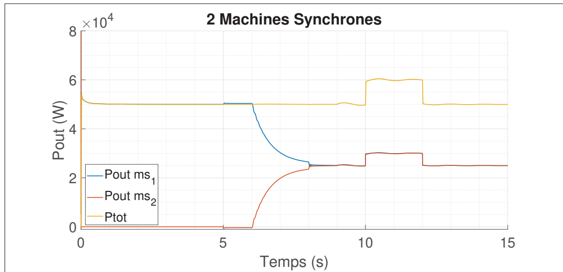
Figure 5.10 Réponse en puissance pour le cas n° 1
