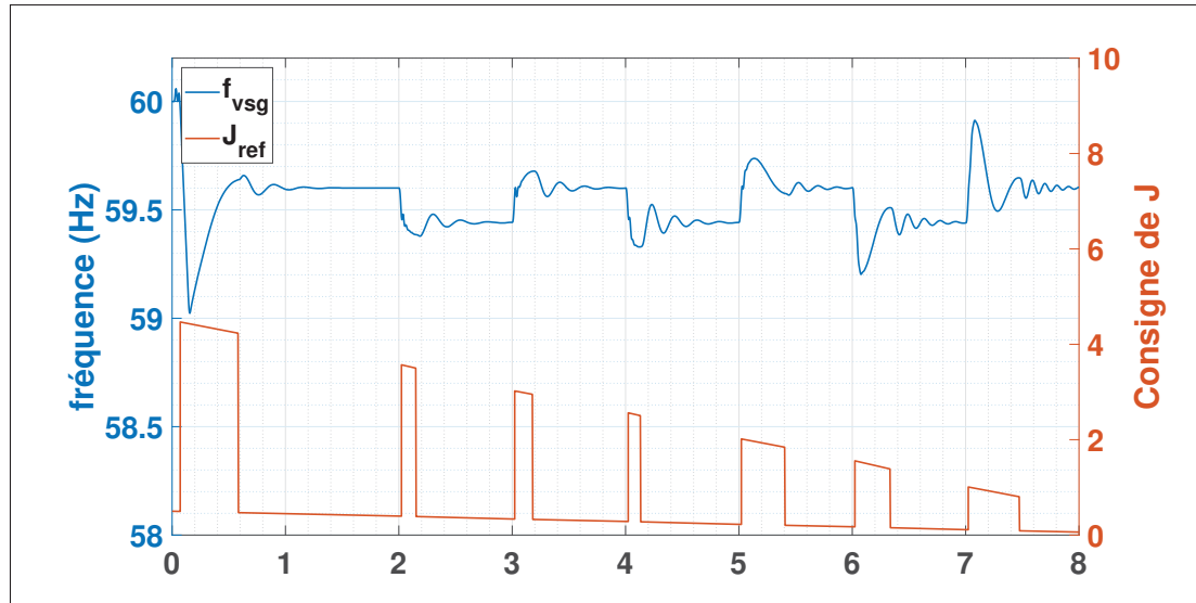
Figure 5.24 Fréquence et moment d'inertie dynamique en réponse à 3 surcharges de 5kW
