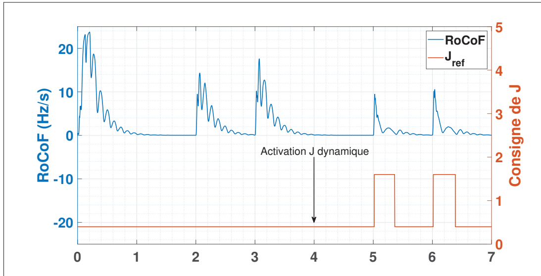
Figure 5.19 RoCoF avant et après activation d'un moment d'inertie dynamique
