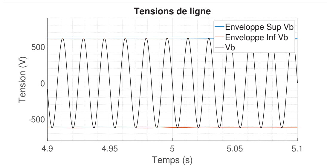
Figure 4.6 Envelopes de la tension V_b en réponse à 2 surcharges
