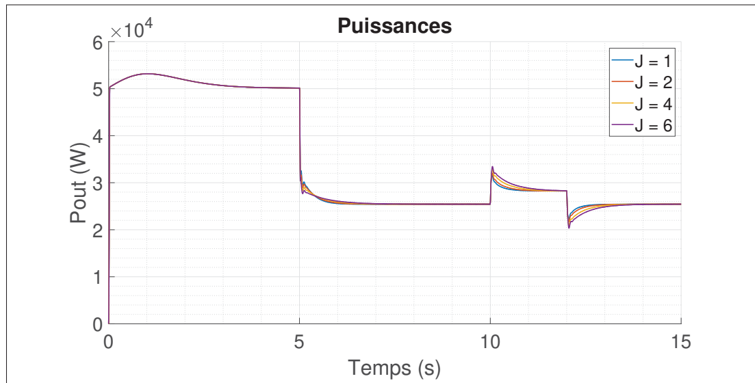
Figure 5.17 Puissances mesurées pour une variation de J
