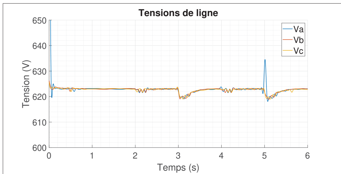
Figure 4.5 Maxima des tensions en réponse à 2 surcharges
