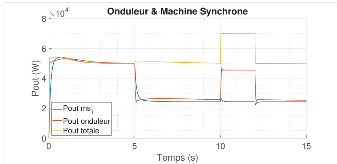
Figure 5.12 Réponse en puissance pour le cas n° 3
