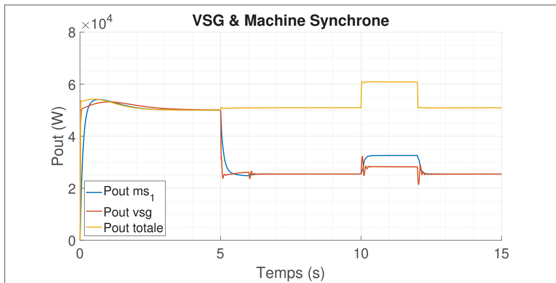
Figure 5.11 Réponse en puissance pour le cas n° 2
