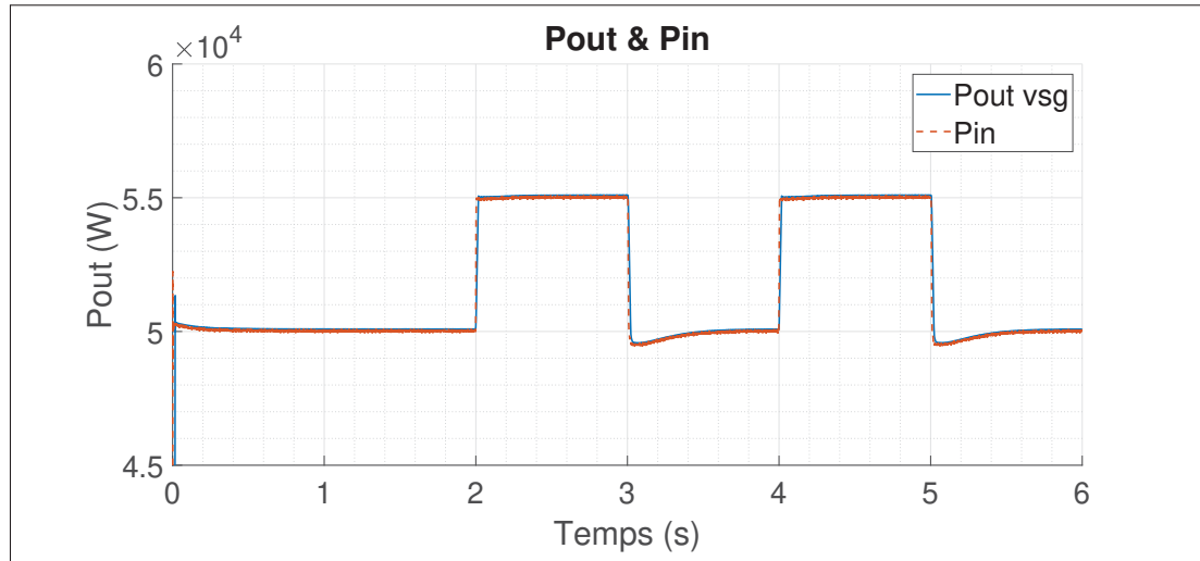
Figure 4.4 Puissance du VSG en réponse à deux surcharges
