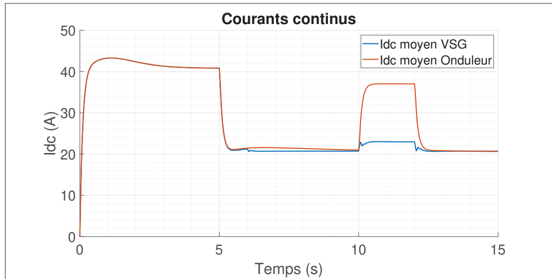
Figure 5.13 Courants continus pour les trois cas
