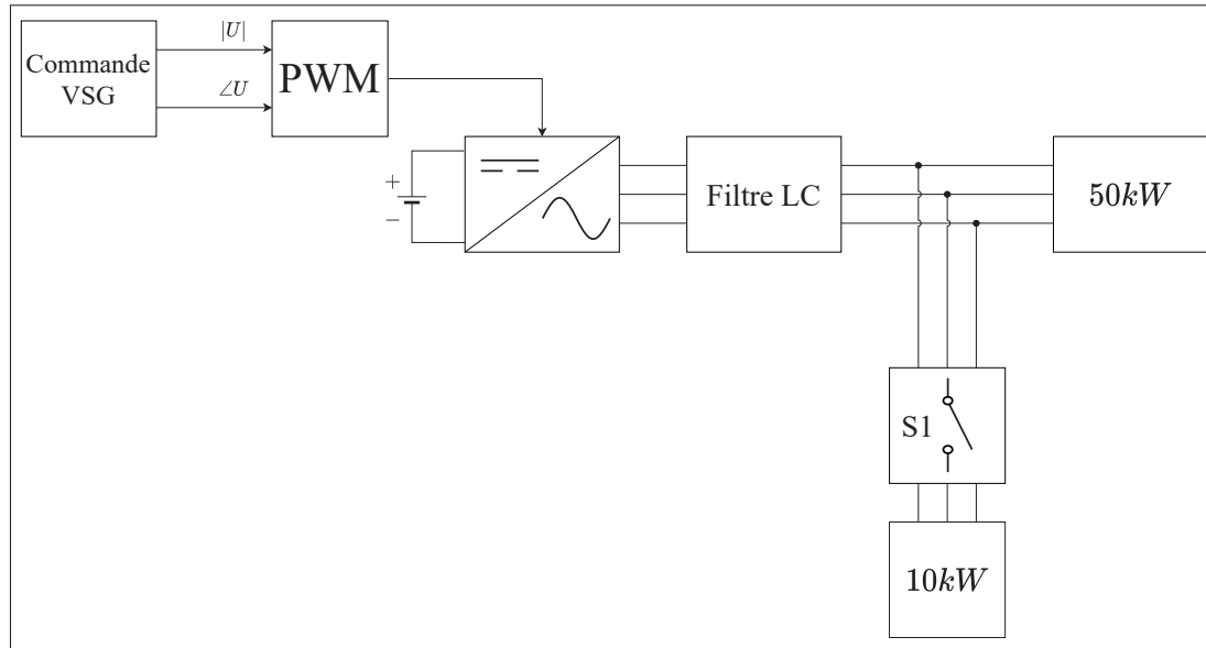
Figure 4.1 Schéma de simulation du VSG seul
