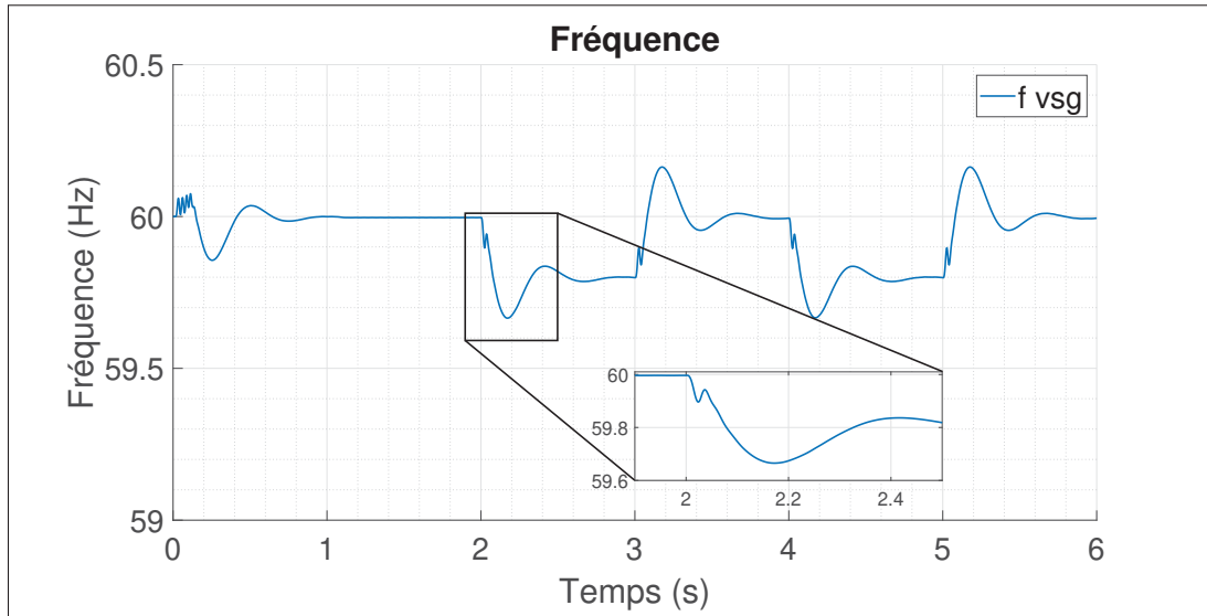
Figure 4.2 Fréquence du VSG en réponse à une surcharge
