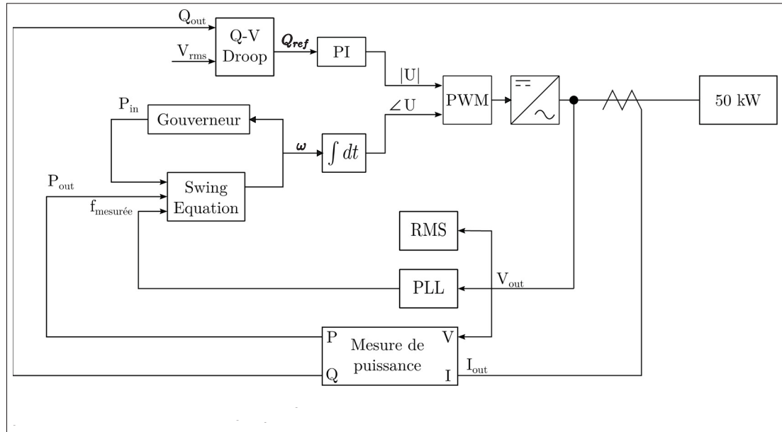
Figure 3.2 Schéma de la commande VSG
