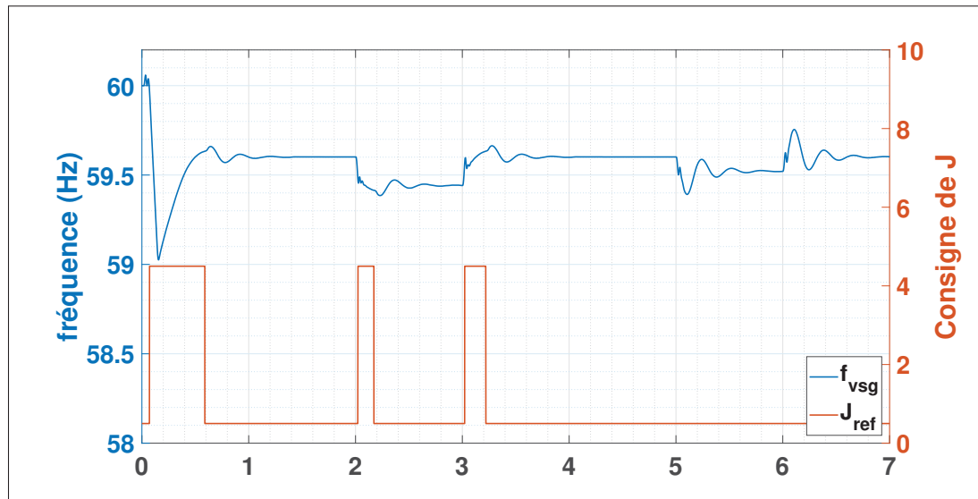
Figure 5.22 Fréquence et consigne de J en réponse à deux surcharges de 10kW puis 5 kW
