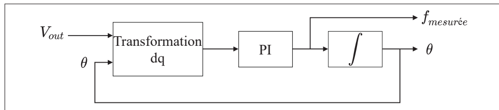
Figure 3.3 Schéma bloc de la boucle à verrouillage de phase
