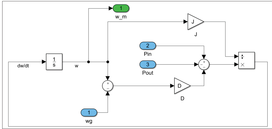
Figure 4.7 Schéma bloc de l'équation du mouvement
