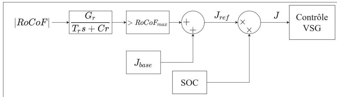
Figure 5.18 Schéma bloc du moment d'inertie dynamique
