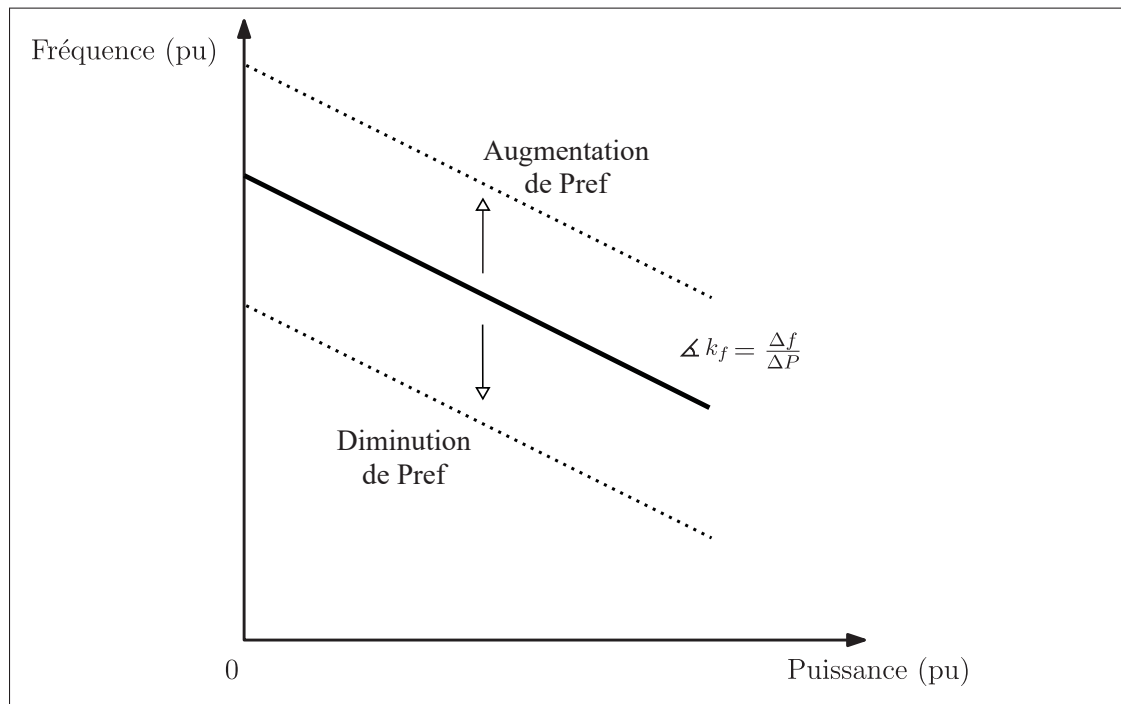
Figure 2.2 Effet de l'ajout d'une puissance de référence sur la courbe de statisme
