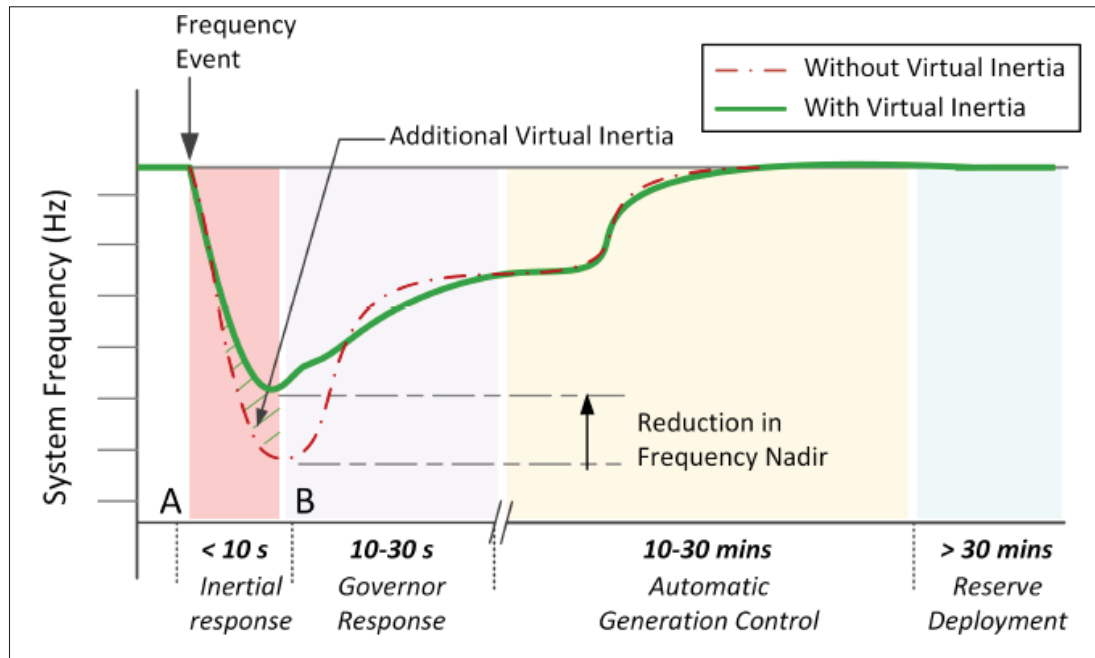
Figure 1.1 Mécanismes de réponses à une perturbation en fonction du temps Tirée de Tamrakar et al. (2017)
