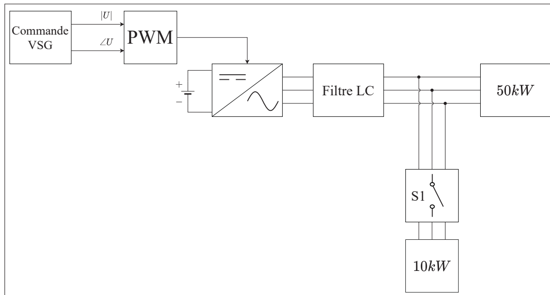
Figure 3.1 Schéma de simulation du modèle
