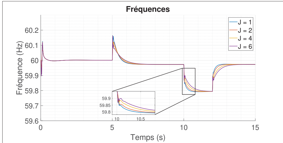
Figure 5.16 Fréquences mesurées pour une variation de J
