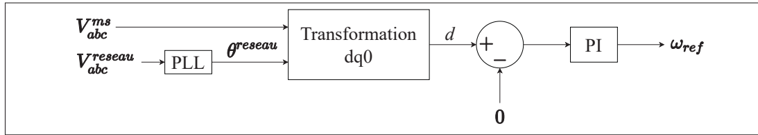
Figure 2.7 Régulation de l'axe d pour aligner les phases
