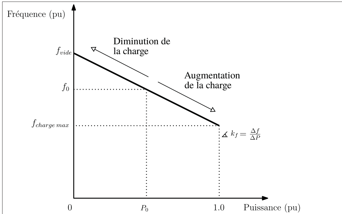
Figure 2.1 P-f contrôle Droop
