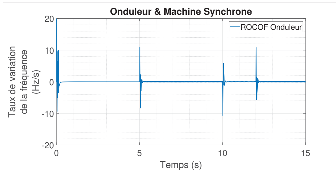
Figure 5.9 Taux de variation de la fréquence pour le cas n° 3
