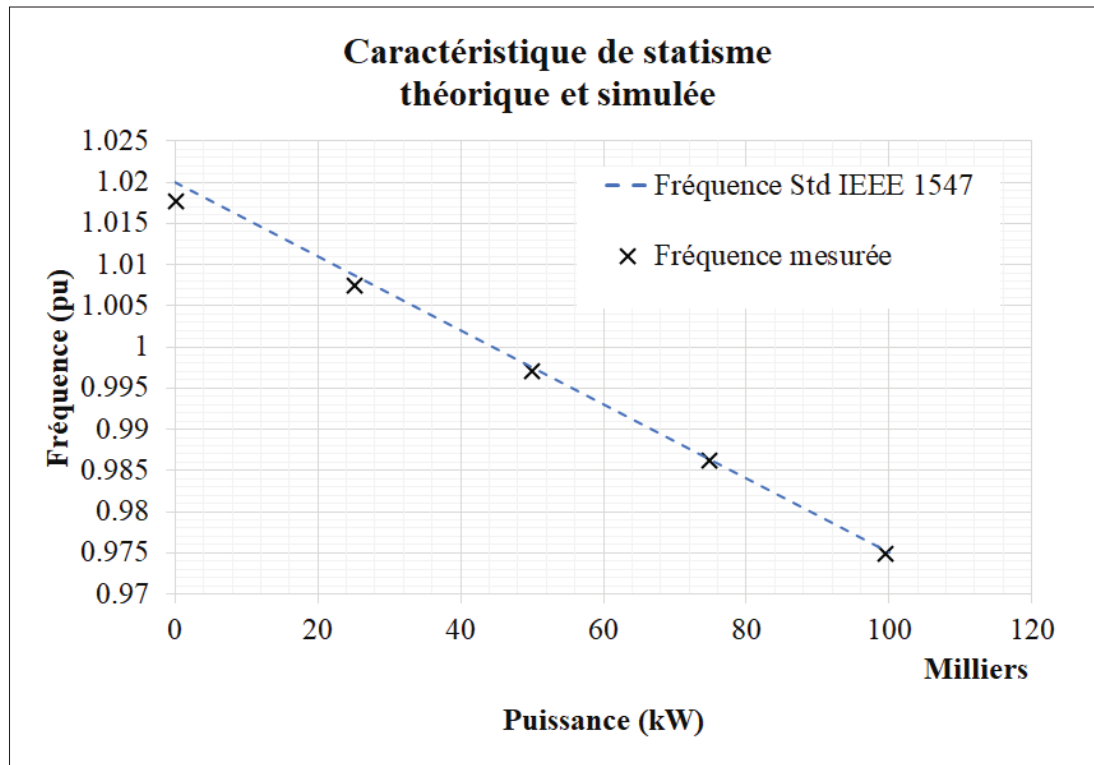
Figure 2.3 Comparaison des caractéristiques de statisme théorique et simulée de la fréquence
