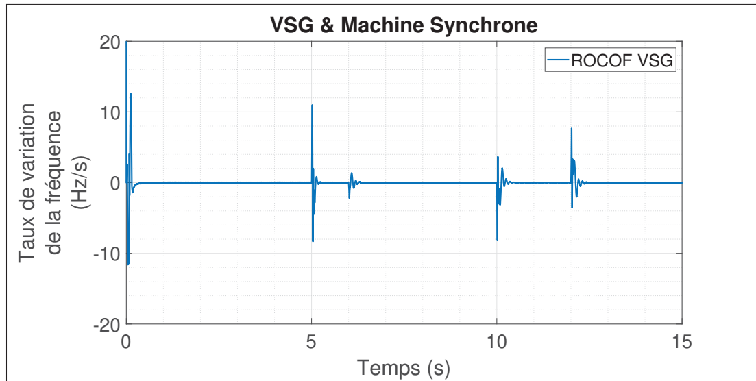
Figure 5.8 Taux de variation de la fréquence pour le cas n° 2
