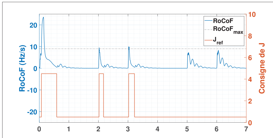
Figure 5.21 RoCoF et consigne de J en réponse à deux surcharges de 10kW puis 5 kW
