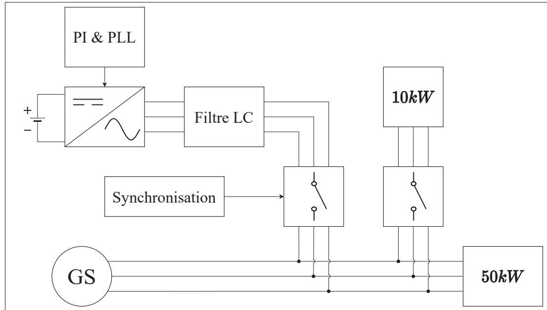
Figure 5.3 Circuit de simulation cas n° 3
