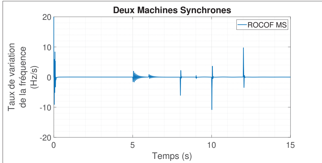
Figure 5.7 Taux de variation de la fréquence pour le cas n° 1
