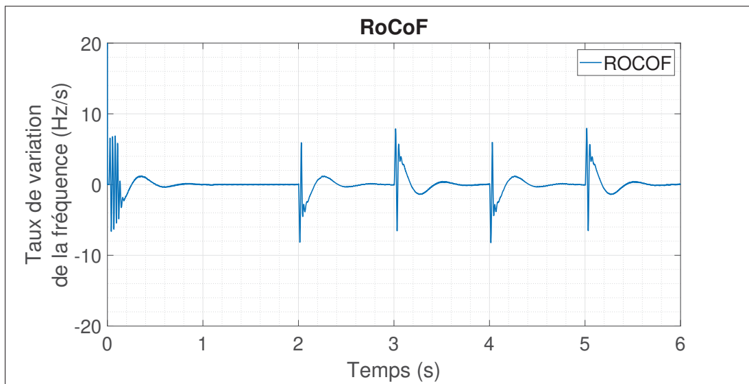
Figure 4.3 RoCoF du VSG en réponse à une surcharge
