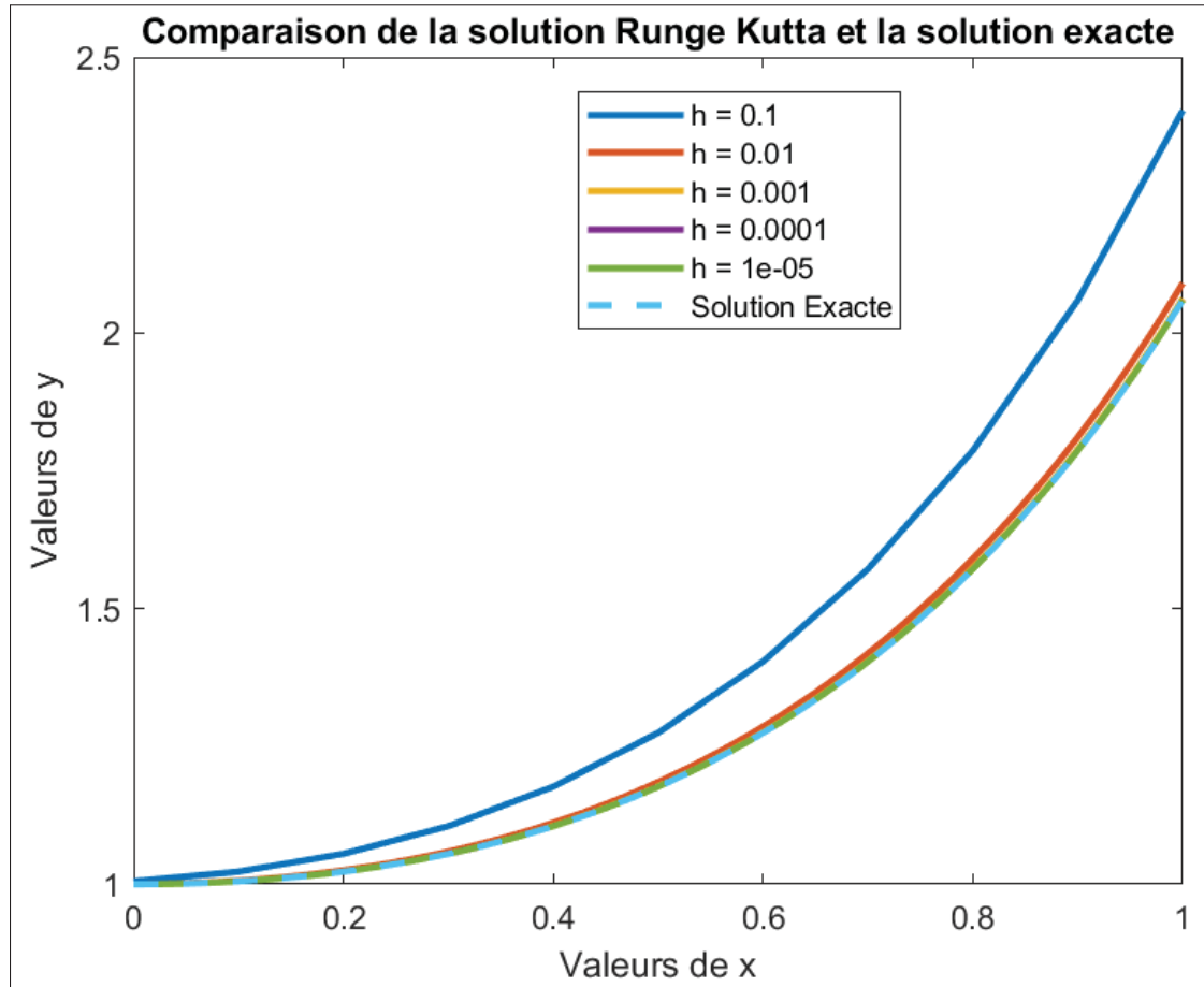
Figure 3.8 Comparaison des différentes résolutions sous Simulink
