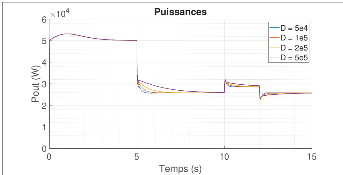
Figure 5.15 Puissances mesurées pour une variation de D
