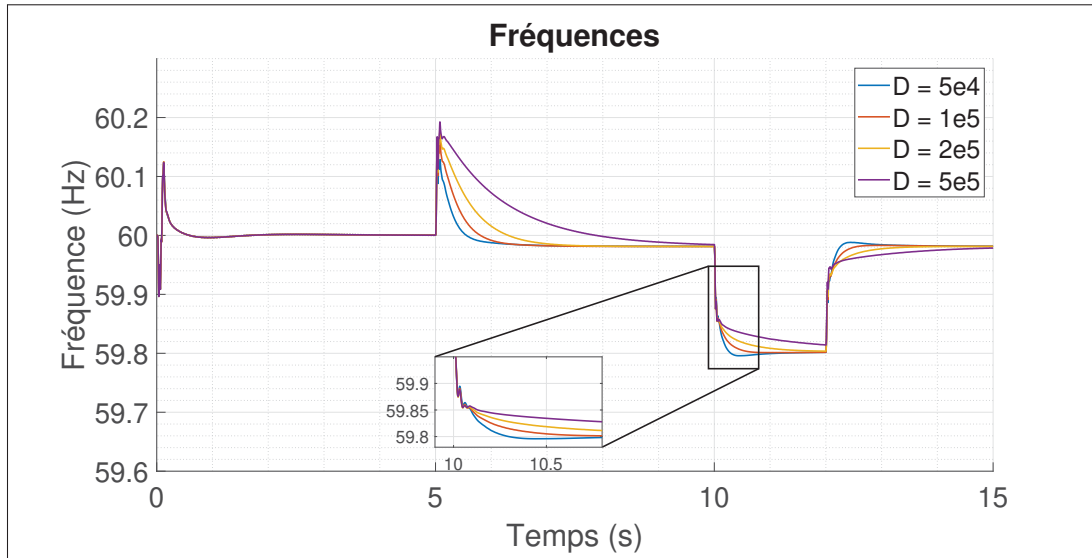
Figure 5.14 Fréquences mesurées pour une variation de D
