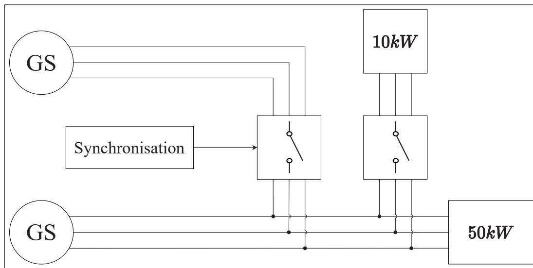
Figure 5.1 Circuit de simulation cas n° 1
