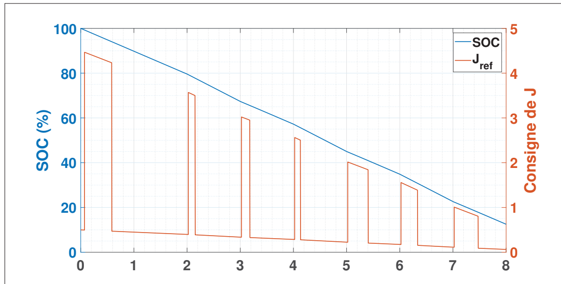
Figure 5.23 État de charge et moment d'inertie dynamique en réponse à 3 surcharges de 5kW
