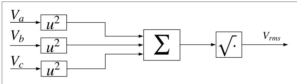
Figure 3.6 Détails du bloc de mesure de la tension RMS
