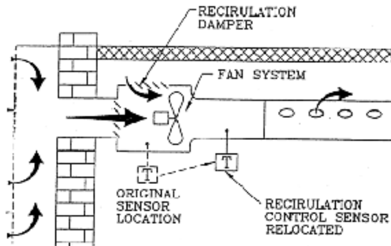
Figure 3.3 Système de contrôle de la température. Tirée de (Shc. IEA, 1999)
