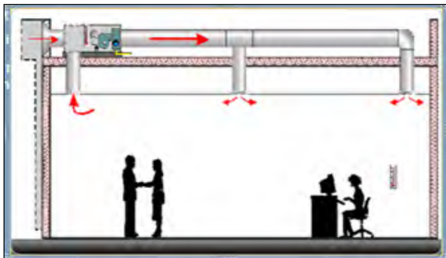
Figure 3.4 Chauffage solaire de l'air, pour bâtiment commercial et résidentiel.
