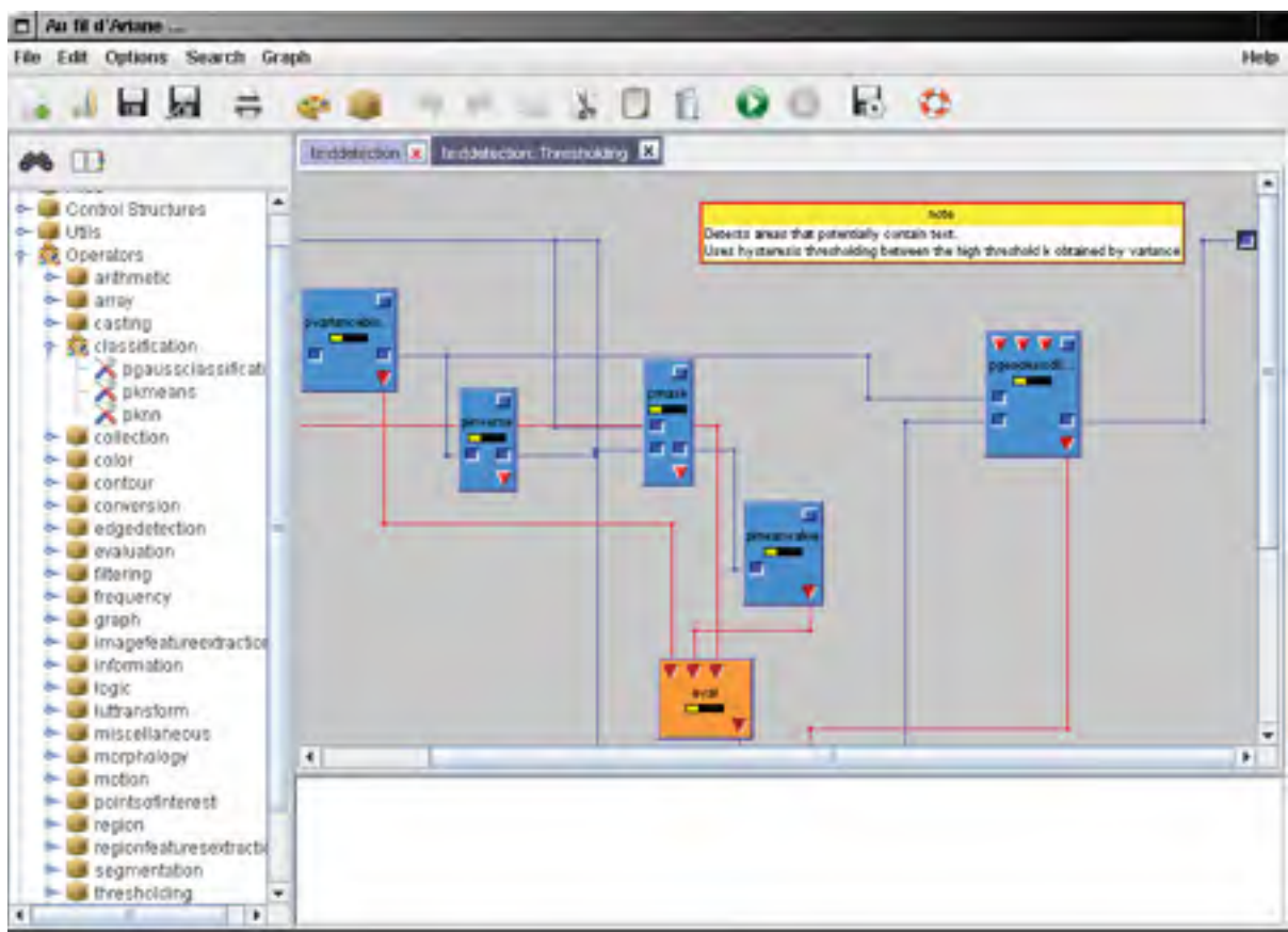
Figure 4.7 Exemple de l'interface Ariane pour Pandore.
