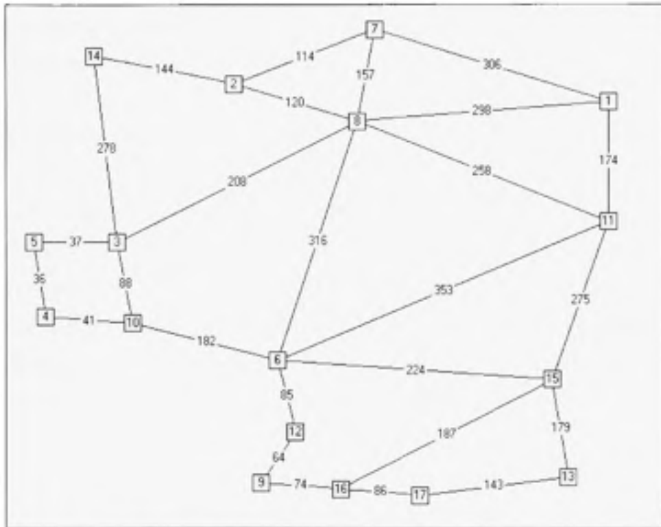
Figure 4.7 Topologie du réseau allemand à 17 nœuds (Betker et al., 2004).
