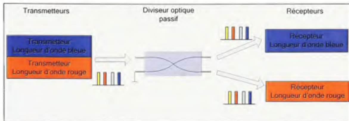
Figure 3.11 Comportement spectral d'un diviseur optique passif.
