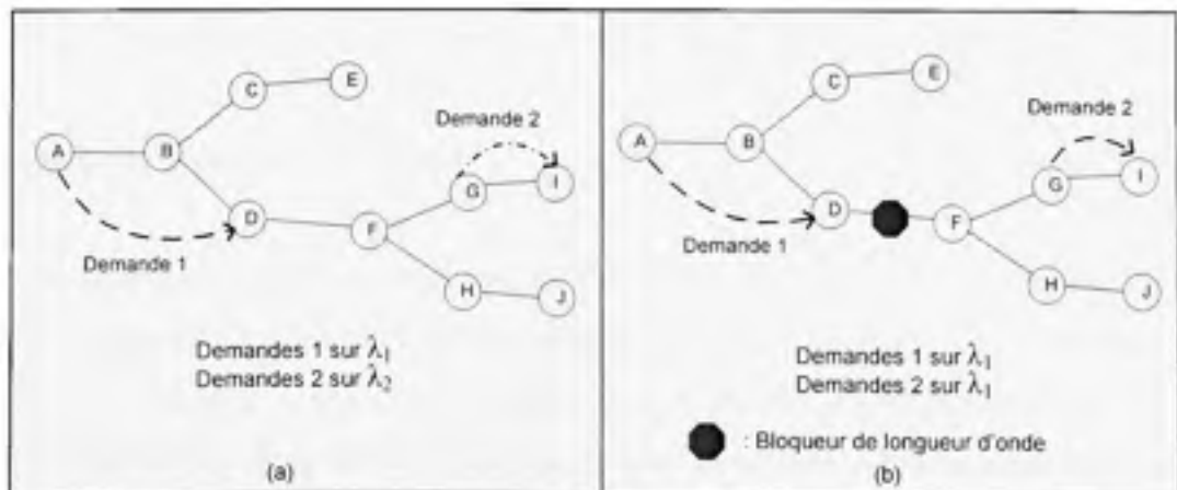
Figure 3.10 Insertion d'un bloqueur de longueurs d'onde dans un arbre de fibres.
