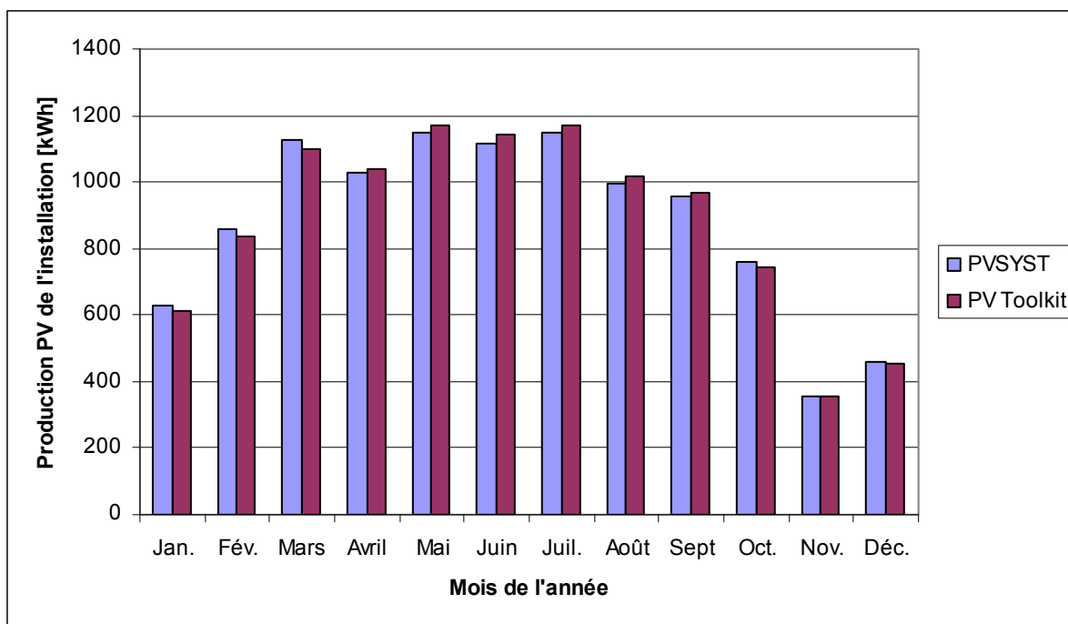
Figure 4.2 Évolution de la production PV sur une année pour 100 panneaux CS5C-85M; pente 37 degrés, azimut 0 degré.
