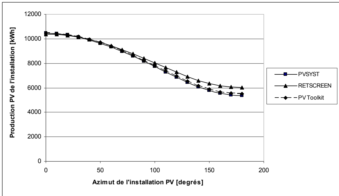
Figure 4.5 Évolution de la production PV annuelle [kWh] en fonction de l'azimut pour 100 panneaux PhotoWatt 750 / 80W; pente 37 degrés.
