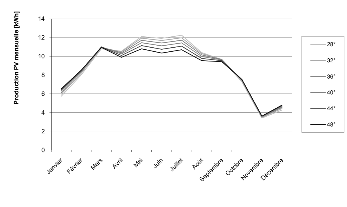
Figure IV.1 Évolution de la production d'électricité PV mensuelle [kWh] en fonction de la pente de l'installation.
