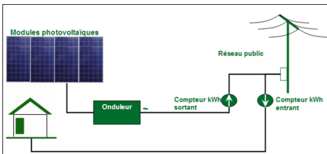
Figure 1.1 Schéma d'un système photovoltaïque relié au réseau. Tirée de LVM Solaire (2007)
