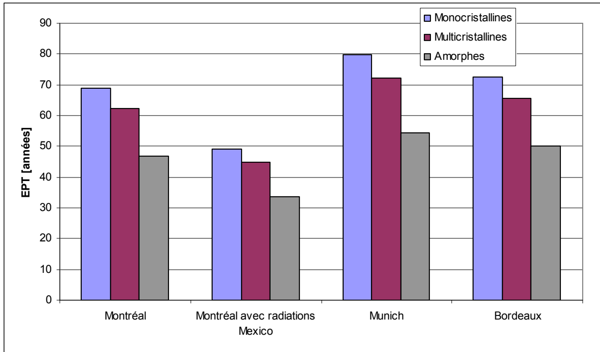
Figure 5.2 Évolution du EPT [années] en fonction de la localisation de l'installation et du type de cellules.
