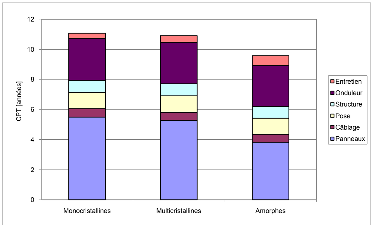
Figure VII.1 Répartition de la période de retour économique (CPT) de l'installation PV en fonction de ses différents composants
