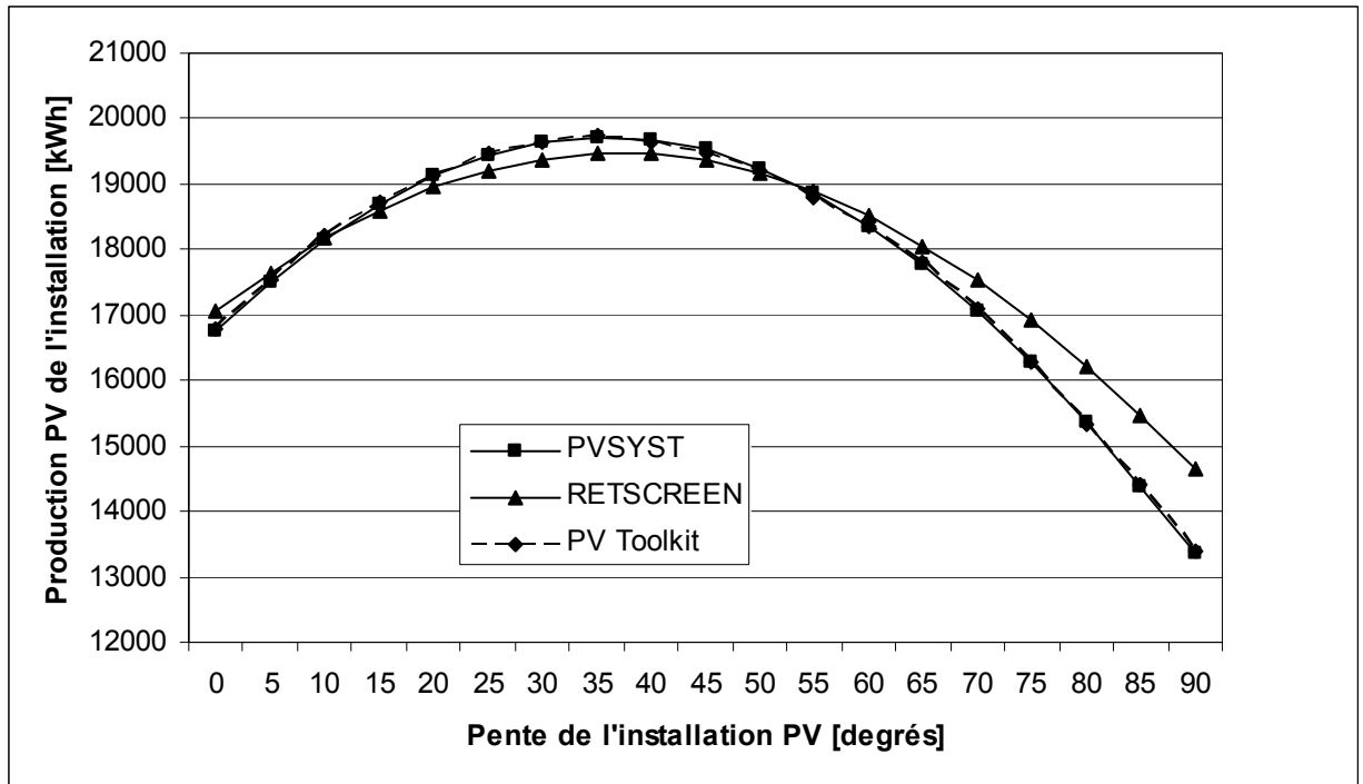
Figure 4.4 Évolution de la production PV annuelle en fonction de la pente pour 100 panneaux Shell SQ 150 C; azimut 0 degré.
