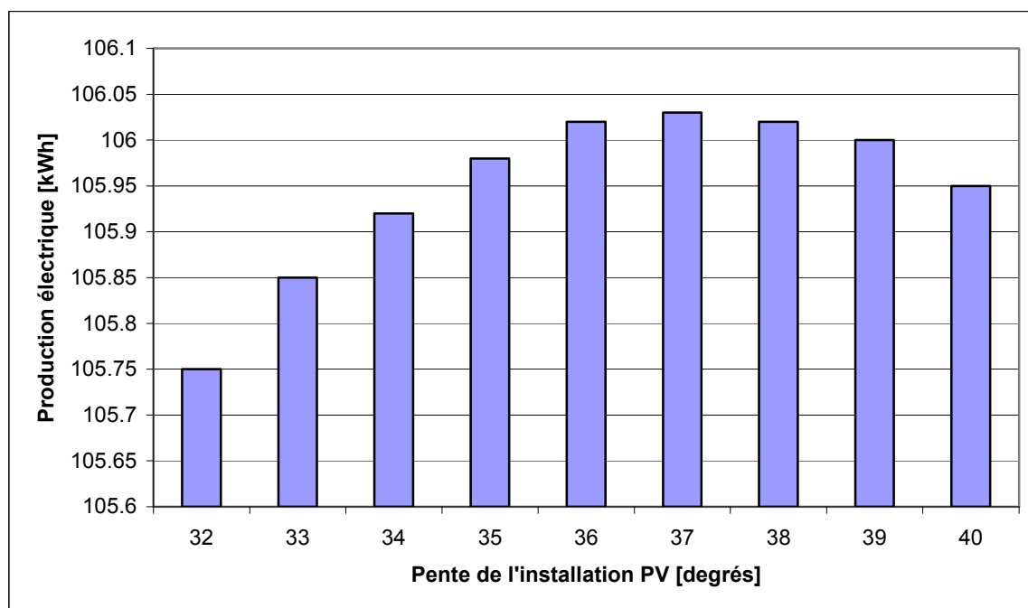
Figure IV.2 Évolution de la production d'électricité PV mensuelle [kWh] en fonction de la pente de l'installation.
