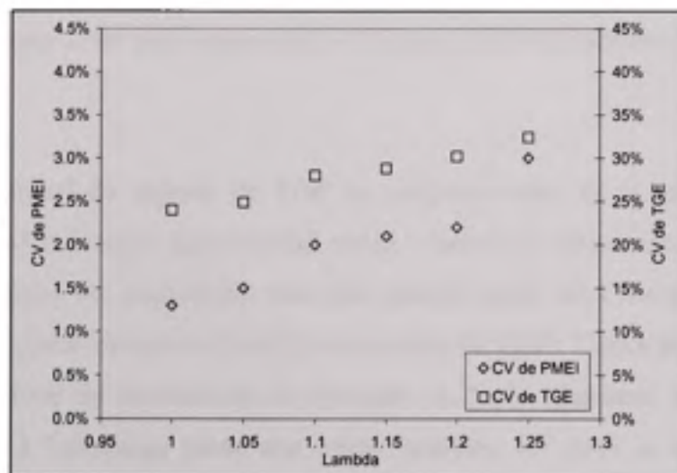
Figure 3.14 Effet de la vitesse, CV de PMEI et de TGE. Tests réalisés à 1500 tr/min, 40 N.m, avance MBT.
