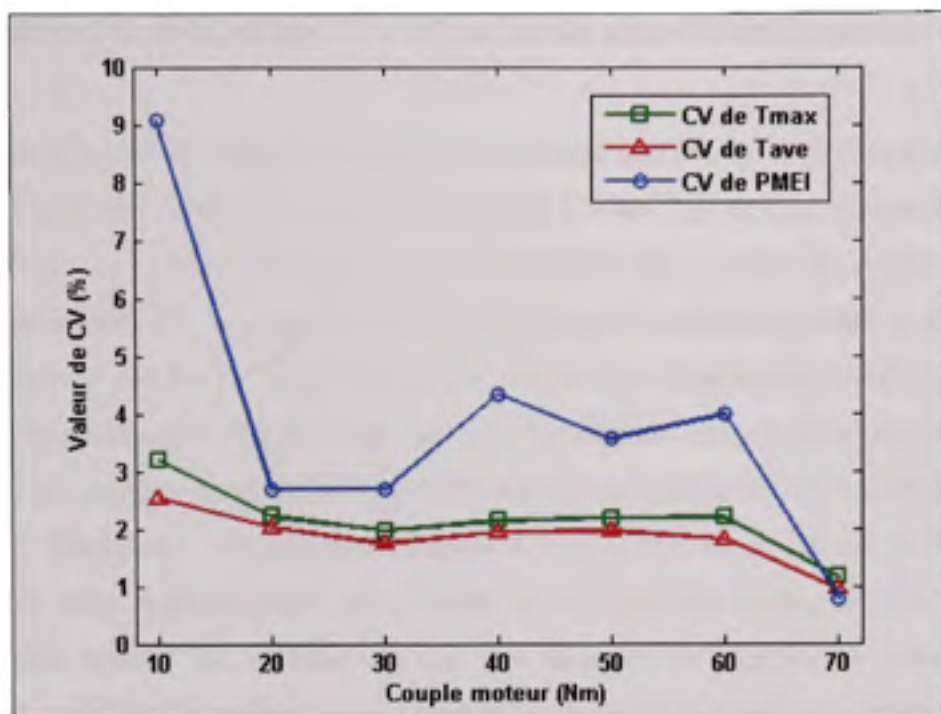
Figure 4.14 CV de PMEI, Tmax et de Tmoy en fonction du couple moteur, 1500 rpm, \lambda=1.10 , avance MBT.
