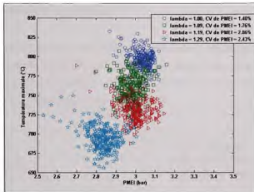
Figure 4.10 Valeurs cycle-à-cycle de PMEI et de Tmax, thermocouple de 25.4 \mu\text{m} , 1500 tr/min, \lambda=1.00 , 262 kPa de PMEI et avance MBT.
