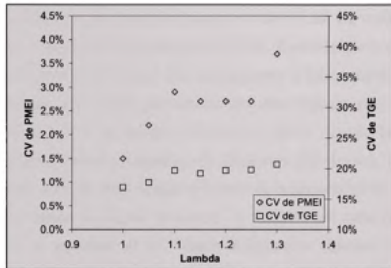
Figure 3.13 Effet de la vitesse, CV de PMEI et de TGE. Tests réalisés à 1000 tr/min, 40 N.m, avance MBT.
