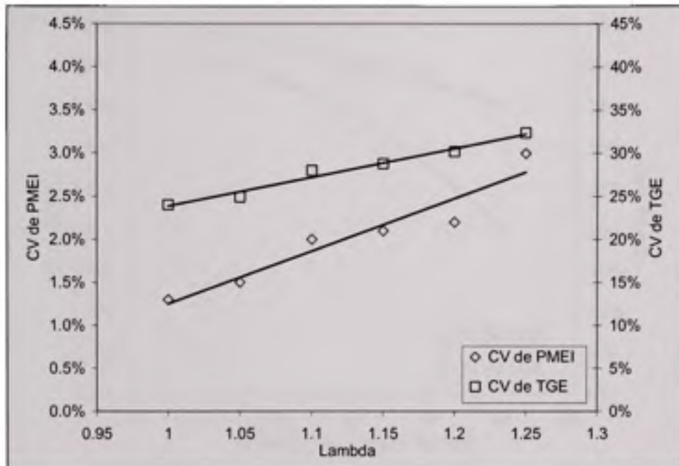
Figure 3.8 Effet du coefficient d'excès d'air, CV de PMEI et de TGE. Test réalisé à 1500 tr/min, 40 N.m et \lambda = 1.1 .
