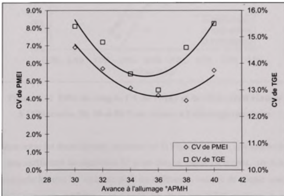
Figure 3.10 Effet de l'avance à l'allumage, CV de PME1 et de TGE. Test réalisé à 1000 tr/min, 30 N.m et \lambda = 1.3 .
