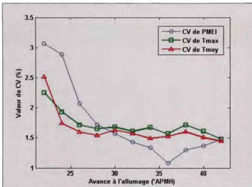
Figure 4.11 Valeurs cycle-à-cycle de PMEI et de T_{max} , thermocouple de 25.4 \mu\text{m} seulement, 1500 tr/min, \lambda=1.00 , 262 kPa de PMEF et avance MBT.
