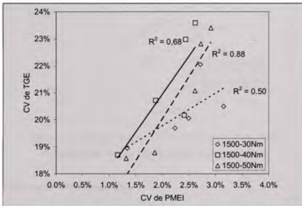
Figure 3.11 Effet du couple, CV de PME1 et de TGE. Tests réalisés à 1500 tr/min, 30, 40 et 50 N.m, avance à l'allumage constante.
