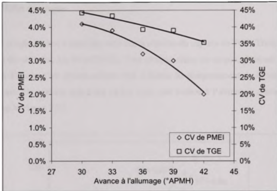
Figure 3.9 Effet de l'avance à l'allumage, CV de PME1 et de TGE. Test réalisé à 2000 tr/min, 30 N.m et \lambda = 1.1 .
