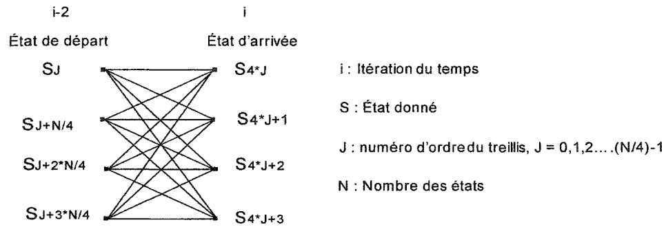
Figure 15 Forme générale de la décomposition en treillis radix-4
