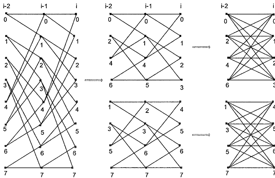
Figure 14 Décomposition du treillis de 8 états, R = 1/2 , en sous-treillis radix-4
