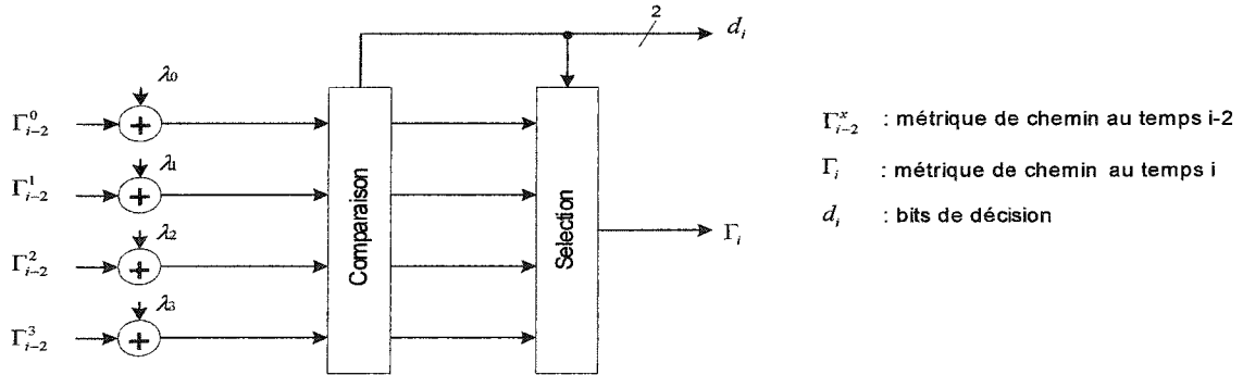
Figure 17 Bloc ACS à 4-chemins représentant un état du treillis radix-4 R = W/S où W = 1,2 et S = 1,2,3,\dots
