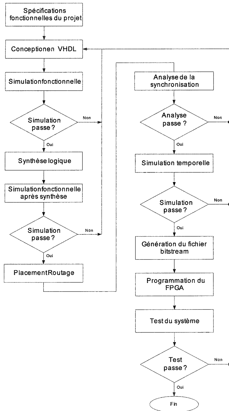
Figure 31 Organigramme du cycle du design
