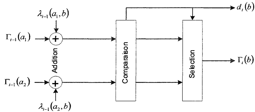
Figure 10 Réalisation d'une opération ACS pour un code de taux R = 1/S
