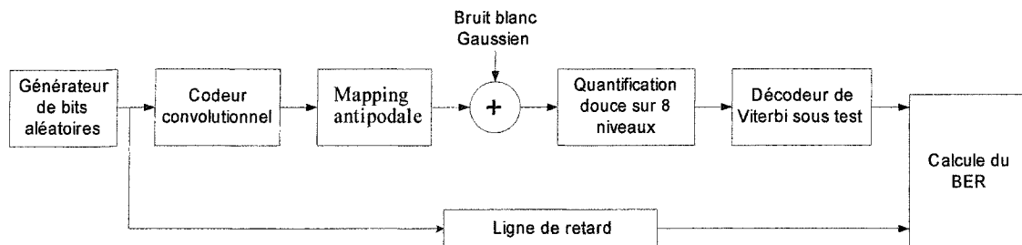
Figure 35 Illustration de l'environnement de test du décodeur.
