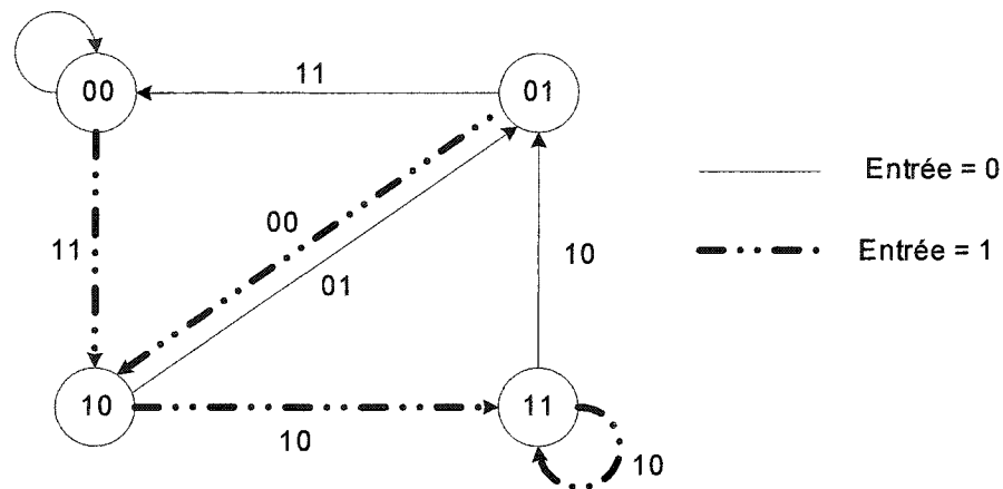
Figure 4 Représentation en machine à états finis de l'action du codeur de la figure 2
