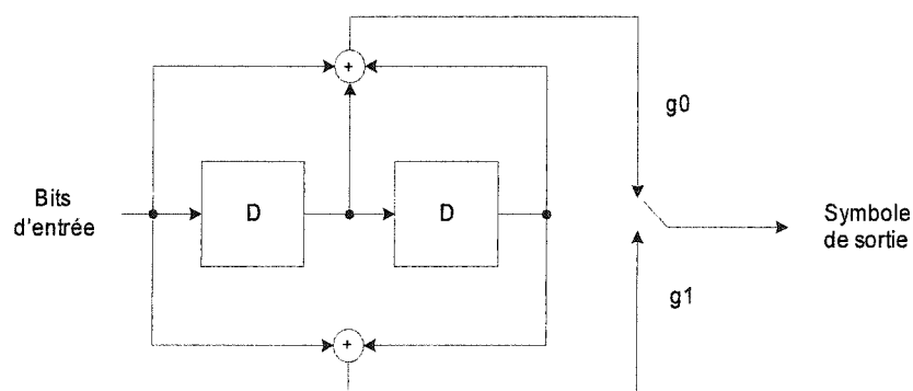
Figure 2 Codeur convolutionnel de taux R = 1/2 , de mémoire m = 2 et ayant les polynômes générateurs (7_8, 5_8)
