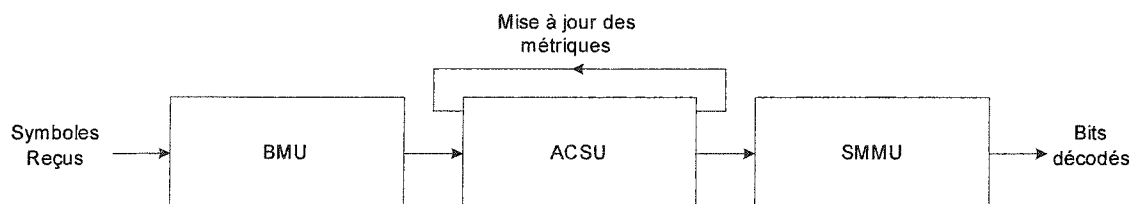
Figure 9 Diagramme bloc du décodeur de Viterbi
