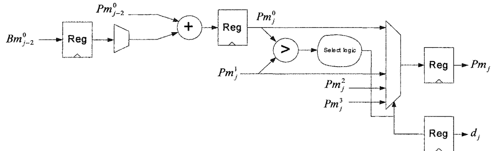
(b) Opération d'addition-comparaison-sélection avec pipeline pour les taux de R = 1/S .
