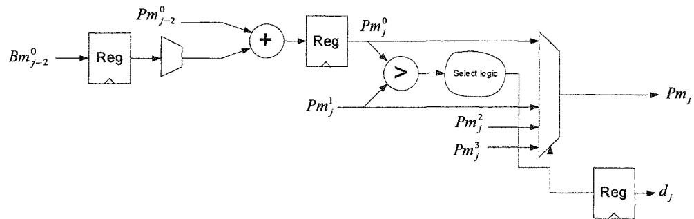
(c) Opération d'addition-comparaison-sélection avec balancement des registres pour les taux de R = 2/S .
