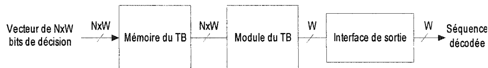
Figure 13 Schéma bloc du trace back pour un code de taux W/S et de nombre d'états N
