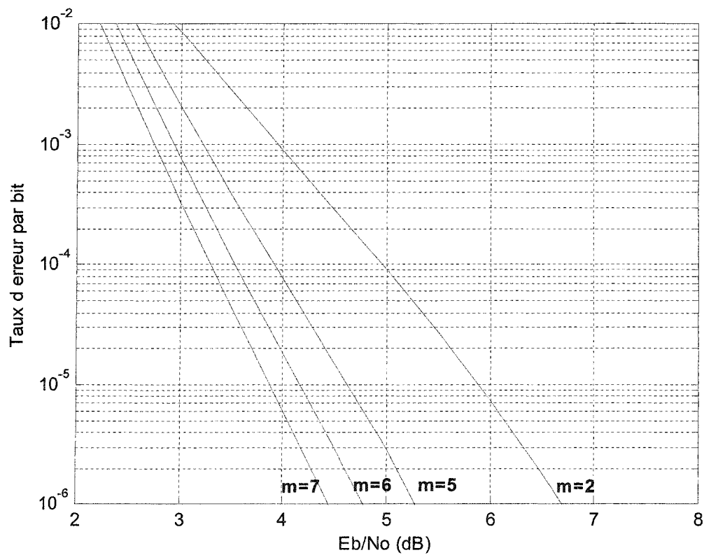
Figure 7 Performance d'erreur pour un code de taux R = 1/2 avec le décodage par l'algorithme de Viterbi à entrée non quantifiée
