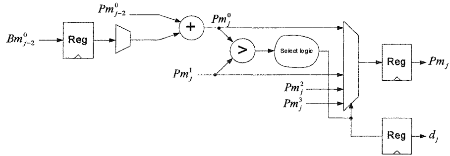
(a) Opération d'addition-comparaison-sélection sans amélioration pour la vitesse.
