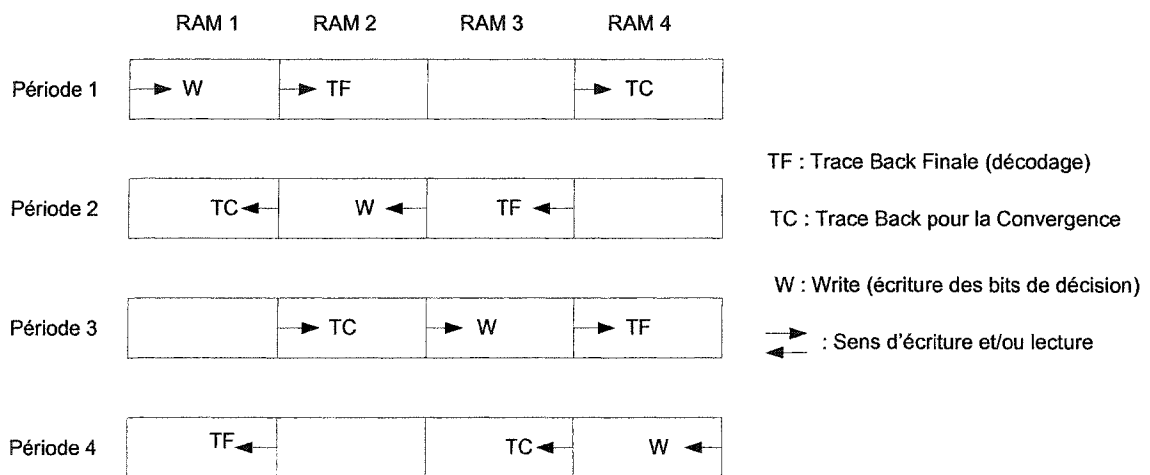
Figure 22 Flot de la mémoire du TB à quatre RAM
