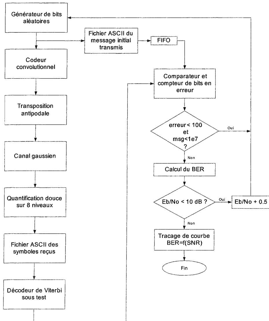
Figure 37 Illustration des procédures de test et prélèvement des résultats.
