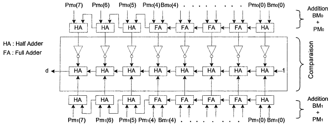
Figure 18 Diagramme bloc illustrant une paire d'addition-comparaison simultanées à 8-bits
