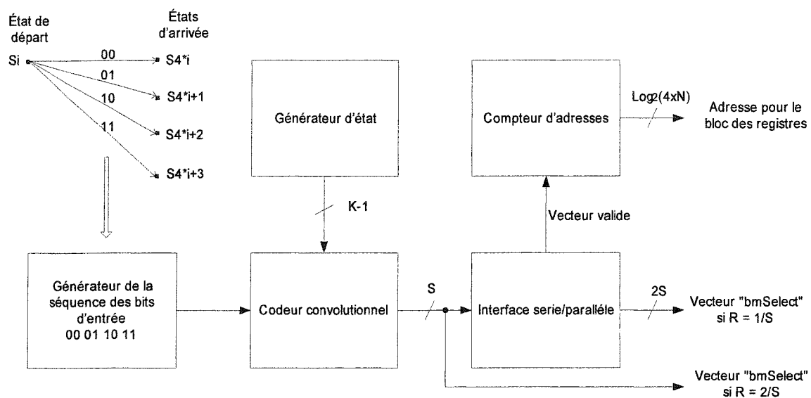
Figure A-2 Schéma fonctionnel pour la méthode de la génération des vecteurs "select"
