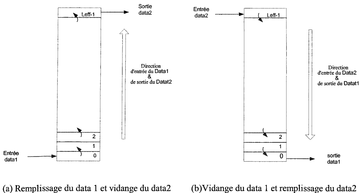
Figure 25 Schéma fonctionnel de la pile LIFO bidirectionnelle
