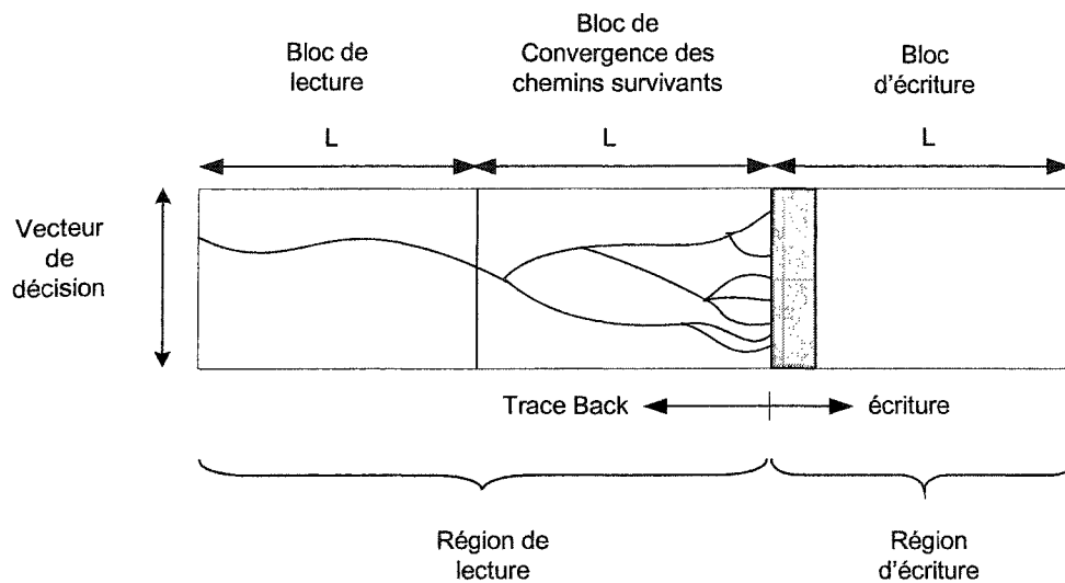
Figure 21 Organisation de la mémoire des décisions en tampon cyclique
