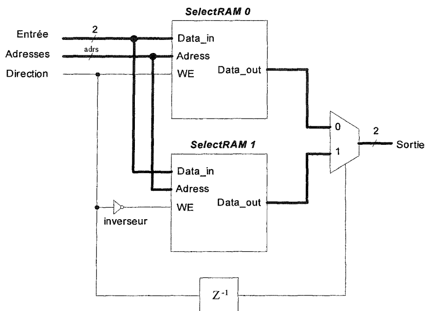
Figure 33 Diagramme bloc de l'unité LIFO utilisant des blocs RAM
