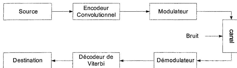
Figure 1 Système de communication utilisant un encodeur convolutionnel avec un décodeur de Viterbi pour la correction d'erreurs
