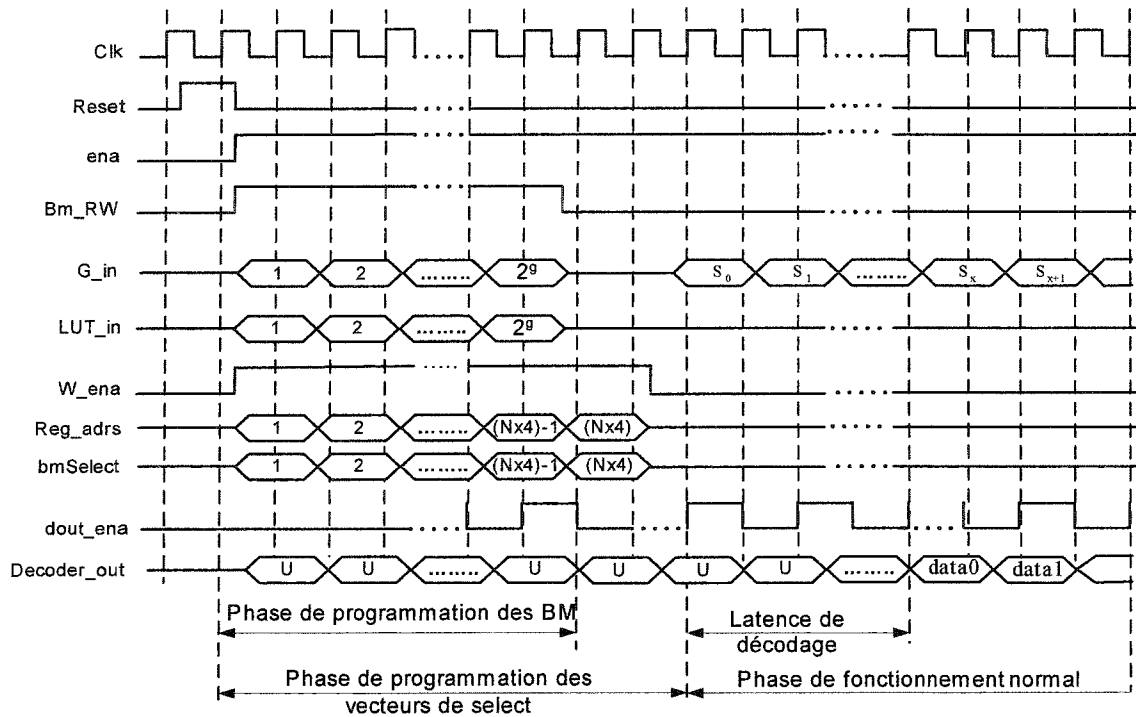
Figure 28 Chronogramme des phases de fonctionnement du décodeur, R = 1/S
