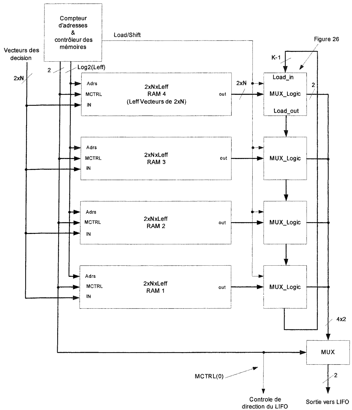
Figure 23 Diagramme bloc du Trace Back
