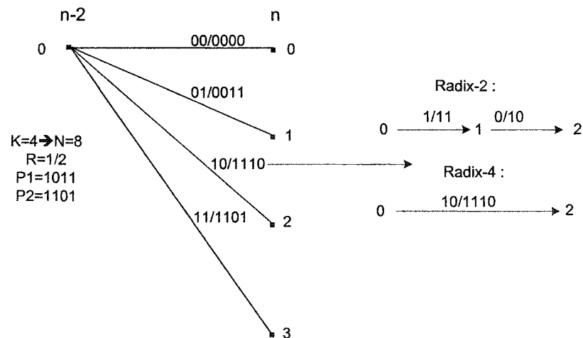
Figure A-1 Passage d'un état aux quatre autres, N = 8 , P1 = 1011 , P2 = 1101 et R = 1/2
