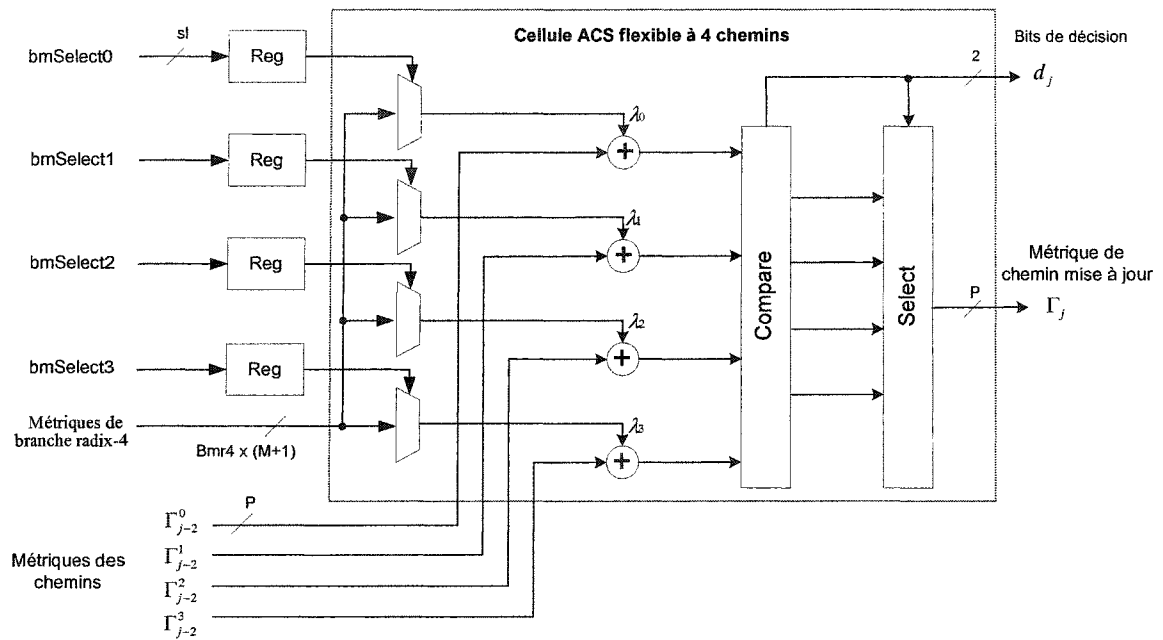
Figure 20 Cellule ACS à 4-chemins, R = W/S où W = 1,2 et S = 1,2,3,\dots bmr4 = 2^{2S} (ou 2^S ) et sl = 2S (ou S ) si R = 1/S (ou 2/S )
