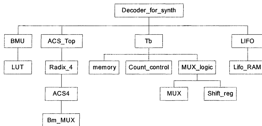
Figure 32 Hiérarchie du design
