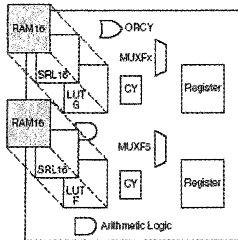
Figure 30 Configuration d'une tranche d'un circuit FPGA Virtex-II [28]
