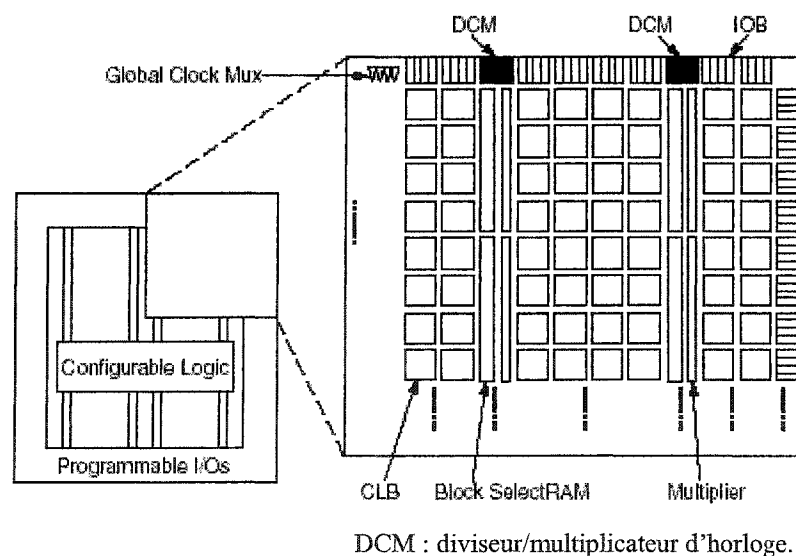
Figure 29 Vue générale de l'architecture d'un circuit FPGA Virtex-II [28]
