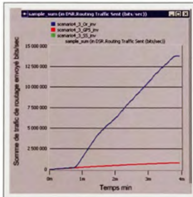
Figure 5.23 Somme du trafic de routage envoyé.
