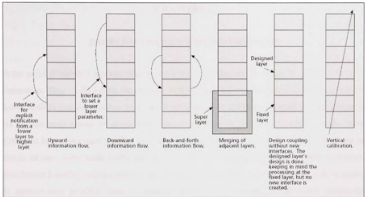
Figure 1.22 Différentes architectures cross-layer. Tiré de Srivastava et al.(2005)
