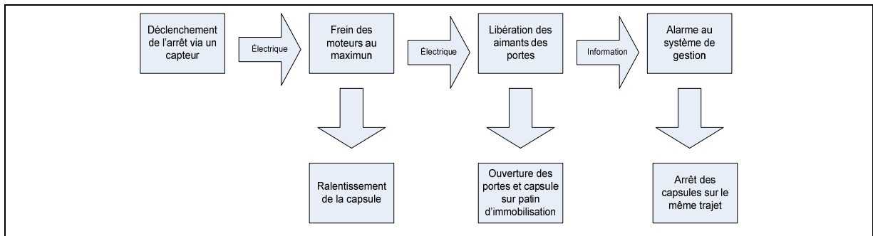
Figure-A I-9 Séquence d'arrêt d'urgence.
