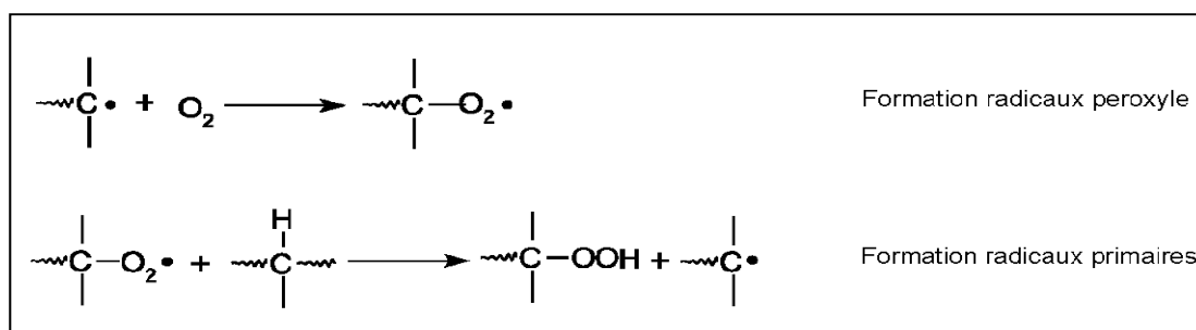
Figure 2.6 Formation de radicaux peroxy et radicaux primaires pendant l'oxydation. Tirée de Carlsson et Wiles (1985, p. 638)
