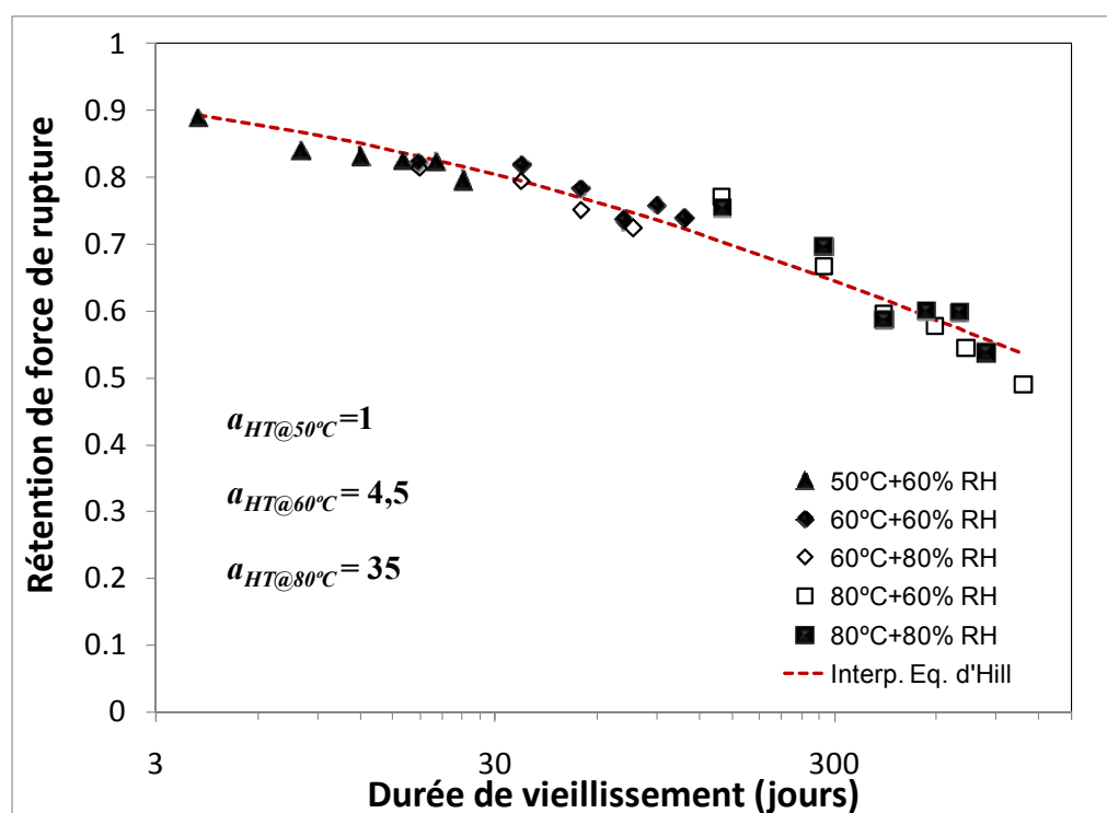
Figure 7.2 Courbe maitresse de rétention de force de rupture en fonction de la durée de vieillissement et son interpolation par l'équation d'Hill pour l'hydrolyse du Kevlar®. Les facteurs de glissement ( a_{HT} ) utilisés sont également inclus.
