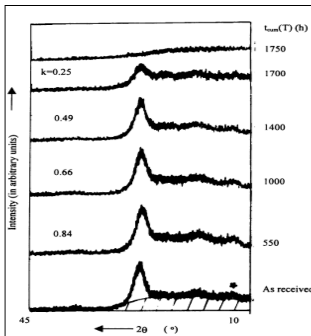
Figure 2.12 Comparaison des profils de diffraction pour le Nomex avant et après exposition à une température de 200 °C pour plusieurs durées. La valeur k représente le degré de cristallinité résiduelle. Tirée de Jain et al. (2002, p. 342)
