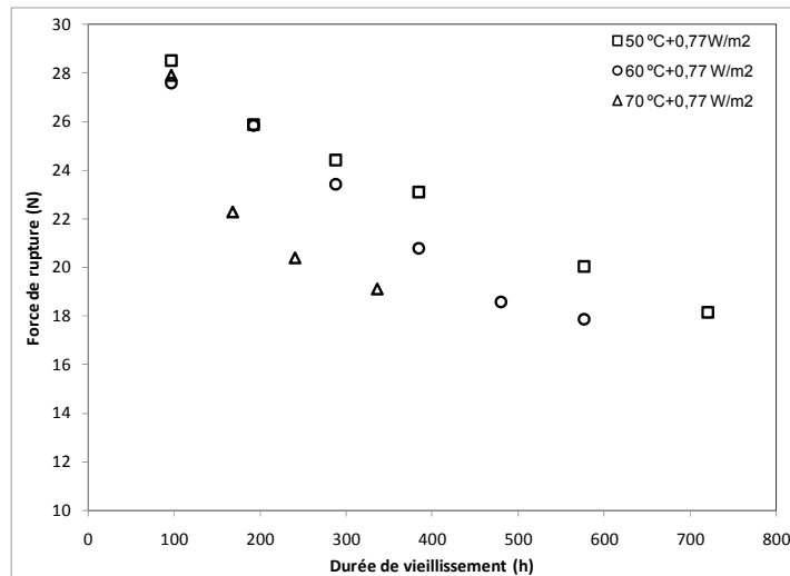
Figure 7.6 Force de rupture en fonction de la durée d'exposition pour différentes conditions de vieillissement photochimique mené à 0,77 \text{ W}\cdot\text{m}^{-2} .
