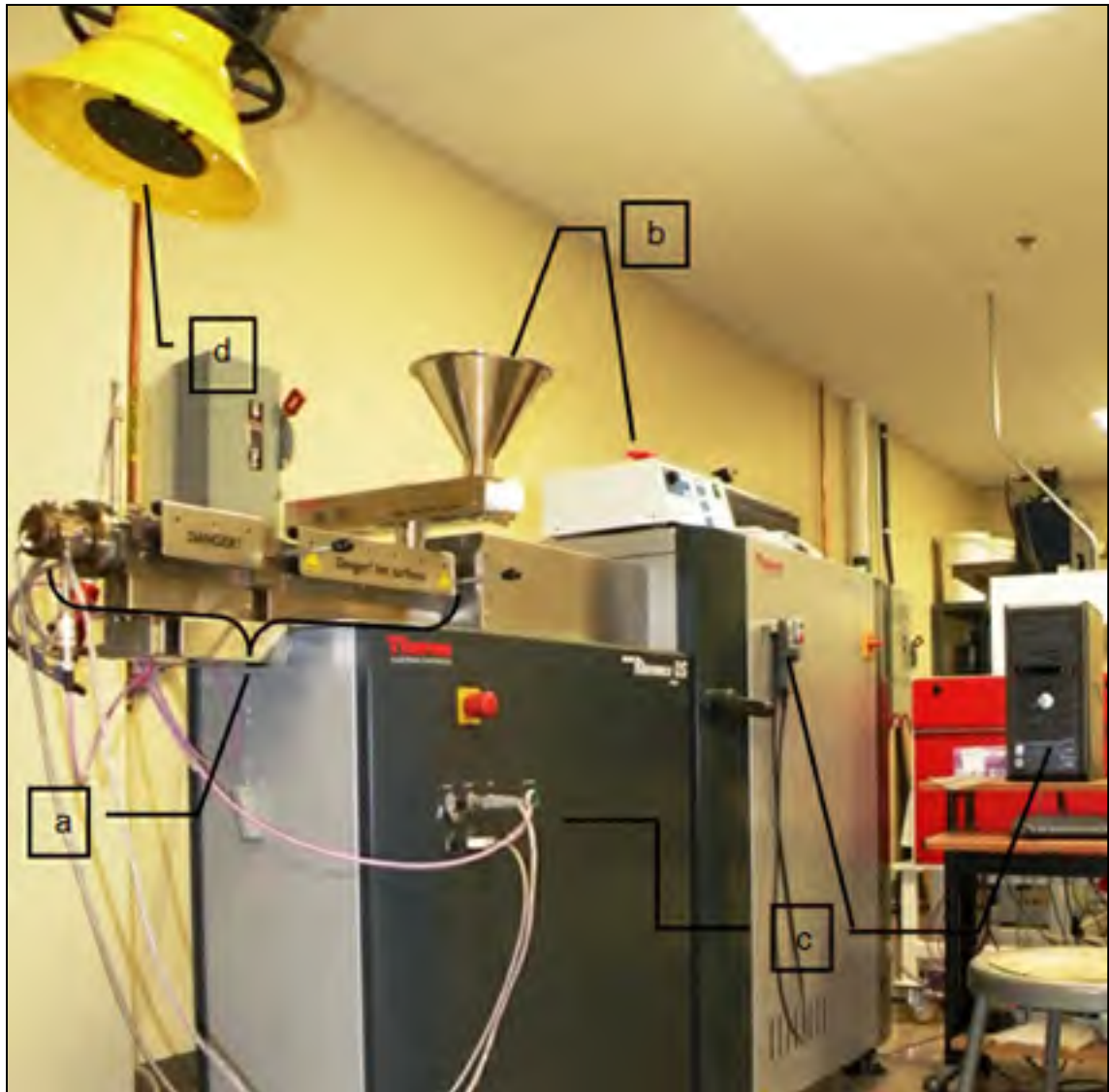
Figure 2.4 Photo représentant les installations de production a) extrudeur à double vis co-rotatives, b) dévidoir externe à contrôle variable, c) Système de contrôle
