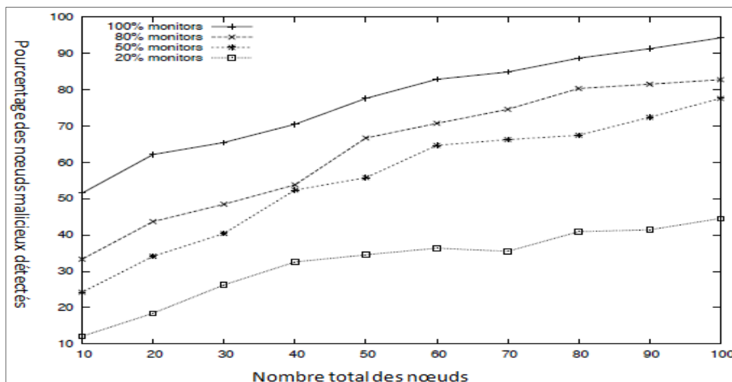
Figure 4.5: Pourcentage des nœuds malicieux détectés pour l'attaque suppression d'un voisin dans le message HELLO
