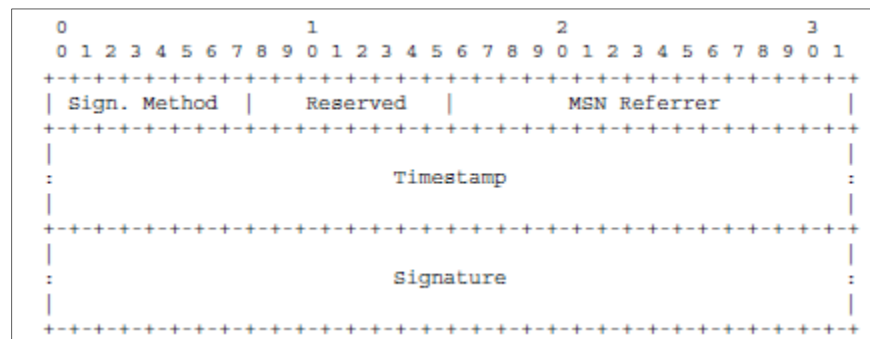
Figure 2.3: Format du message de signature généré Tirée de Adjih et al (2003)
