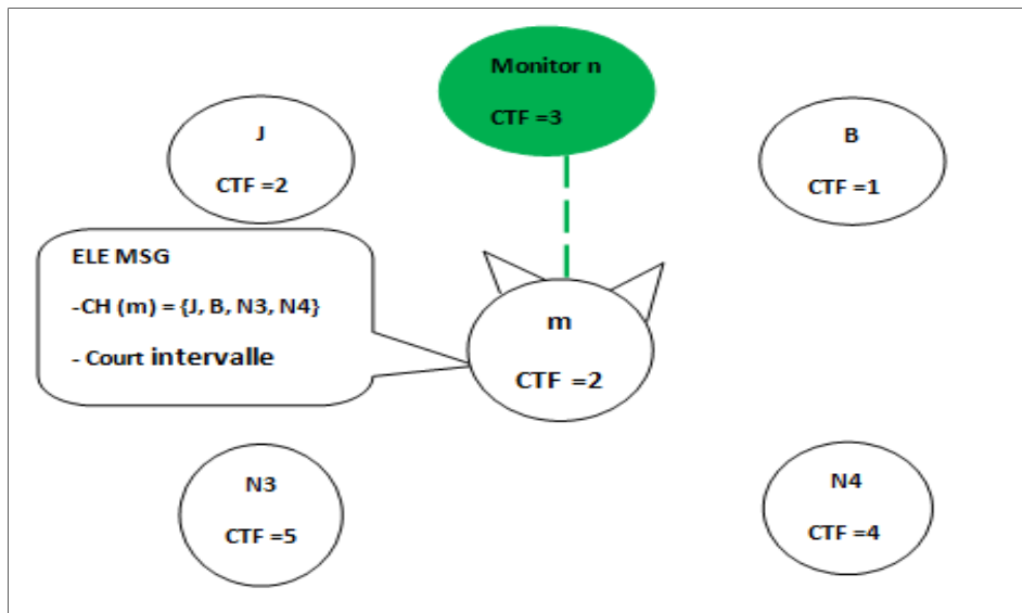
Figure 3.9 : Détection de l'attaque de vote pour plusieurs CH
