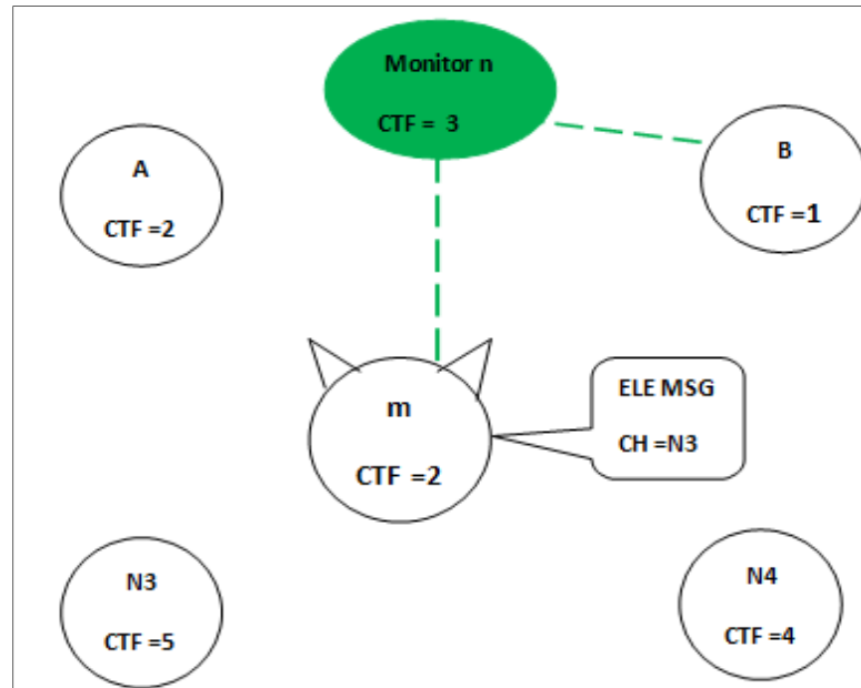
Figure 3.8 : Détection de l'attaque vote pour le nœud faible
