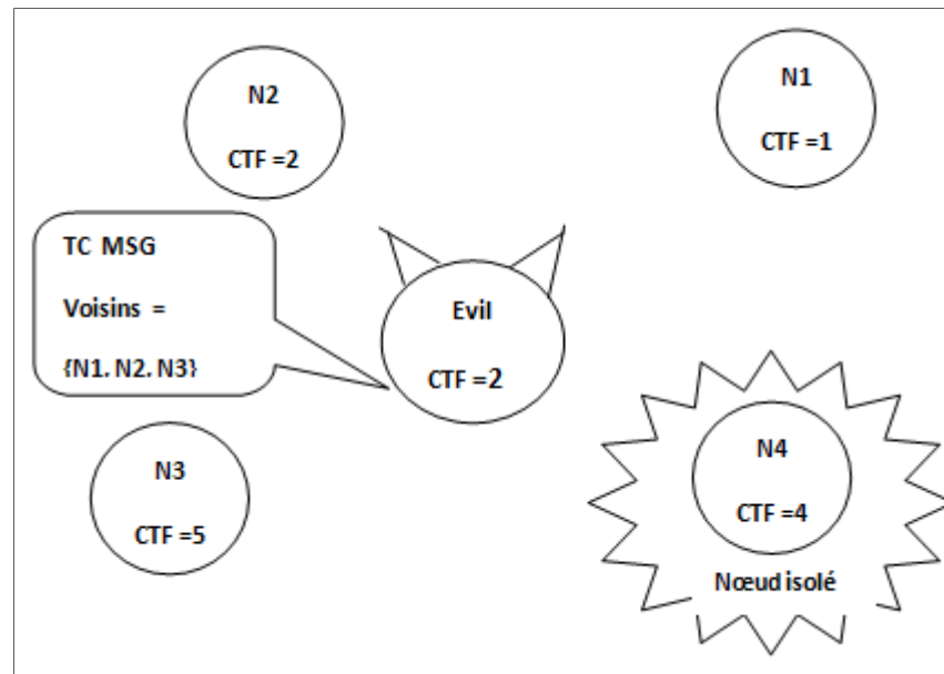
Figure 3.7 : Suppression d'un nœud sélectionneur légitime
