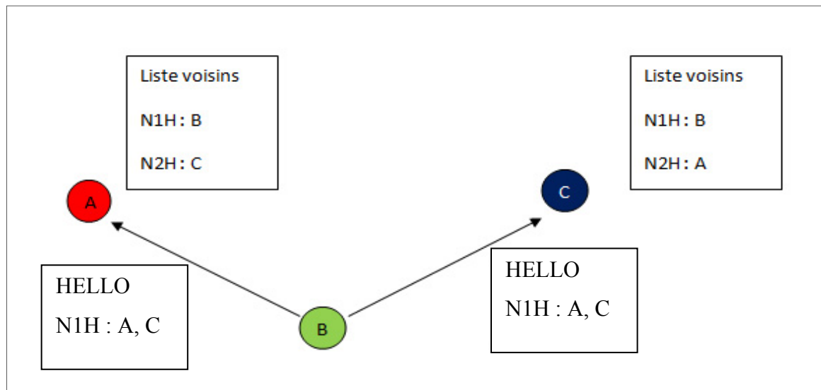
Figure 1.6 : Découverte de voisins N1H et N2H avec le message HELLO
