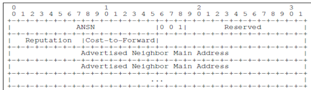
Figure 1.12 Message TC modifié Tirée de Chriqi et al. (2009)
