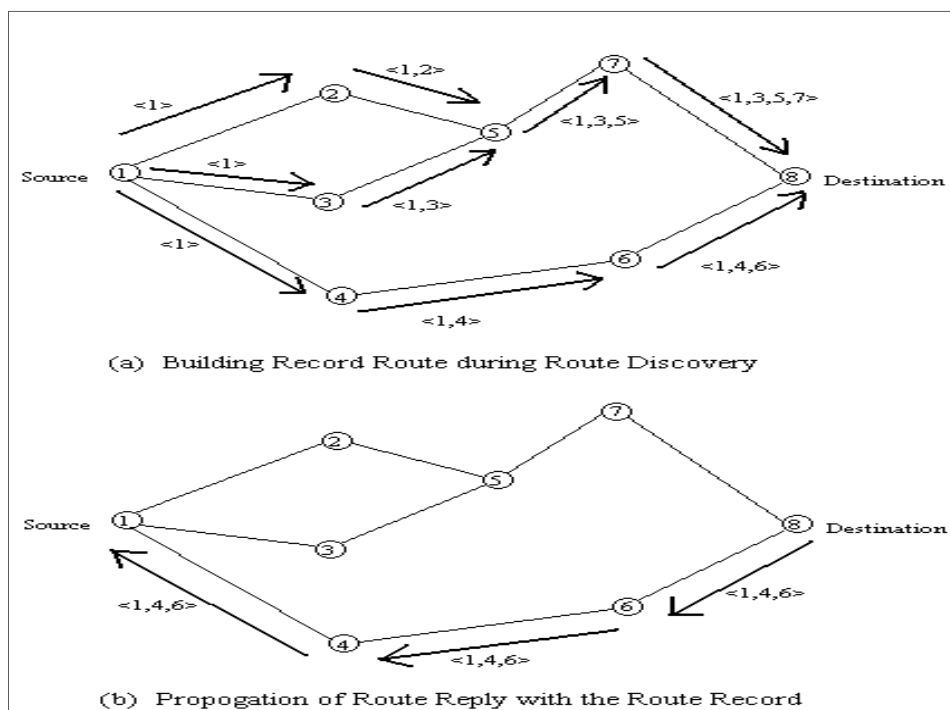
Figure 1.3: Phase de découverte de routes dans le protocole DSR Tirée de Johnson et al. (2001)
