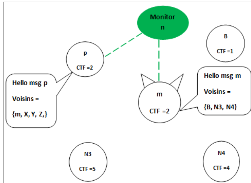
Figure 3.10: Détection de l'attaque suppression d'un voisin dans le message HELLO
