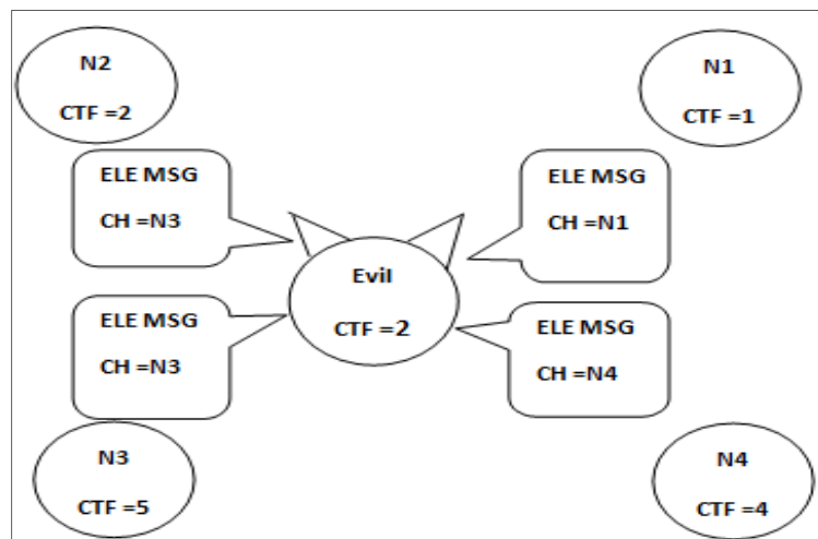
Figure 3.4: Attaque de vote pour plusieurs CH
