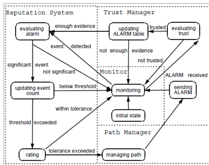
Figure 3.2: Mécanisme de détection CONFIDANT Tirée de Buchegger et Le Boudec (2002)
