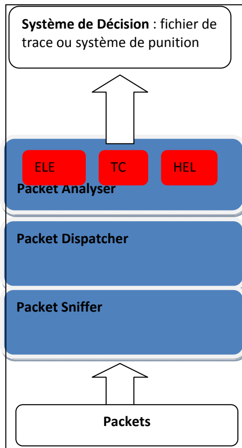
Figure 3.13 : Architecture du système de détection d'intrusion proposée
