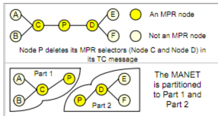
Figure 2.2 Usurpation de lien avec les messages TC Tirée de Wang et al. (2005)
