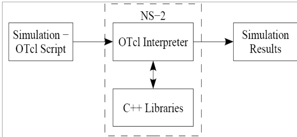
Figure 4.1: Flot de simulation de scénarios sous NS2
