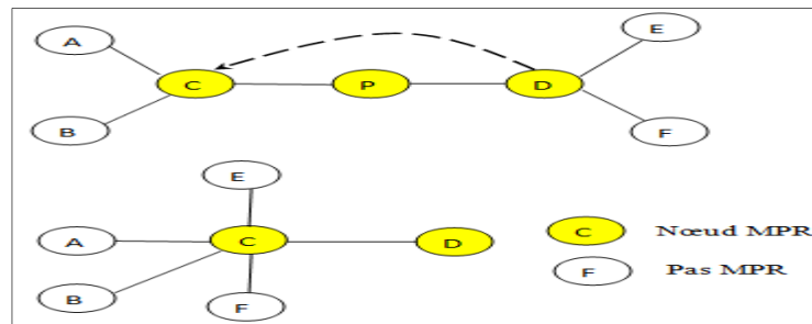
Figure 2.1 Usurpation d'identité avec le message HELLO
