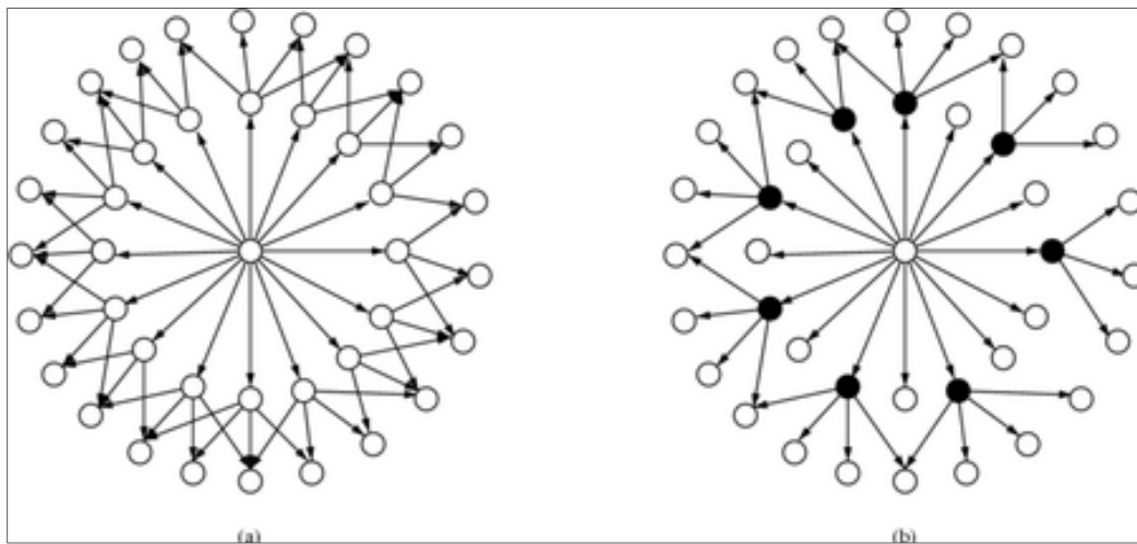
Figure 1.7 (a) Processus d'inondation classique, (b) Processus d'inondation MPR Tirée de Clausen et al. (2003)
