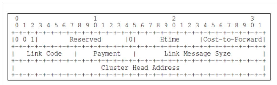
Figure 1.13 Le nouveau message ELECTION Tirée de Chriqi et al. (2009)
