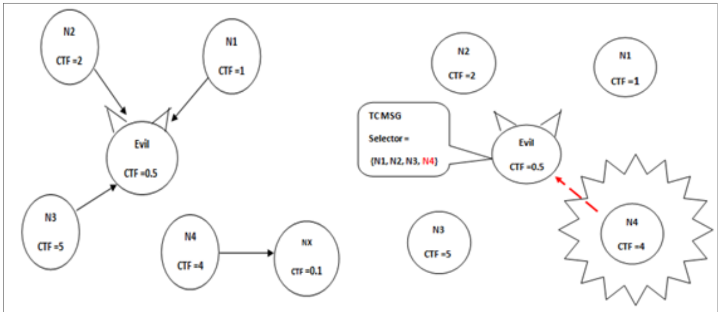
Figure 3.6: Attaque d'ajout de sélectionneur illégitime
