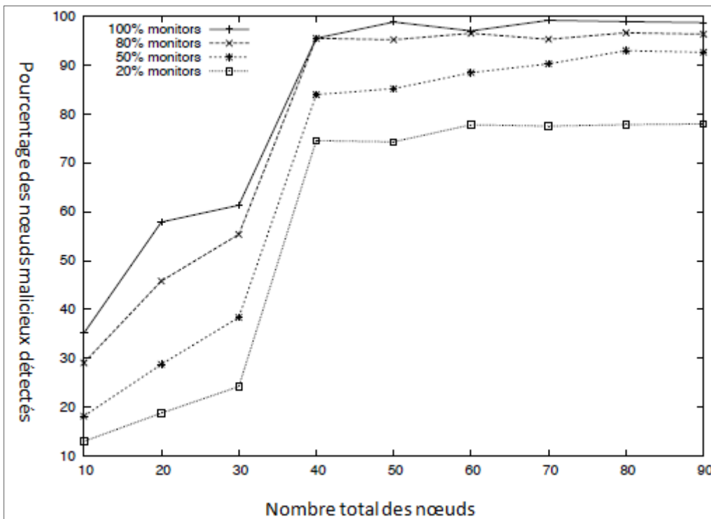
Figure 4.6 : Pourcentage des nœuds détectés pour l'attaque suppression d'un sélectionneur légitime
