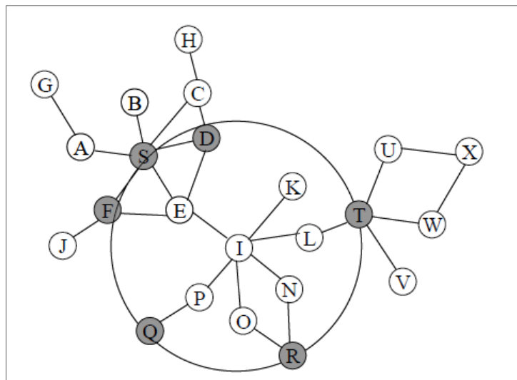
Figure 1.4 Fonctionnement du protocole ZRP Tirée de Beijar (2002)
