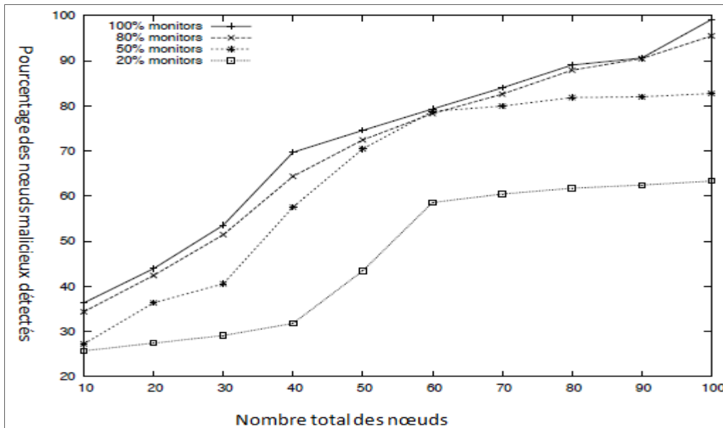
Figure 4.3: Pourcentage de détection des nœuds malicieux pour l'attaque vote pour le noeud faible comme CH
