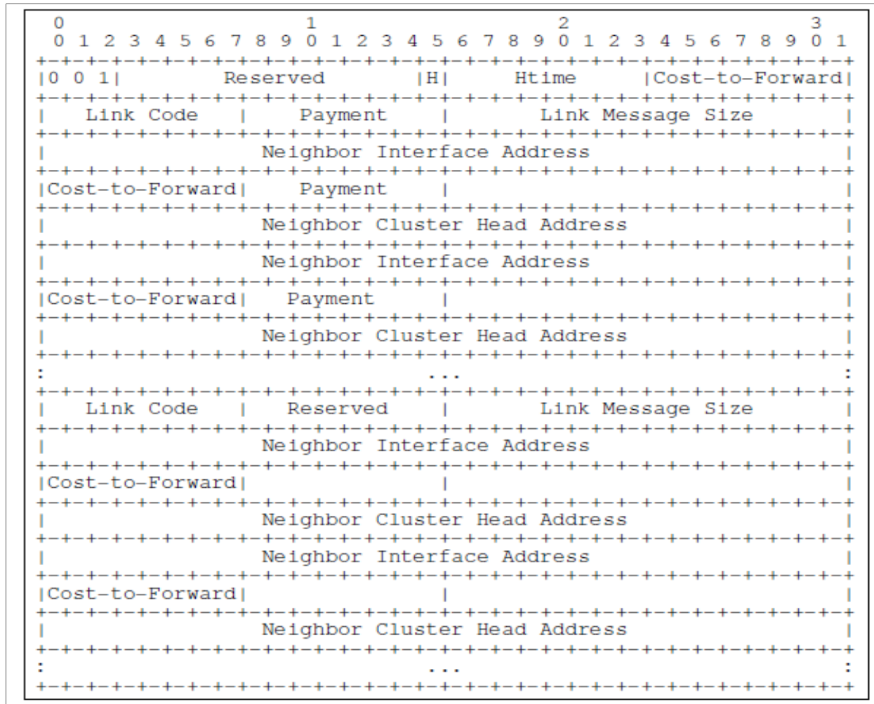
Figure 1.11 Message HELLO modifié Tirée de Chriqi et al. (2009)
