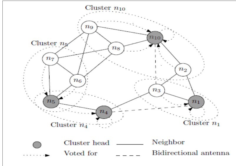
Figure 1.9 Principe de vote pour un CH dans SC-OLSR Tirée de Chriqi et al. (2009)
