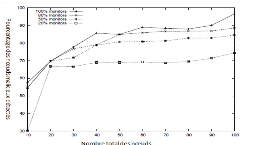
Figure 4.4: Pourcentage de détection des nœuds malicieux contre l'attaque vote pour des CH multiples
