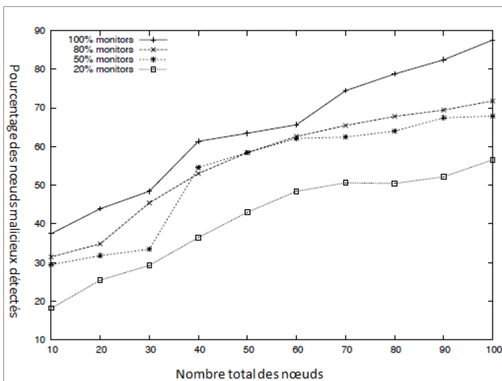
Figure 4.7 : Pourcentage des nœuds détectés pour l'attaque ajout d'un sélectionneur illégitime
