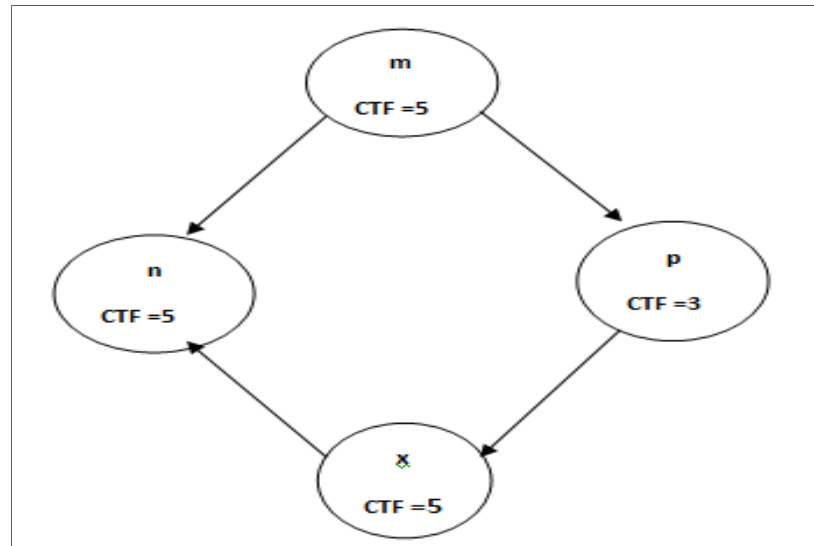
Figure 3.11: Détection à distance avec l'algorithme 4
