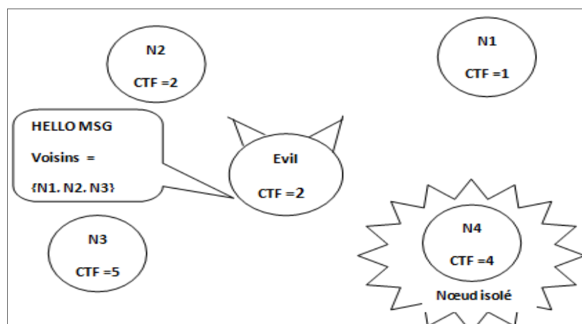
Figure 3.5: Attaque de suppression de voisins dans message HELLO
