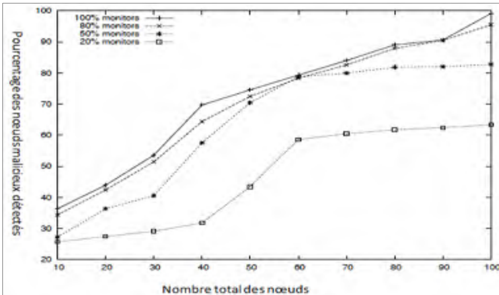
Figure 4.3: Pourcentage de détection des nœuds malicieux pour l'attaque vote pour le nœud faible comme CH
