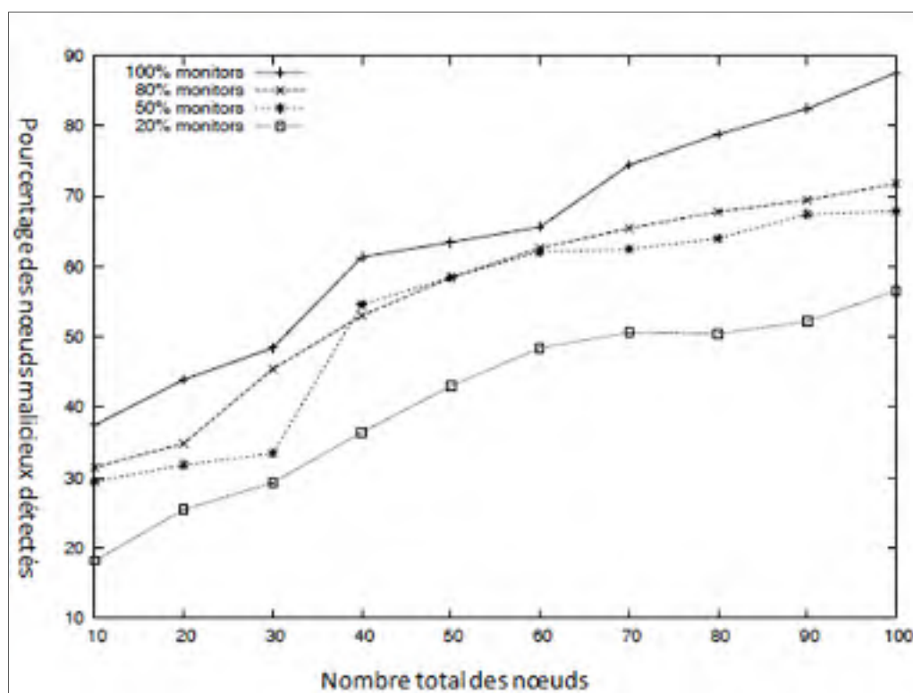
Figure 4.7 : Pourcentage des nœuds détectés pour l'attaque ajout d'un sélectionneur illégitime
