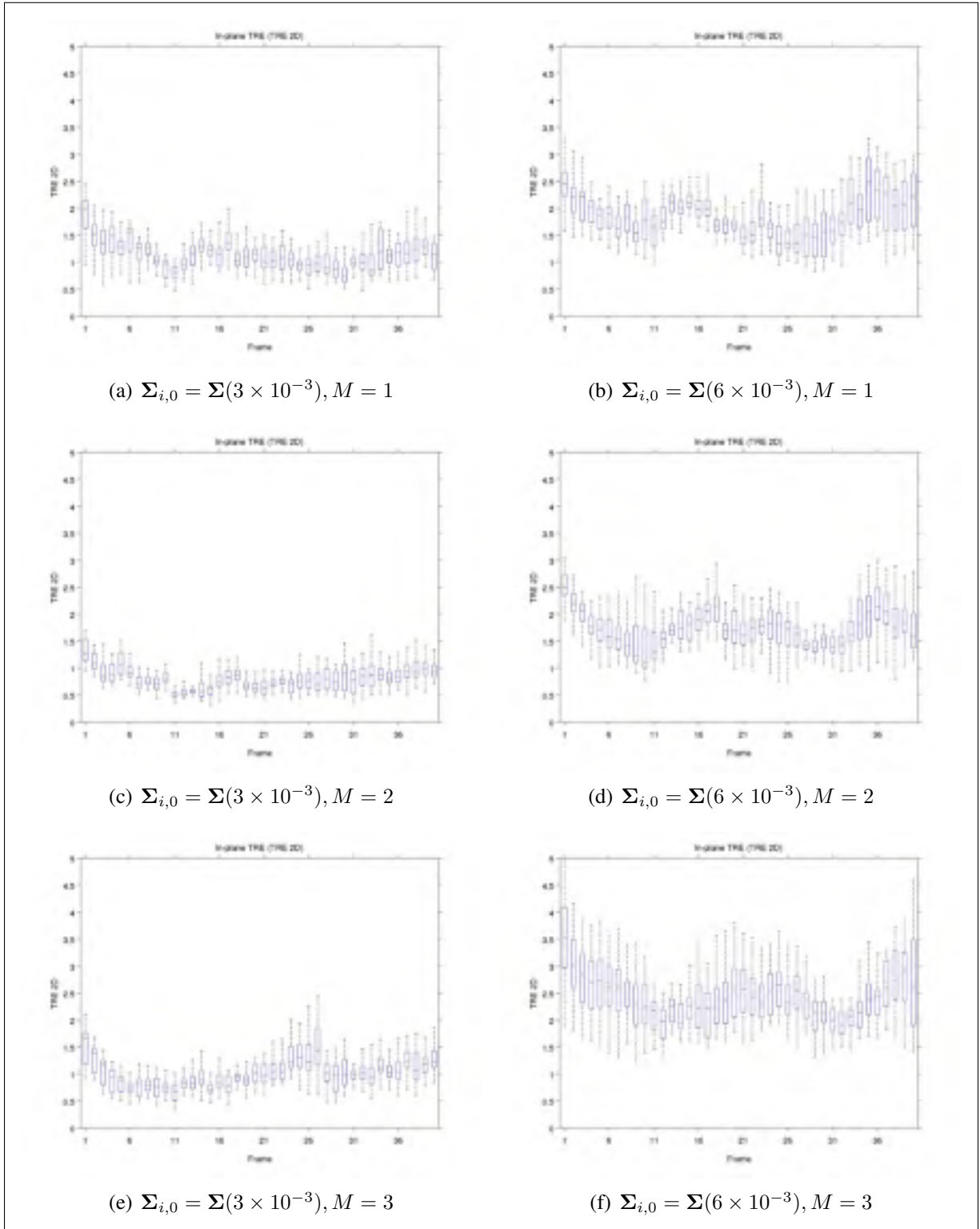
Figure-A II.3 - Évolution de l'erreur TRE 2D au cours des séquences de mouvement pour \Sigma_{i,0} \in \{\Sigma(3 \times 10^{-3}), \Sigma(6 \times 10^{-3})\} .
