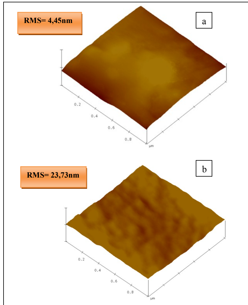
Figure 4.18 Image par AFM de la surface d'une fibre de Nomex® non- vieillie (a) et vieillie à 0,68 W/m 2 à 80°C pendant 168 heures (b)
