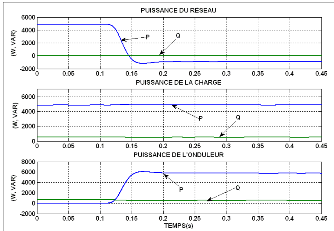
Figure 4.22 Écoulement de puissance avec ensoleillement G=800\text{W/m}^2
