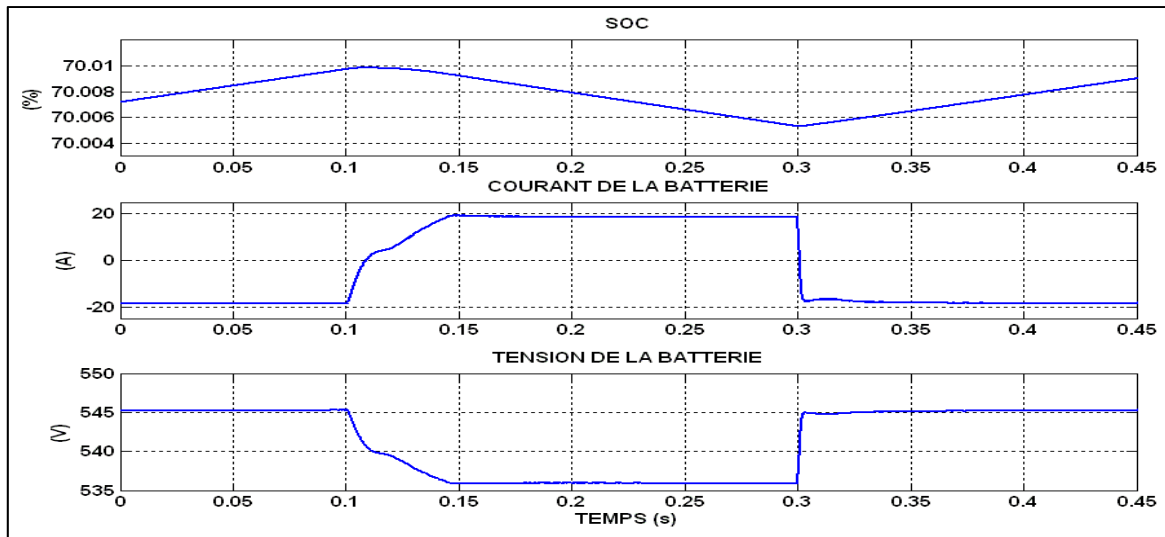
Figure 4.26 État de charge de la batterie
