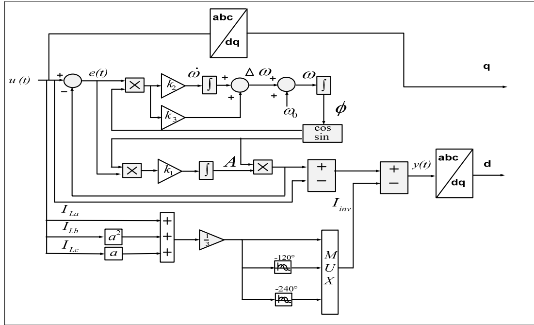
Figure 4.13 Schéma final de l'ANF modifié
