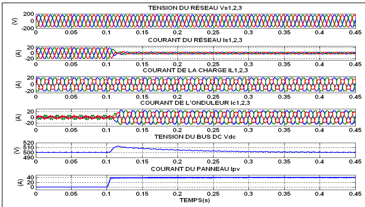
Figure 4.31 Réponse en régime dynamique avec ensoleillement G=800\text{W/m}^2
