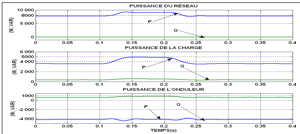
Figure 4.59 Écoulement de puissance avec variation de la charge
