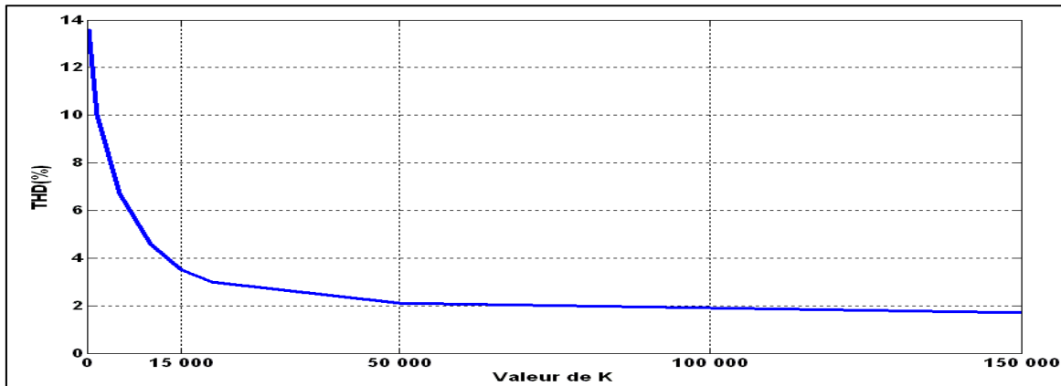
Figure 4.16 THDi en fonction de la valeur de K
