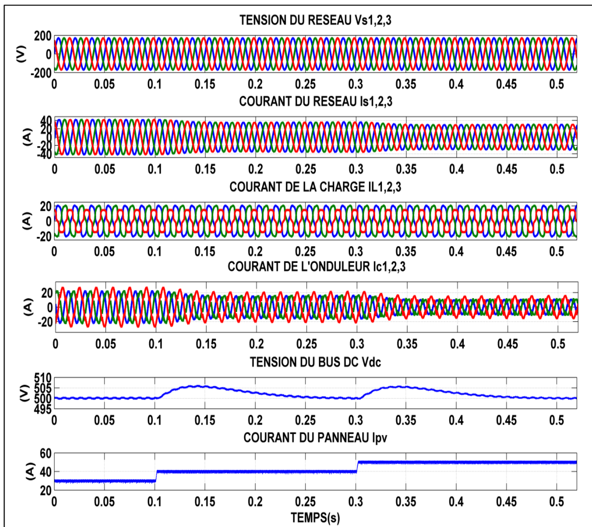
Figure 4.50 Réponse en régime dynamique avec variation de l'ensoleillement
