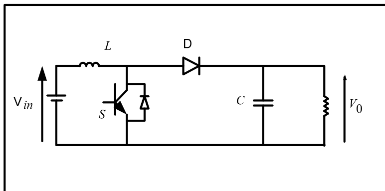
Figure 4.2 Schéma du convertisseur Boost
