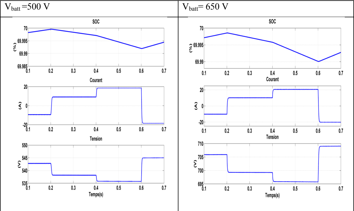
Figure 2.21 Résultat de simulation avec Boost-Buck pour V_{\text{batt}} = 500 et 650 \text{ V}
