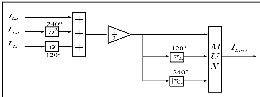
Figure 4.12 Schéma de l'extraction des courants inverse
