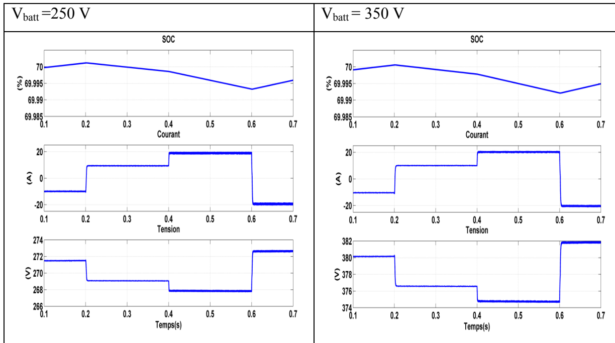
Figure 2.26 Résultat de simulation avec Buck-Boost modifié pour V_{\text{batt}} = 250 et 350 \text{ V}
