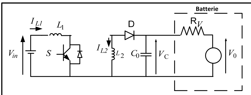
Figure 2.14 Schéma du montage du convertisseur Sepic lorsque l'interrupteur est passant
