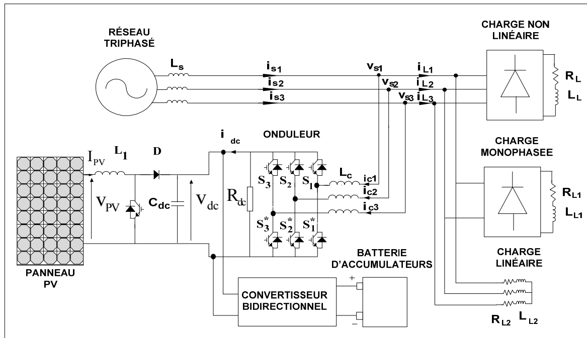
Figure 4.20 Schéma global du système PV raccordé au réseau
