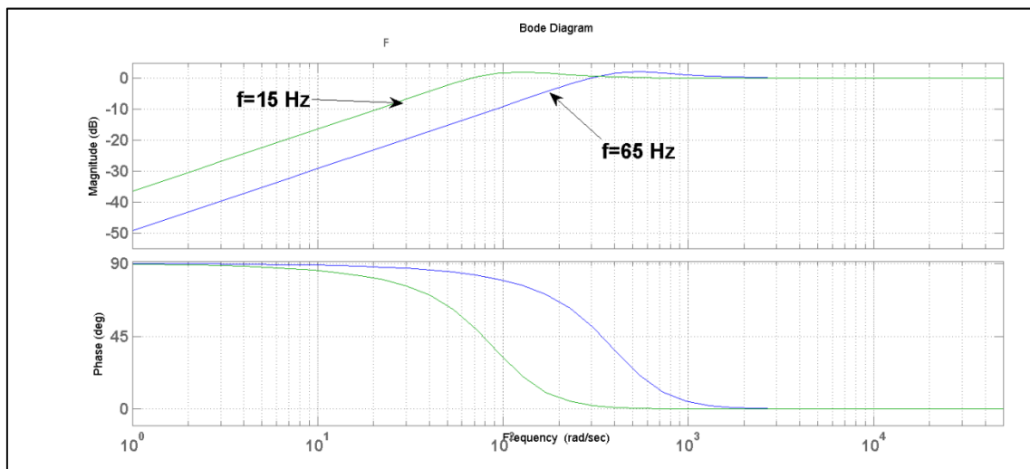
Figure 4.7 Diagramme de Bode du filtre pour différentes fréquences de coupures
