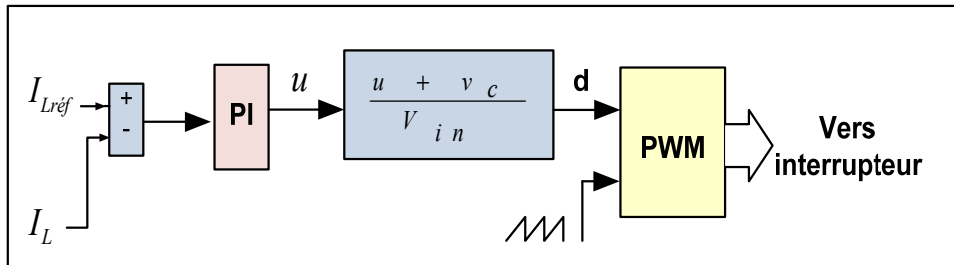
Figure 2.10 Schéma de la commande du convertisseur Buck
