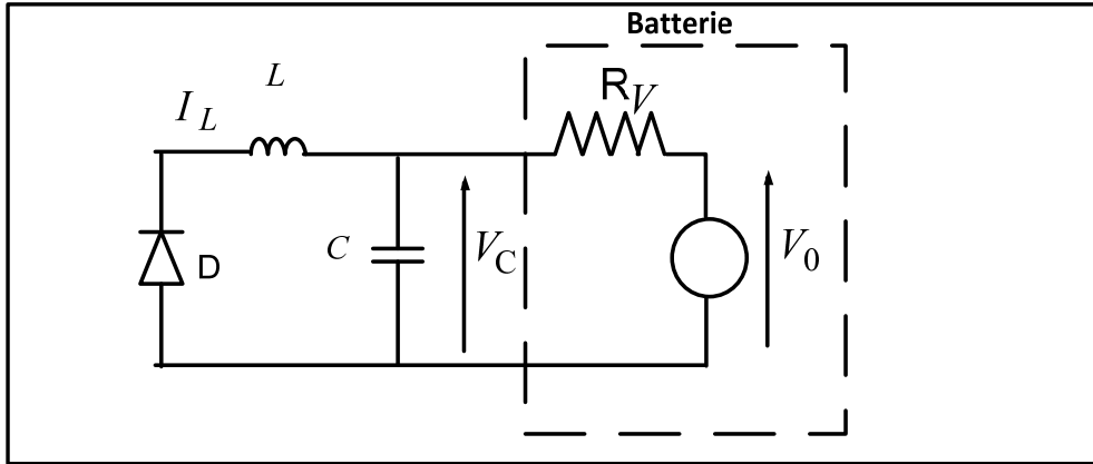
Figure 2.9 Schéma du montage du convertisseur quand l'interrupteur est bloqué
