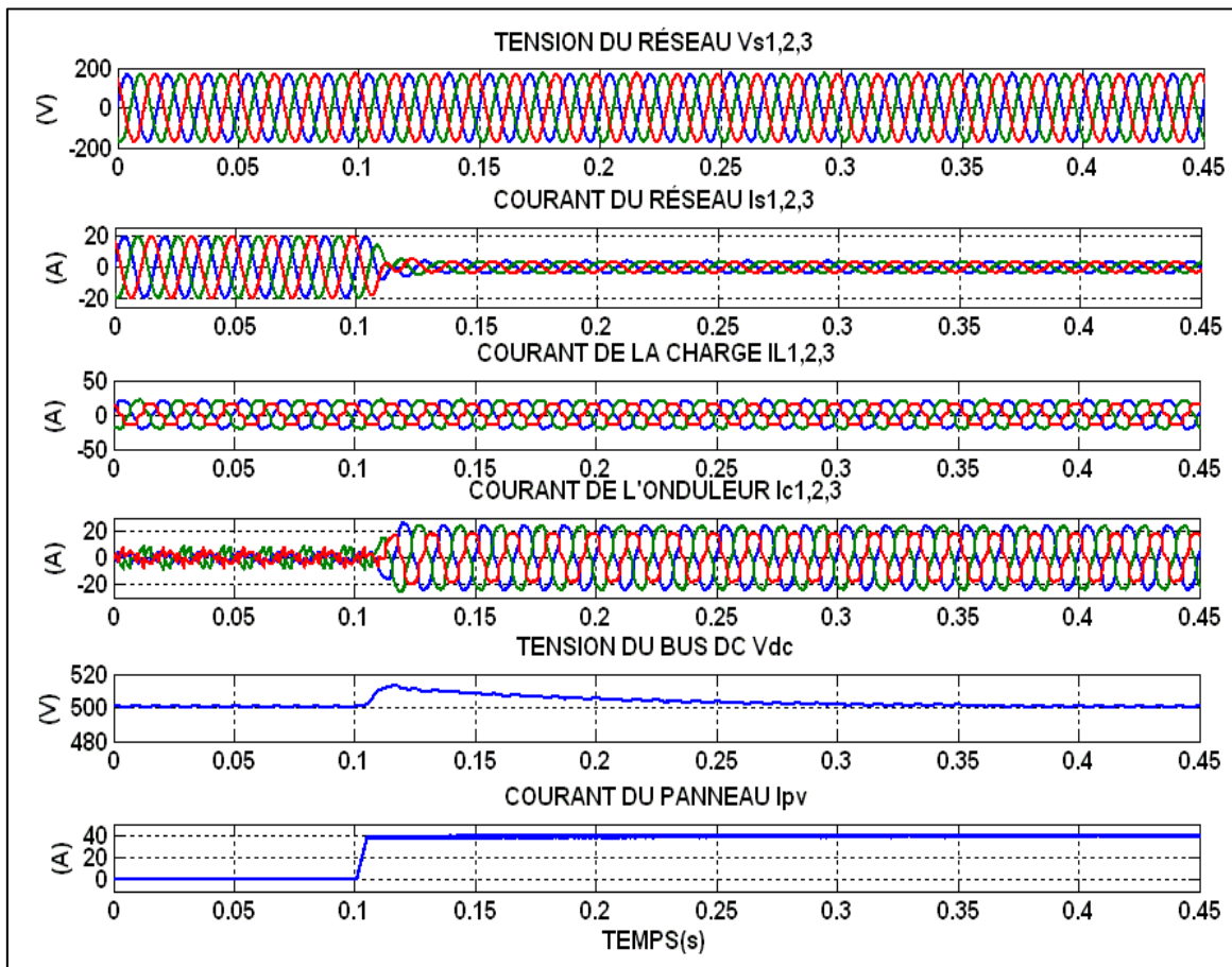
Figure 4.21 Réponse en régime dynamique avec ensoleillement G=800\text{W/m}^2
