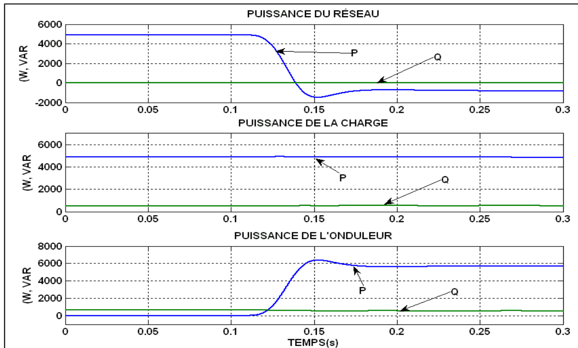
Figure 4.53 Écoulement de puissance avec ensoleillement G=800\text{W/m}^2
