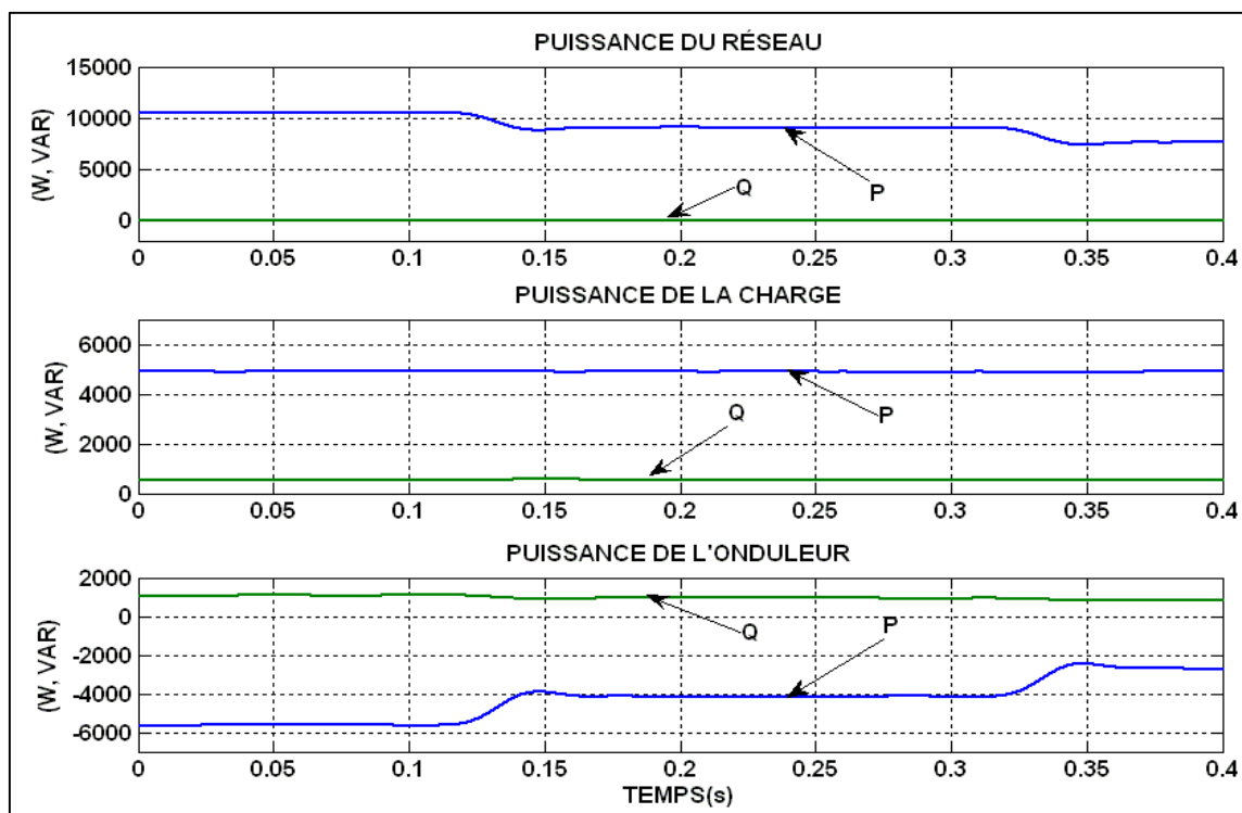
Figure 4.40 Écoulement de puissance avec variation de l'ensoleillement
