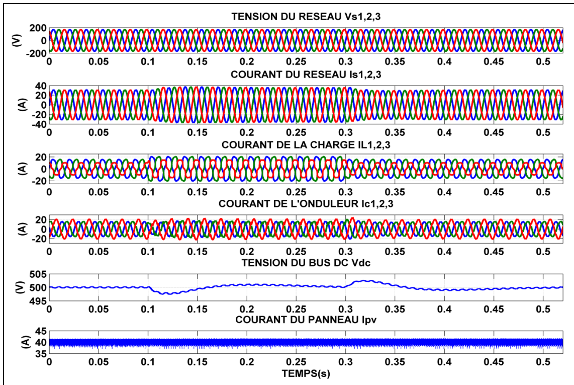
Figure 4.48 Réponse en régime dynamique avec variation de la charge
