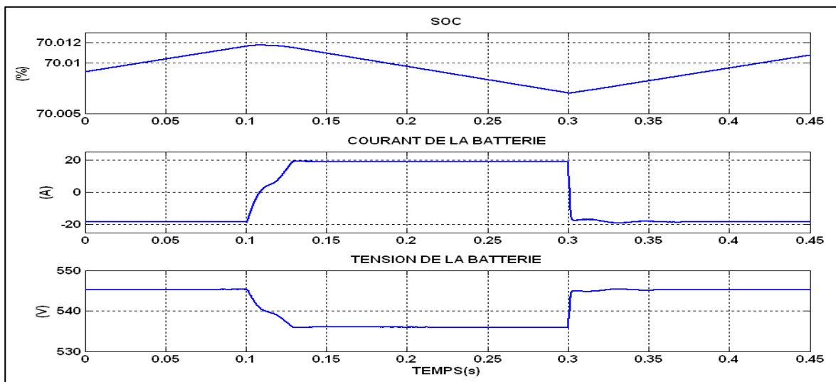
Figure 4.36 État de charge de la batterie
