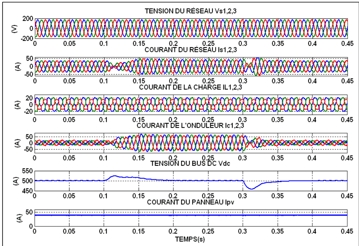
Figure 4.24 Réponse en régime dynamique avec variation de la charge de la batterie
