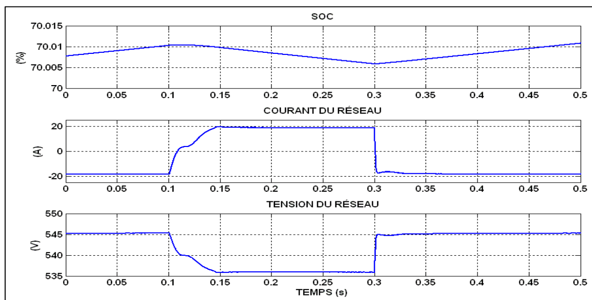
Figure 4.56 État de charge de la batterie
