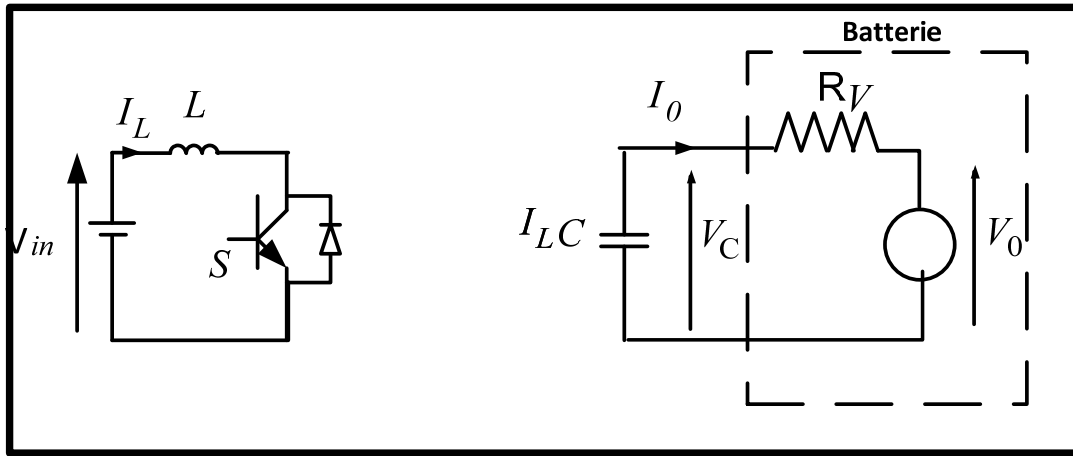
Figure 2.3 Schéma du convertisseur Boost quand l'interrupteur est passant
