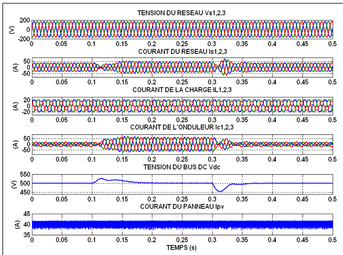
Figure 4.55 Réponse en régime dynamique avec variation de la charge de la batterie
