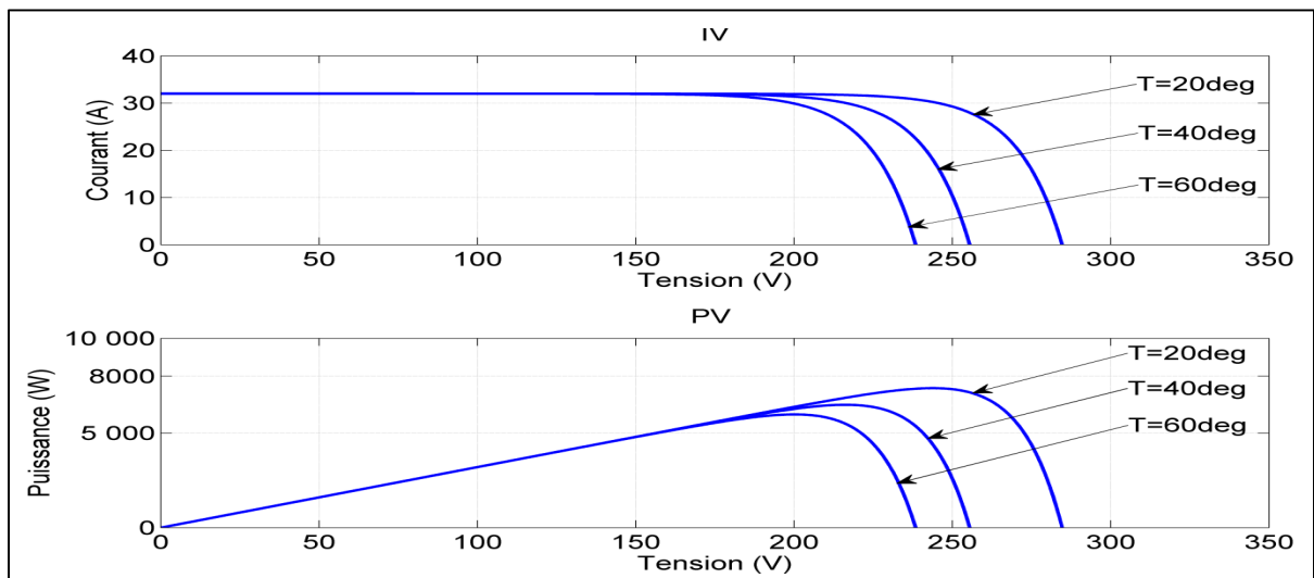
Figure 3.4 Courbe V-I et P-V des modules PV avec variation de la température
