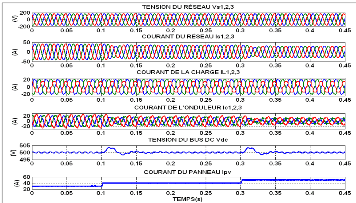
Figure 4.60 Réponse en régime dynamique avec variation de l'ensoleillement
