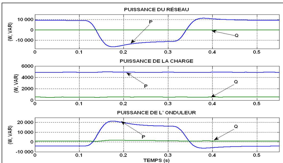
Figure 4.46 Écoulement de puissance avec variation de la charge de la batterie
