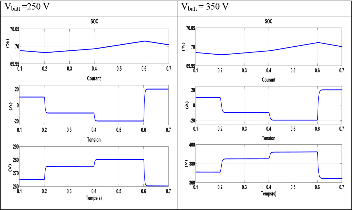
Figure 2.23 Résultat de simulation avec Buck-Boost pour V_{batt}=250 et 350V
