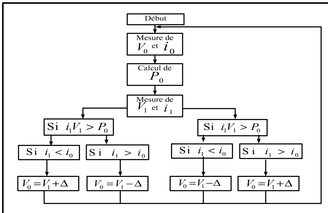
Figure 3.6 Algorithme du MPPT perturbation et observation
