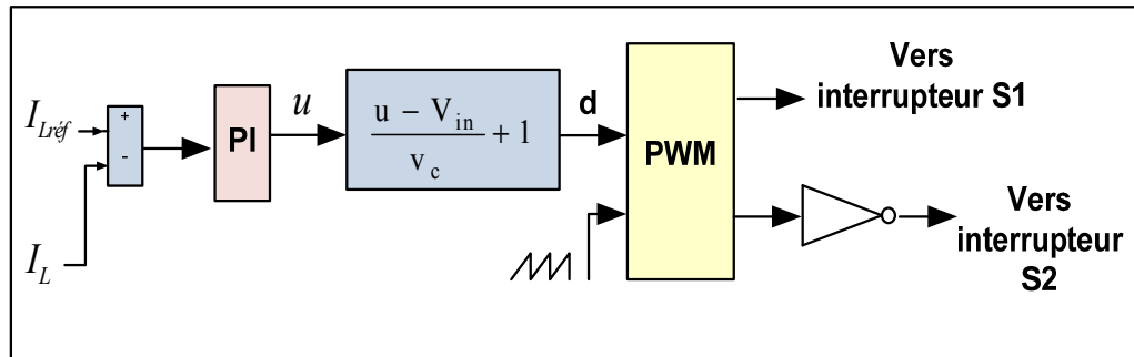
Figure 2.19 Schéma de la commande du convertisseur Boost-Buck
