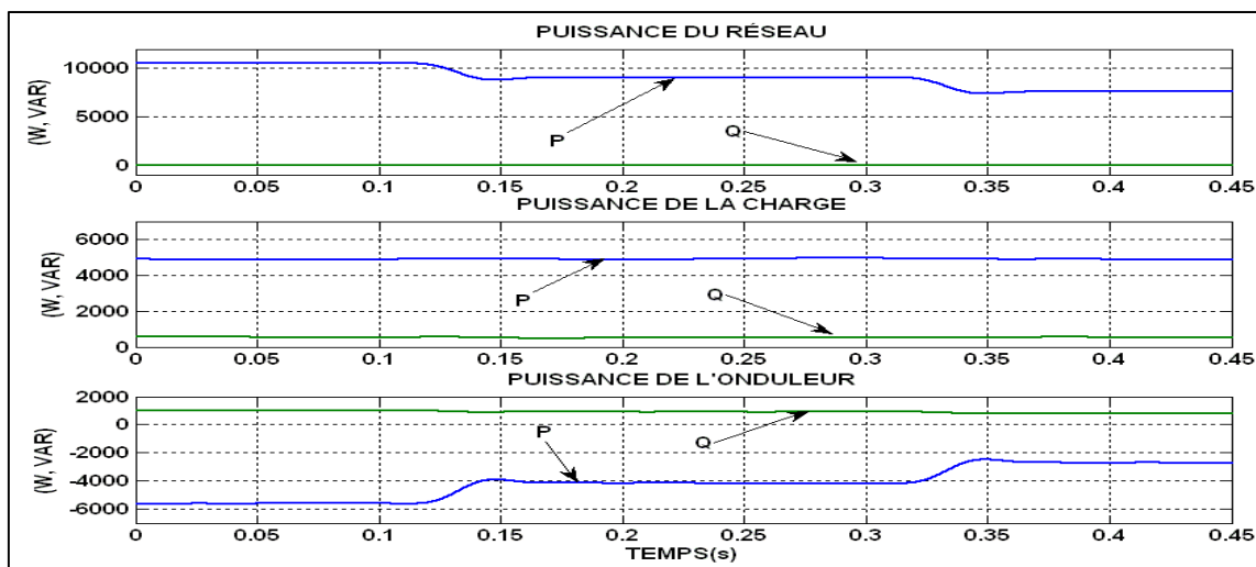
Figure 4.61 Écoulement de puissance avec variation de l'ensoleillement
