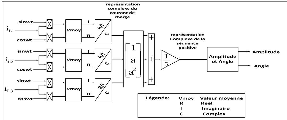
Figure 4.18 Extraction de la séquence positive du courant de charge
