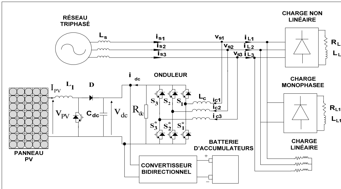
Figure 4.1 Schéma global du système PV raccordé au réseau
