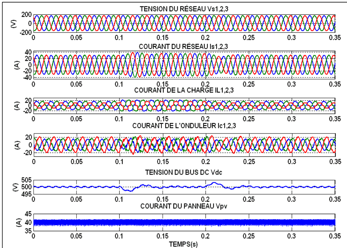
Figure 4.37 Réponse en régime dynamique avec variation de la charge
