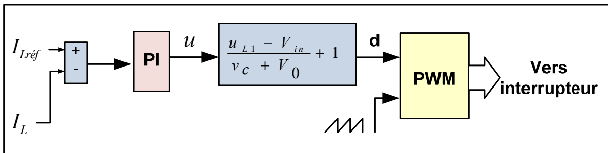
Figure 2.15 Schéma de la commande du convertisseur Sepic
