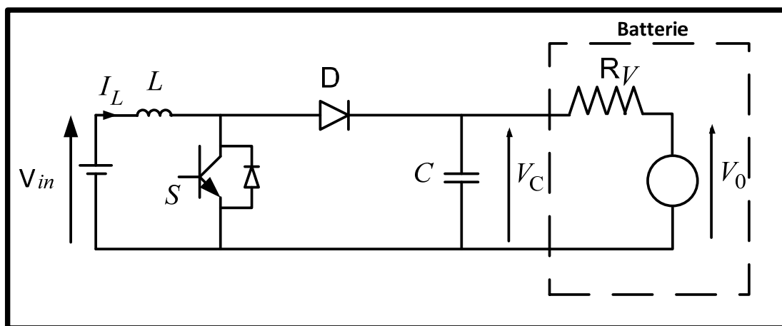
Figure 2.1 Schéma du convertisseur Boost alimentant une batterie
