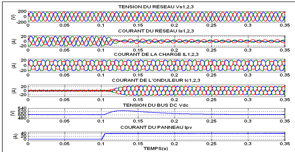
Figure 4.41 Réponse en régime dynamique avec ensoleillement G=800\text{W/m}^2
