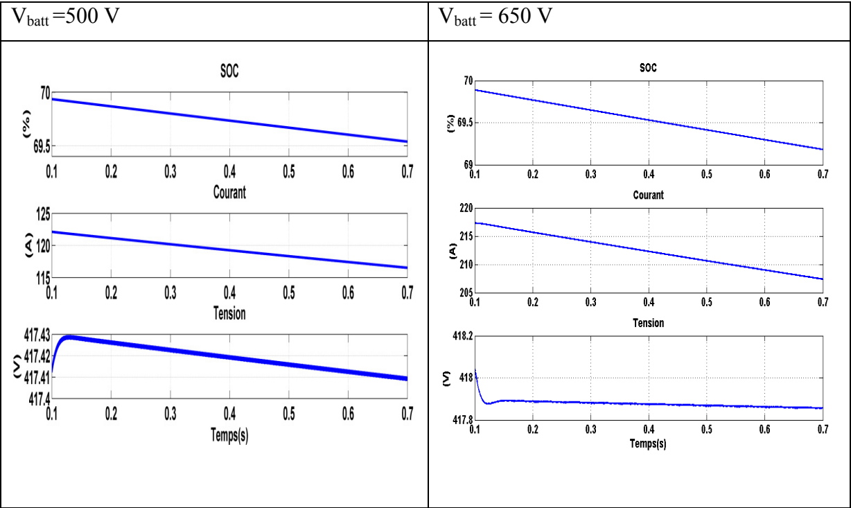
Figure 2.24 Résultat de simulation avec Buck-Boost pour V_{batt}=500 et 650V
