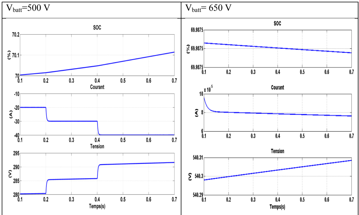
Figure 2.12 Résultat de simulation avec Buck pour V_{batt}=500 et 650V
