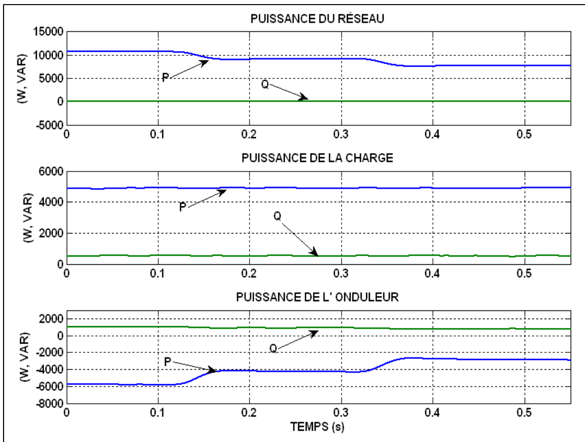
Figure 4.51 Écoulement de puissance avec variation de l'ensoleillement
