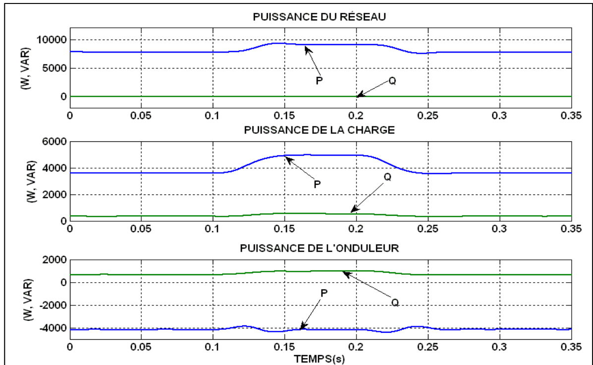
Figure 4.38 Écoulement de puissance avec variation de la charge
