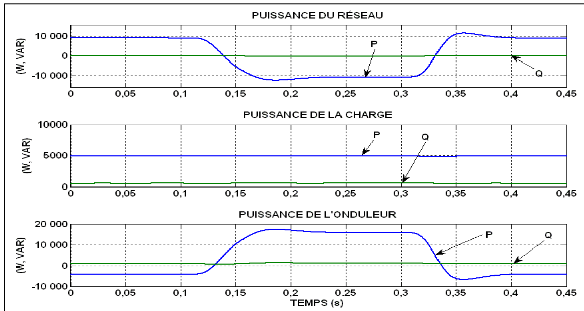
Figure 4.25 Écoulement de puissance avec variation de la charge de la batterie
