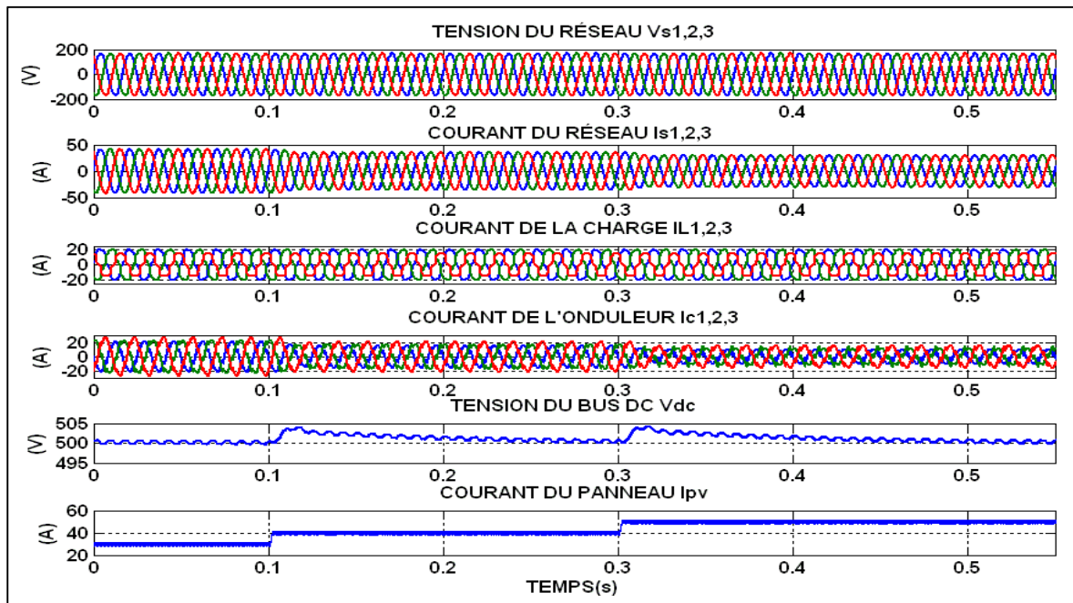
Figure 4.29 Réponse en régime dynamique avec variation de l'ensoleillement
