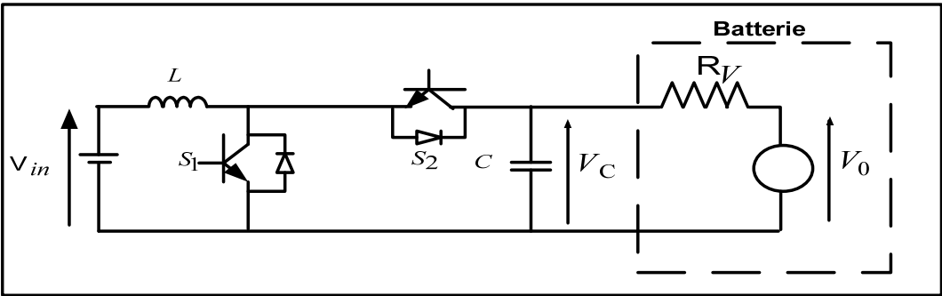
Figure 2.18 Schéma du montage du convertisseur Boost-Buck
