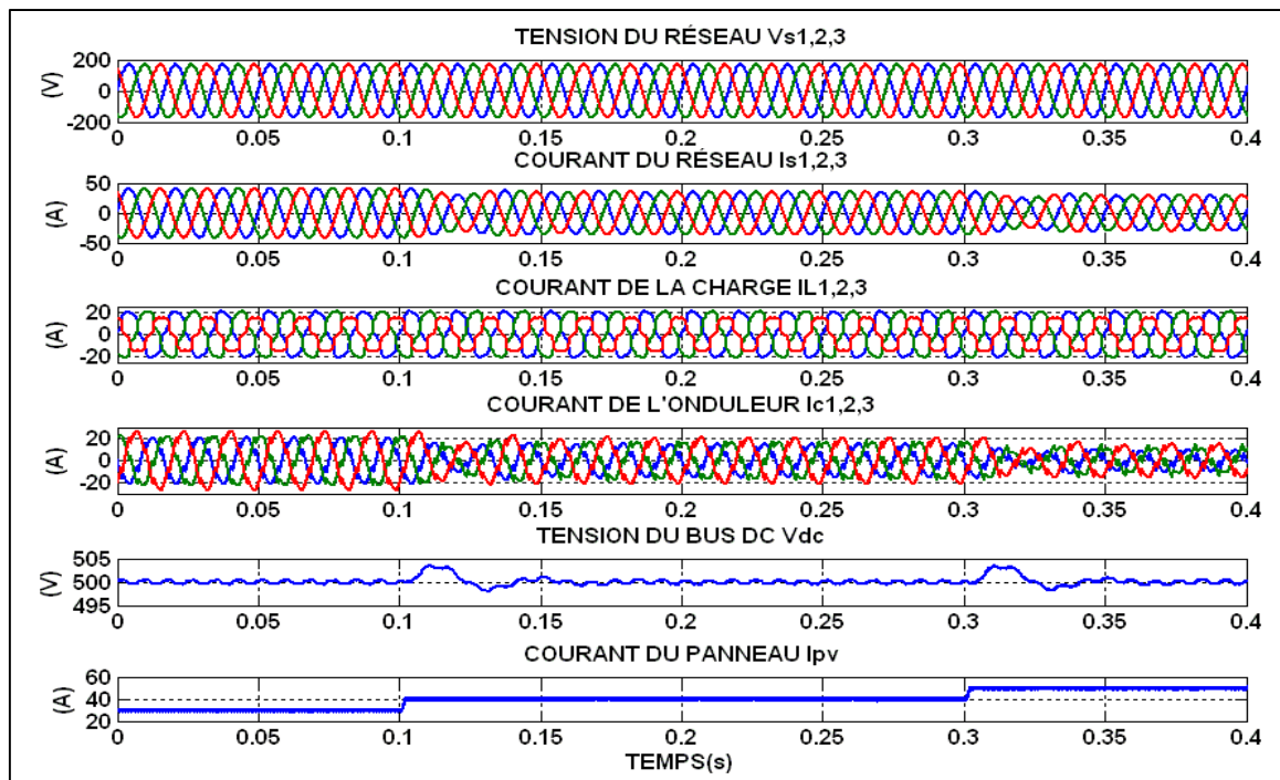
Figure 4.39 Réponse en régime dynamique avec variation de l'ensoleillement
