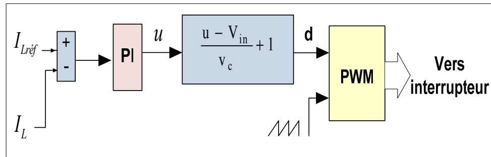
Figure 4.3 Schéma de la commande du convertisseur Boost
