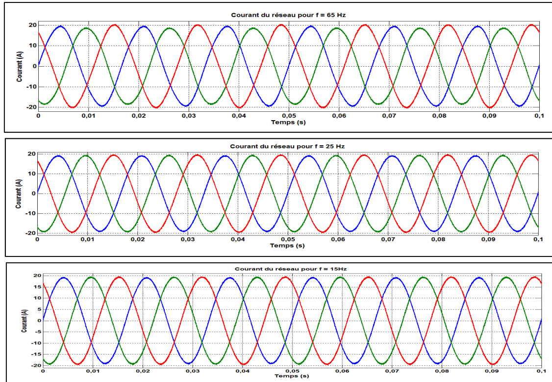
Figure 4.9 Courant du réseau en régime permanent pour f_c = 15\text{Hz} , 25\text{Hz} et 65\text{Hz}
