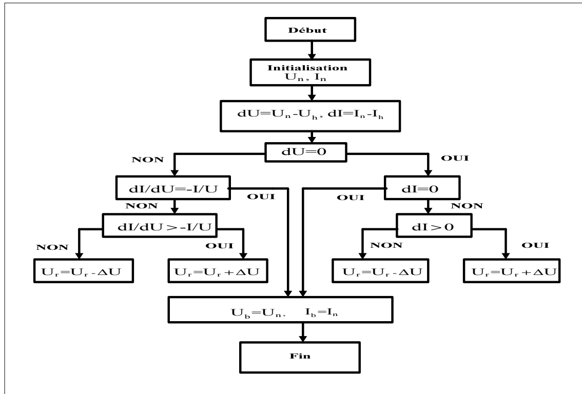
Figure 3.7 Algorithme du MPPT conductance incrémentale
