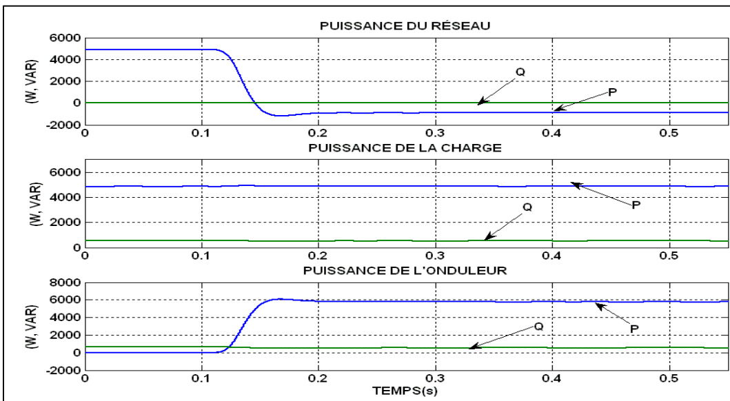
Figure 4.43 Écoulement de puissance avec ensoleillement G=800\text{W/m}^2
