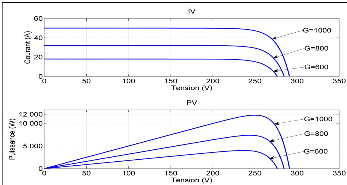
Figure 3.5 Courbe V-I et P-V des modules PV avec variation de l'ensoleillement
