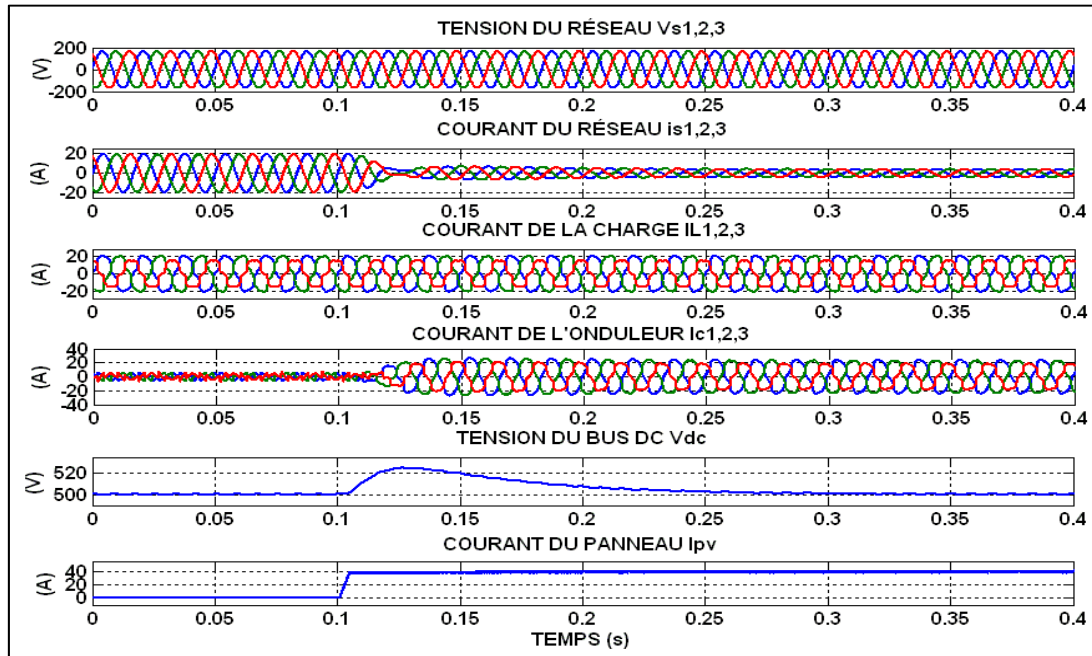
Figure 4.42 Réponse dynamique avec ensoleillement G=800\text{W/m}^2
