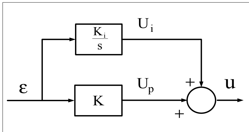
Figure 2.3 Schéma du régulateur PI
