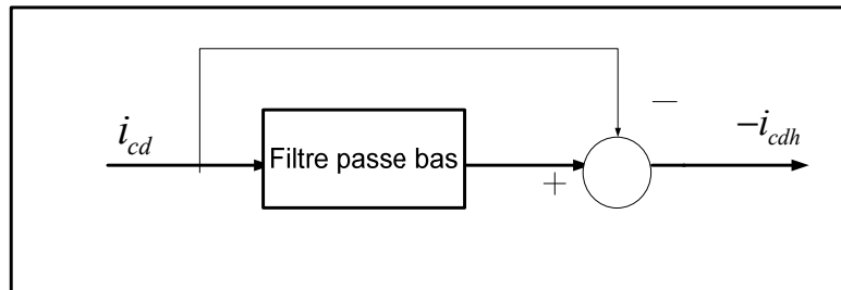
Figure 4.6 Schéma du principe d'extraction des courants harmoniques
