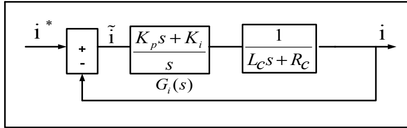
Figure 4.4 Schéma de la boucle interne du courant
