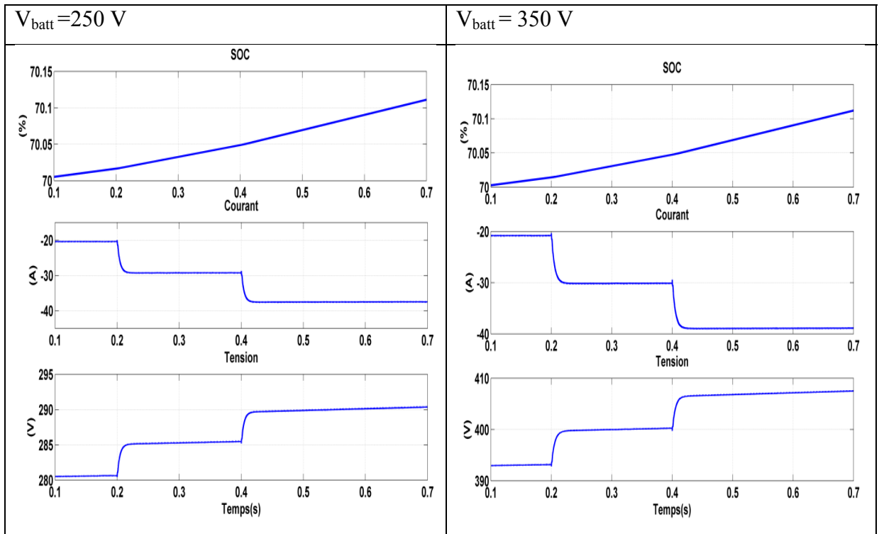
Figure 2.16 Résultat de simulation avec Sepic pour V_{\text{batt}} = 250 et 350 \text{ V}
