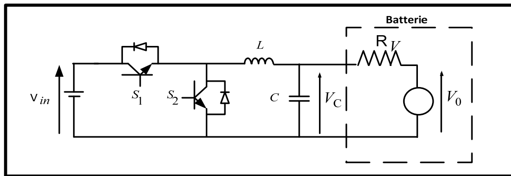
Figure 2.22 Schéma du montage du convertisseur Buck-Boost
