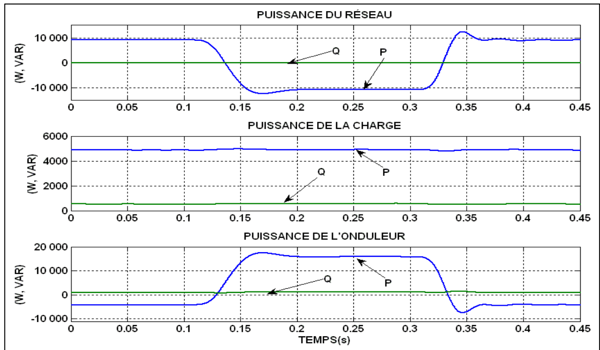
Figure 4.35 Écoulement de puissance avec variation de la charge de la batterie
