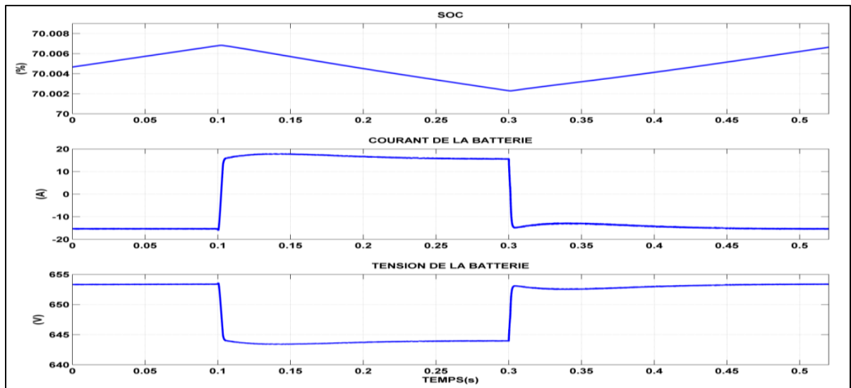
Figure 4.47 État de charge de la batterie
