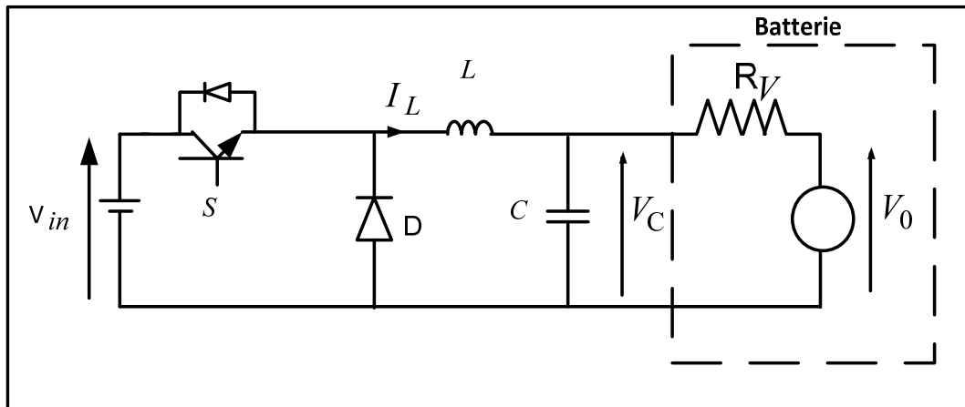
Figure 2.7 Schéma du montage du convertisseur Buck
