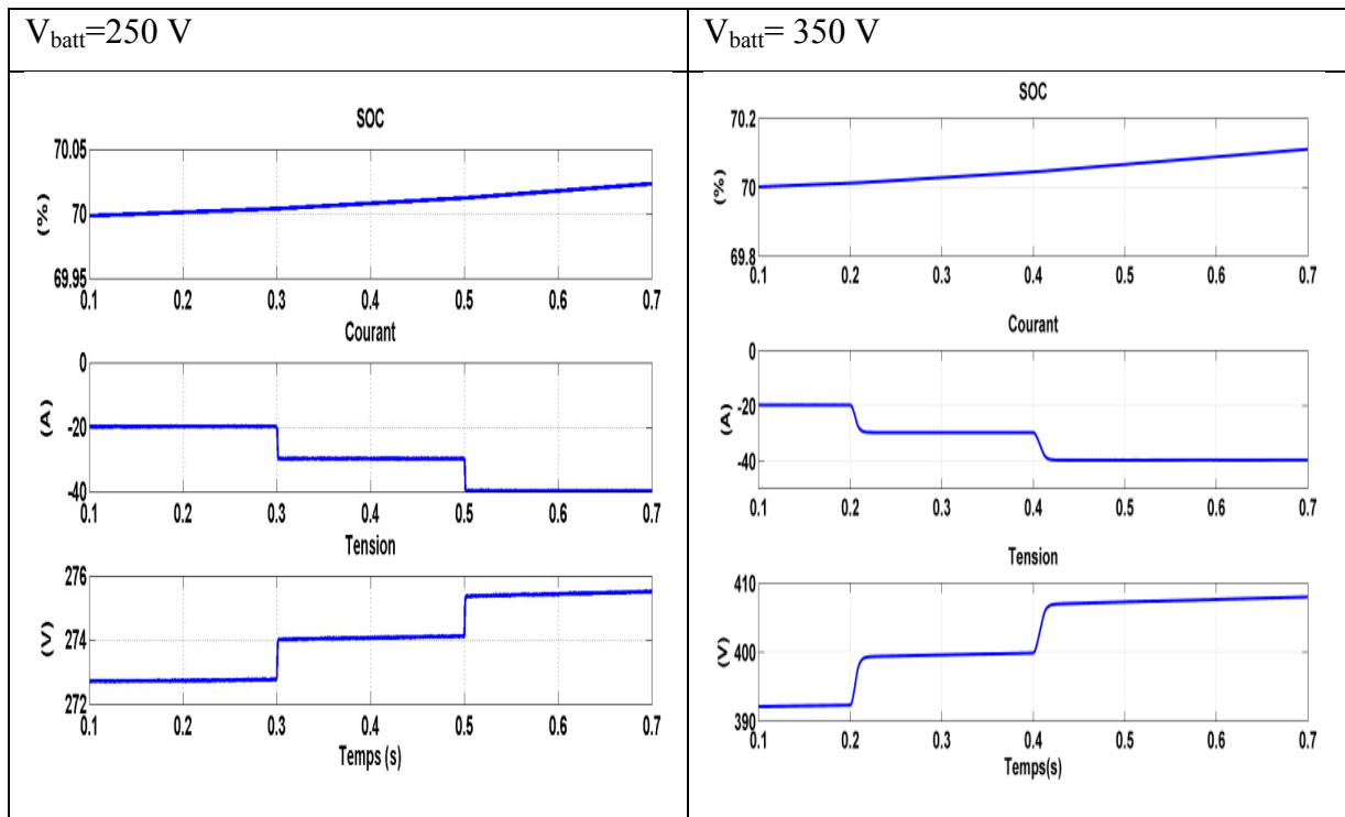
Figure 2.11 Résultat de simulation avec Buck pour V_{batt}=250 et 350\text{V}
