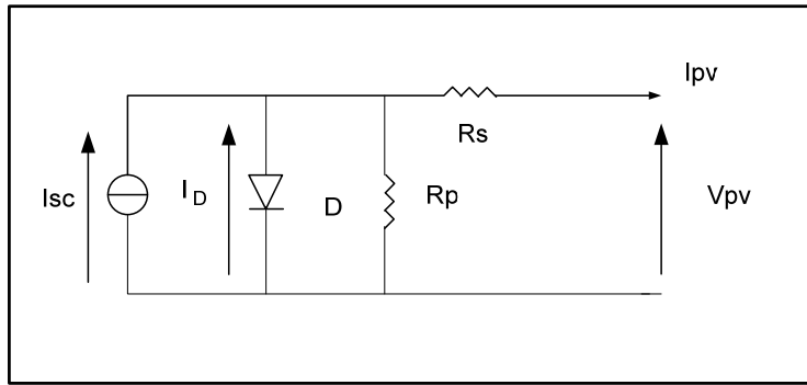
Figure 3.3 Modélisation du circuit électrique équivalent d'une cellule PV
