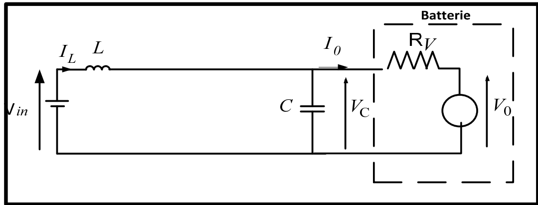
Figure 2.3 Schéma du convertisseur Boost quand l'interrupteur est bloqué
