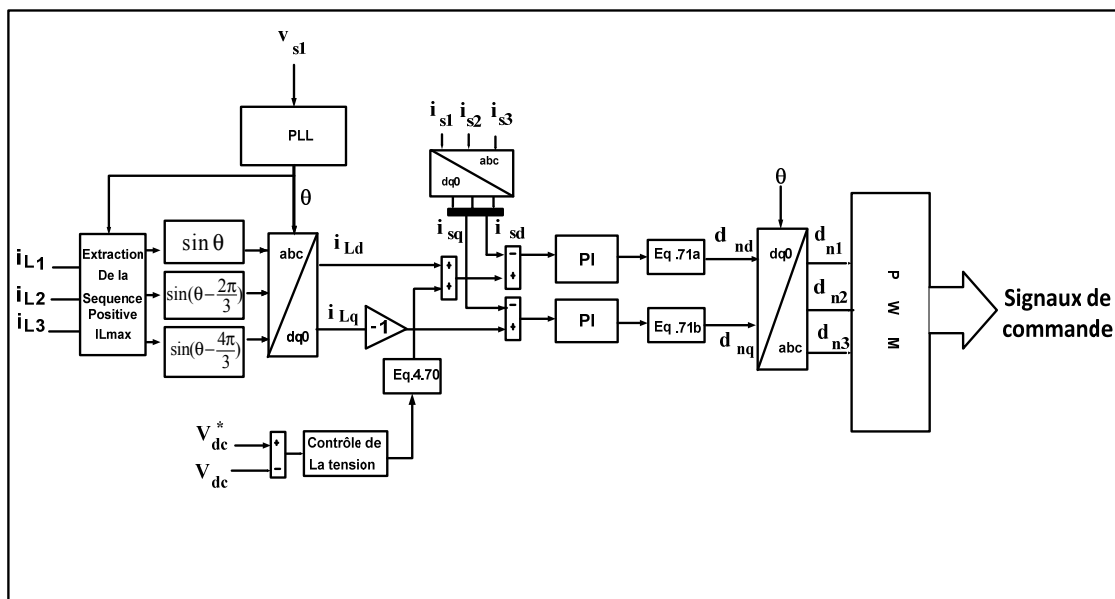
Figure 4.19 Schéma de la commande sans filtre de l'onduleur
