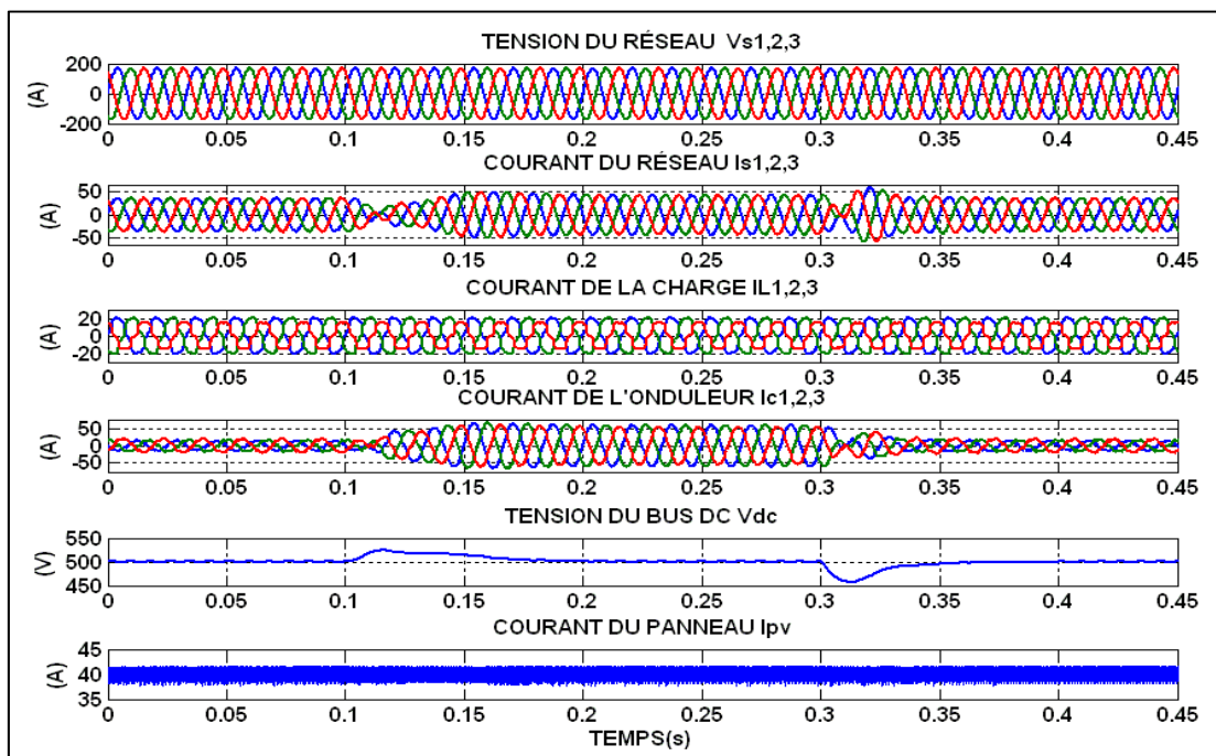
Figure 4.34 Réponse en régime dynamique avec variation de la charge de la batterie
