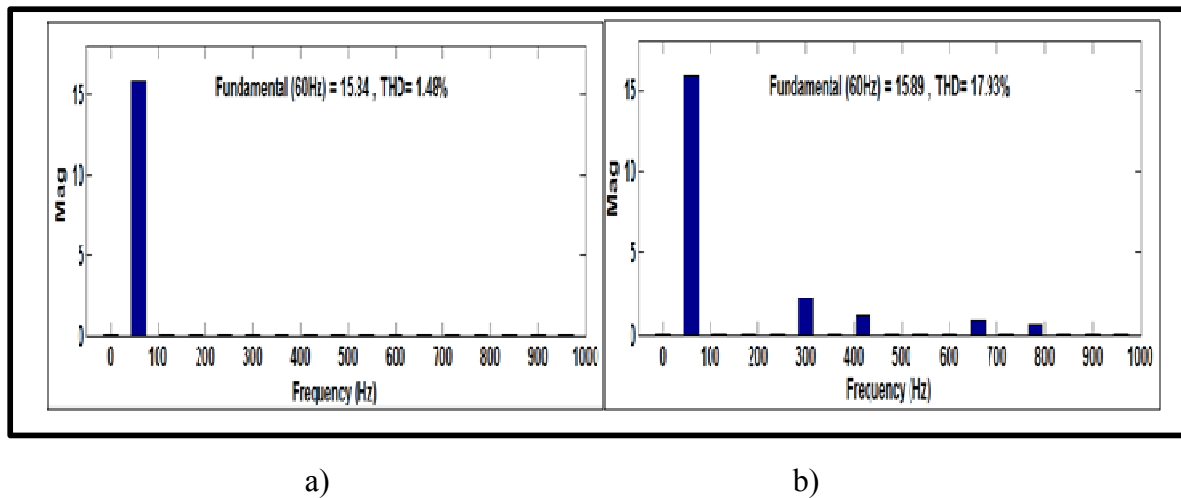
Figure 4.54 Spectre harmonique : a) du courant du réseau, b) du courant de la charge
