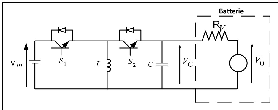
Figure 2.25 Schéma du montage du convertisseur Buck-Boost n°2
