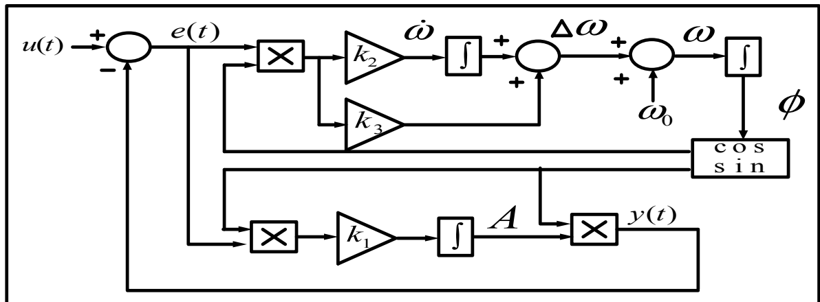
Figure 4.11 Schéma fonctionnel de l'ANF
