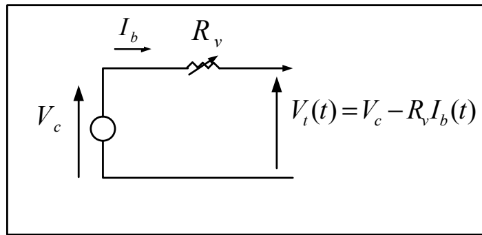
Figure 1.1 Modèle simplifié de l'accumulateur
