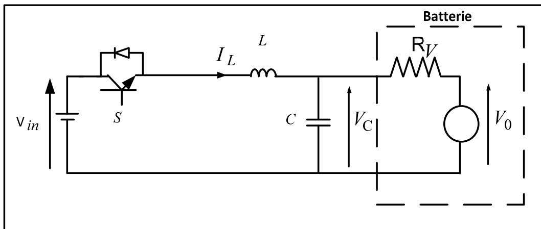
Figure 2.8 Schéma du montage du convertisseur quand l'interrupteur est passant
