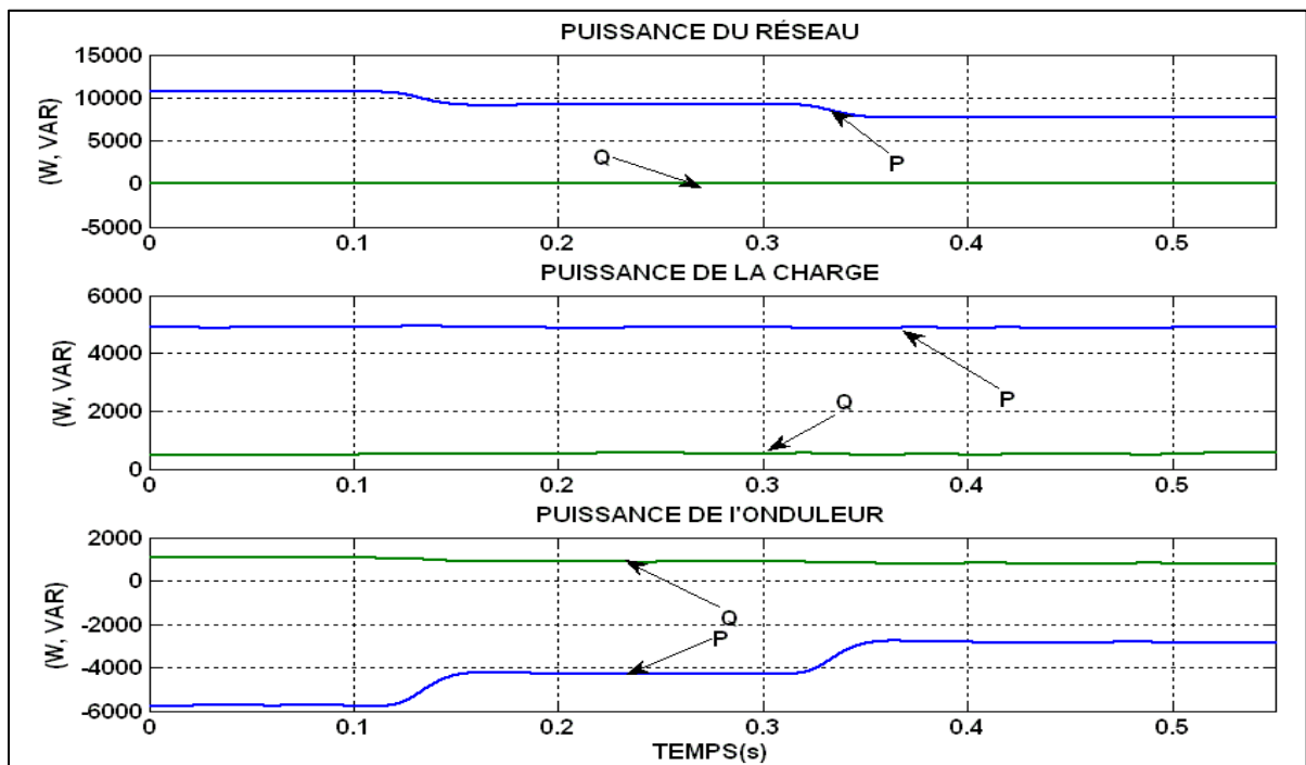
Figure 4.30 Écoulement de puissance avec variation de l'ensoleillement
