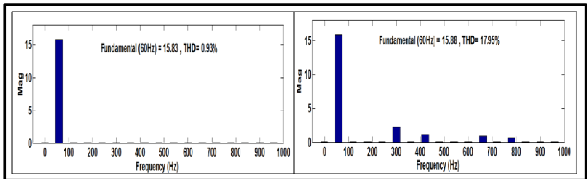
Figure 4.23 Spectre harmonique a) courant du réseau, b) courant de la charge
