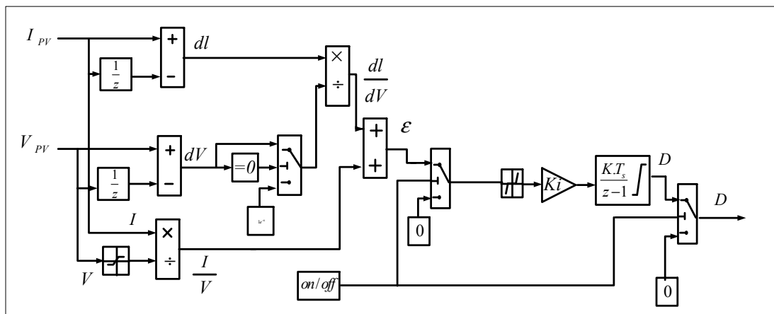
Figure 3.8 Schéma de la synthèse du MPPT sous Matlab/Simulink
