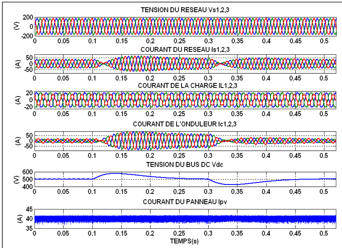
Figure 4.45 Réponse en régime dynamique avec variation de la charge de la batterie
