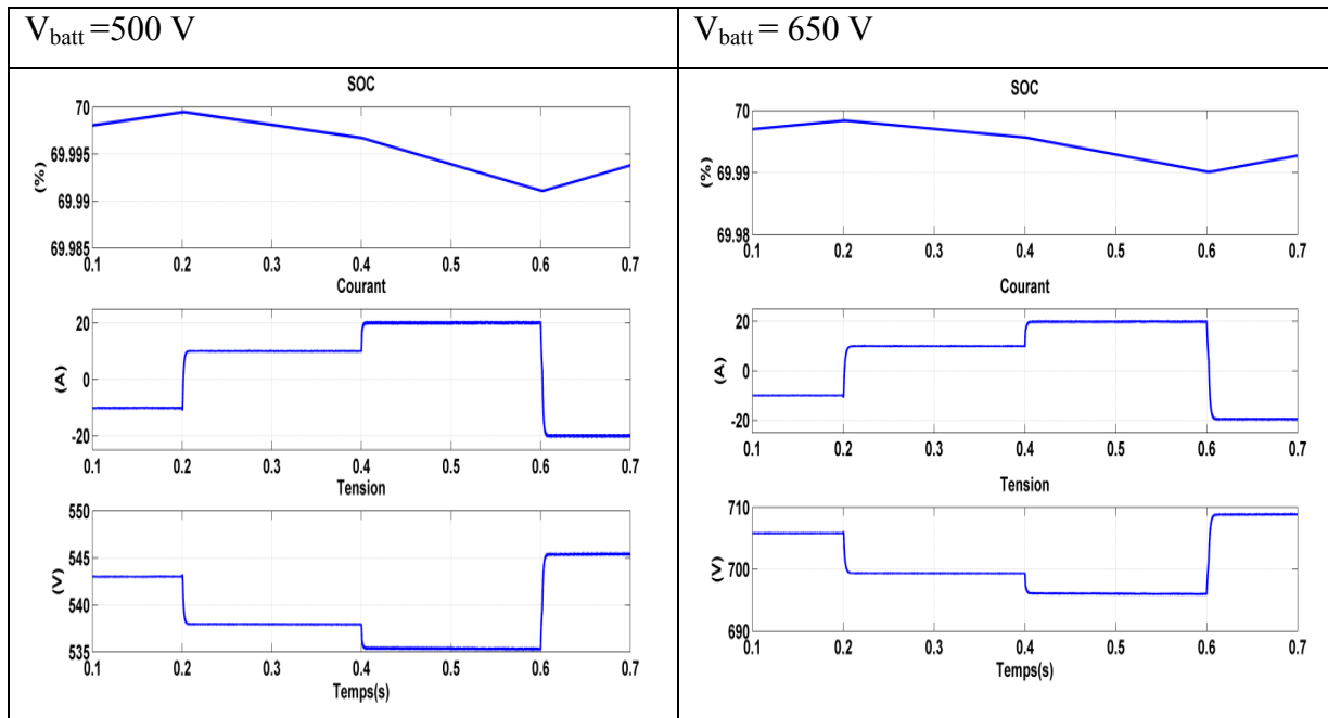
Figure 2.27 Résultat de simulation avec Buck-Boost modifié pour V_{\text{batt}} = 500 et 650 \text{ V}
