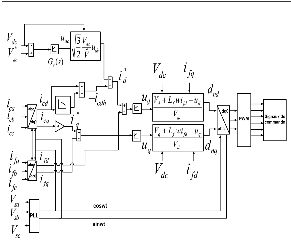
Figure 4.10 Schéma de la commande non linéaire
