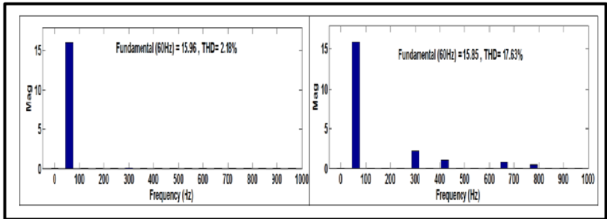
Figure 4.44 Spectre harmonique : a) courant du réseau, b) charge
