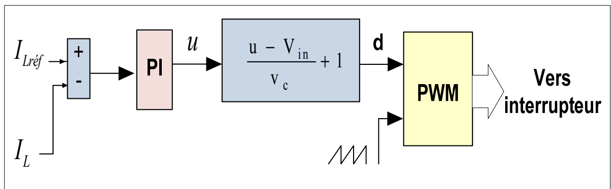
Figure 2.4 Commande du convertisseur Boost
