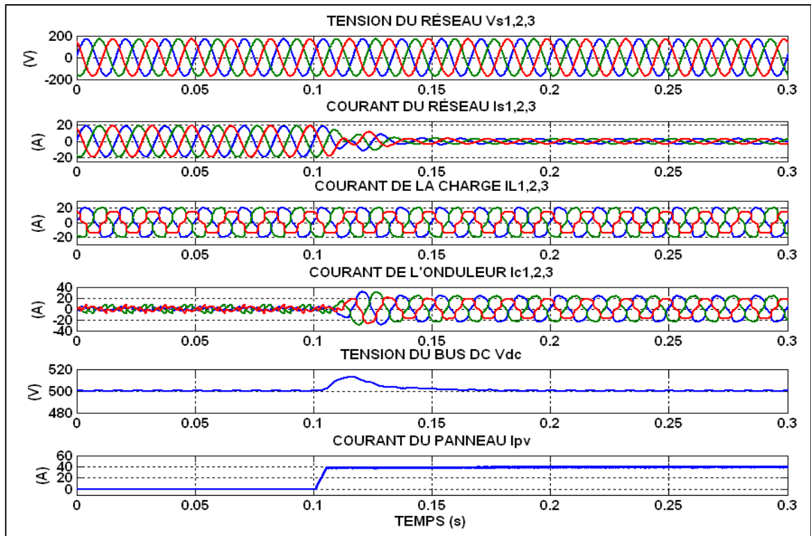
Figure 4.52 Réponse en régime dynamique avec ensoleillement G=800\text{W/m}^2
