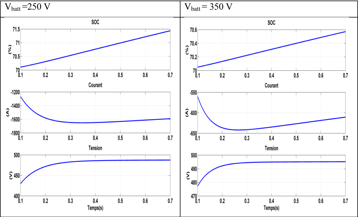
Figure 2.20 Résultat de simulation avec Boost-Buck pour V_{\text{batt}} = 250 et 350 \text{ V}
