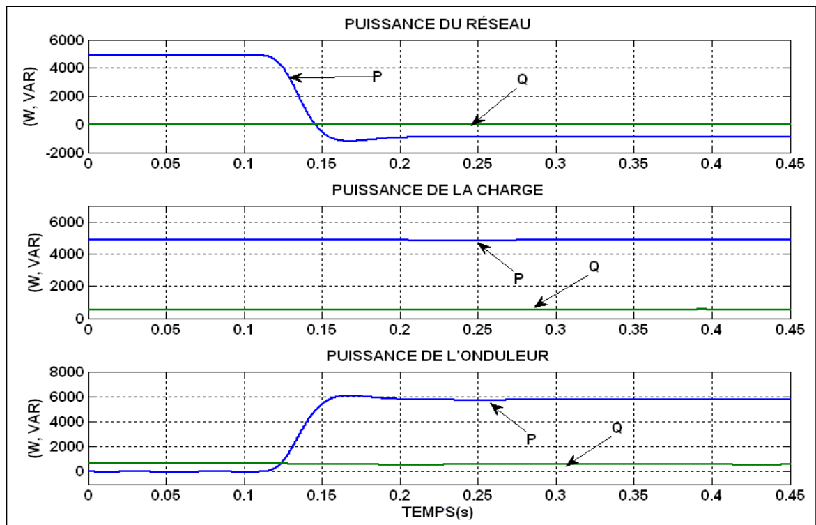
Figure 4.32 Écoulement de puissance avec ensoleillement G=800\text{W/m}^2
