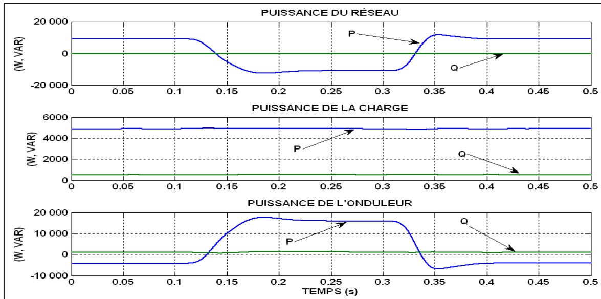
Figure 4.57 Écoulement de puissance avec variation de la charge de la batterie
