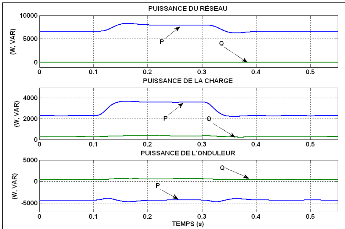
Figure 4.49 Écoulement de puissance avec variation de la charge
