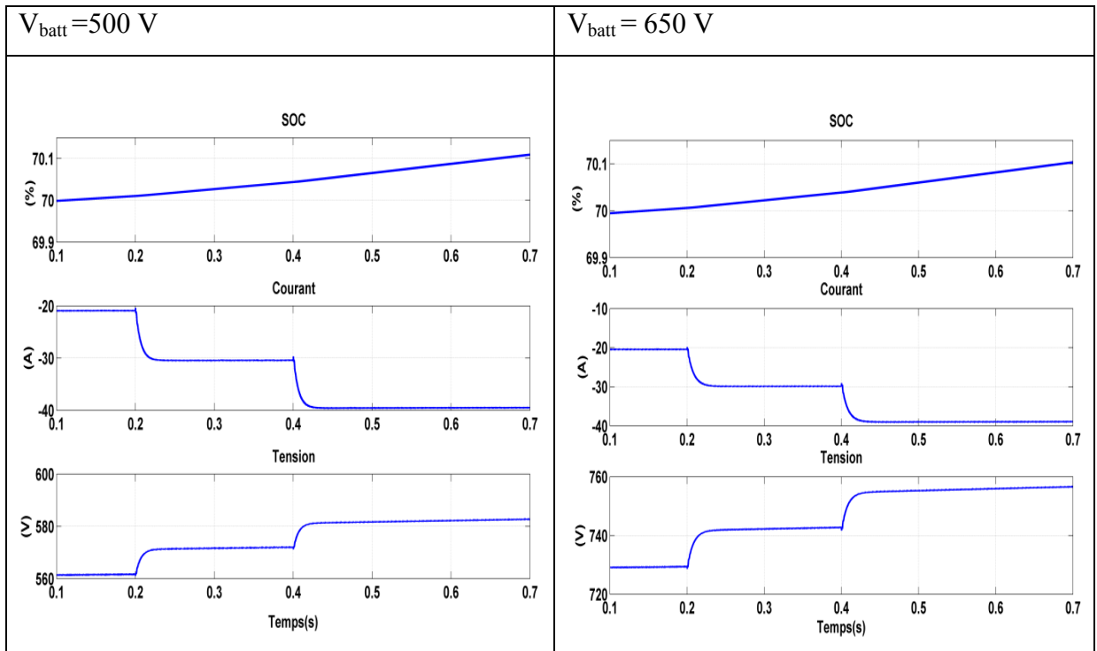
Figure 2.17 Résultat de simulation avec Sépic pour V_{\text{batt}} = 500 et 650 \text{ V}
