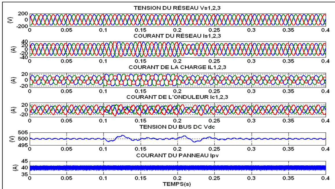
Figure 4.58 Réponse en régime dynamique avec variation de la charge
