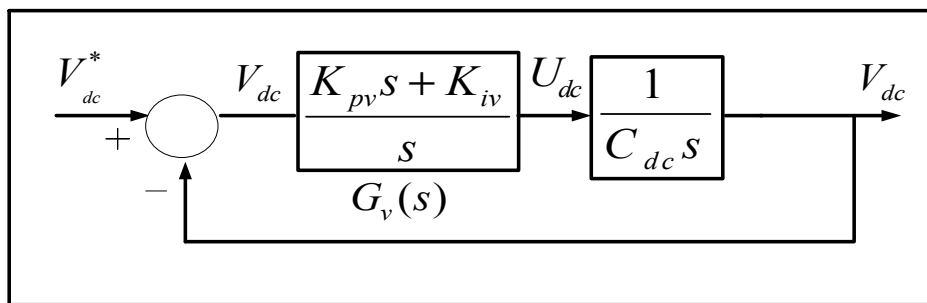
Figure 4.5 Schéma de la boucle externe de la tension
