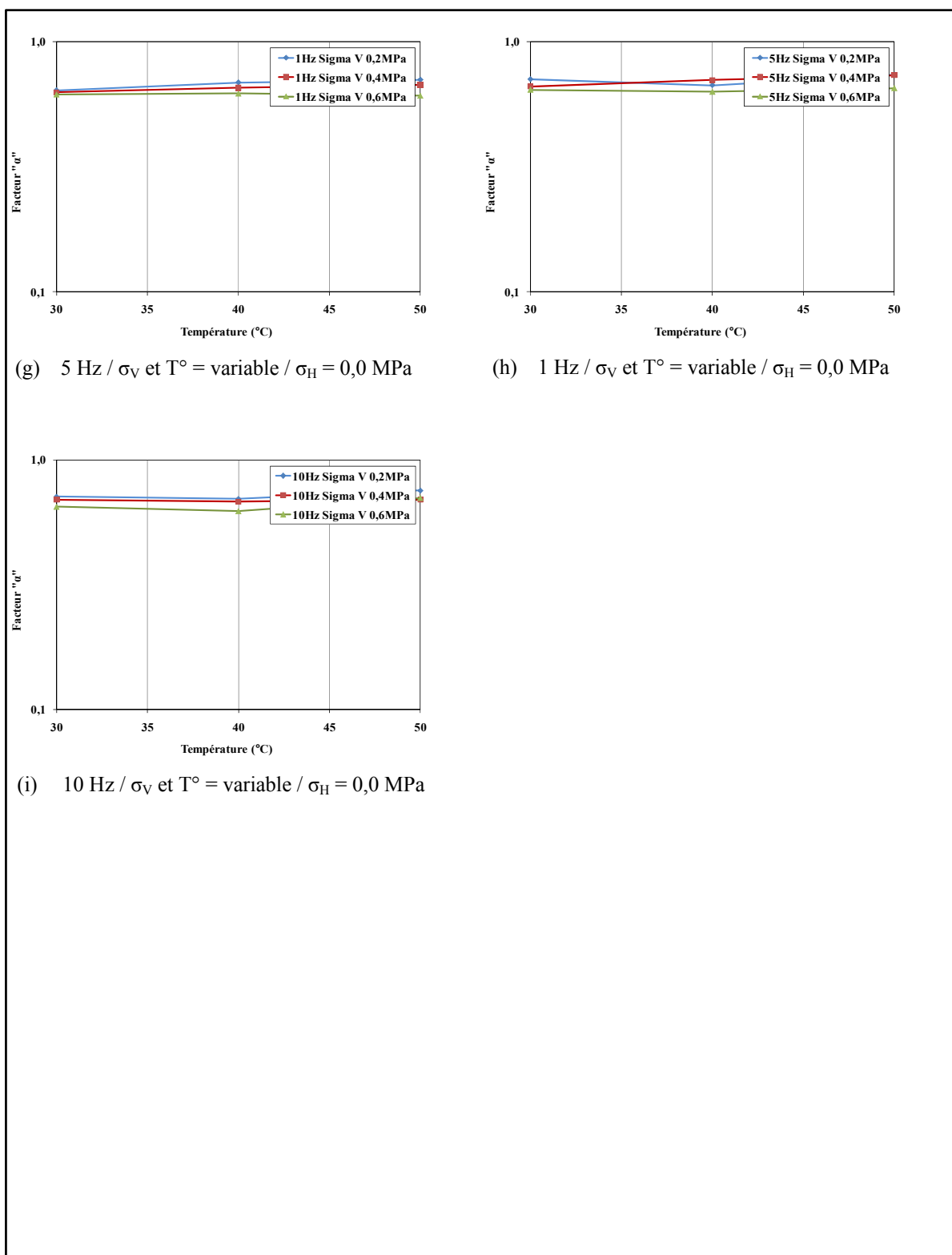
Figure-A XXIII-4 Synthèse des facteurs « \alpha » pour l'enrobé ESG-10 Partie 2 de 2
