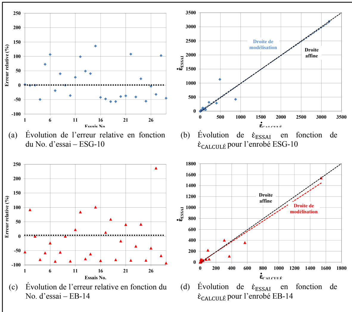
Figure 6.13 Analyses des erreurs relatives des valeurs de \dot{\varepsilon} obtenues suivant la nouvelle approche de modélisation des constantes du modèle ESSO
