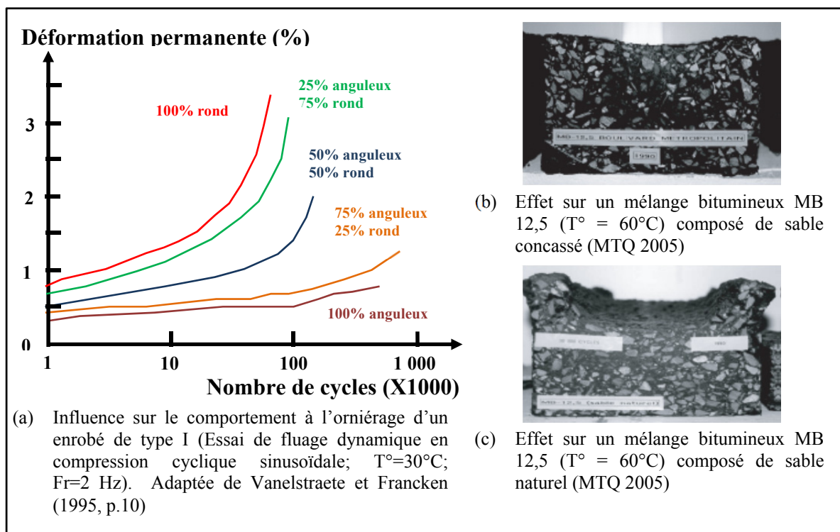
Figure 1.6 Effet de l'introduction de sable non concassé
