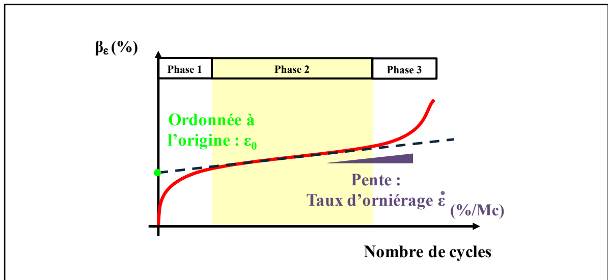
Figure 5.8 Courbe de déformation permanente typique d'où sont tirés les paramètres ESSO
