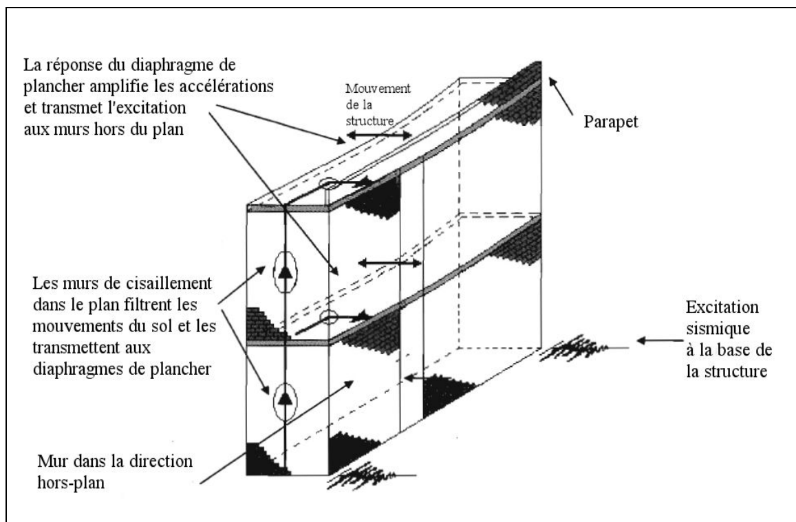
Figure 1.28 Représentation du chemin de l'énergie développée par le séisme et mise en évidence de l'effet de filtre dynamique du bâtiment Adaptée de Priestley et al. (2007)
