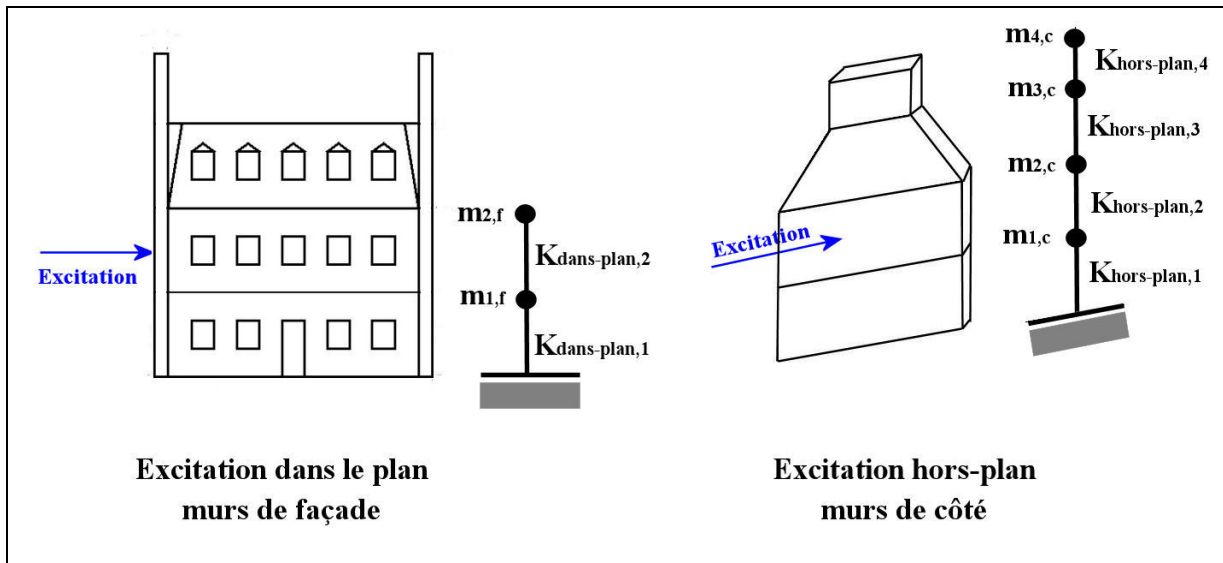
Figure 4.2 Modélisation à plusieurs DDLD et mise en évidence des deux systèmes dans le cas d'une excitation dans le plan des murs de façade pour un bâtiment de 2 étages
