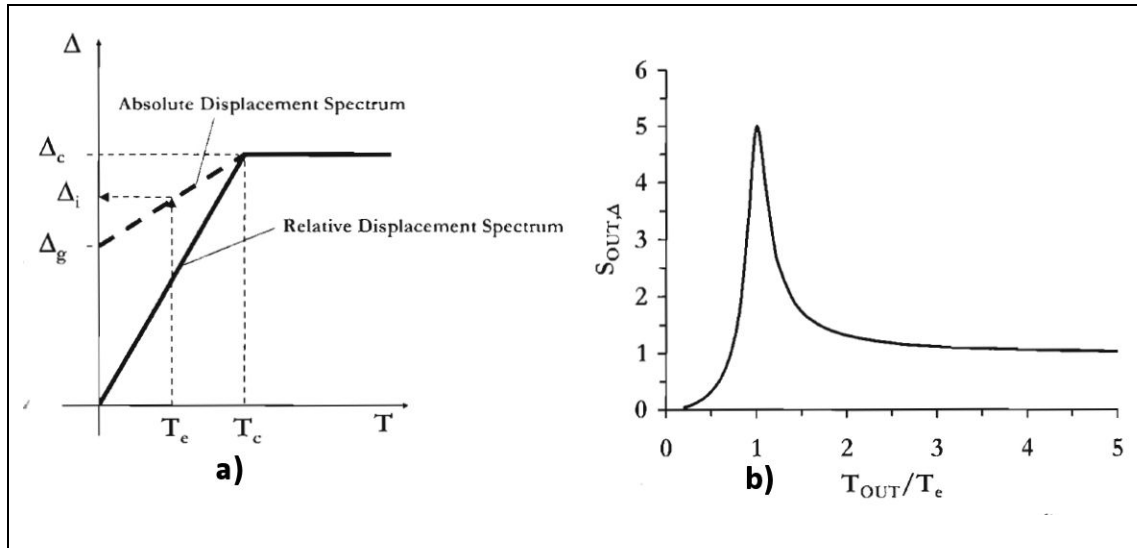
Figure 1.29 a) Spectre de déplacement absolu avec composante de sol \Delta_g b) Représentation graphique de la fonction de transfert du bâtiment pour un mur de maçonnerie dans la direction hors-plan avec \xi_{OUT} = 0.1 Tirée de Priestley et al. (2007)
