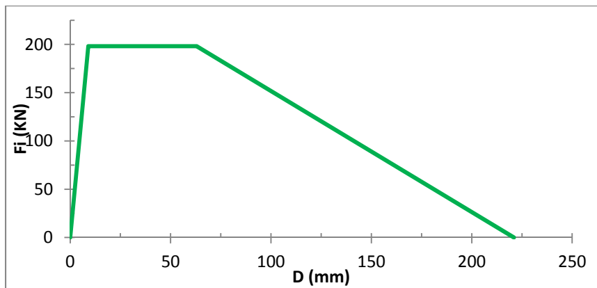
Figure-A VI-16 Modèle tri-linéaire du mur de côté – 2 ème étage
