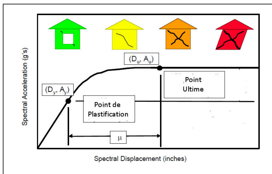
Figure 1.9 Exemple de courbe de capacité illustrant les points spécifiques et les positions approximatives des degrés de dommages Adaptée de FEMA (2003)
