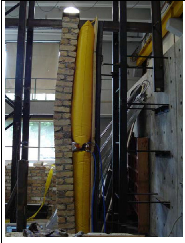
Figure 1.23 Dispositif à sac gonflable utilisé pour obtenir la courbe de capacité par analyse pushover, d'un mur de MNA dans la direction hors-plan Tirée de Derakshan et al. (2009)
