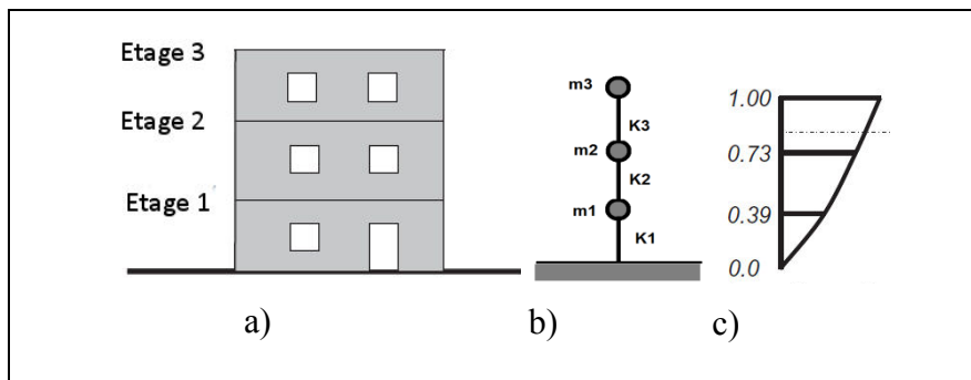
Figure 1.4 Exemple d'un système à plusieurs DDLD. a) Schéma du bâtiment de 3 étages, b) Modélisation du système à plusieurs degrés de liberté, c) Représentation des facteurs de formes et de la forme d'onde du premier mode de vibration Adaptée de Menon et Magenes (2011b)
