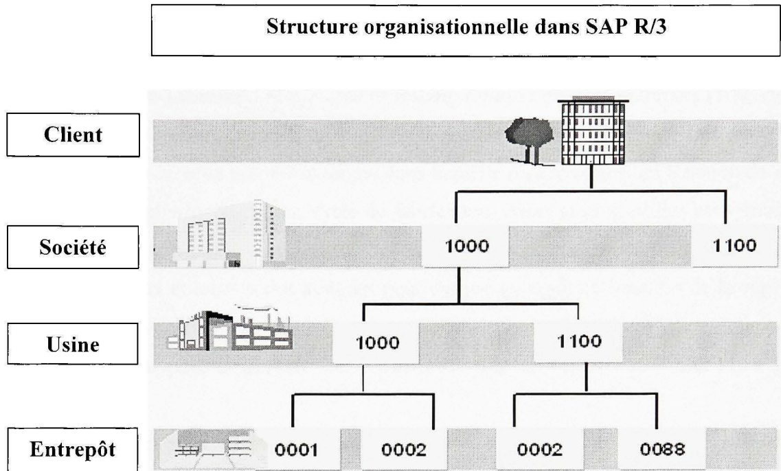
Figure 2.1 Structure organisationnelle dans SAP R/3.
