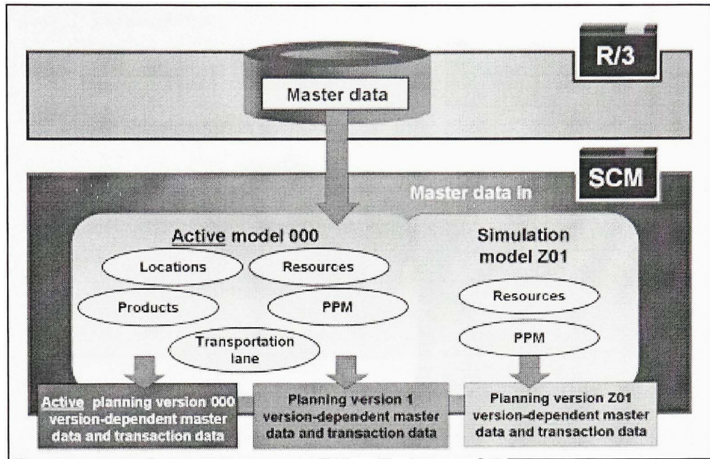
Figure 4.6 Le modèle actif « 000 ».
