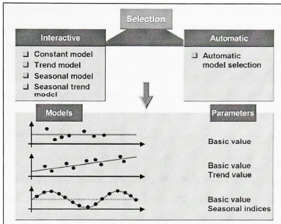
Figure 3.3 Sélection du modèle.
