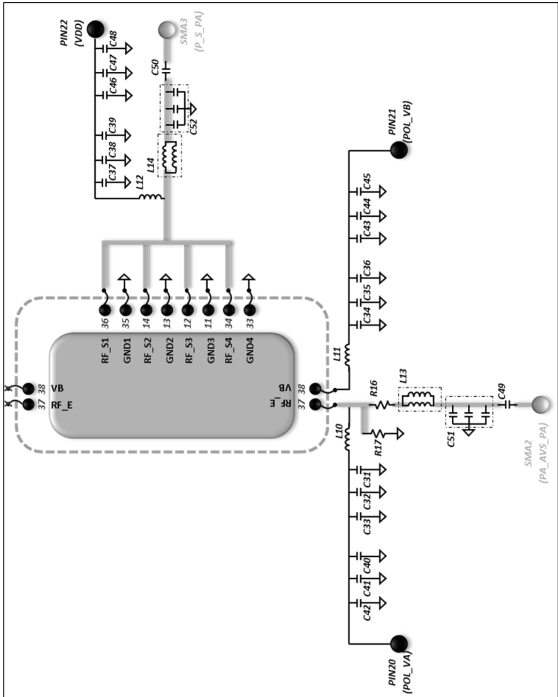
Figure-A II.4 Schéma électrique du PCB pour l'amplificateur
