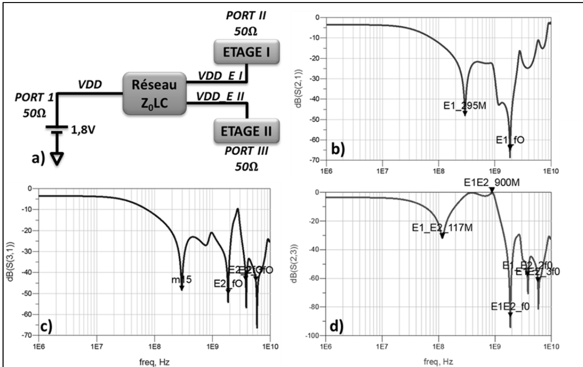
Figure 3.17 a) Schéma de test pour l'évaluation du réseau Z_0LC de filtrage d'alimentation b) Isolation entre l'étage I et la source DC c) Isolation entre l'étage II et la source DC d) Isolation entre l'étage I et l'étage II
