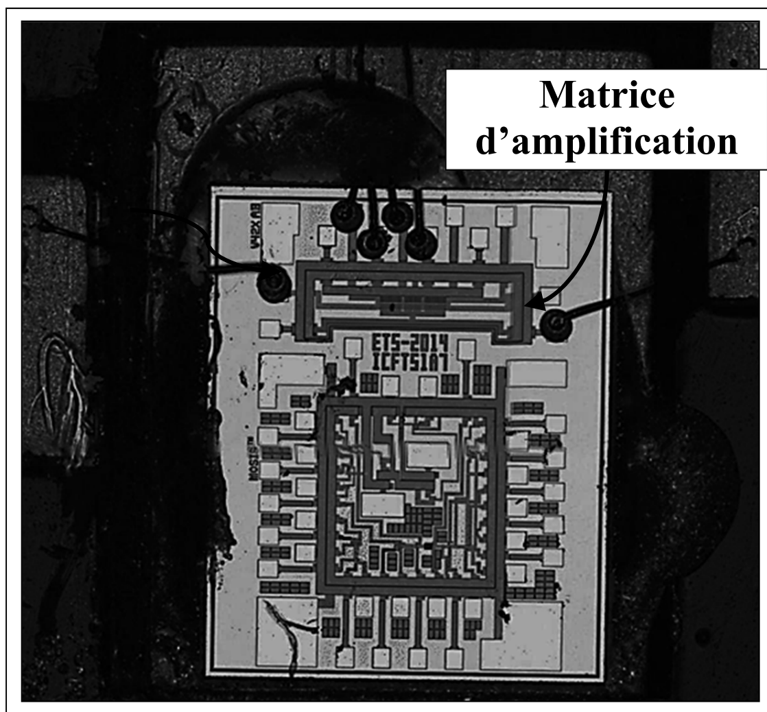
Figure-A II-11 Photo du montage de la puce pour les mesures de l'amplificateur
