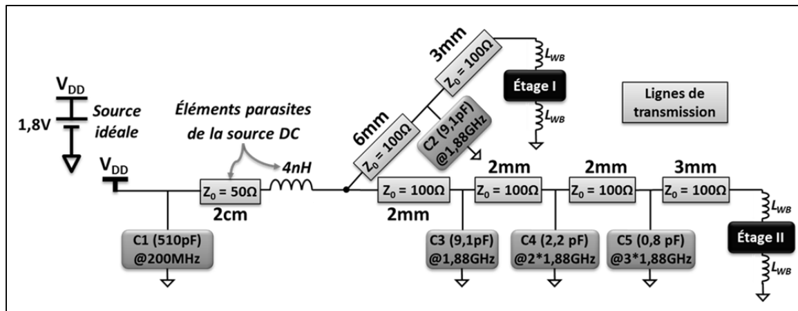
Figure 3.16 Schéma bloc du réseau Z_0LC de filtrage
