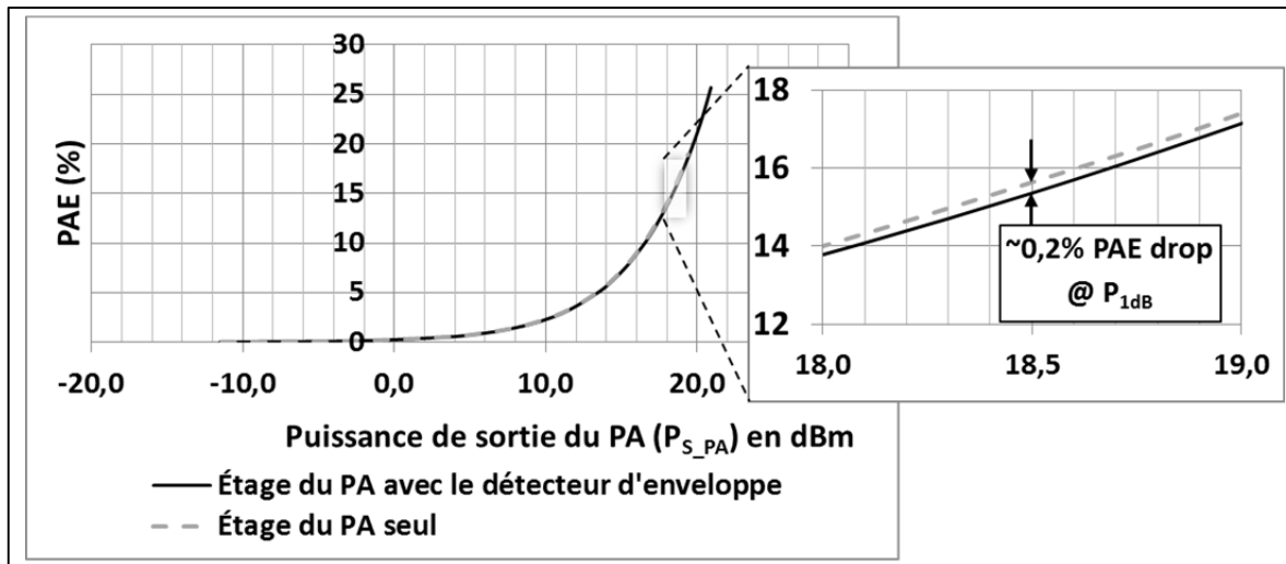
Figure 5.6 Efficacité (PAE) de l'amplificateur au sein du système RF comparée au PAE de l'amplificateur opéré seul
