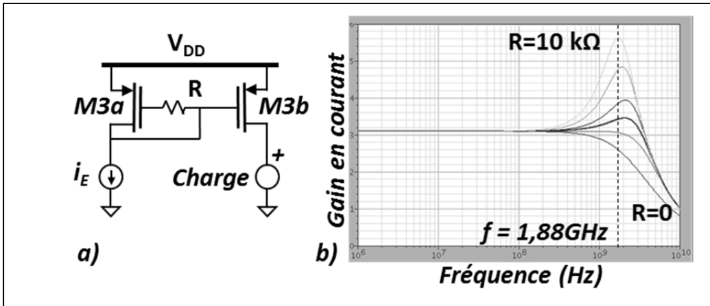
Figure 3.7 a) Miroir de courant PMOS modifié b) Réponse en fréquence du miroir de courant pour des valeurs de R allant de 0 à 10\text{ k}\Omega
