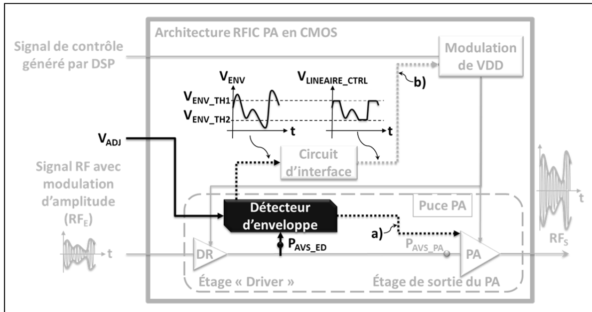
Figure 0.1 Architecture d'un RFIC PA à l'étude (en gris pâle) nécessitant le détecteur d'enveloppe conçu dans ce mémoire (en noir) avec trois signaux de contrôle pour : a) la modulation de la polarisation du PA en fonction de l'enveloppe b) la réduction du courant des circuits du bloc de modulation de V_{DD} en fonction des basses composantes en fréquence de l'enveloppe
