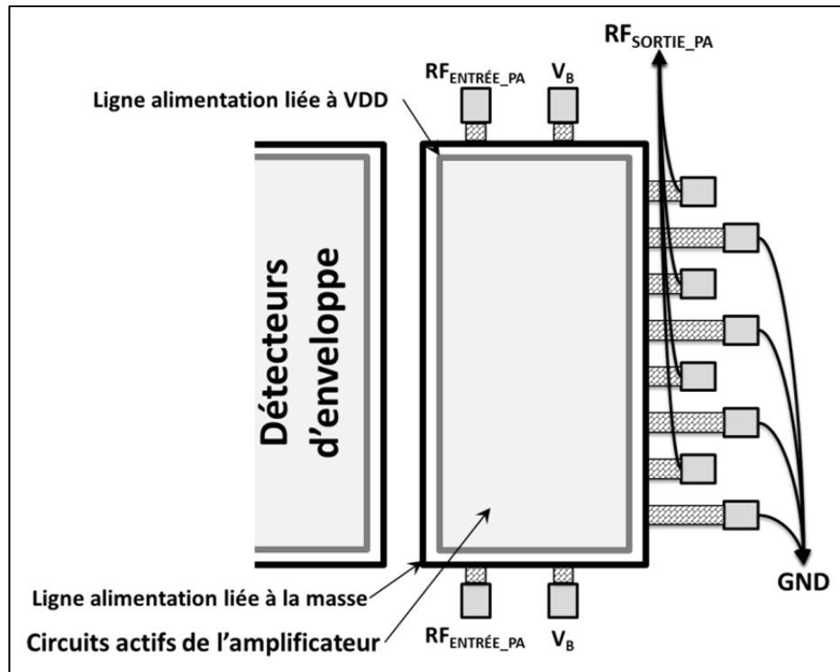
Figure 4.5 Structure des lignes d'alimentation et des plots
