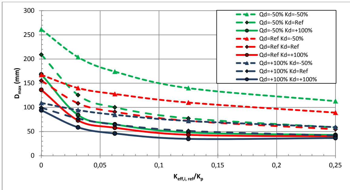
Figure 5.13 Variation du déplacement maximal de l'ouest D_{\max} de l'Ouest en fonction du rapport de la rigidité effective de l'isolateur de référence par la rigidité de la pile K_{eff,i,ref}/K_p pour différents taux de paramètres hystérétiques ( Q_d, K_d ) selon le CNBC 2010
