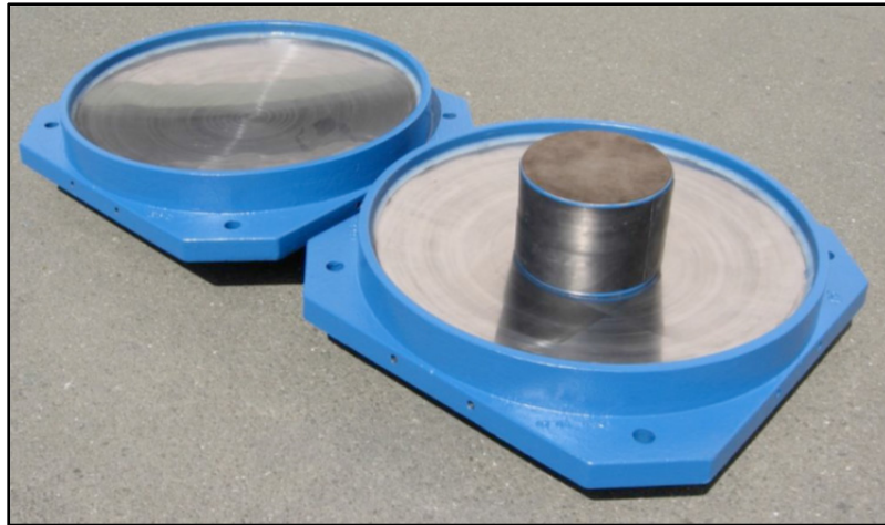
Figure 1.21 Exemple de pendule à friction Tirée de Ogorzalek et Stephen (2010)
