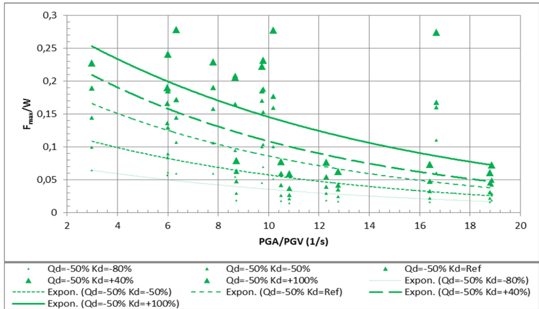
Figure-A III-7 Variation de la force maximale par ratio du poids sismique F_{max}/W en fonction des caractéristiques des séismes PGA/PGV pour différents K_d et Q_d = -50\% a) (points) Valeurs b) (courbe) approximation exponentielle
