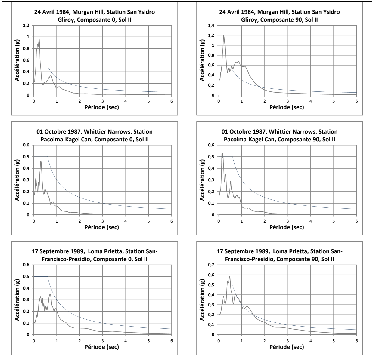
Figure-A II-4 Spectres de réponse avant calibration pour les séismes de (station) : Morgan Hill, 1984 (San Ysidro Gliroy), Whittier Narrows, 1987 (Pacoima-Kagel Can), Loma Prieta, 1989 (San-Francisco-Presidio) et Northridge, 1994 (San Pedro et Castaic Old Rte) et le spectre cible de Vancouver pour le sol de classe II
