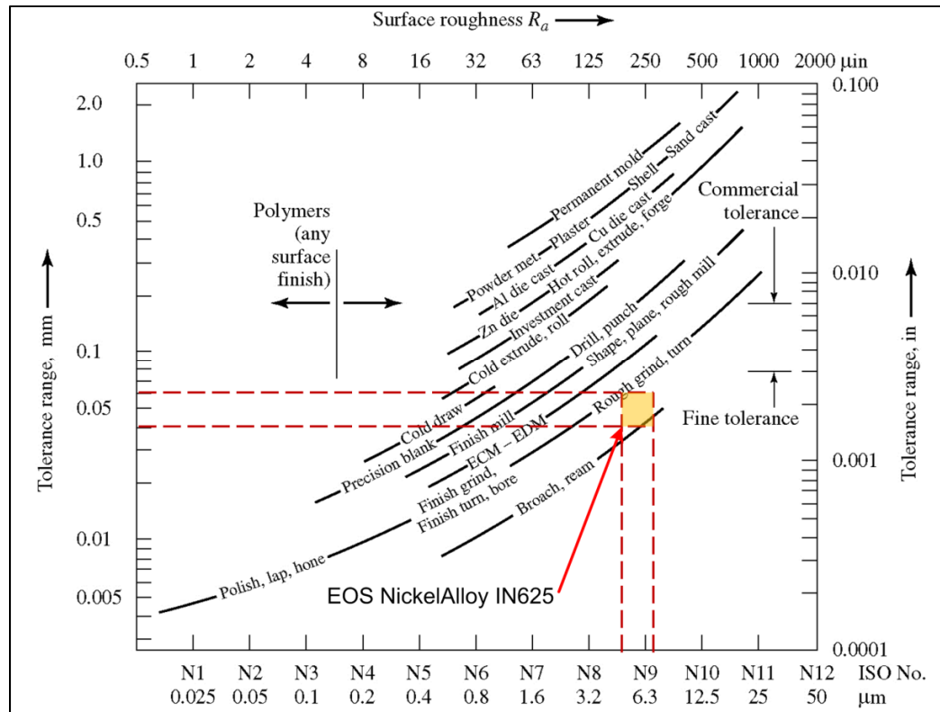
Figure 1.5: Fini de surface en regard des tolérances de fabrication de différentes techniques de fabrication. Tirée et adaptée de Schey (1987)
