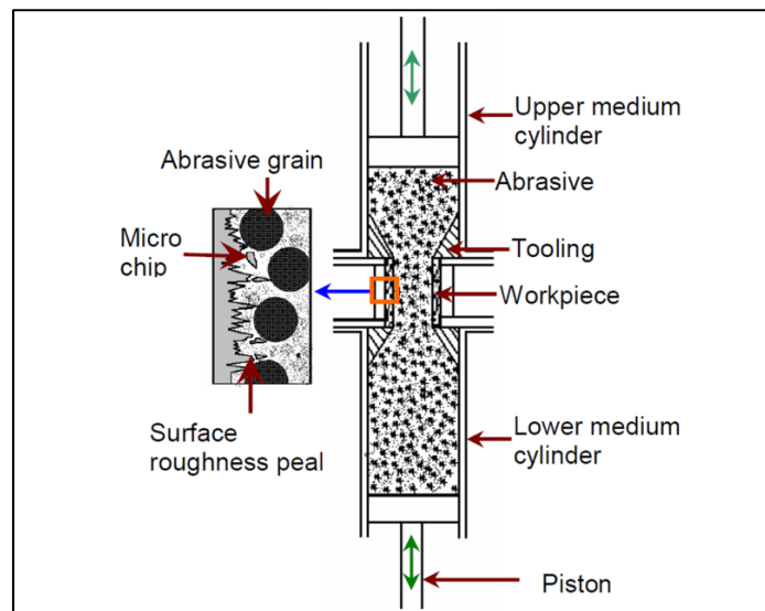
Figure 1.18: Principe d'enlèvement de matière de l'AFM (Sankar, Jain et Ramkumar, 2011)
