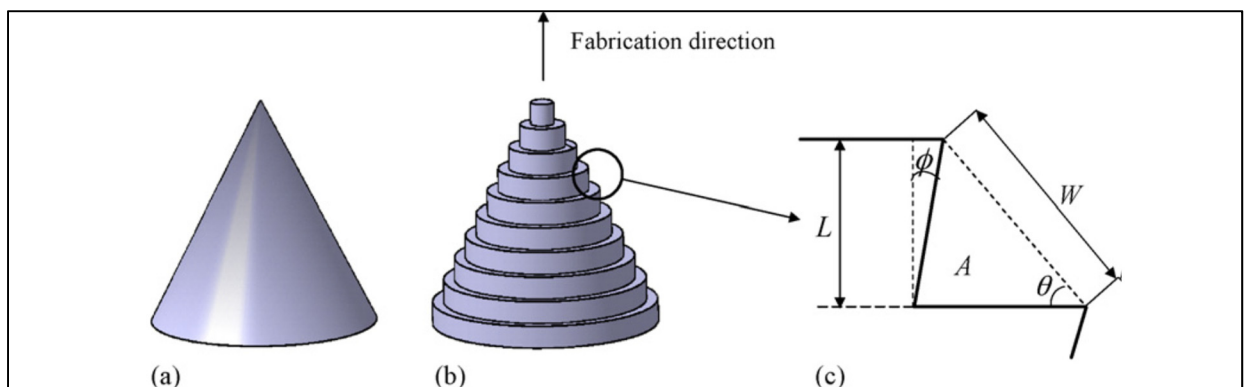
Figure 1.11: Effet d'escalier dans la FA: (a) modèle CAO; (b) découpage en tranches de la pièce; (c) schématisation du profil de surface (Ahn, Kim et Lee, 2009)
