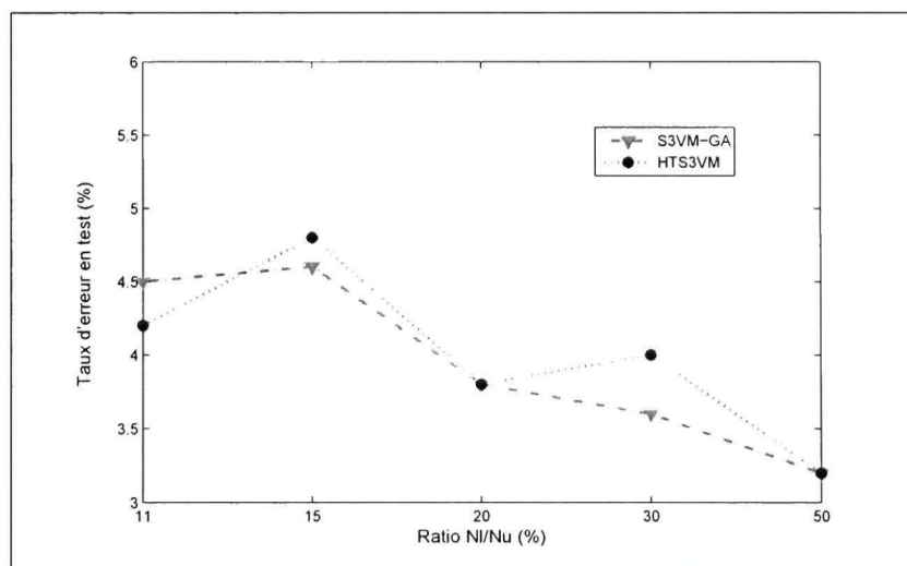
Figure 5.5 Variation de la performance des classifieurs S^3VM en fonction du ratio \frac{N_l}{N_u} sur la base Text.
