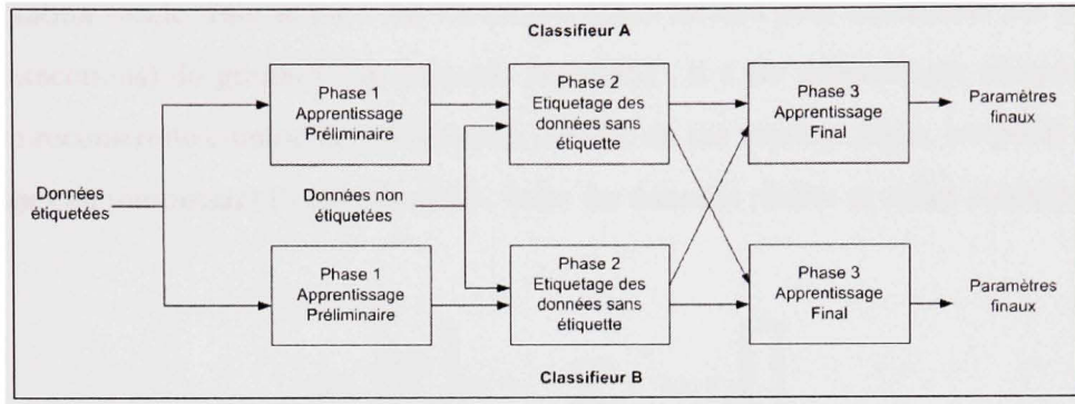
Figure 1.4 Représentation schématique du co-apprentissage.
