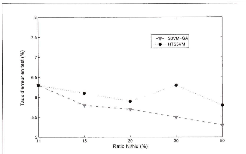
Figure 5.4 Variation de la performance des classifieurs S^3VM en fonction du ratio \frac{N_l}{N_u} sur la base Gaus50.
