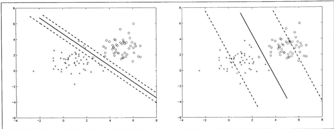
Figure 1.6 Figures montrant la marge et l'hyperplan de séparation trouvés par la SVM (à gauche) et par la LS-SVM (à droite) pour un problème binaire 2D.
