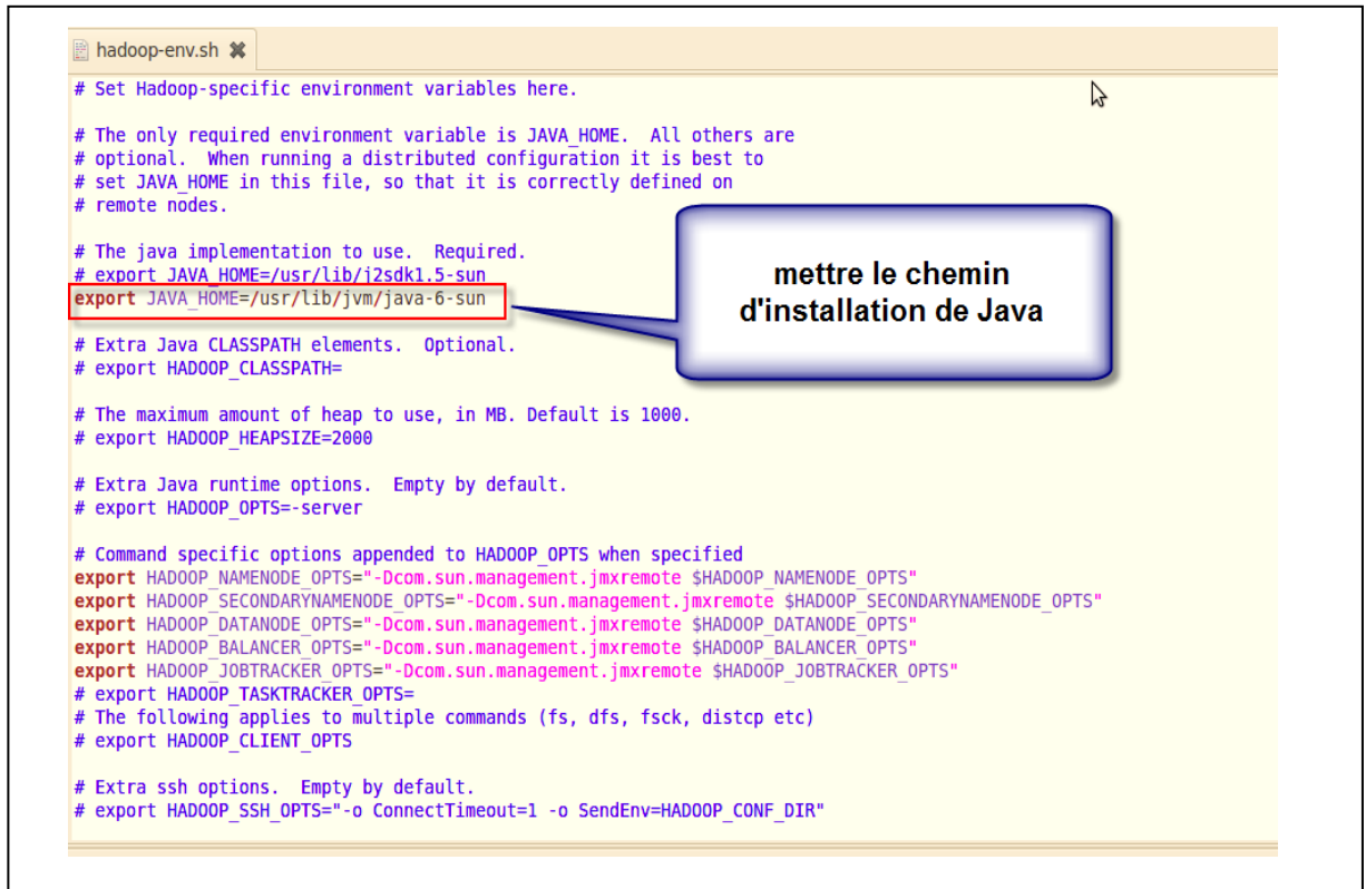
Figure III.12 Configuration de la variable globale de Java pour hadoop
