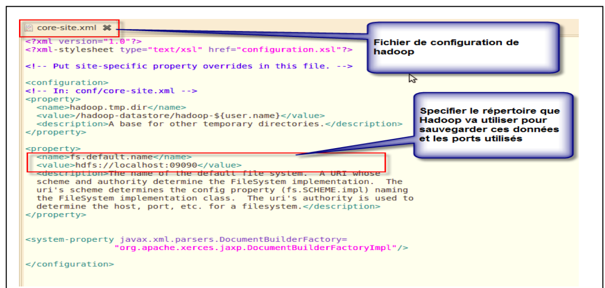
Figure III.2 Configuration du système du fichier de Hadoop
