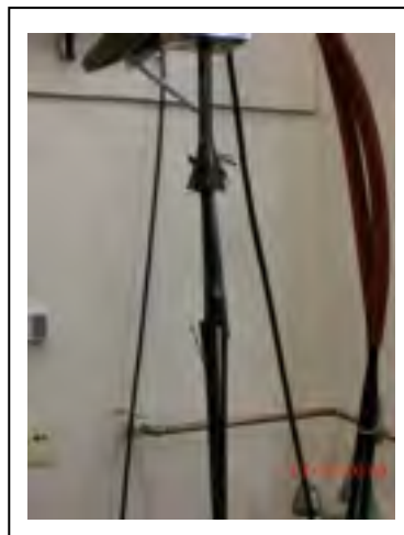
Figure 4.11 Rupture d'une barre en CFRP soumise à la traction
