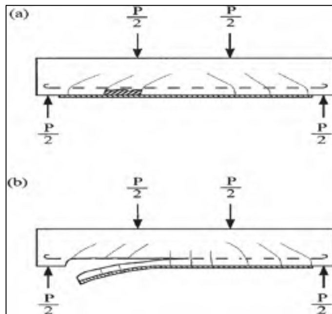
Figure 3.3 Mode de rupture le plus répandu dans le système poutre : (a) décollement de la plaque de FRP, (b) décollement de la couche de béton Tirée de Chaallal et al (1998)
