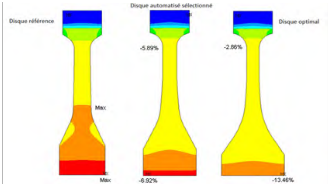
Figure 3.12 Contraintes mécaniques de 3 disques LPT
