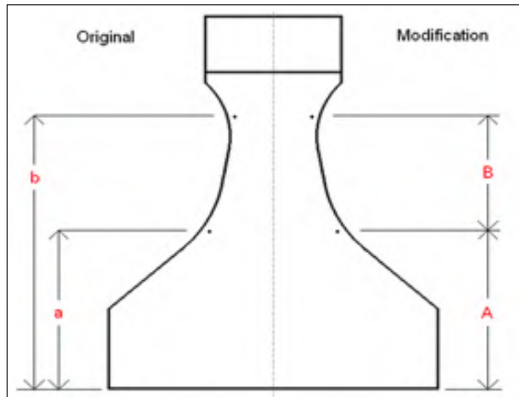
Figure 3.4 Modification du dimensionnement des côtés du disque
