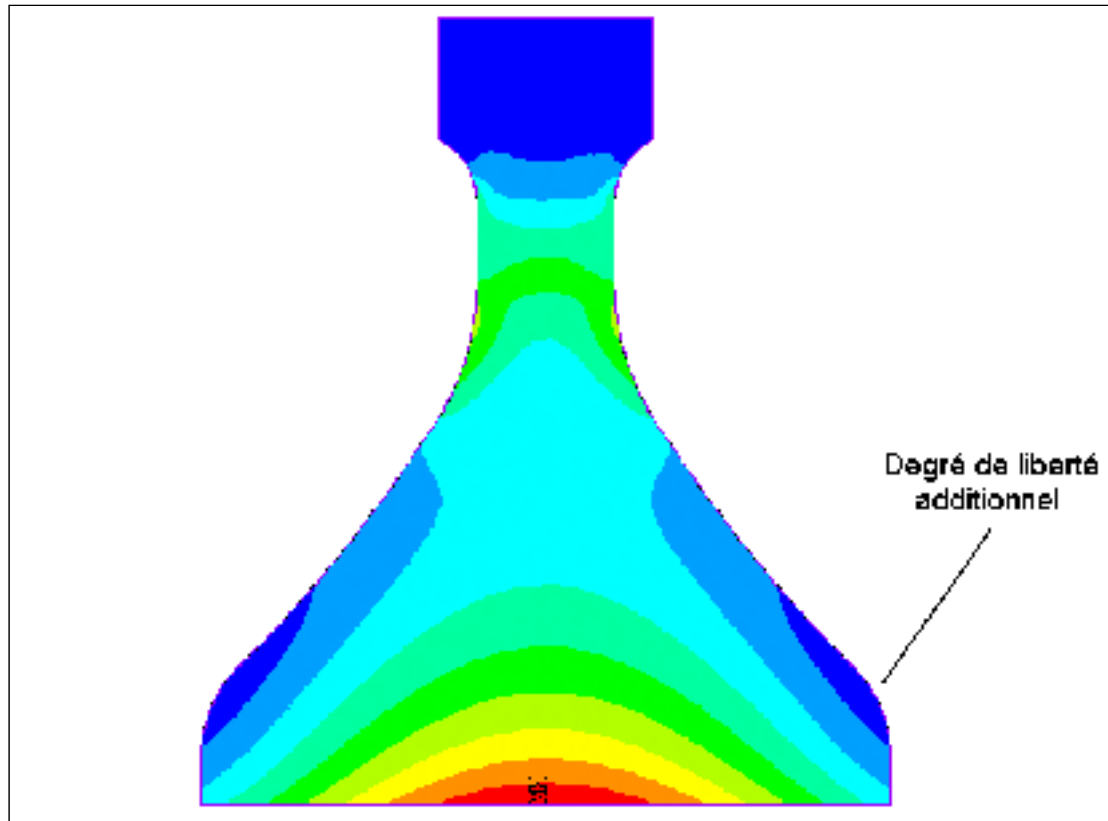
Figure 3.20 Géométrie optimisée du modèle #4
