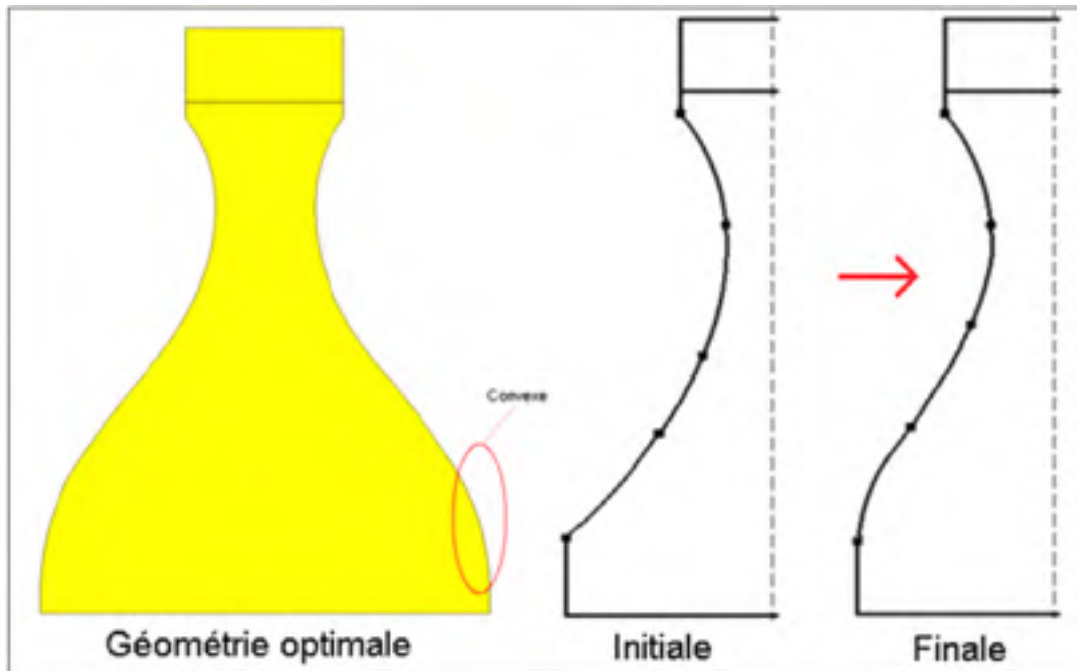
Figure 3.19 Géométrie optimale
