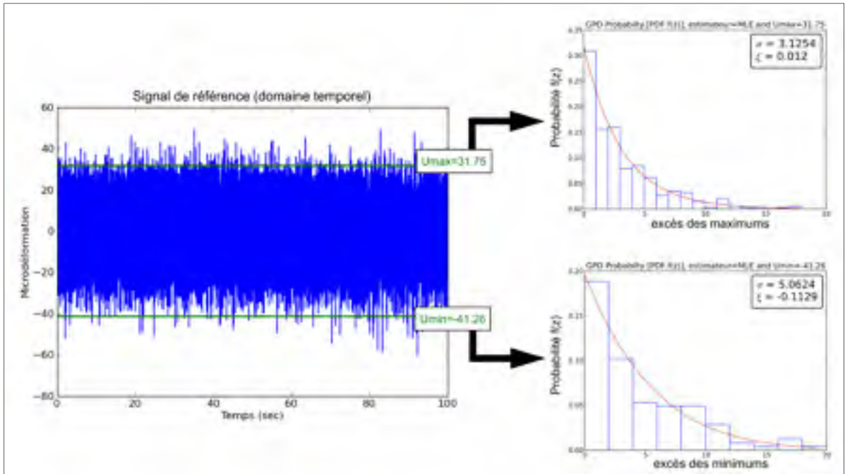
Figure A.68 Modélisation avec la théorie des valeurs extrêmes à la condition d'opération de pleine charge (GTA2)
