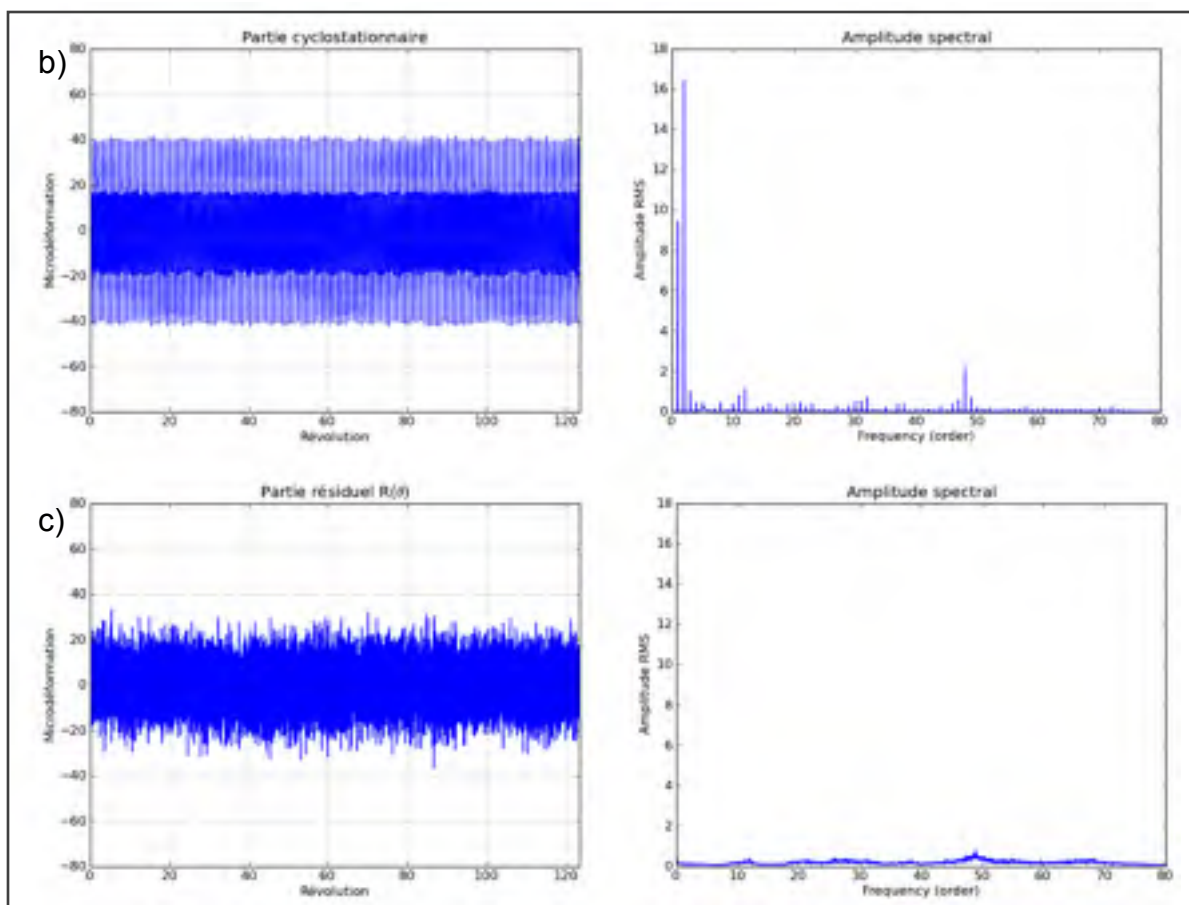
Figure A.48 Domaine angulaire et fréquentiel du a) signal de référence; b) partie cyclostationnaire; c) partie résiduelle (condition d'opération PC du GTA1)
