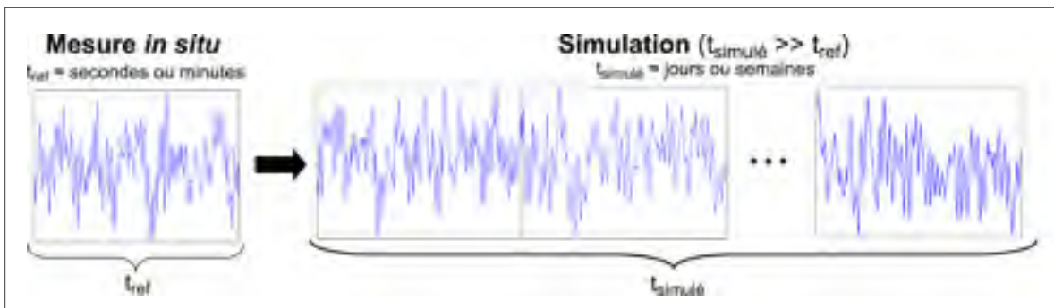
Figure 1.1 Exemple d'un signal de référence mesuré par rapport au signal simulé
