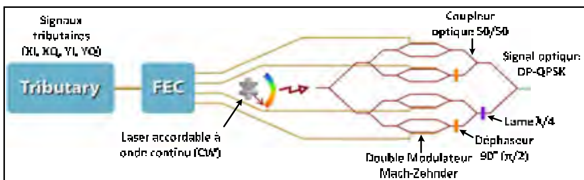
Figure 2.4 Schéma à haut niveau du transmetteur cohérent DP-QPSK Adaptée de Roberts et al. (2009, p.3)
