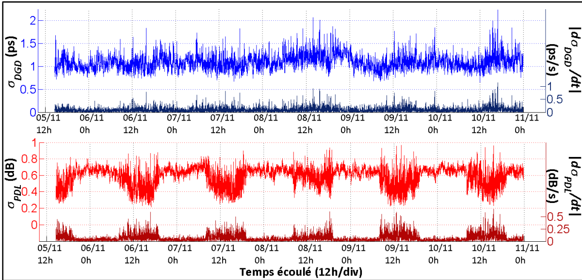
Figure 3.10 Évolution temporelle des valeurs de \sigma_{DGD} , de \sigma_{PDL} , de |d\langle\sigma_{DGD}\rangle/dt| et de |d\langle\sigma_{PDL}\rangle/dt| à chaque minute sur le lien optique cohérent du réseau Verizon
