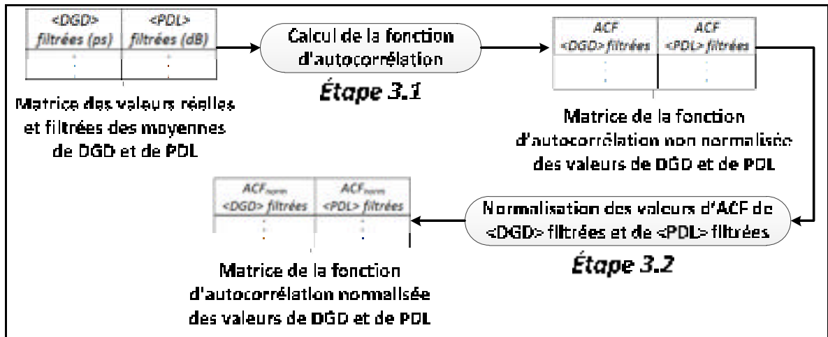
Figure 3.15 Séquence de calcul de la fonction d'autocorrélation normalisée sur les valeurs de <DGD> filtrées et sur les valeurs de <PDL> filtrées
