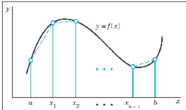
Figure-A XXVI-1 Représentation de la méthode des trapèzes Tirée de Kreyszig et al. (2011)
