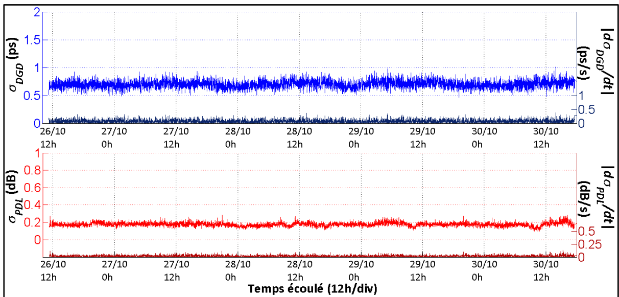
Figure 3.9 Évolution temporelle des valeurs de \sigma_{DGD} , de \sigma_{PDL} , de \left| \frac{d\langle \sigma_{DGD} \rangle}{dt} \right| et de \left| \frac{d\langle \sigma_{PDL} \rangle}{dt} \right| à chaque minute sur le lien optique cohérent du réseau CANARIE
