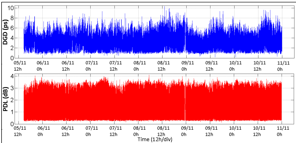
Figure 3.5 Courbes d'évolution temporelle des valeurs de DGD et des valeurs de PDL mesurées à chaque milliseconde par le transpondeur cohérent
