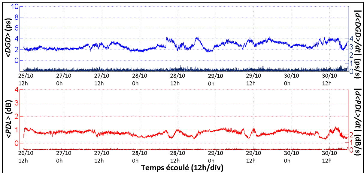
Figure 3.7 Évolution temporelle des valeurs de \langle DGD \rangle , de \left| \frac{d\langle DGD \rangle}{dt} \right| , de \langle PDL \rangle et de \left| \frac{d\langle PDL \rangle}{dt} \right| à chaque minute sur le lien optique cohérent du réseau Canarie
