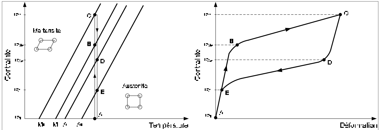
Figure 1.14 Chargement thermomécanique permettant d'obtenir l'effet superélastique Adaptée de Brailovski et al., (2003)
