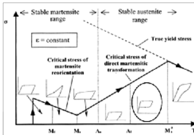
Figure 1.15 Diagramme d'état d'un alliage à mémoire de forme Ti-Ni Comportement superélastique encerclé Tirée de Brailovski et al., (2003)
