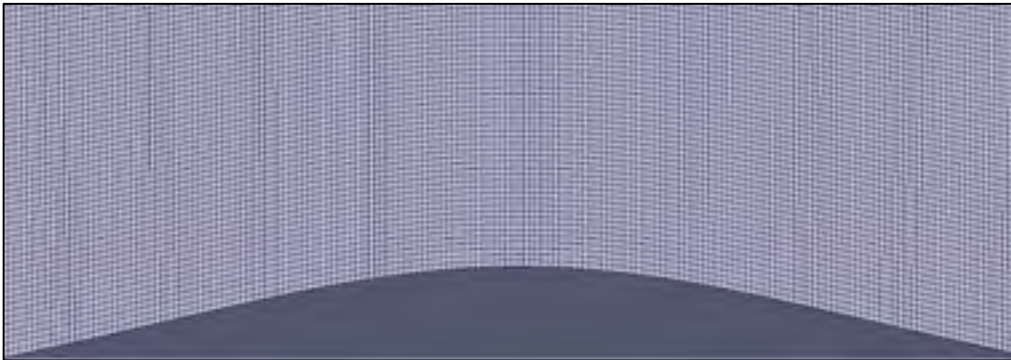
Figure 5.11 : Maillage proche de la surface de la colline
