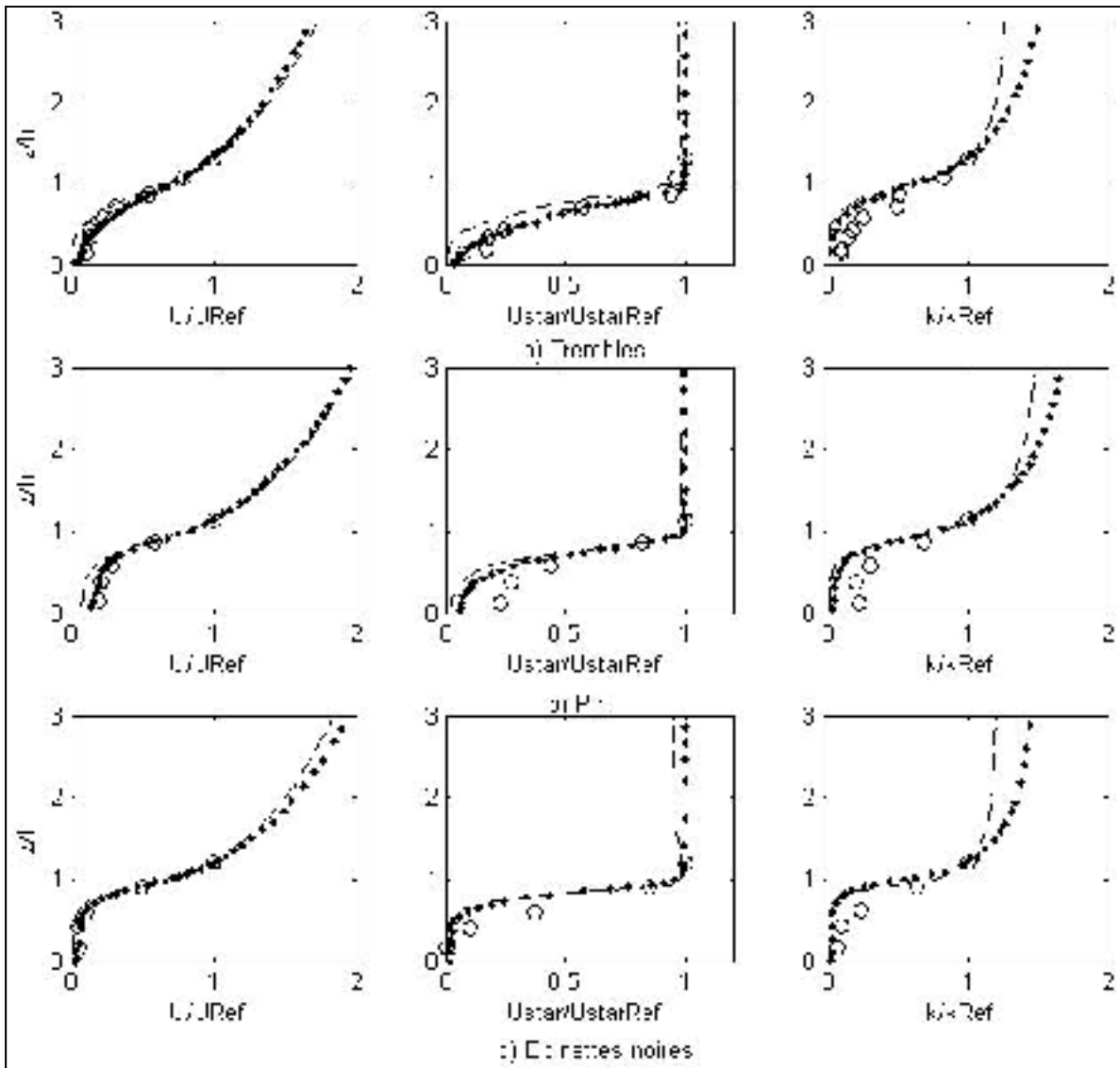
Figure 4.12: Comparaison entre les profils numériques calculés par le modèle k-\epsilon (trait interrompu), le modèle k-\epsilon de Dalpé et Masson (2008) (points) et les mesures expérimentales (cercles) pour la vitesse, la vitesse locale de friction et l'énergie cinétique turbulente pour les trois types de forêts proche de la surface
