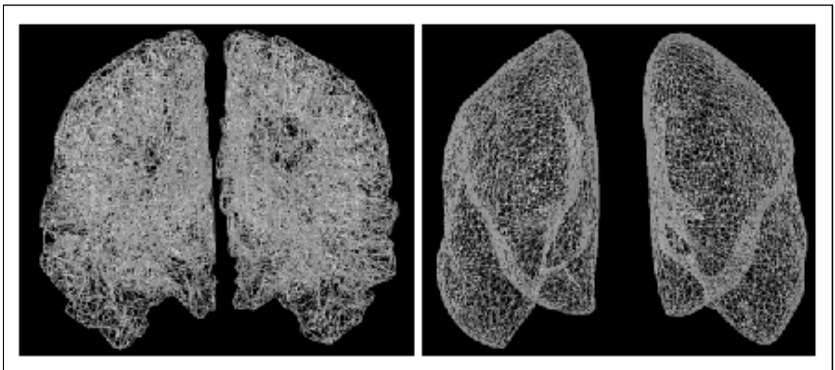
Figure 2.1 Exemple d'un maillage de cortex vu de face contenant 8004 sources. À gauche, le cortex utilisé et à droite, ce même cortex, mais « gonflé » pour faciliter la visualisation
