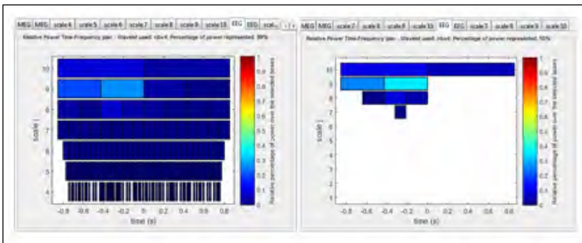
Figure 3.27 Plan T-S avec respectivement 99% et 50% de la puissance du signal d'intérêt. La couleur des boîtes est différente entre les deux plans, puisque la puissance totale du signal gardé n'est plus la même
