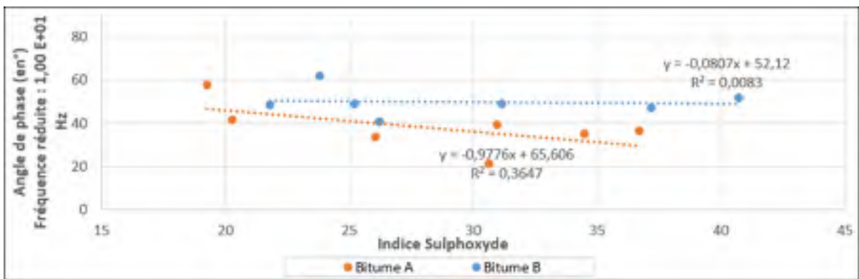
Figure-A VI-6 Angle de phase en fonction de l'indice sulphoxyde – Fréquence : 10 Hz
