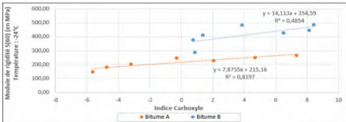
Figure 5.14 Module de rigidité S(60) à -24^\circ\text{C} en fonction de l'indice carboxyle
