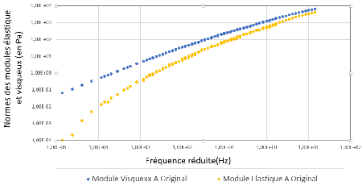
Figure 3.13 Module élastique et module visqueux du « Bitume A Original » à T_{ref} = 25^{\circ}\text{C}
