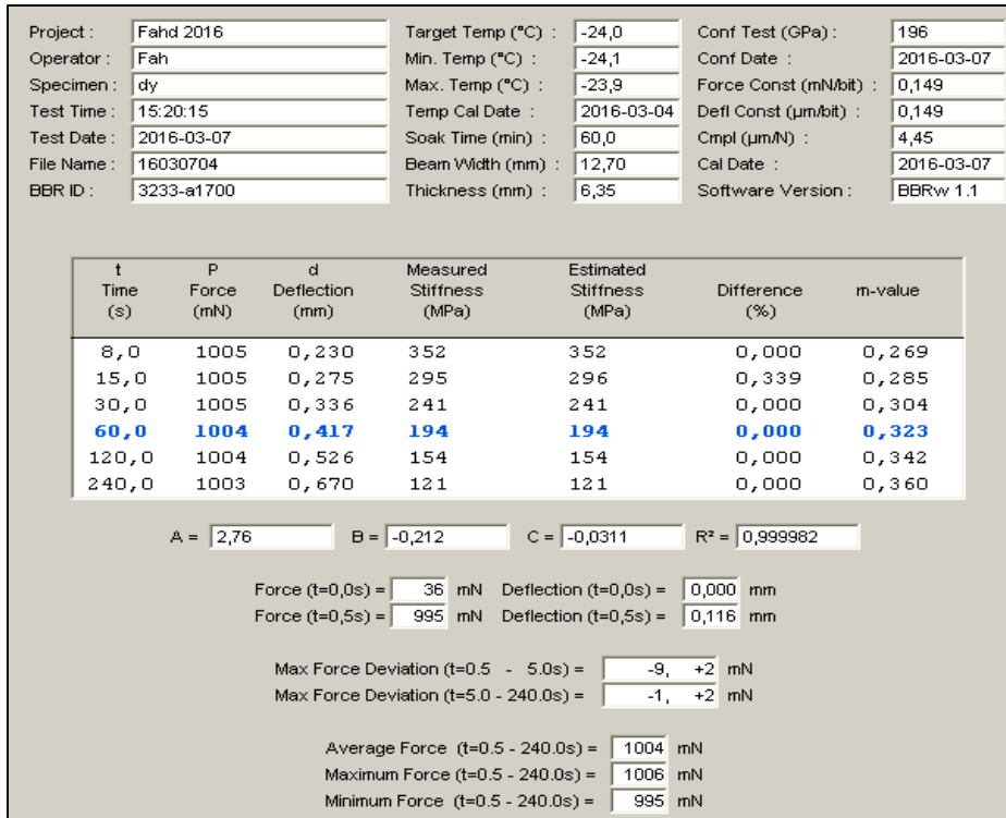
Figure-A III-10 Essai BBR du « Bitume A RTFO 85 min » à -24°C n°1
