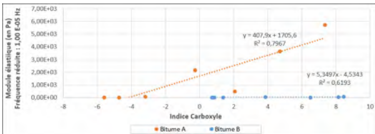
Figure 5.7 Module élastique en fonction de l'indice carboxyle – Fréquence : 0,00001 Hz
