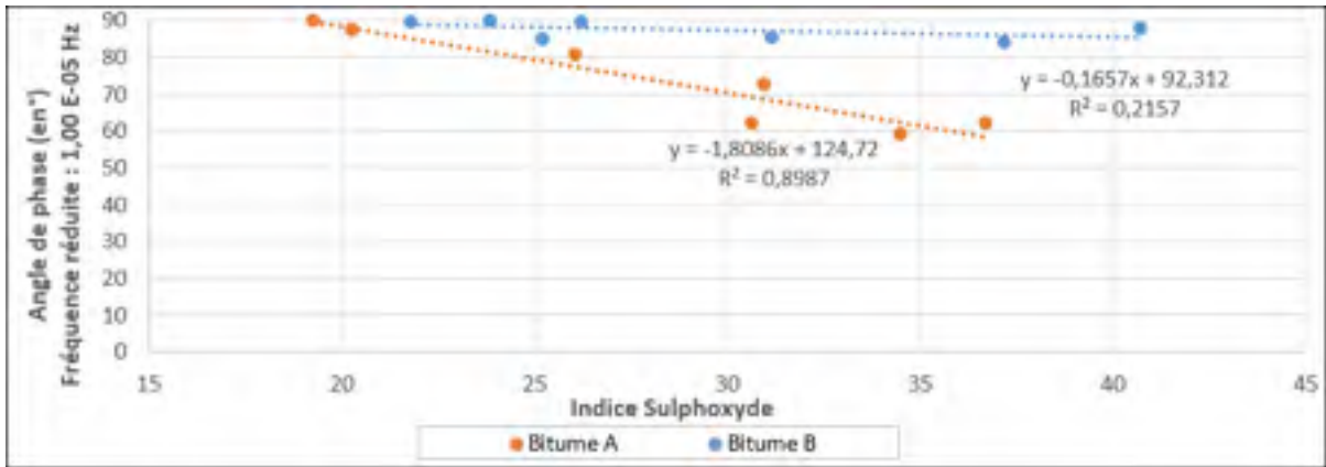
Figure-A VI-4 Angle de phase en fonction de l'indice sulphoxyde – Fréquence : 0,00001 Hz
