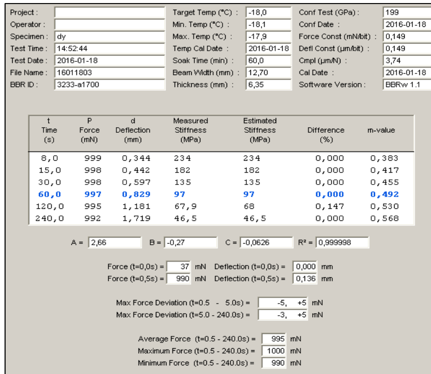
Figure-A III-45 Essai BBR du « Bitume B Original » à -18°C n°3
