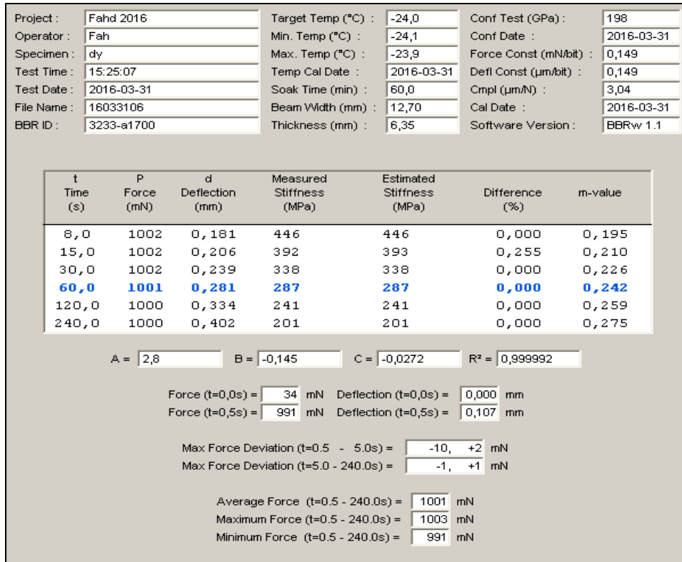
Figure-A III-42 Essai BBR du « Bitume A PAV 40 heures » à -24°C n°3
