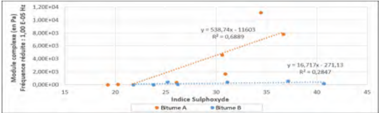
Figure-A VI-1 Module complexe en fonction de l'indice sulphyde – Fréquence : 0,00001 Hz
