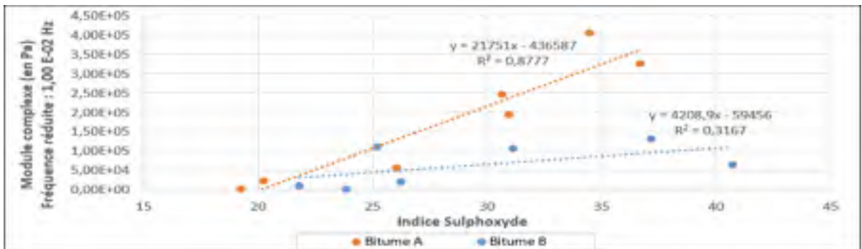
Figure-A VI-2 Module complexe en fonction de l'indice sulphyde – Fréquence : 0,01 Hz
