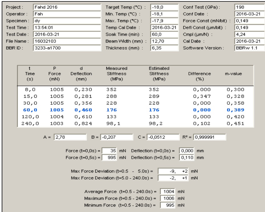
Figure-A III-57 Essai BBR du « Bitume B RTFO 150 min » à -18°C n°3
