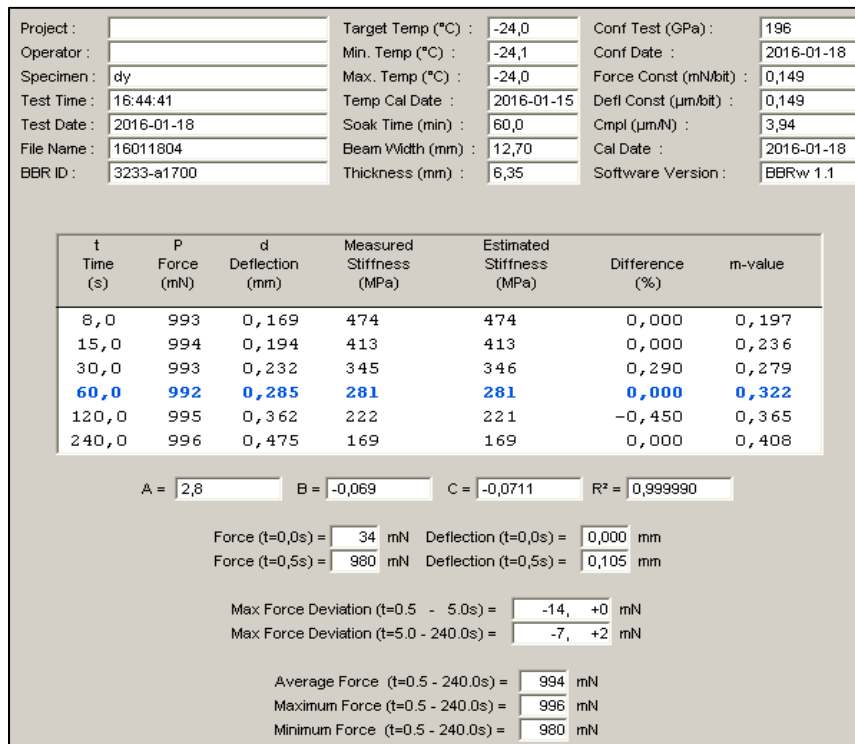
Figure-A III-46 Essai BBR du « Bitume B Original » à -24°C n°1
