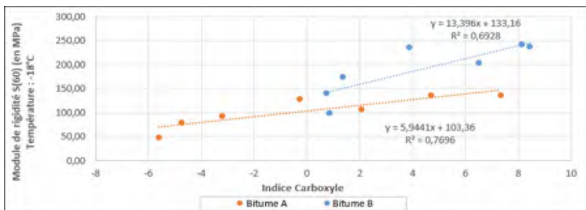
Figure 5.13 Module de rigidité S(60) à -18^\circ\text{C} en fonction de l'indice carboxyle
