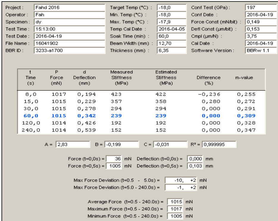
Figure-A III-73 Essai BBR du « Bitume B PAV 30 heures » à -18°C n°2
