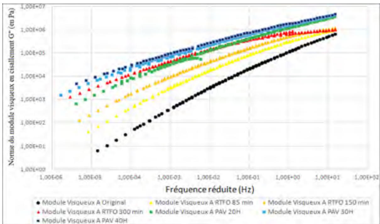
Figure 3.17 Comparatif des modules visqueux des différents états du bitume A à T_{ref} = 25^{\circ}C
