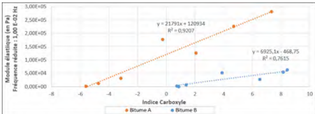
Figure 5.8 Module élastique en fonction de l'indice carboxyle – Fréquence : 0,01 Hz
