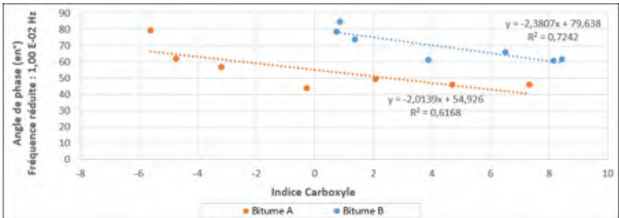
Figure 5.5 Angle de phase en fonction de l'indice carboxyle – Fréquence : 0,01 Hz
