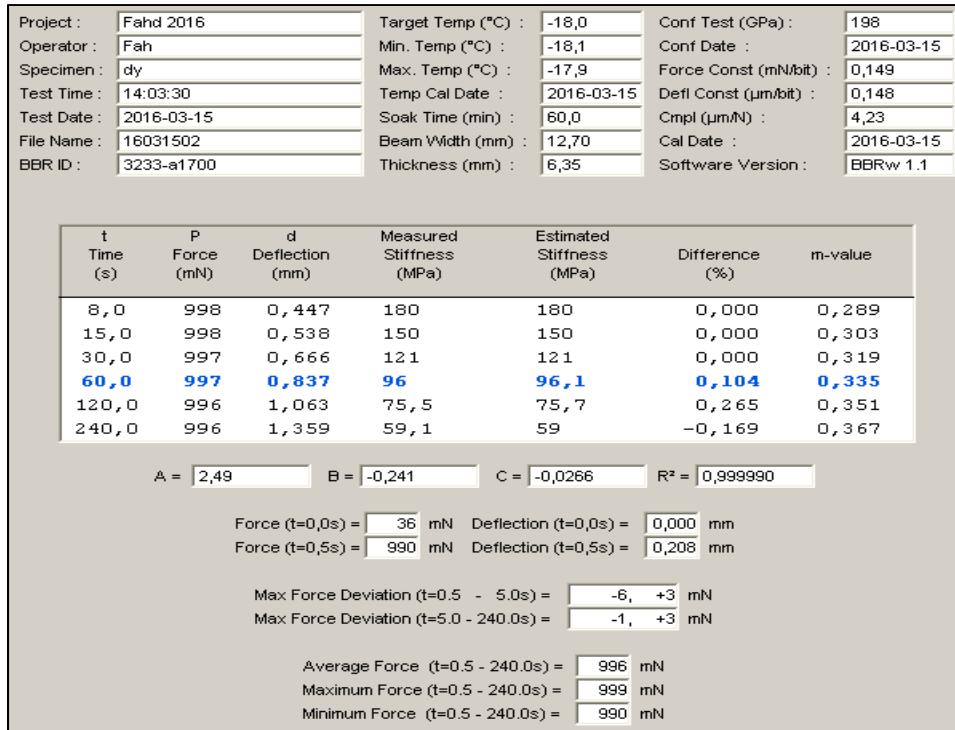
Figure-A III-14 Essai BBR du « Bitume A RTFO 150 min » à -18°C n°2
