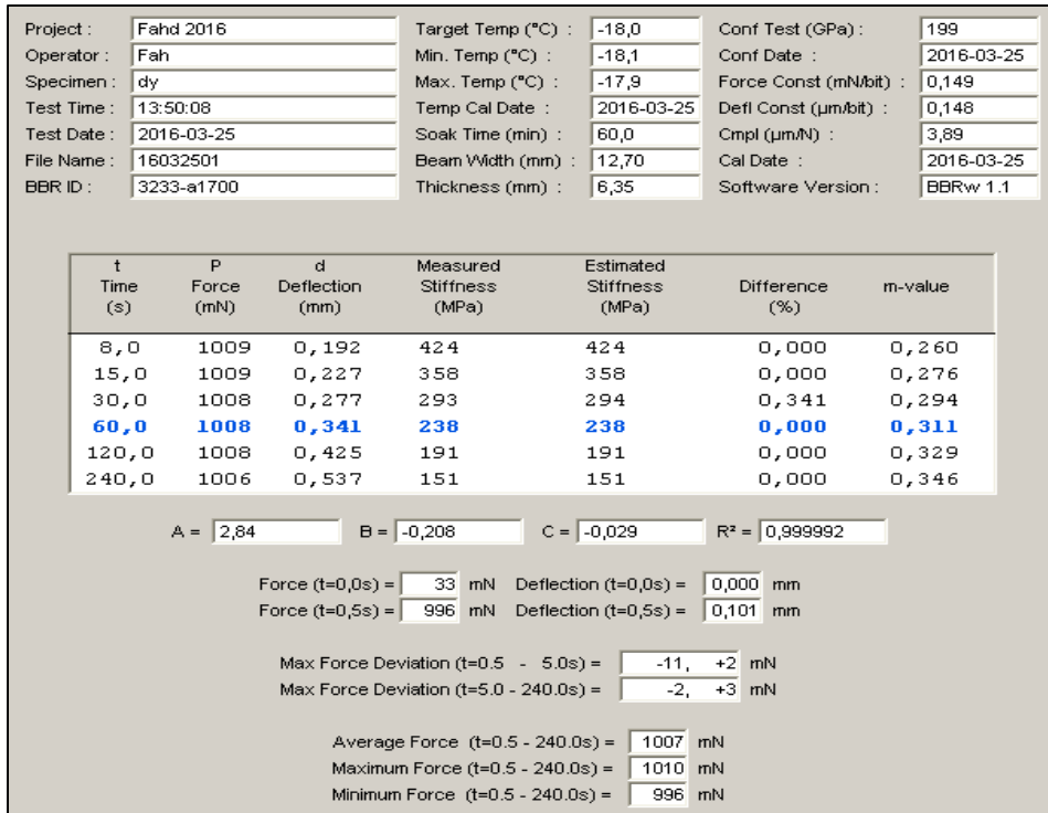
Figure-A III-61 Essai BBR du « Bitume B RTFO 300 min » à -18°C n°1
