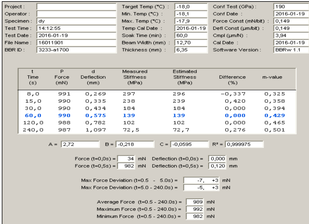
Figure-A III- Essai de l'essai BBR du « Bitume B RTFO 85 min » à -18°C n°1
