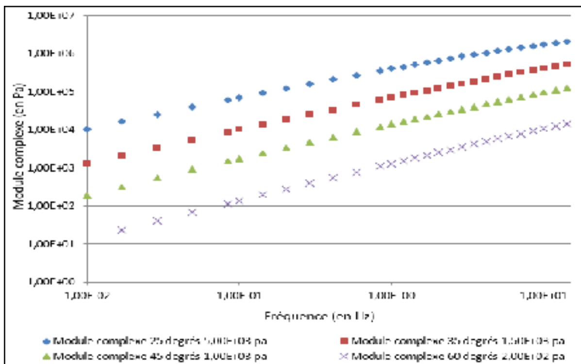
Figure-A II-34 Superposition des isothermes de module complexe du Bitume B RTFO 85 min
