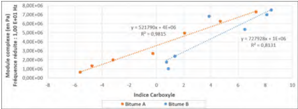
Figure 5.3 Module complexe en fonction de l'indice carboxyle – Fréquence : 10 Hz
