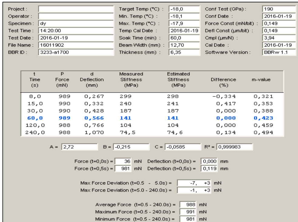
Figure-A III-50 Essai BBR du « Bitume B RTFO 85 min » à -18°C n°2
