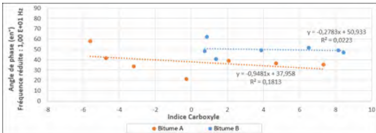
Figure 5.6 Angle de phase en fonction de l'indice carboxyle – Fréquence : 10 Hz
