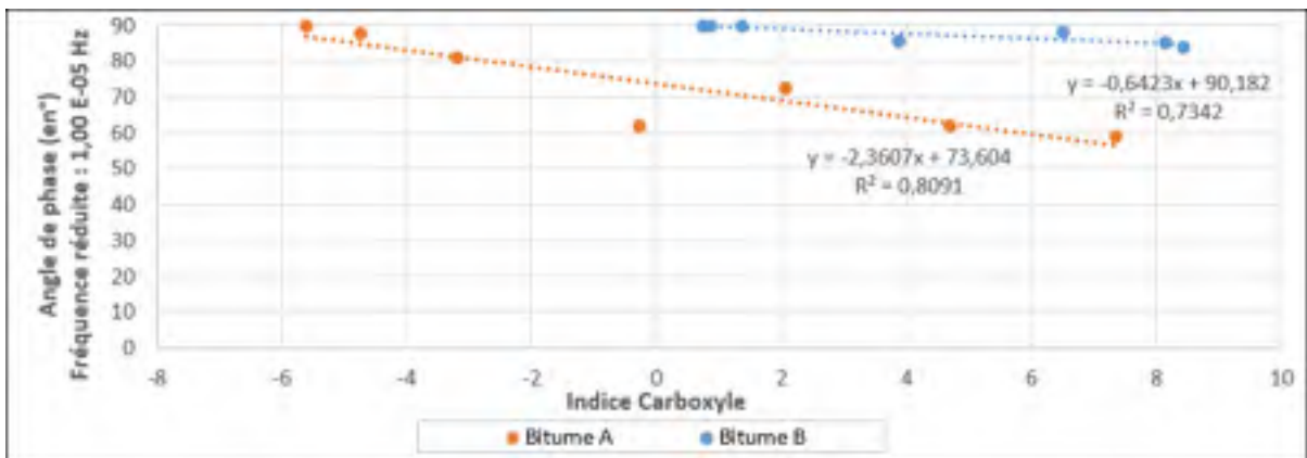
Figure 5.4 Angle de phase en fonction de l'indice carboxyle – Fréquence : 0,00001 Hz
