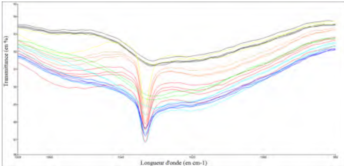
Figure 4.6 Pic sulphoxyde des différents états du bitume A
