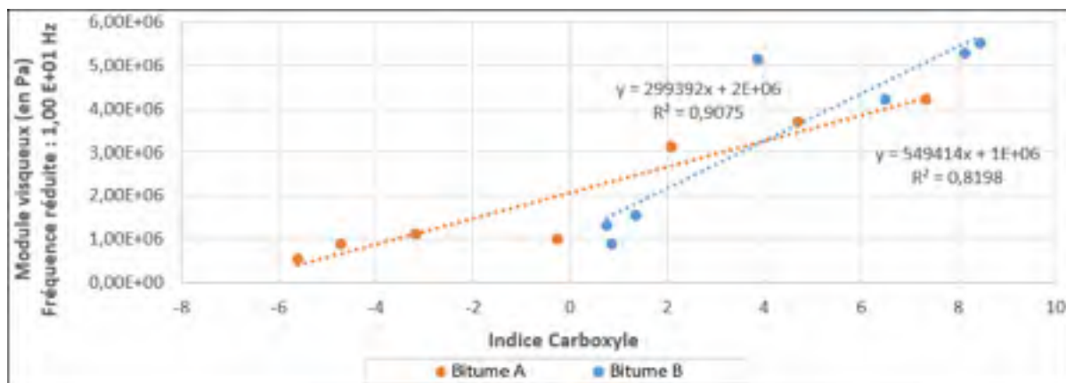
Figure 5.12 Module visqueux en fonction de l'indice carboxyle – Fréquence : 10 Hz
