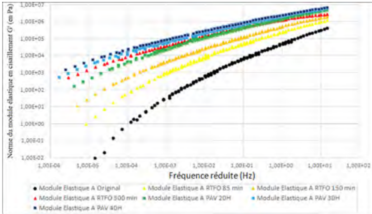
Figure 3.16 Comparatif des modules élastiques des différents états du bitume A à T_{ref} = 25^{\circ}C
