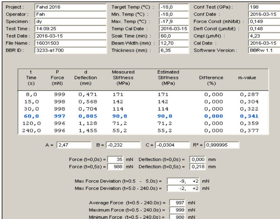
Figure-A III-15 Essai BBR du « Bitume A RTFO 150 min » à -18°C n°3
