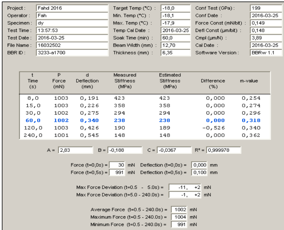
Figure-A III-62 Essai BBR du « Bitume B RTFO 300 min » à -18°C n°2
