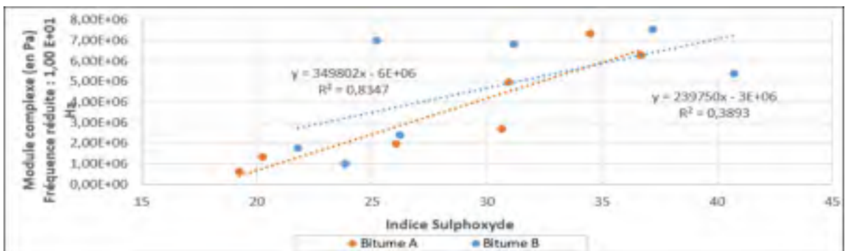
Figure-A VI-3 Module complexe en fonction de l'indice sulphyde – Fréquence : 10 Hz
