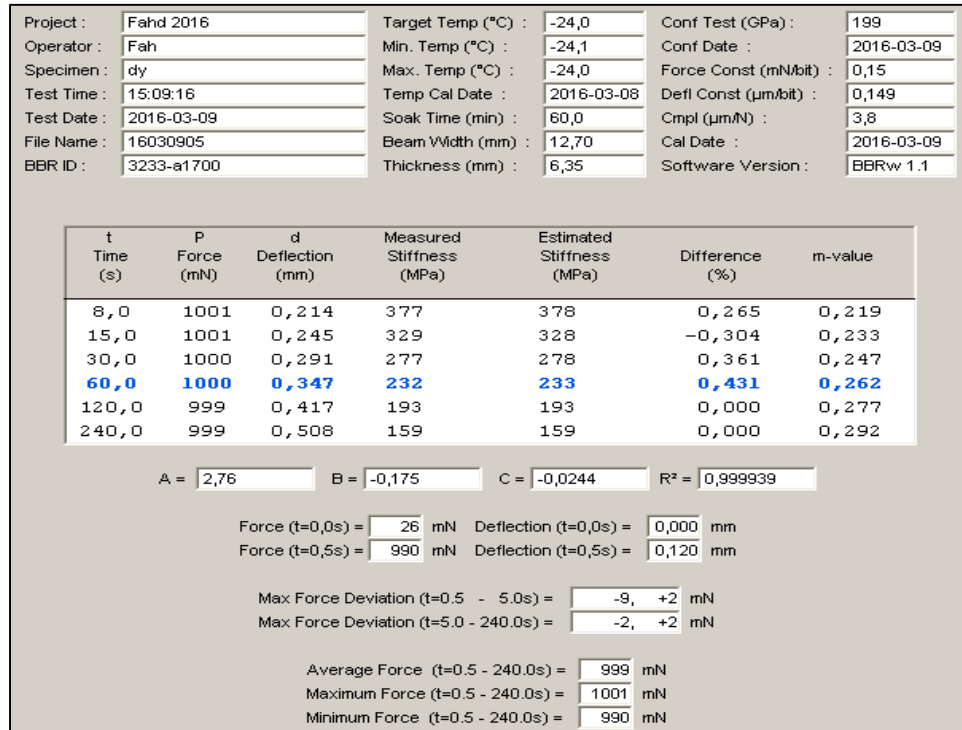
Figure-A III-29 Essai BBR du « Bitume A PAV 20 heures » à -24°C n°2
