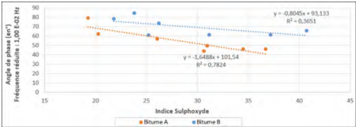
Figure-A VI-5 Angle de phase en fonction de l'indice sulphoxyde – Fréquence : 0,01 Hz
