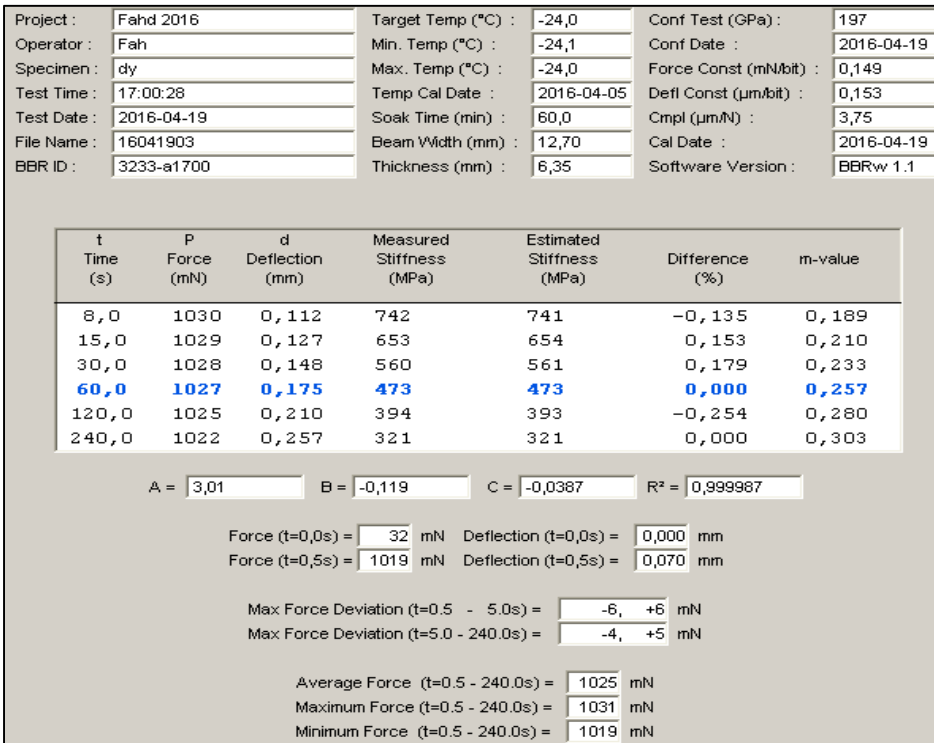
Figure-A III-74 Essai BBR du « Bitume B PAV 30 heures » à -24°C n°1
