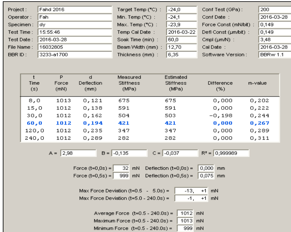
Figure-A III-71 Essai BBR du « Bitume B PAV 20 heures » à -24°C n°2
