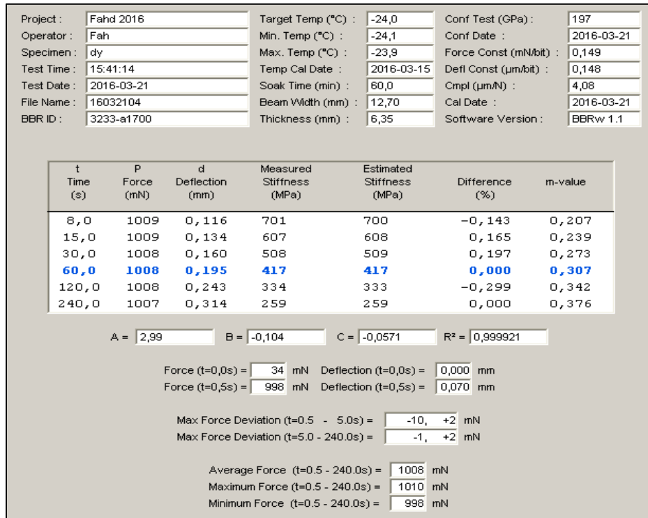
Figure-A III-58 Essai BBR du « Bitume B RTFO 150 min » à -24°C n°1
