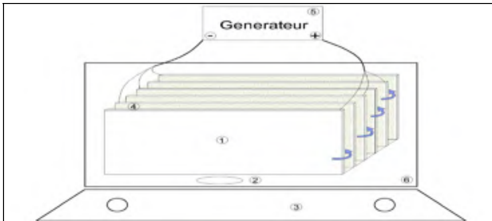
Figure 2.2 : Dispositif expérimental
