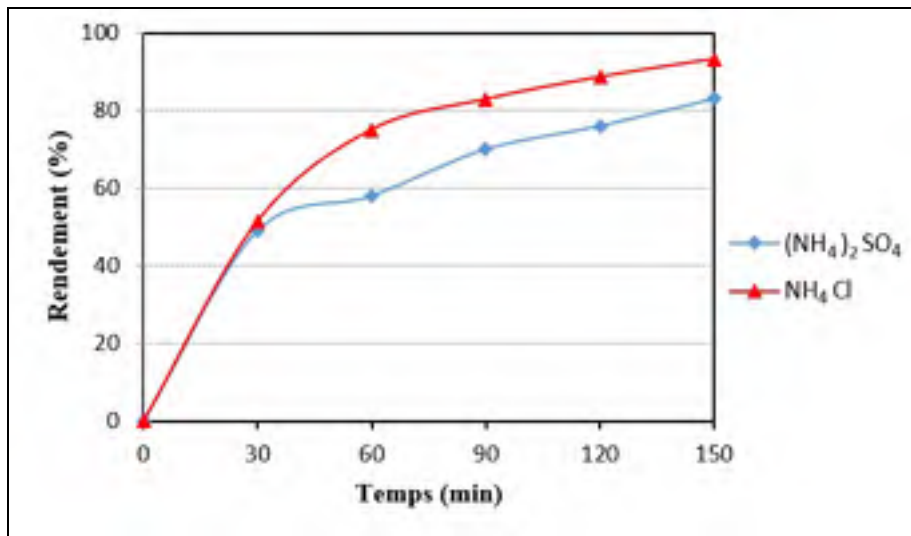
Figure 3.11 : Évolution dans le temps du rendement d'électro-conversion de l'azote ammoniacal. V = 1 \text{ L} ; masse de zéolite = 150 g; [\text{NH}_4^+]_0 = 700 \text{ mg-N/L} ; pH initial = 7,5; D = 4 \text{ mm} ; 6 électrodes en acier : 15,2 cm x 7,62 cm x 0,03 cm; U = 5,0 \text{ V} ; densité de courant : 17,2 mA/cm 2 .
