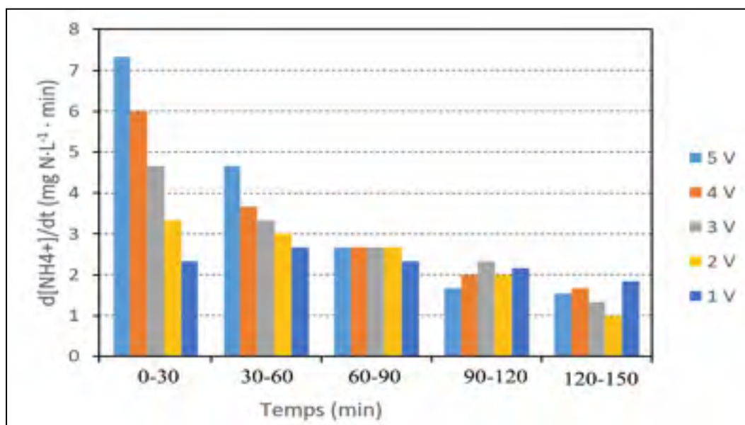
Figure 3.2 : Variation de la vitesse d'électro-conversion de l'azote ammoniacal au cours du temps. V = 1 \text{ L} ; masse de zéolite = 150 g (dans le cas b); [\text{NH}_4^+]_0 = 700 \text{ mg-N/L} ; pH initial = 7,5; D = 4 \text{ mm} ; 6 électrodes en cuivre-nickel (70 %-30 %): 15,2 cm x 7,62 cm x 0,03 cm; U : 1,0 \text{ à } 5,0 \text{ V} ; densité courant : 1,72 à 17,2 mA/cm 2 .
