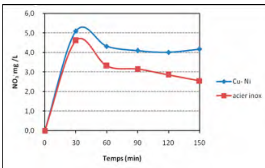
Figure 4.2 Variation concentration des nitrates pour les deux sources d'ammonium au cours de temps. V = 1 L; masse de zéolite = 150 g; [NH_4^+]_0 = 700 mg-N/L; pH initial = 7,5; D = 4 mm; 6 électrodes métalliques : 15,2 cm x 7,62 cm x 0,03 cm; U = 5,0 V; densité de courant : 17,2 mA/cm 2 .
