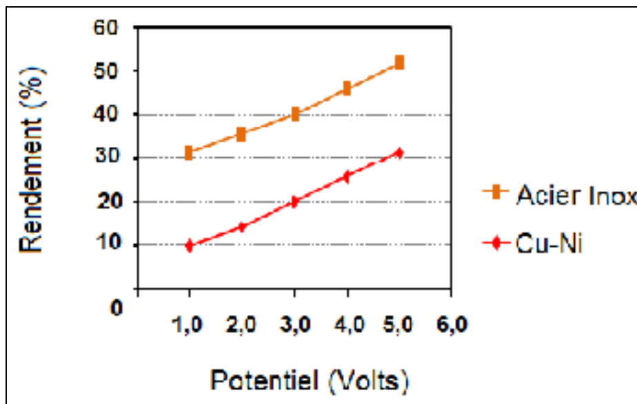
Figure 4.1 : Comparaison des rendements d'électro-conversion de l'azote ammoniacal obtenus pour les deux types d'électrodes étudiées. V = 1 L; masse de zéolite = 150 g; [\text{NH}_4^+]_0 = 700 mg-N/L; pH initial = 7,5; D = 4 mm; 6 électrodes métalliques : 15,2 cm x 7,62 cm x 0,03 cm; U = 1,0 à 5,0 V; densité de courant : 1,72 à 17,2 mA/cm 2 .
