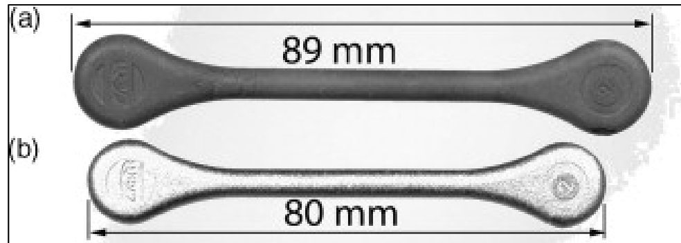
Figure 1.8 (a) pièce déliantée (avant frittage) et (b) pièce après frittage (Obasi, Ferri, Ebel, & Bormann, 2010)
