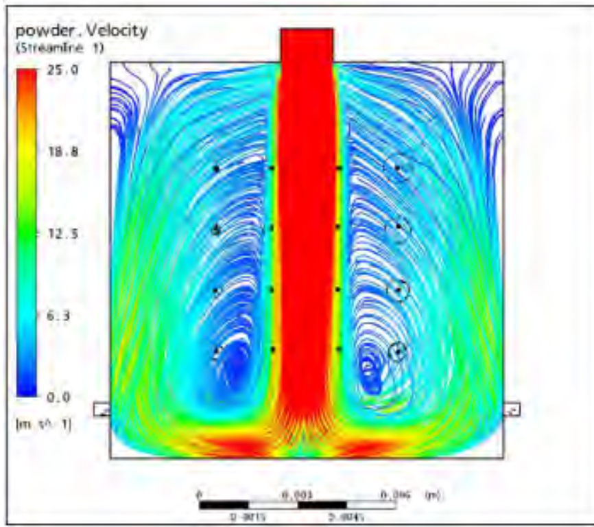
Figure 1.12 Détection de la vitesse des particules de la poudre (Yin et al., 2011)
