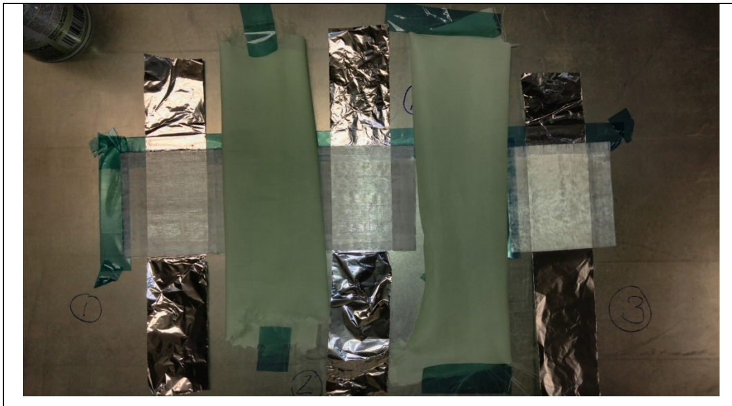
Figure-A I-1 Condensateurs de la série LAM_04 en Thinpreg 402, avant cuisson
