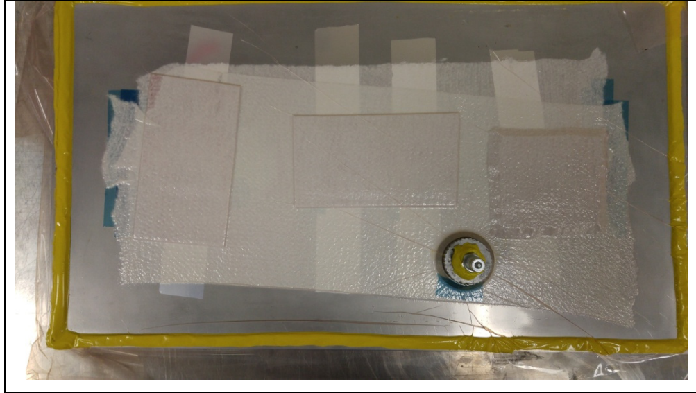
Figure 3.8 Moulage de condensateurs plats FM300 lors d'un essai de tenu du vide du sac
