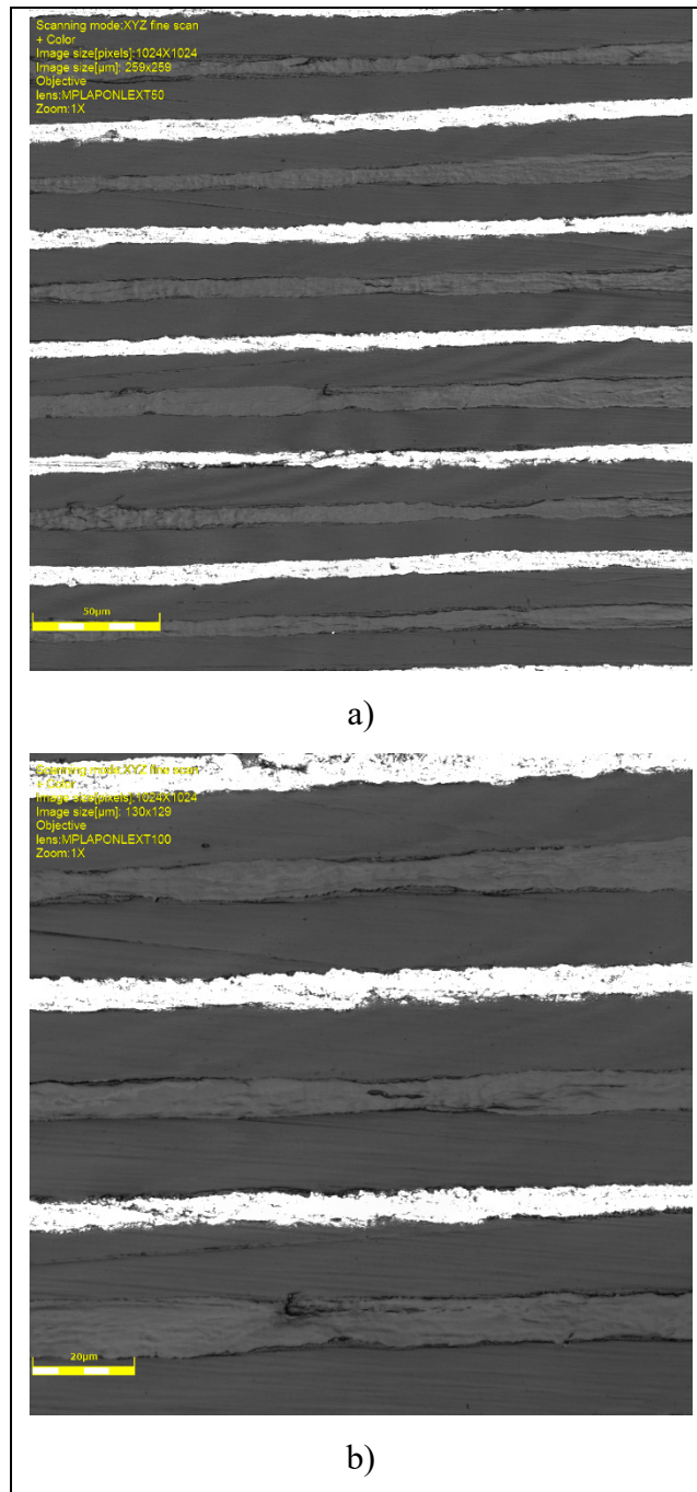
Figure 4.24 Coupe transversale de VPI 22 : a) à un grossissement de 500X et b) à un grossissement de 1000X
