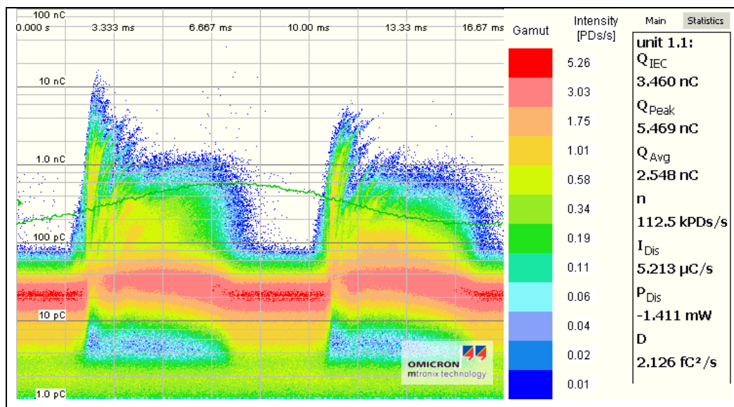
Figure-A III-4 Mesures de décharges partielles de VPI 23 à U_{\text{nominale}} = 1,5 \text{ kV} Le bruit de fond du montage avant mesure est inférieur à 9 pC
