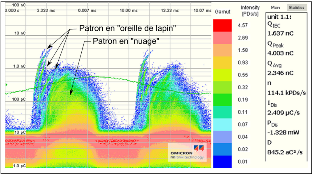
Figure 4.13 Mesures de décharges partielles de VPI 22 à U_{nominale} = 1,5 kV Le bruit de fond du montage avant mesure est inférieur à 6 pC
