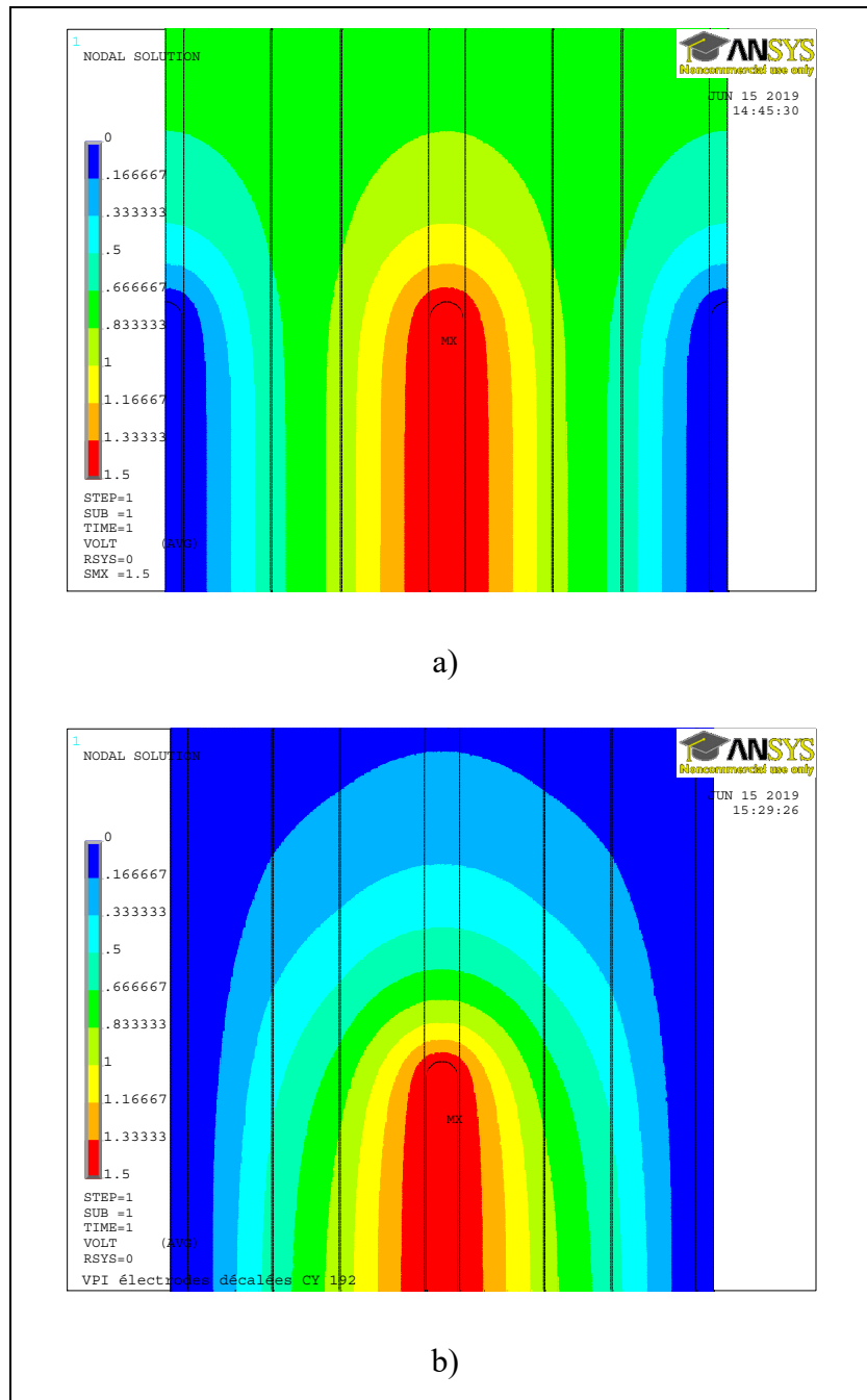
Figure 6.3 Distribution du potentiel électrostatique en kV pour a) des électrodes alignées, b) des électrodes décalées
