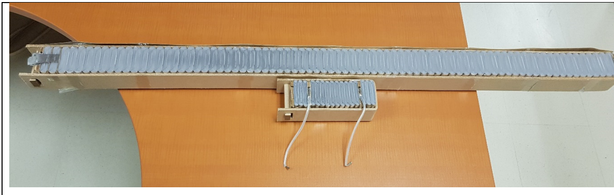
Figure 2.1 Photo de parties actives de condensateur haute tension
