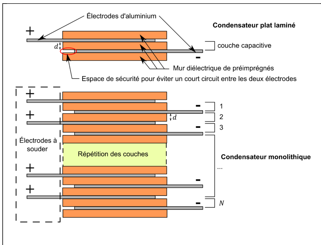
Figure 3.1 Condensateur monolithique formé de N couches capacitives
