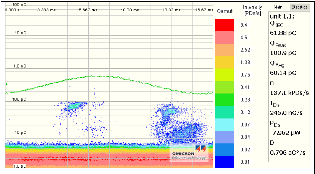
Figure 4.16 Mesures de décharges partielles de VPI 26 à U_{\text{nominale}} = 1,5 \text{ kV} Le bruit de fond du montage avant mesure est inférieur à 8 pC
