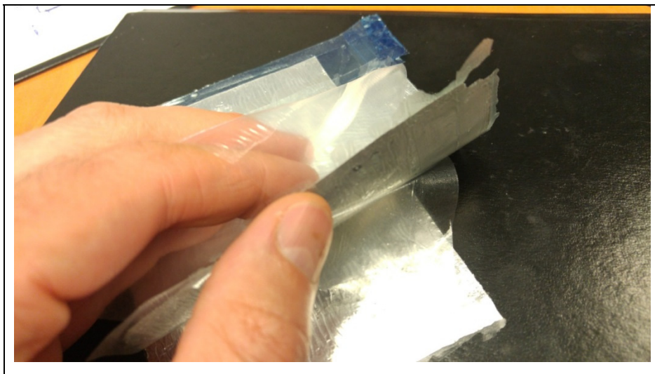
Figure 3.13 Délamination entre l'électrode d'aluminium et le film de polypropylène du condensateur LAM_06_D
