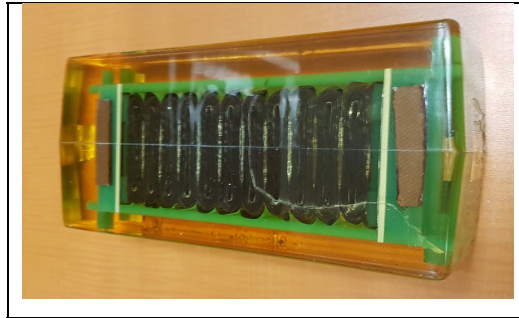
Figure 5.2 Fissure pénétrant dans la PA du prototype 1
