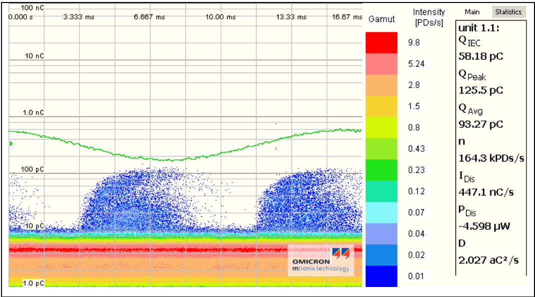
Figure 4.17 Mesures de décharges partielles de VPI 27 à U_{\text{nominale}} = 1,5 \text{ kV} Le bruit de fond du montage avant mesure est inférieur à 10 pC
