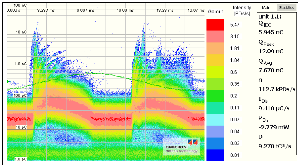
Figure-A III-5 Mesures de décharges partielles de VPI 25 à U_{\text{nominale}} = 1,5 \text{ kV} Le bruit de fond du montage avant mesure est inférieur à 8 pC
