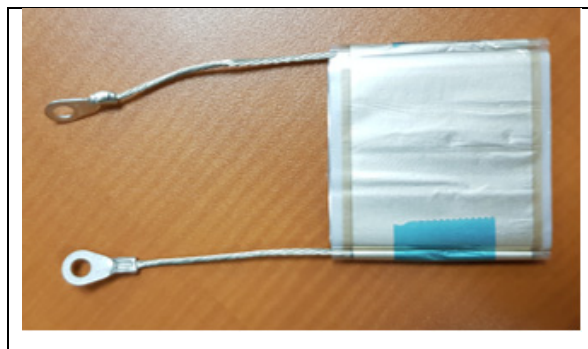
Figure 4.5 Enroulement capacitif avec ses connexions avant imprégnation
